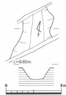
第2図 A区SD-1 平面・断面図(1/80)
