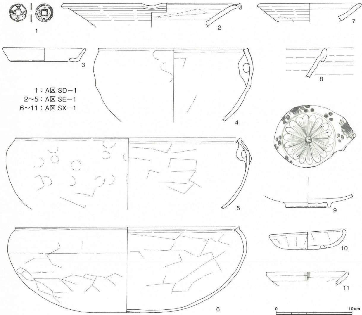
第4図 A区出土遺物（1/3）
