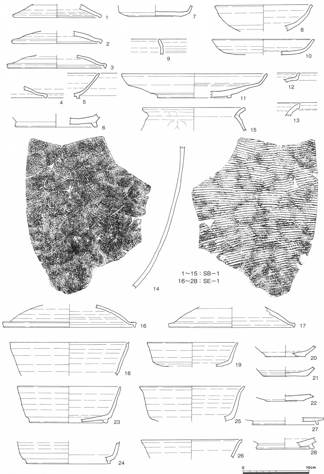
第11図 出土遺物-1 (1/3)
