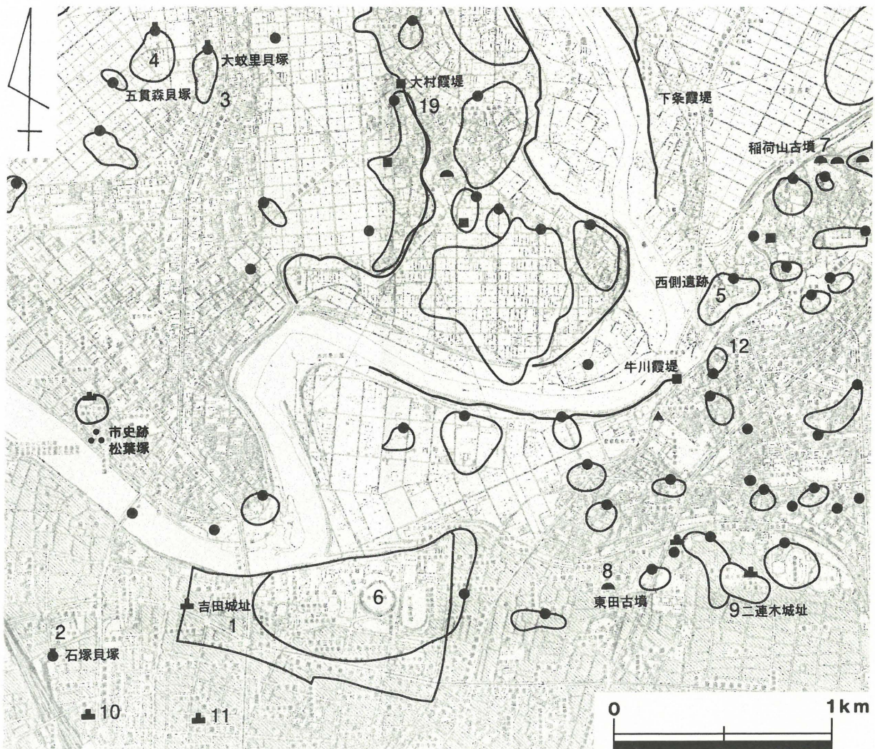
第2図 周辺の遺跡分布図 (1/25,000)
