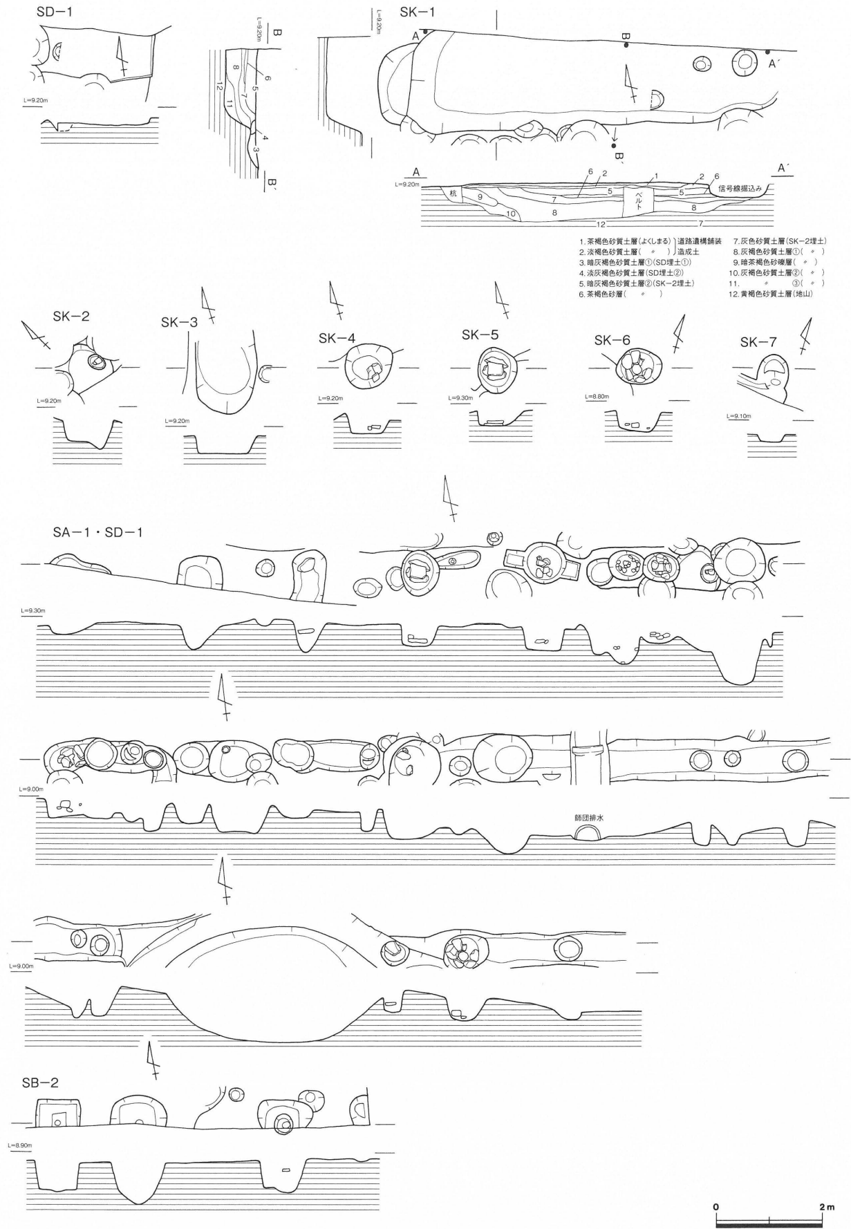
第9図 土坑・塀平面・断面図 (1/100)
