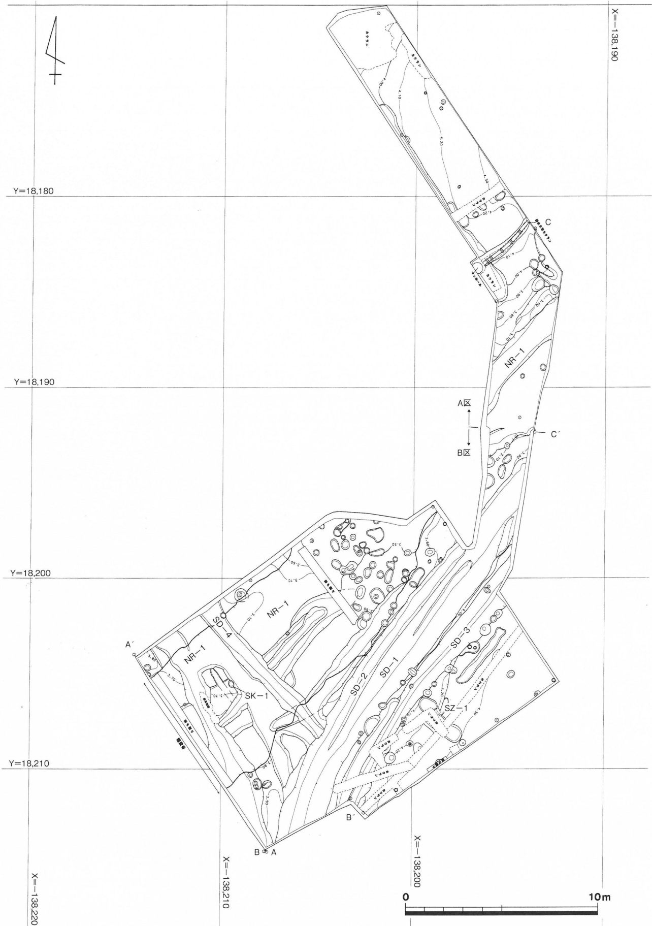
第4図 調査区平面図 (1/200)
