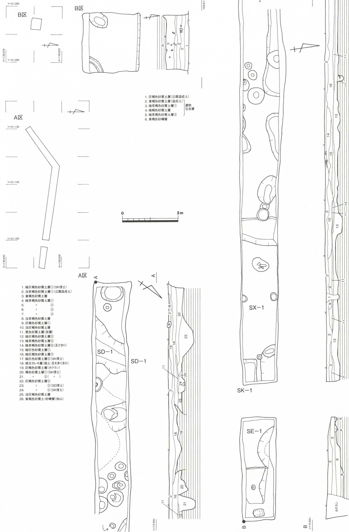
第3図 調査区平面・断面図 (1/80)
