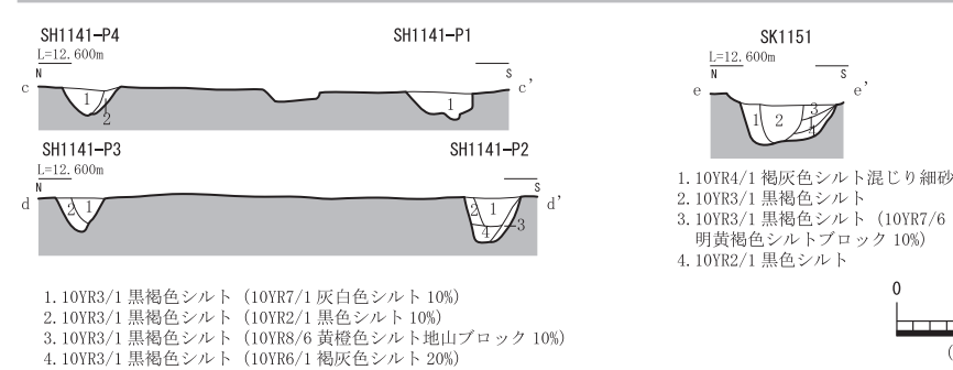
第81図 SH1141 断面図
