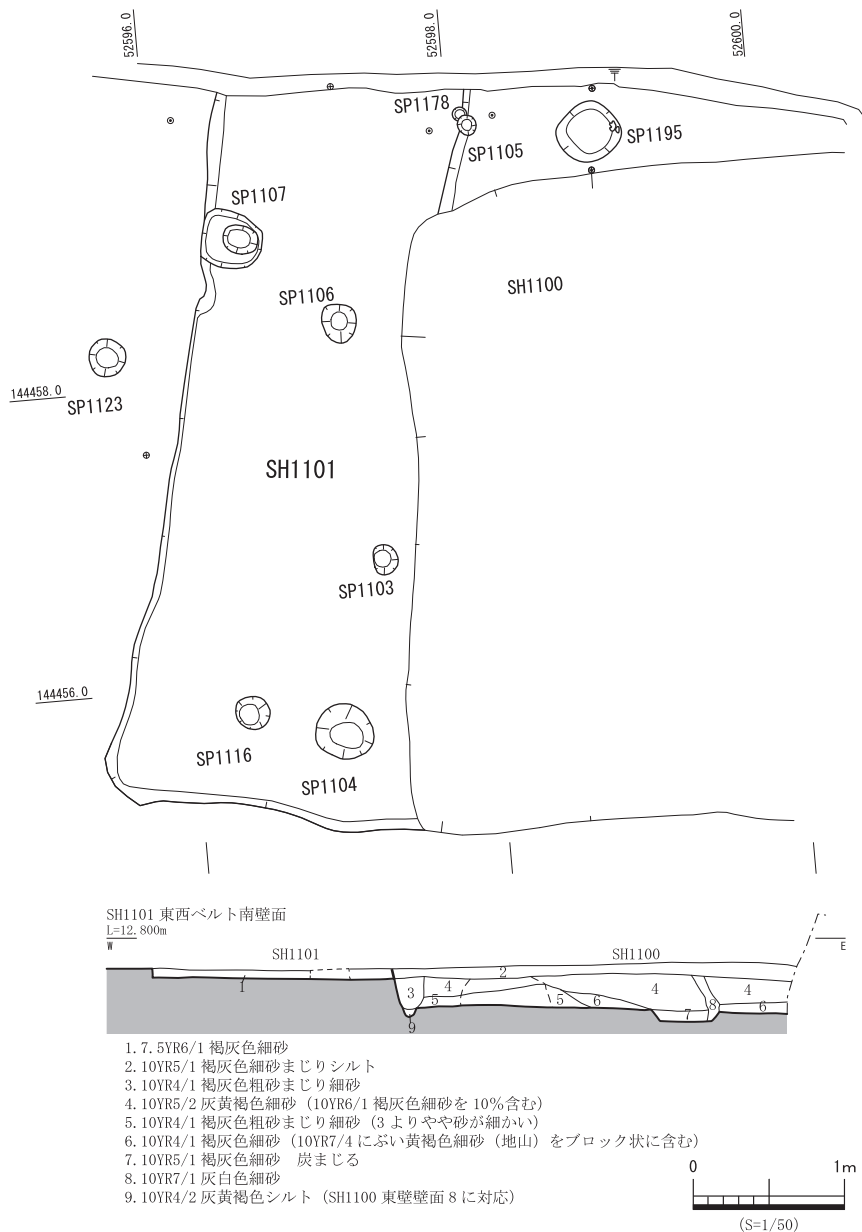
第73図 SH1101 平・断面図
