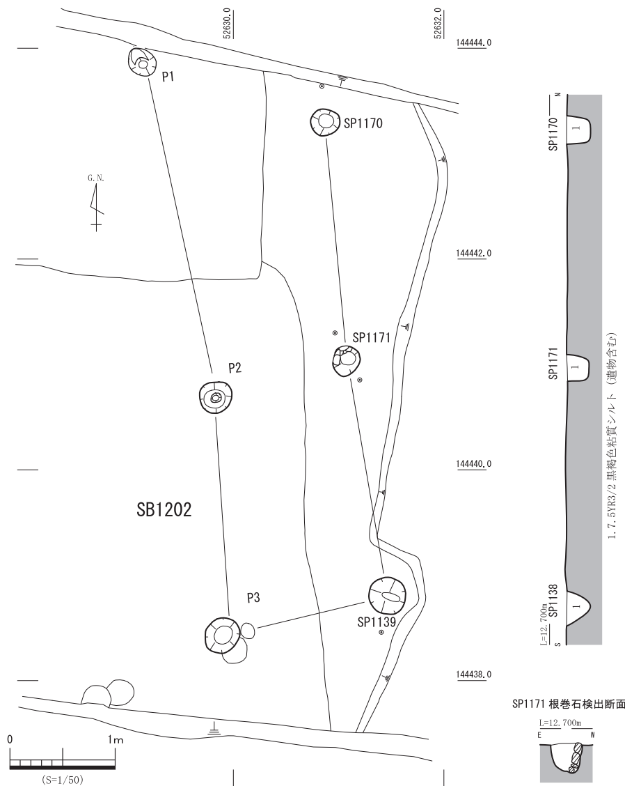
第90図 SB1202 平・断面図
