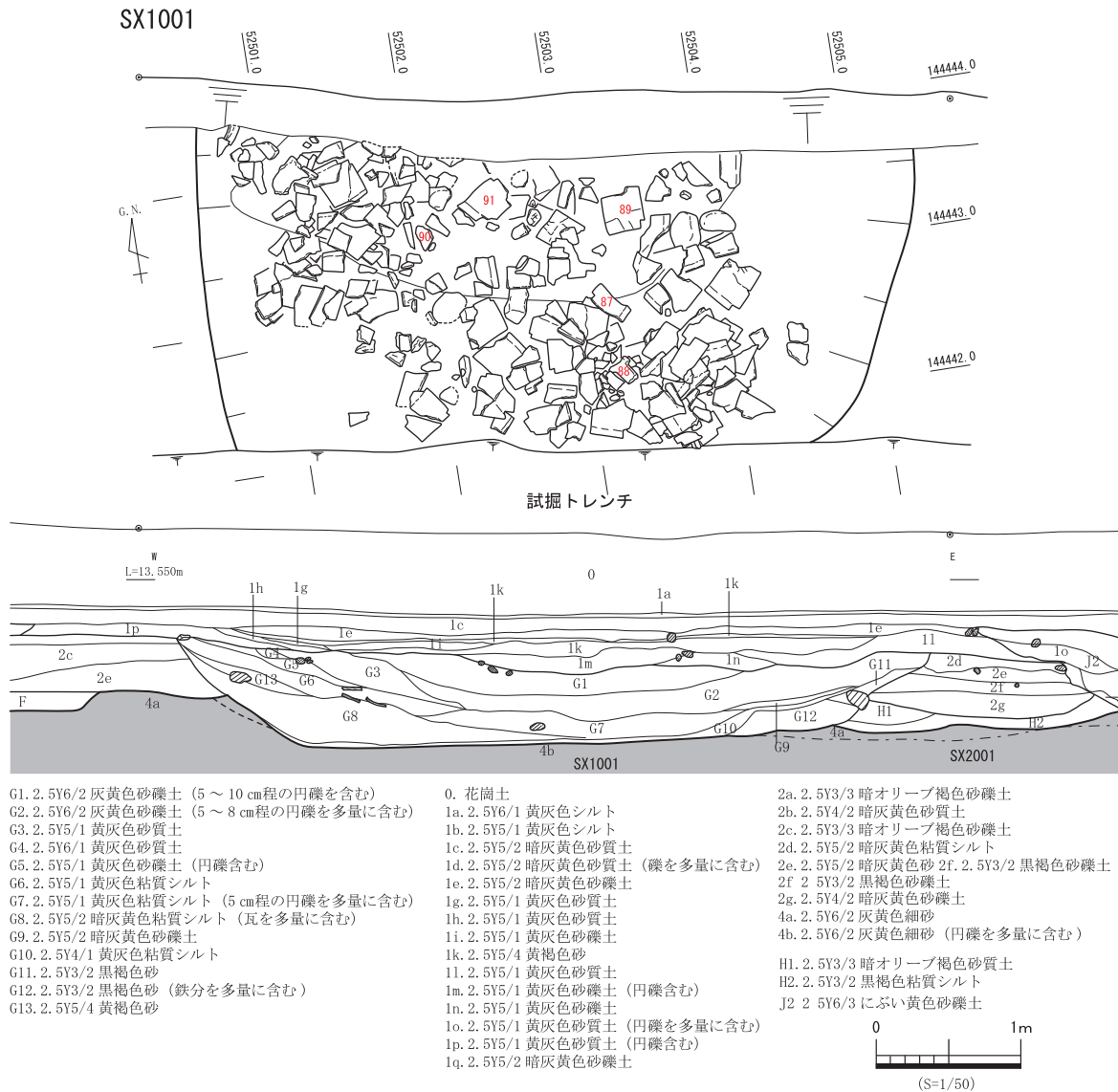
第 23 図 SX1001 平・断面図
