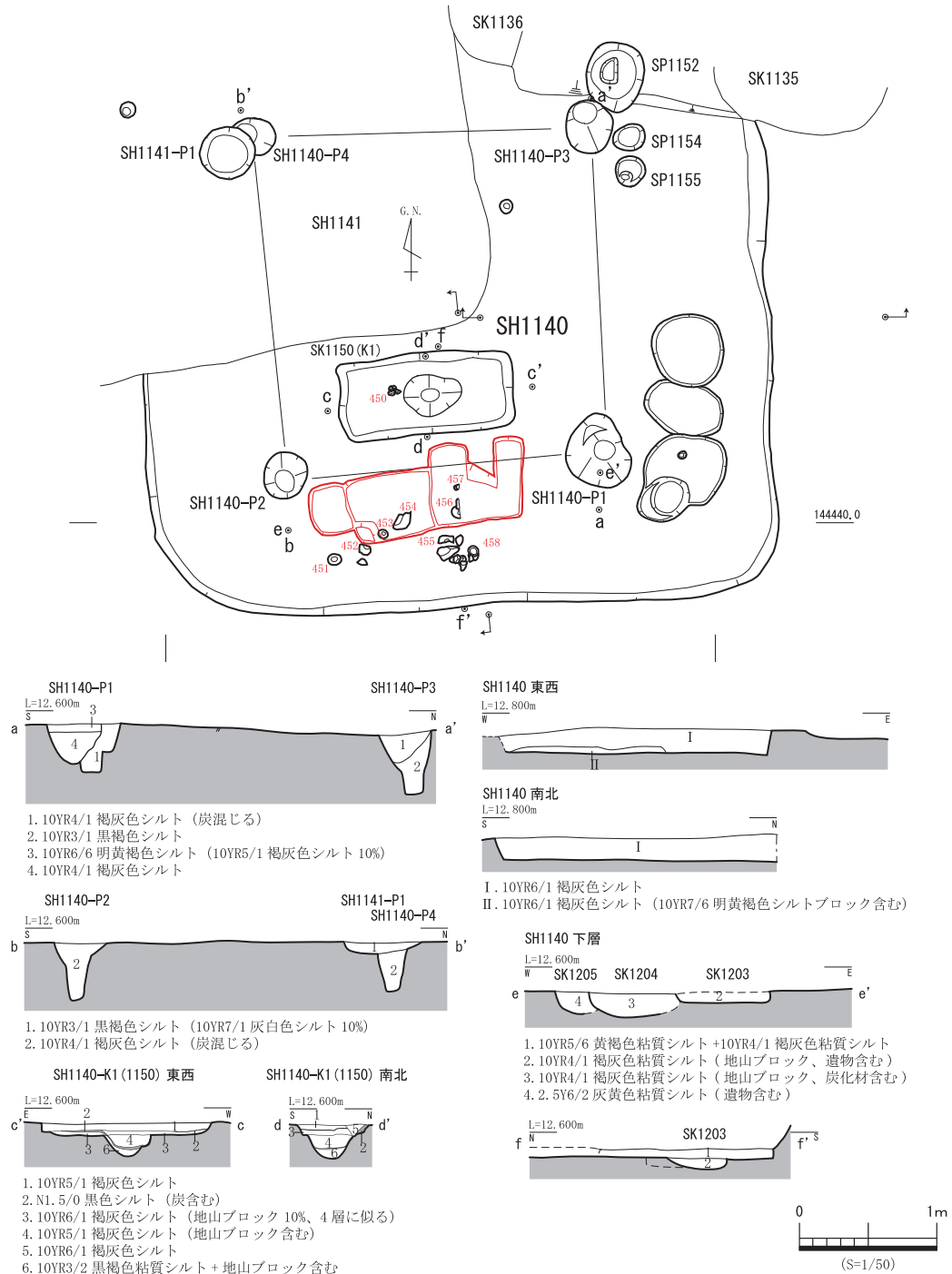
第 78 図 SH1140 平・断面図
