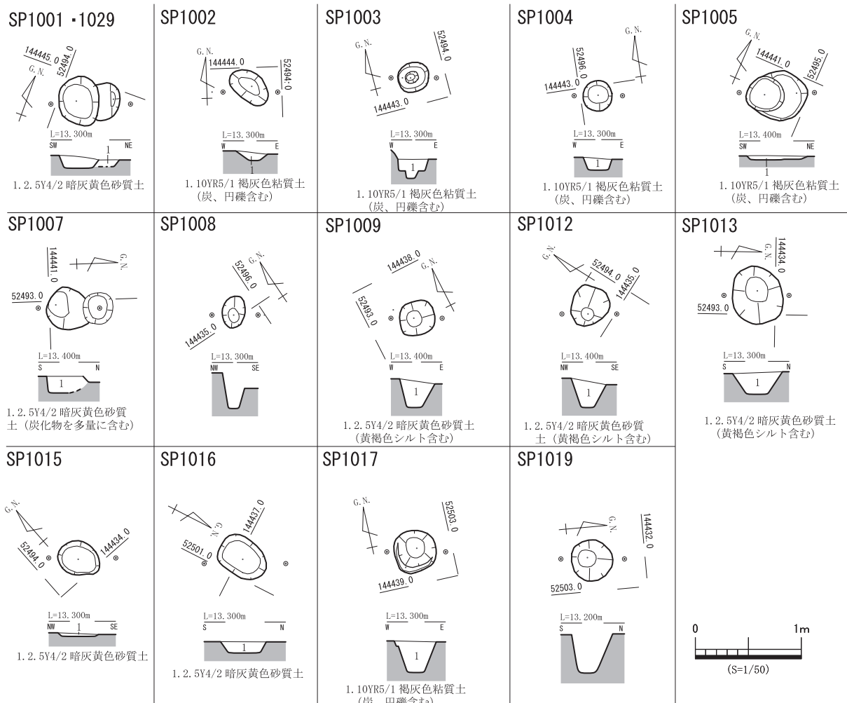
第 20 図 A-1SP 平・断面図①
