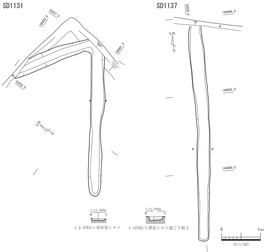
第 91 図 SD1131・1137 平・断面図
