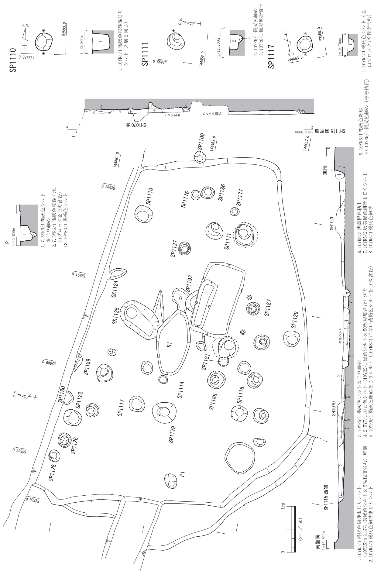
第74図 SH1115平・断面図
