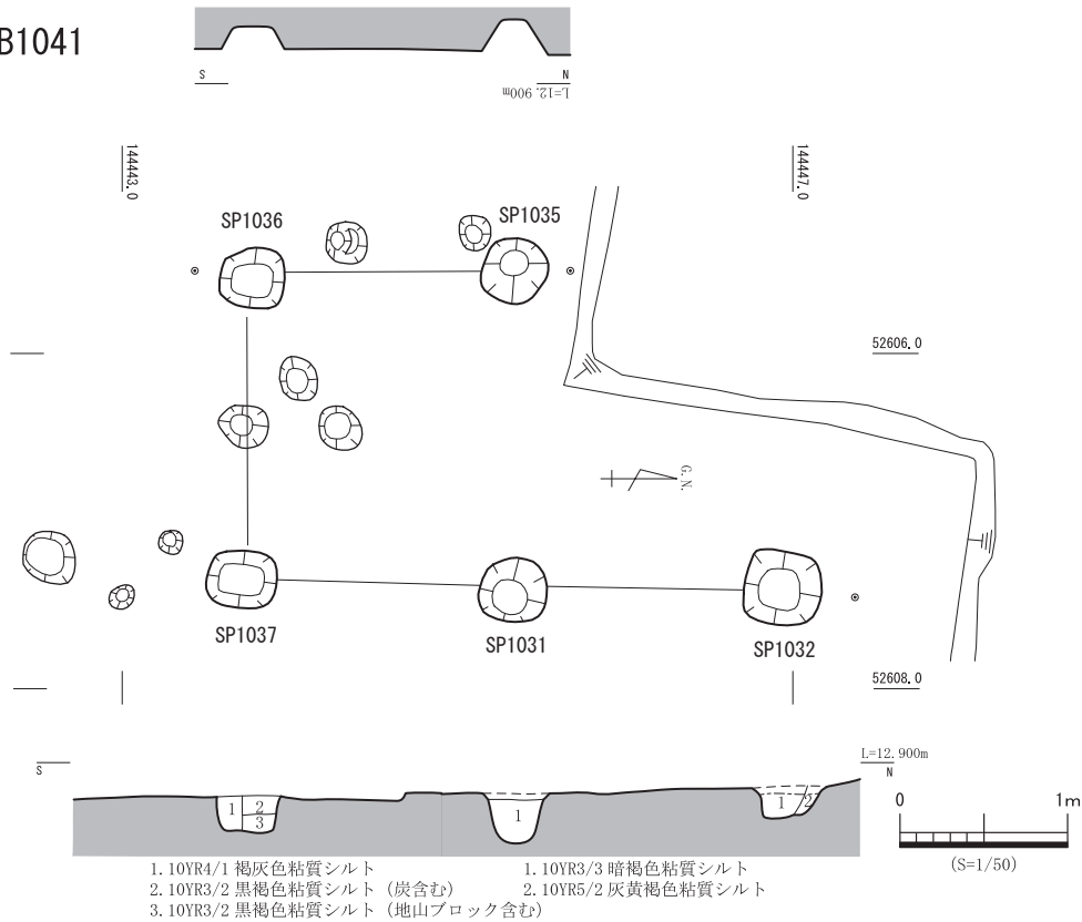
第 62 図 SB1041 平・断面図
