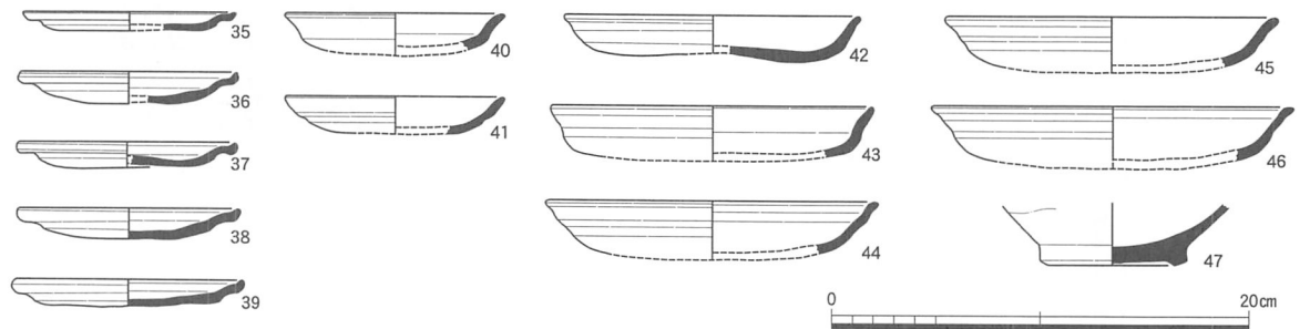
図40 SG1出土土器実測図(1:4)
