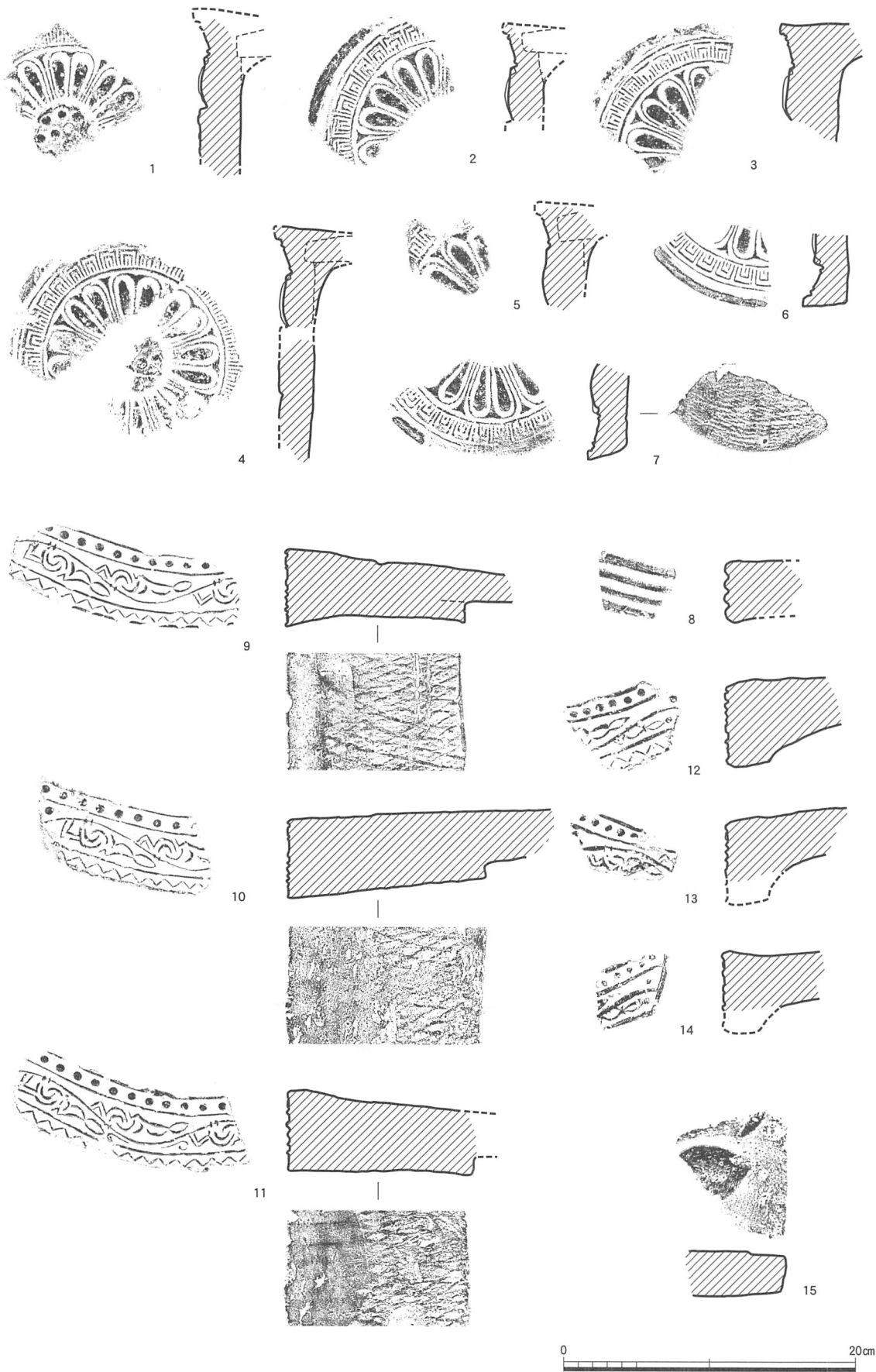
图8 軒瓦・鬼瓦拓影および実測図 (1:4)
