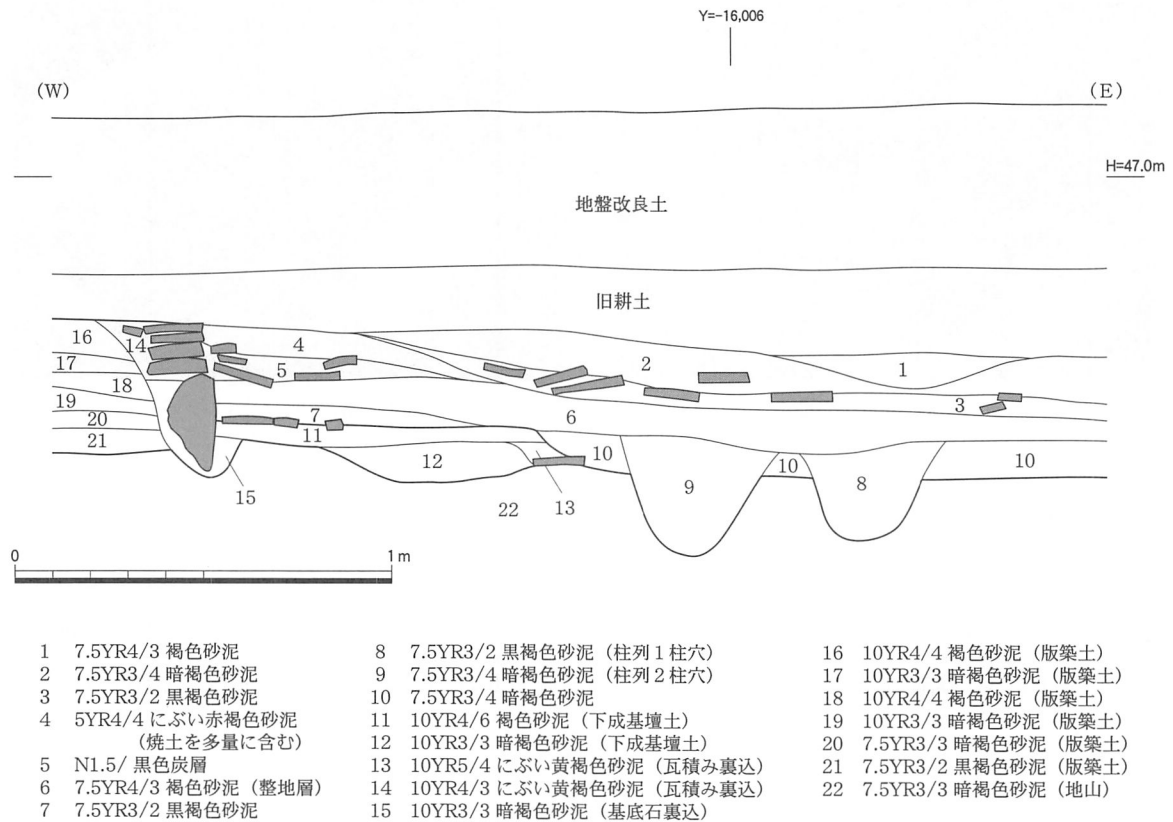
図5 X=-114,871ライン断面実測図 (1:20)
