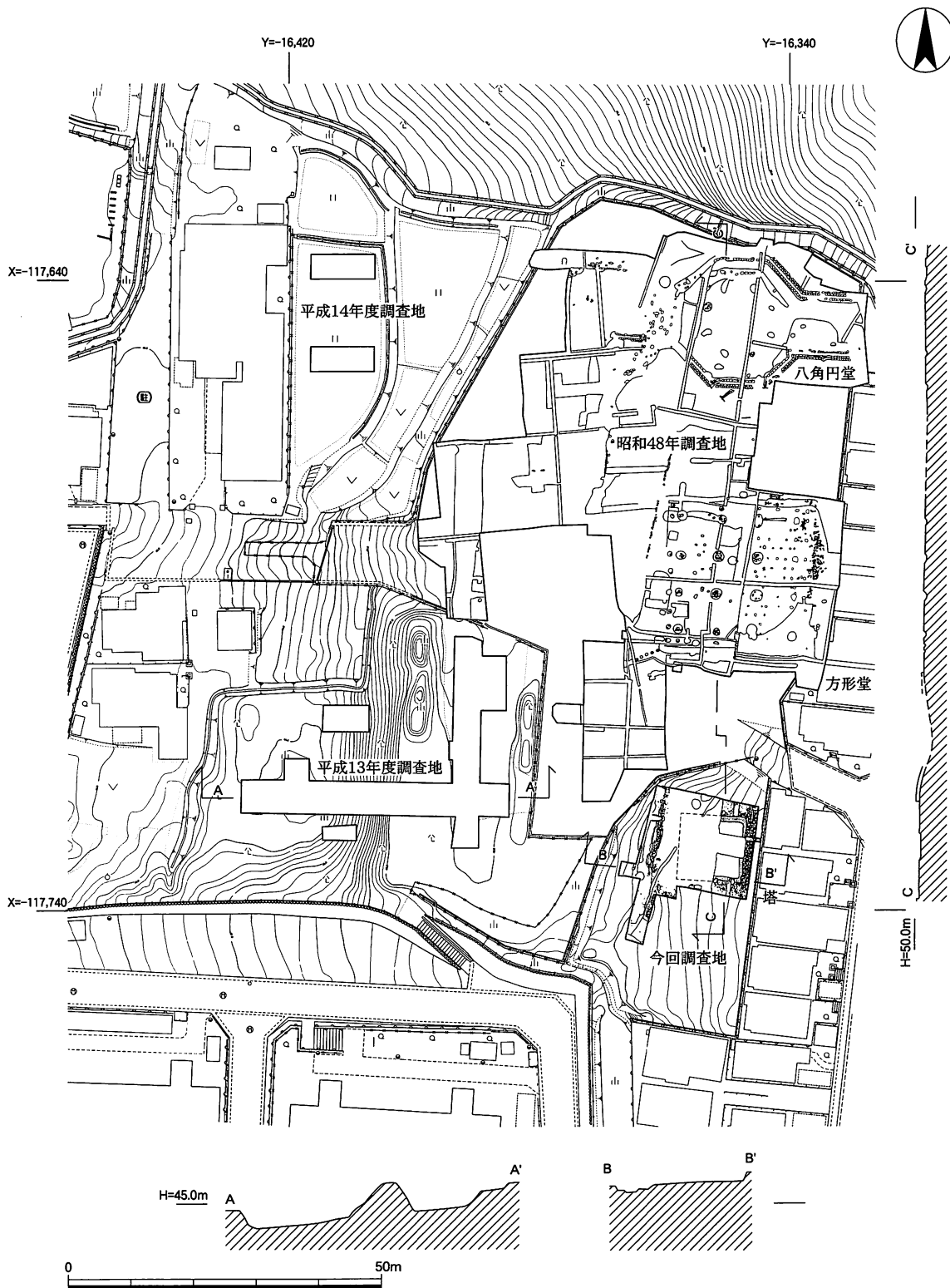
図44 栢ノ杜遺跡調査区配置図 (1:1,000)
