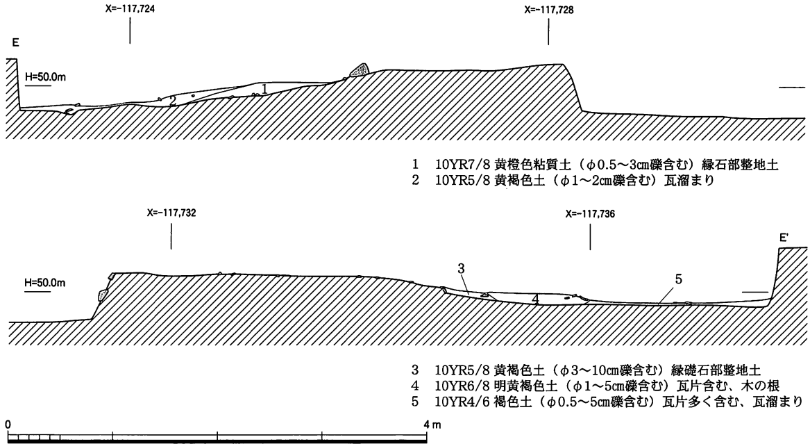
図46 基壇南北断面実測図 (1:50)
