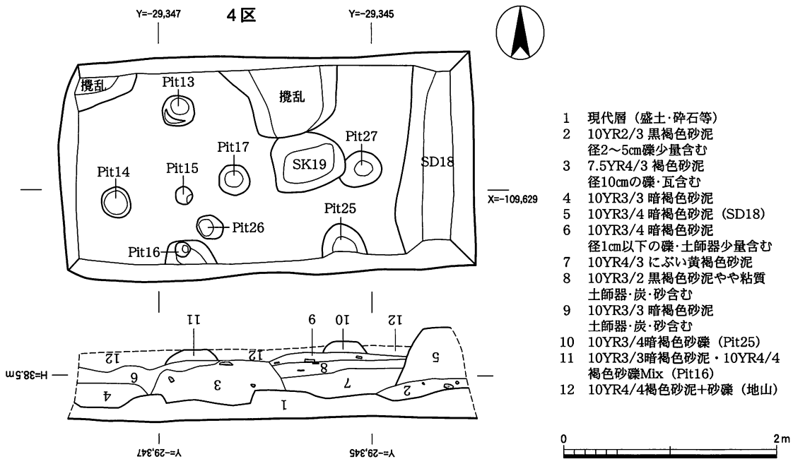
図64 3・4区遺構平面および断面実測図 (1:50)
