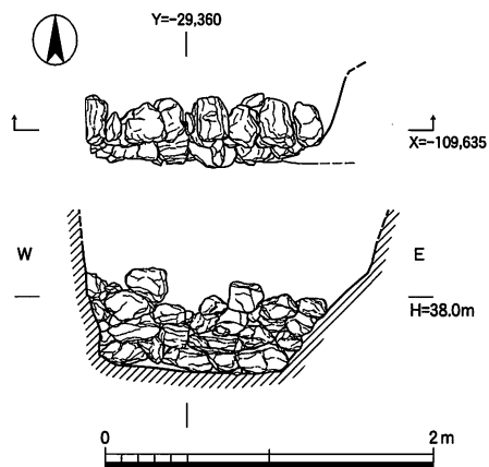
図61 SD20石垣実測図(1:50)
