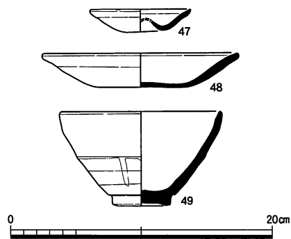
図68 SX33出土土器実測図（1：4）
