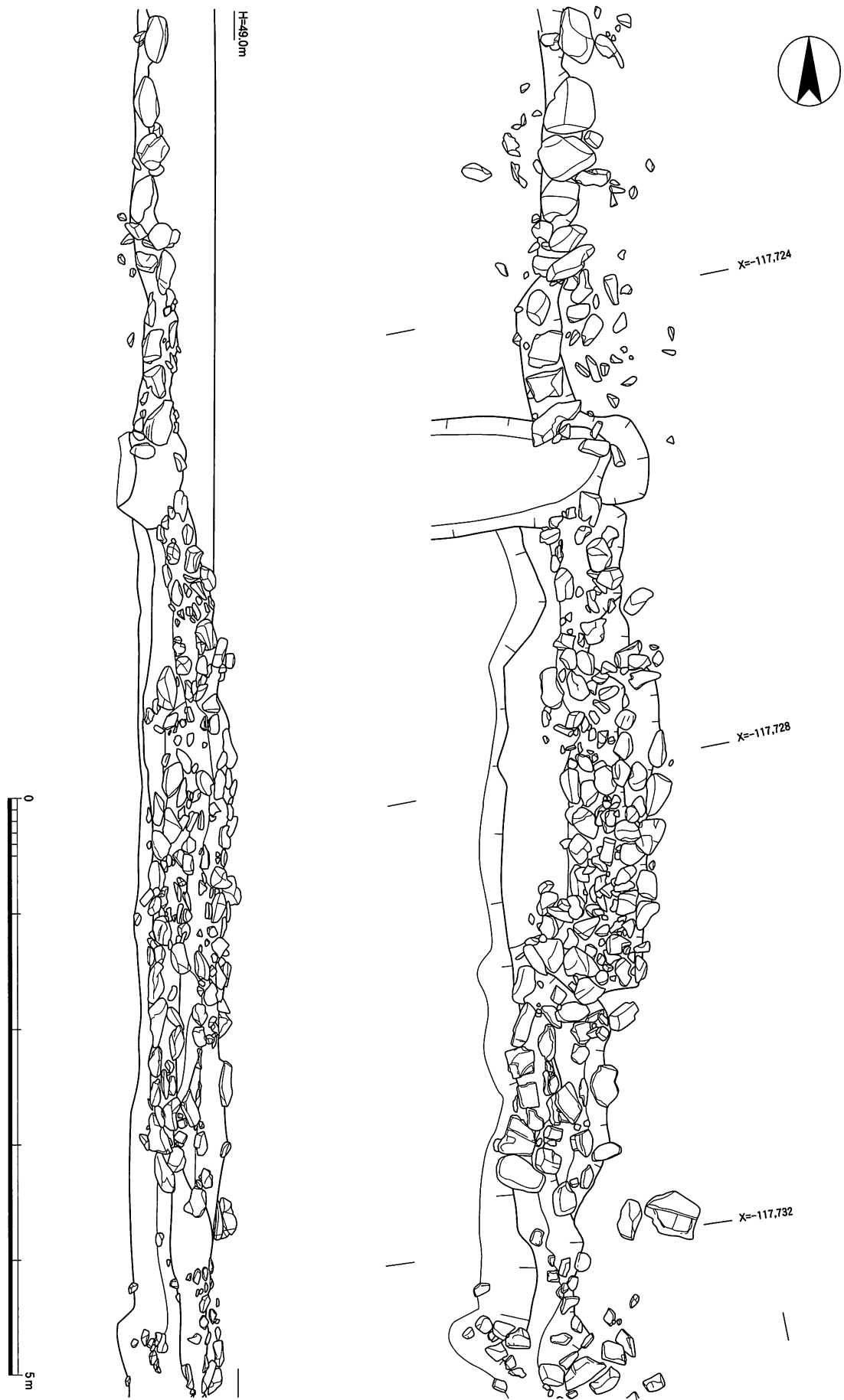
図48 石垣2平面および見通し実測図 (1:50)
