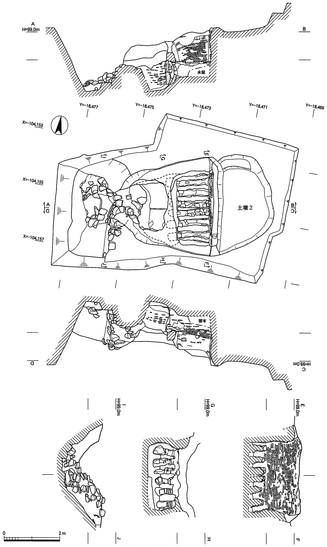
图24 1号窰实测图 (1 : 80)
