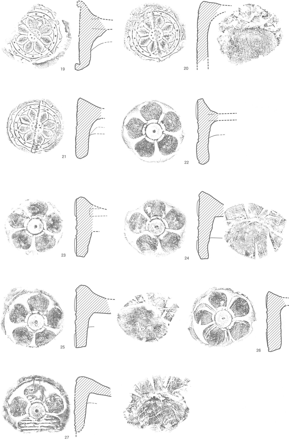
図29 軒丸瓦拓影および実測図 (1 : 4)
