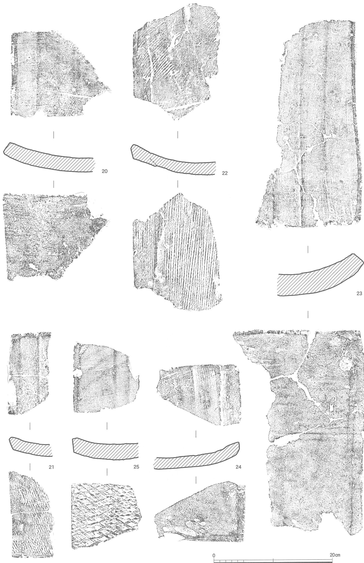
図10 A型式・B型式平瓦拓影および実測図（1：4）
