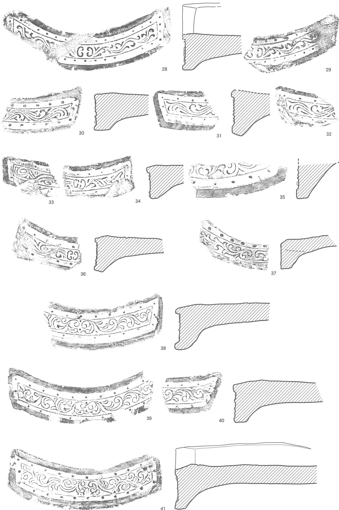
図30 軒平瓦拓影および実測図（1：4）
