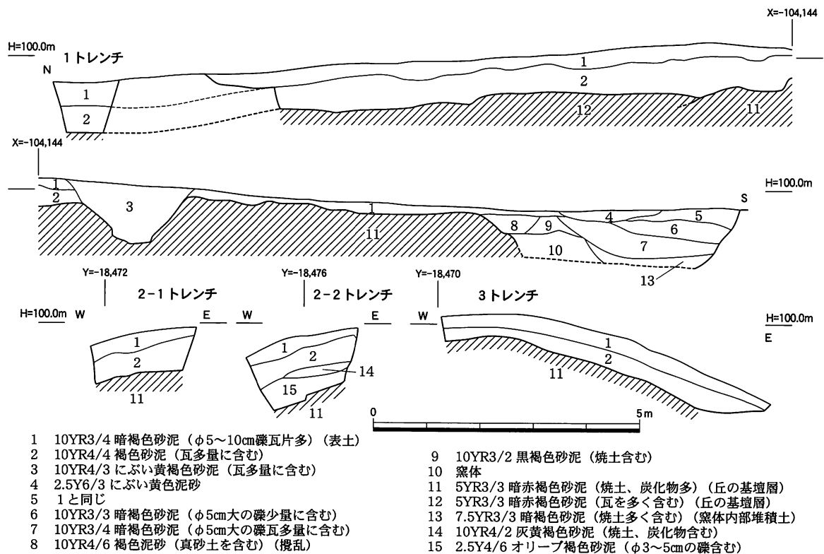
図23 土層断面実測図 (1:100)
