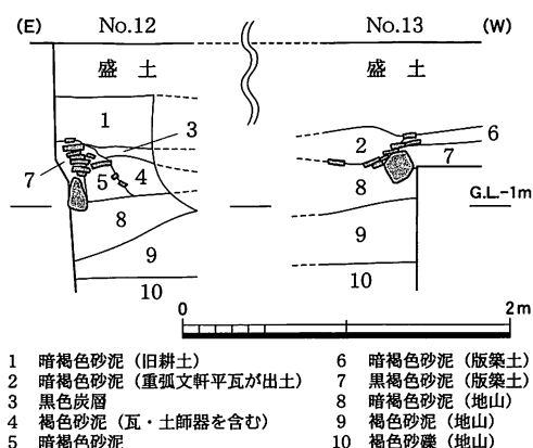
図16 立会調査No.12・No.13地点南壁断面実測図 (1:50)
