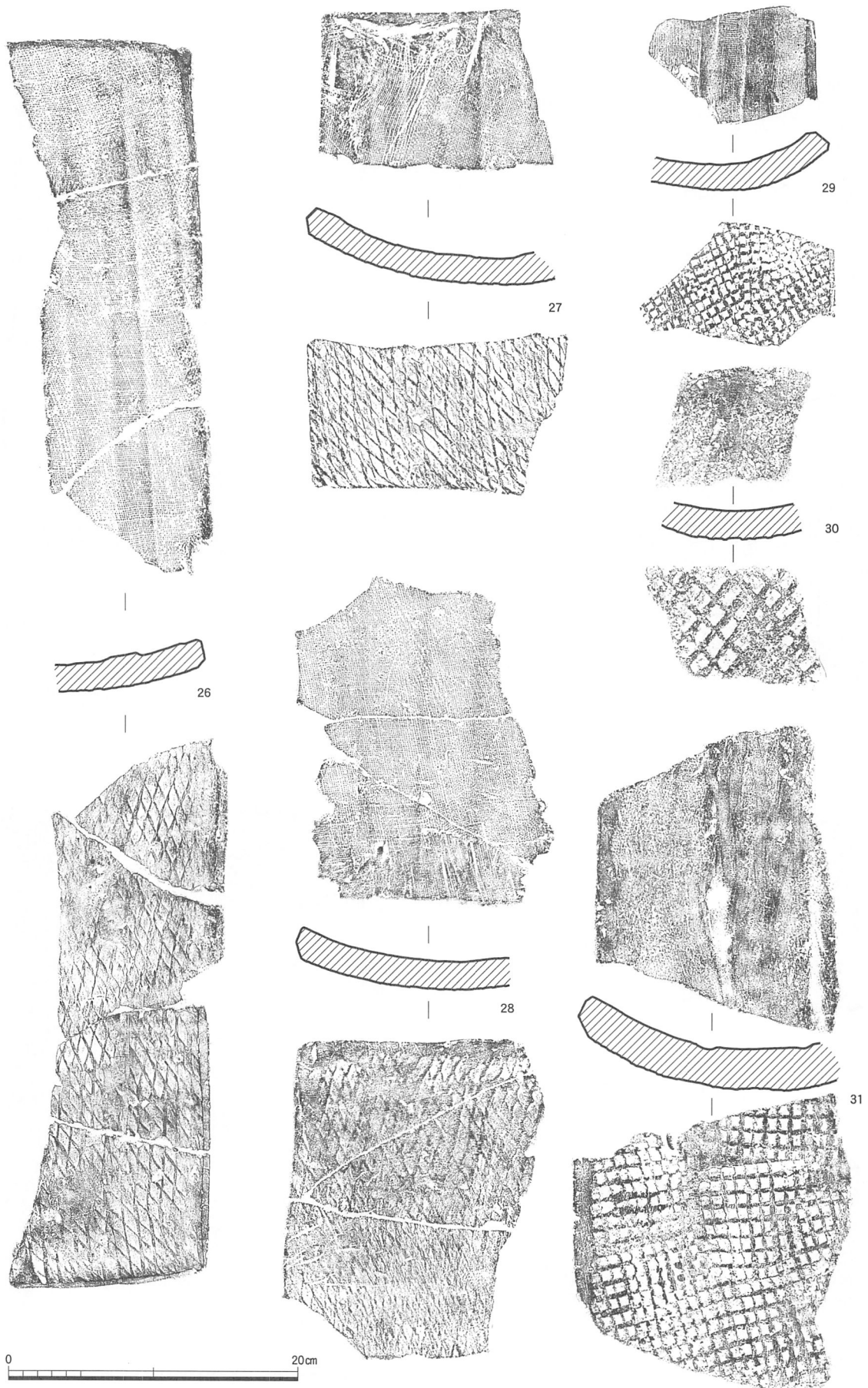
図11 C型式・D型式平瓦拓影および実測図（1：4）
