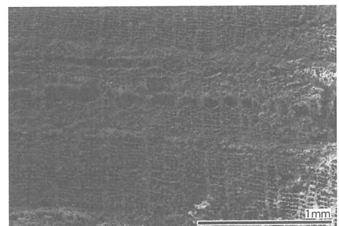
図15 炭化材電子顕微鏡写真（×25）
