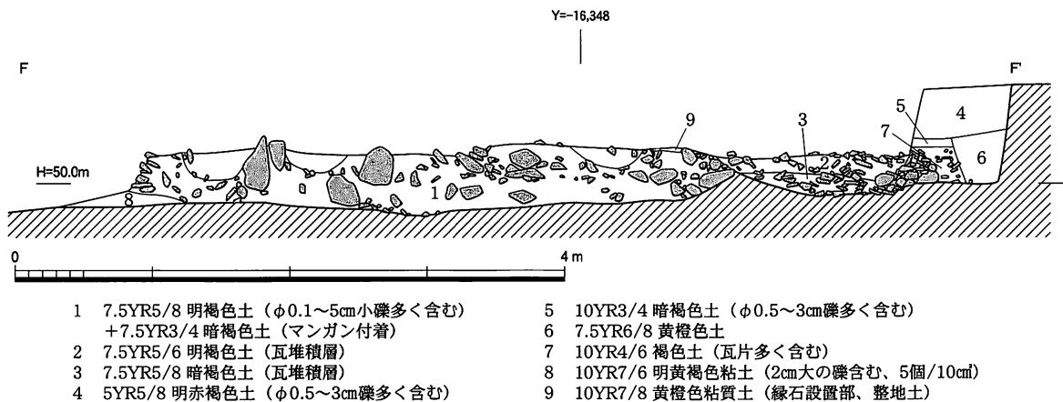
図47 基壇東西断面実測図 (1:50)
