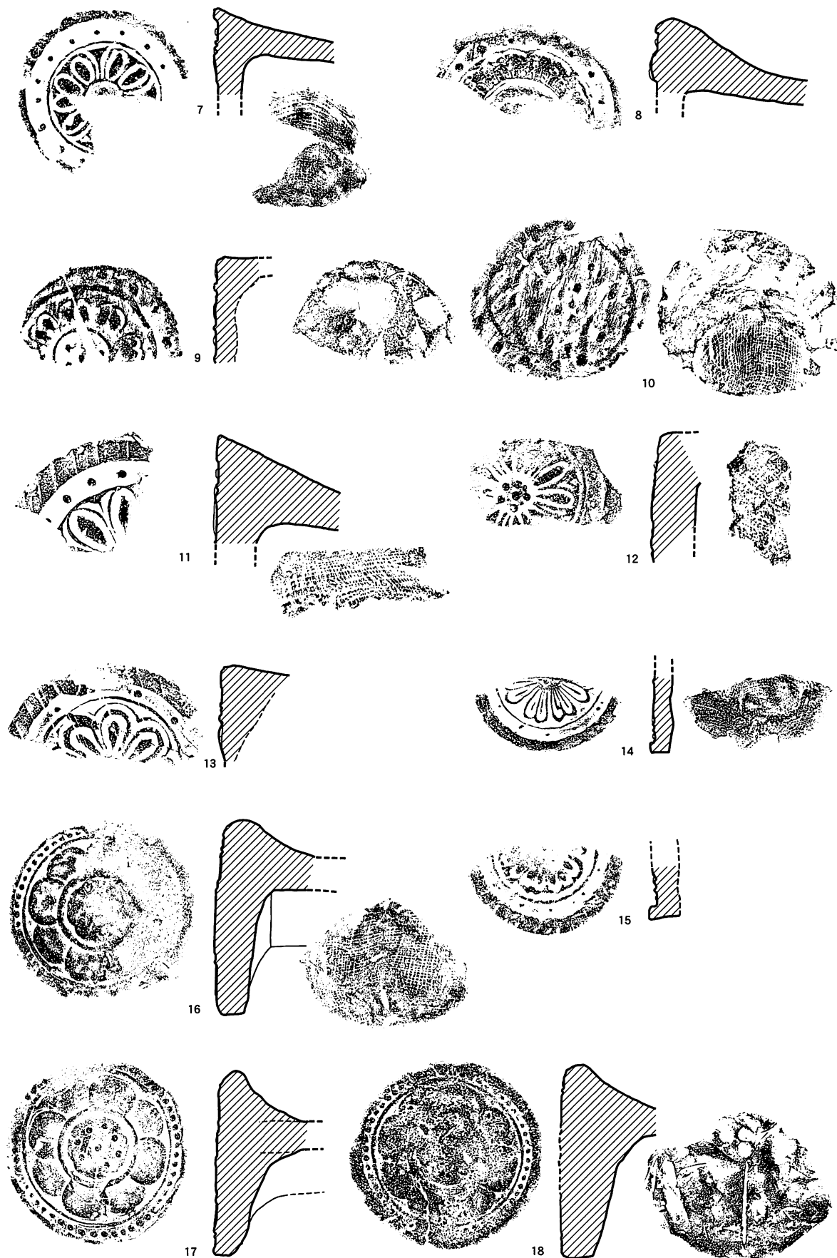
図28 軒丸瓦拓影および実測図 (1 : 4)
