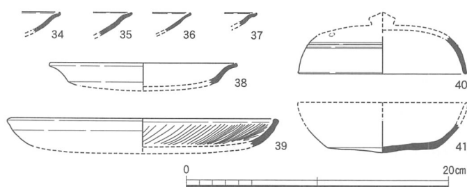
図13 出土土器実測図（1：4）
