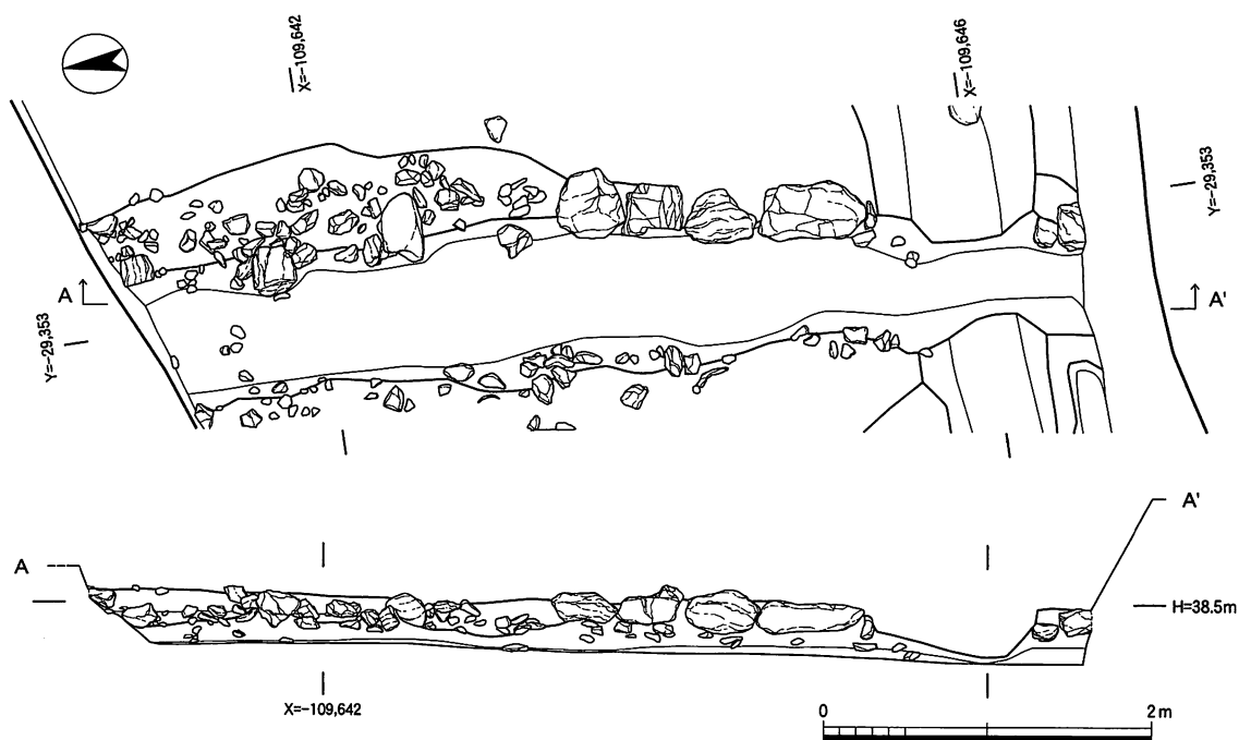
図62 SD24(b)平面および見通し実測図(1:50)
