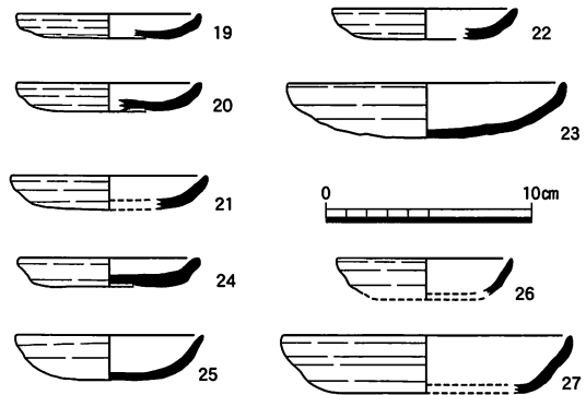
図55 出土土器実測図 (1:4)
