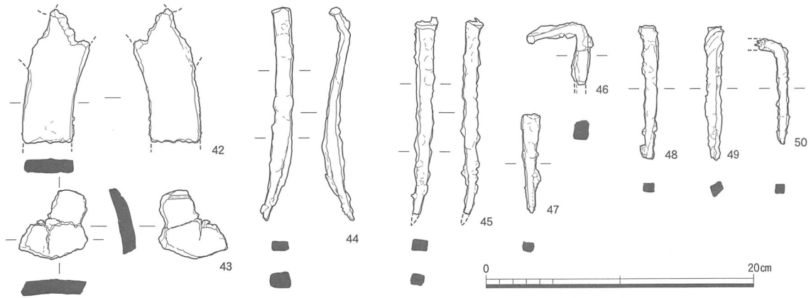
図14 金属製品実測図（1：4）
