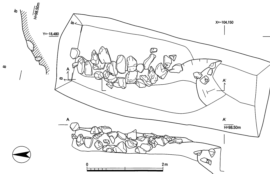
図25 石積3実測図(1:50)
