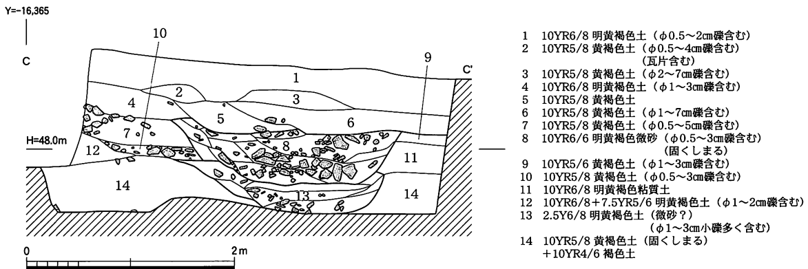
図50 溝3東西断面実測図 (1:50)
