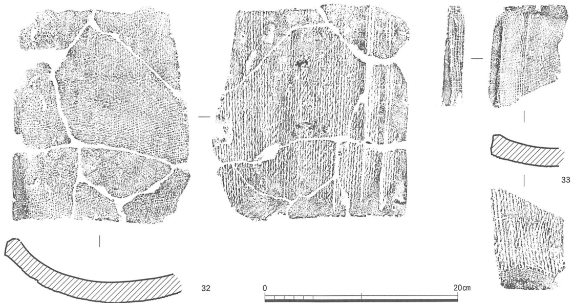
図12 E型式平瓦拓影および実測図（1：4）
