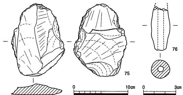
図27 石器実測図 (1:4)・土錘実測図 (1:2)
