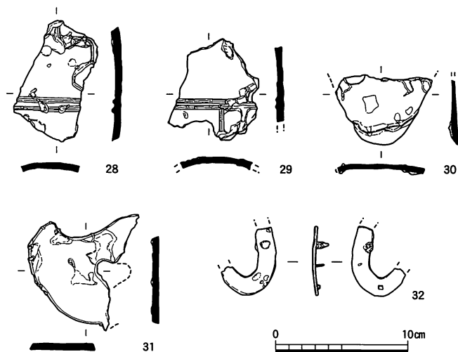
図56 鉄製品実測図 (1:4)
