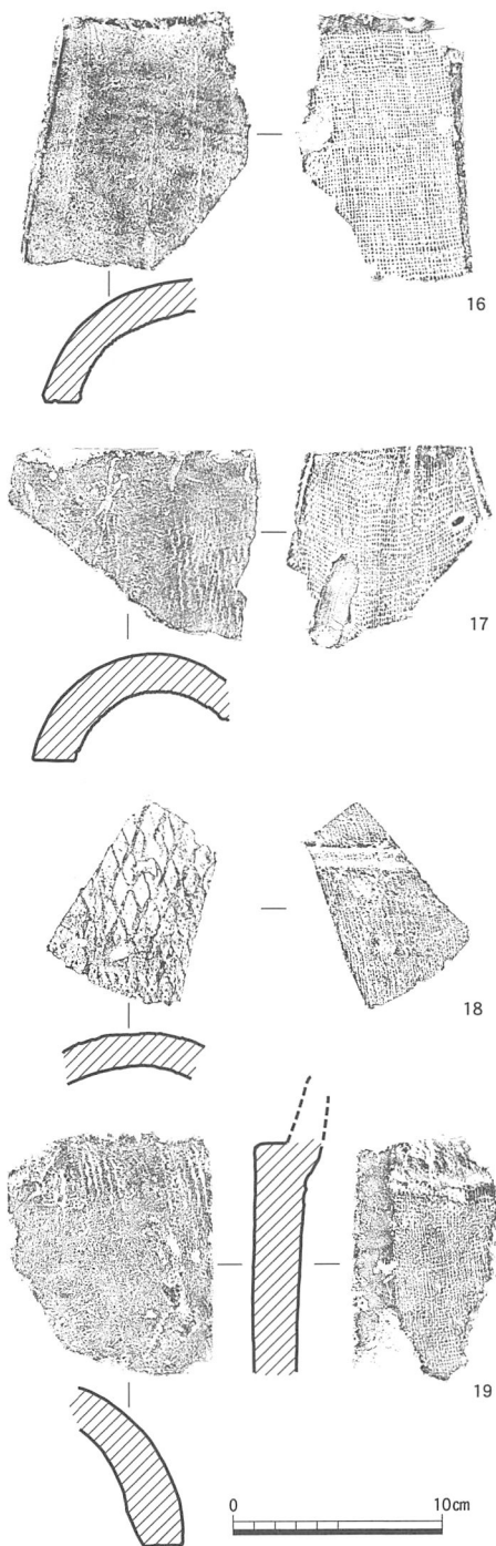
図9 丸瓦拓影および実測図(1:4)
