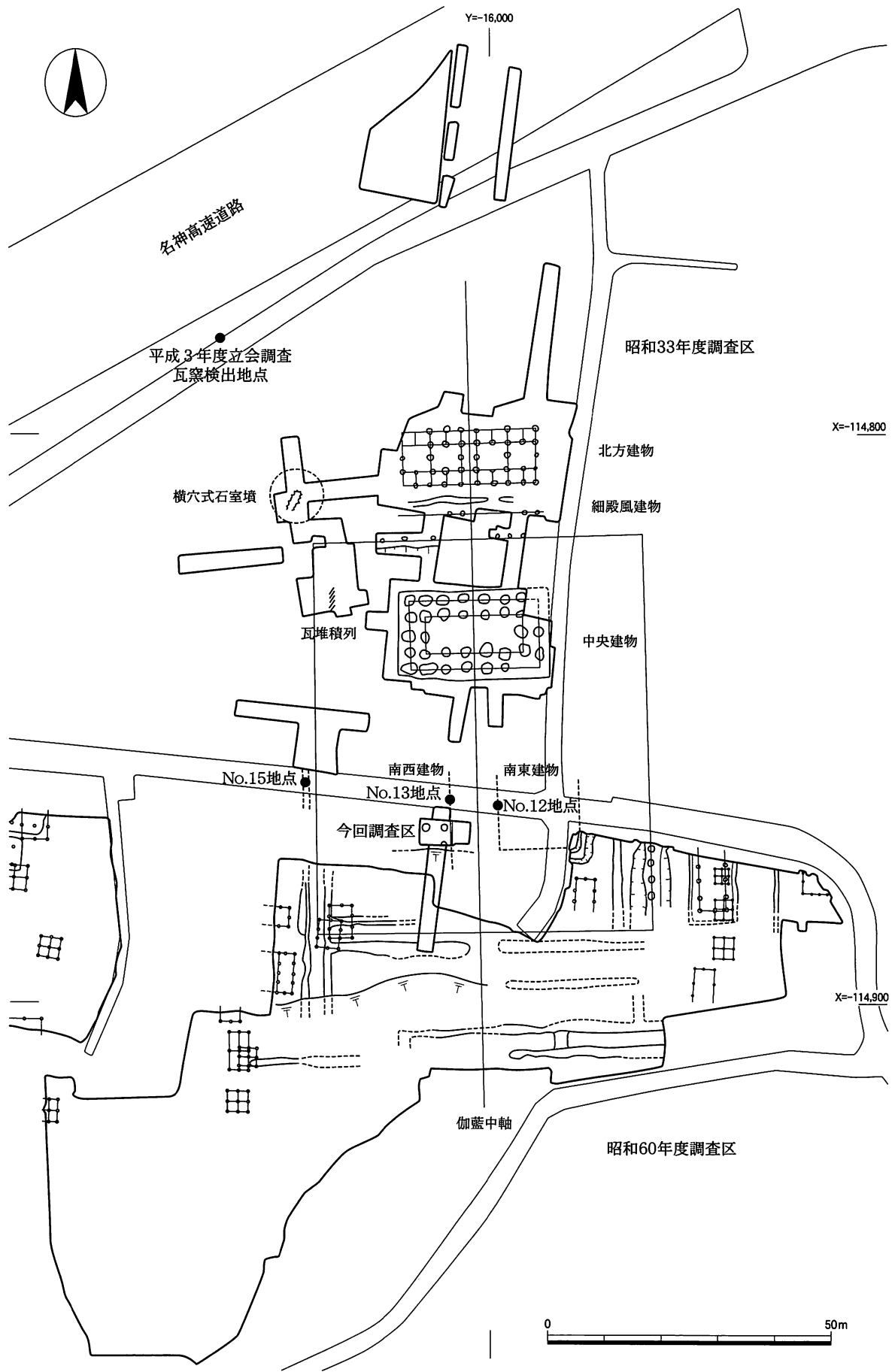
図18 大宅廃寺遺構配置図 (1 : 1,000)
