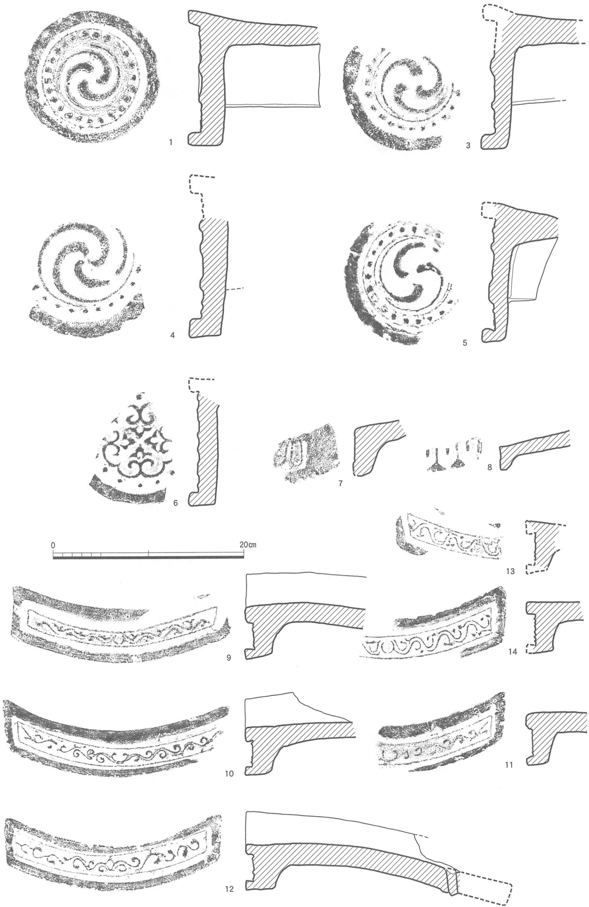
图52 軒瓦拓影および実測図 (1 : 4)
