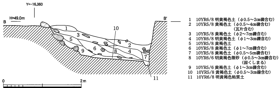
図49 石垣2東西断面実測図 (1:50)
