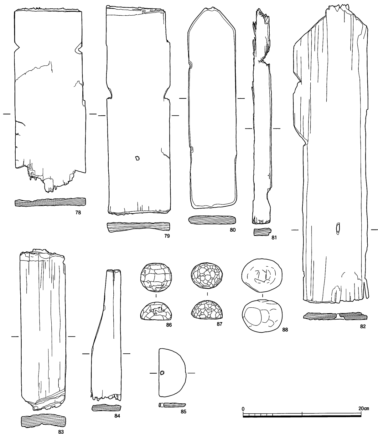
図42 SG1出土木製品実測図(1:4)
