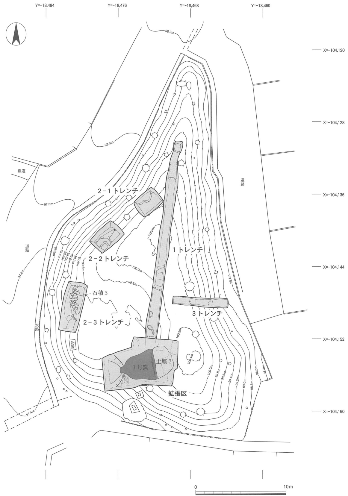
図22 地形及び調査区配置図 (1 : 250)
