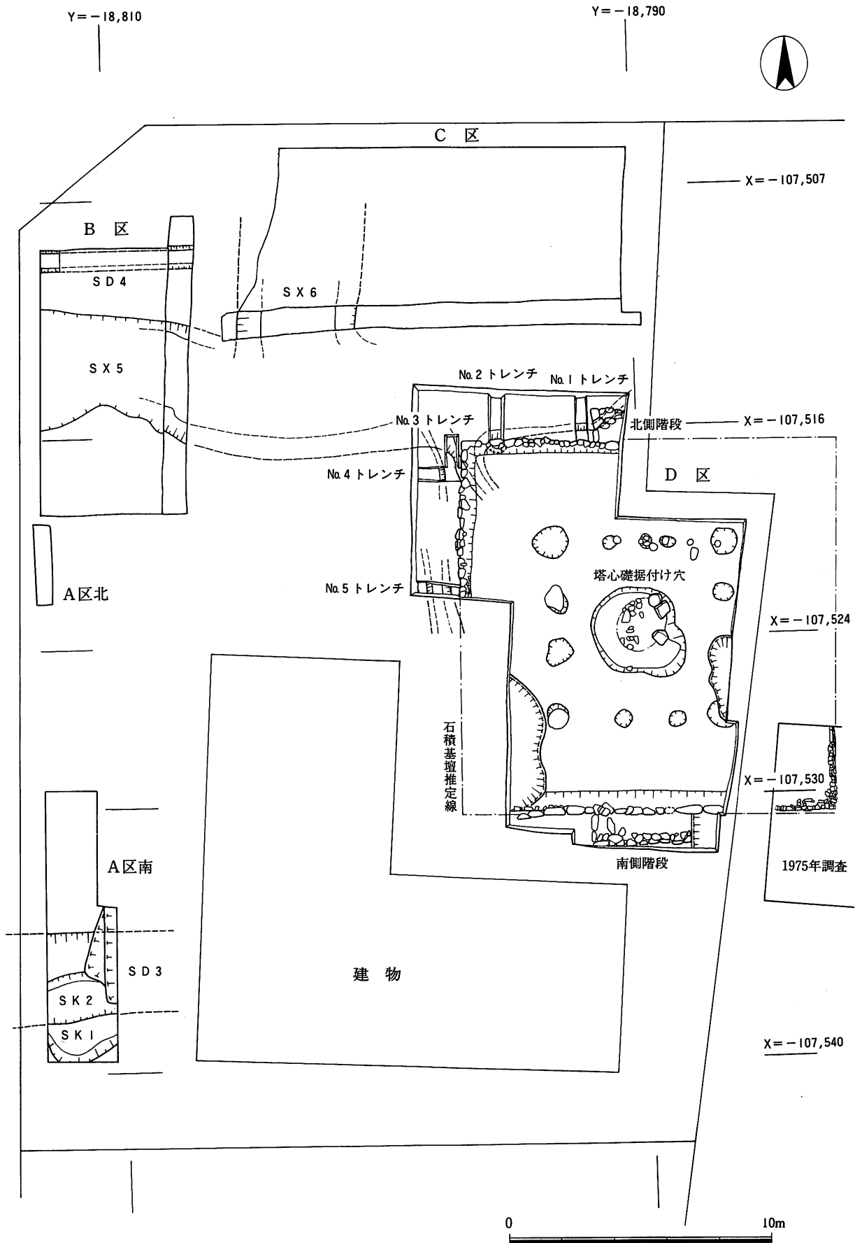
調査区配置図 (1:200)
