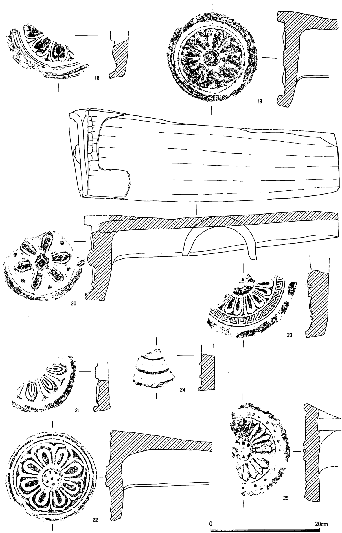
軒丸瓦拓影・実測図 (1:4)
