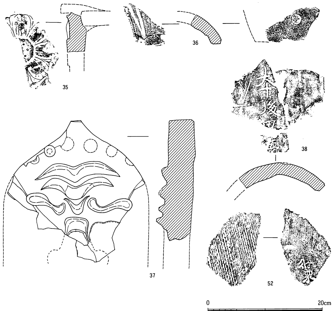
図4 瓦拓影・実測図 (1:4)
