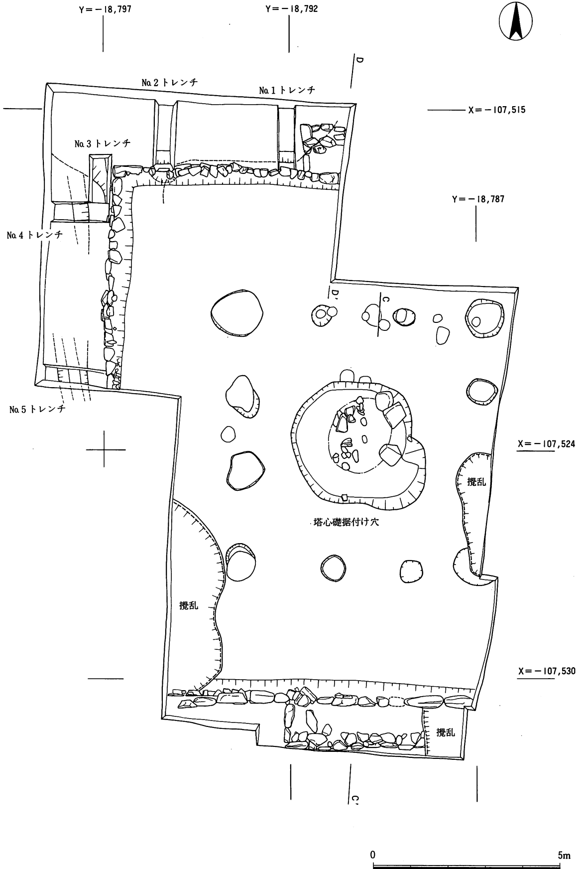
D区平面図 (1:100)
