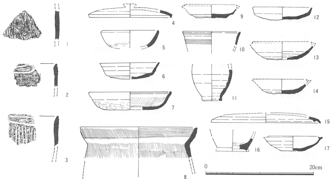
図3 遺物実測図 (1:4)
