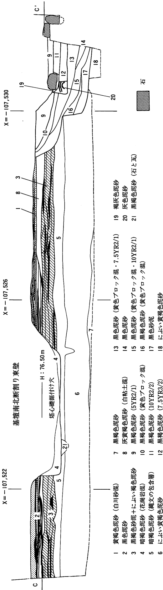
基壇南北断割り・No.5 トレンチ断面図 (1:50)
