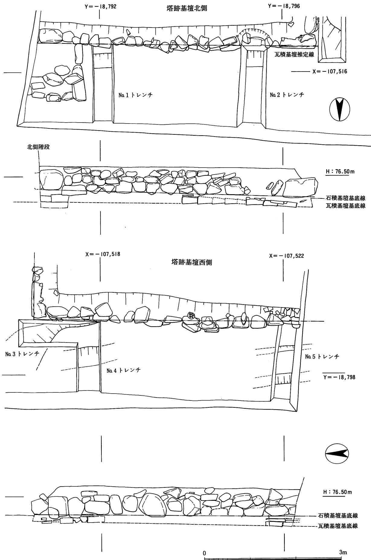
基壇北・西側平面・立面図 (1:50)
