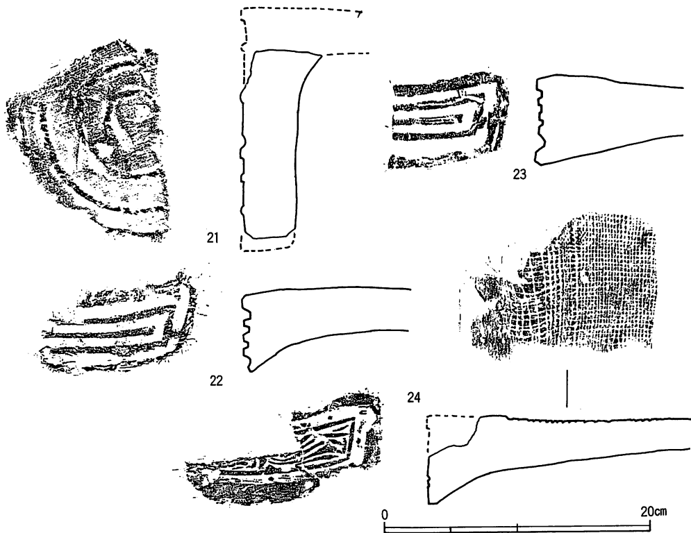
図5 軒瓦拓影・実測図
