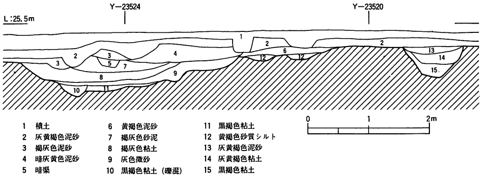
図 14 SD 17・23 断面実測図
