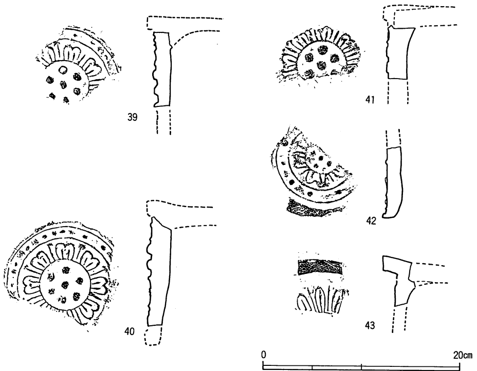
図11 軒瓦拓影・実測図
