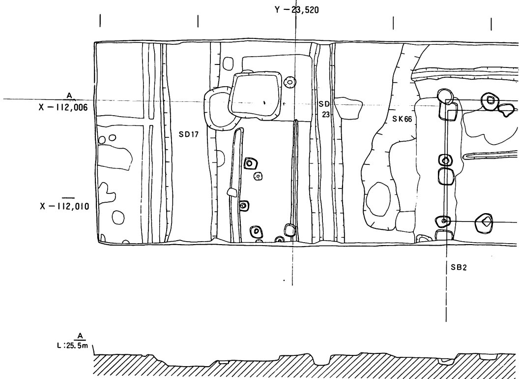
図 13 遺構実測図
