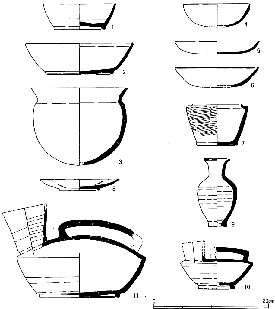
図 15 遺物実測図
