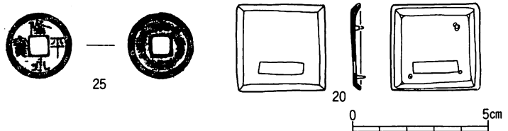
図4 遺物実測図
