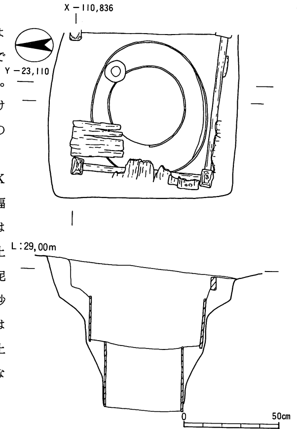
図9 SE12 実測図
