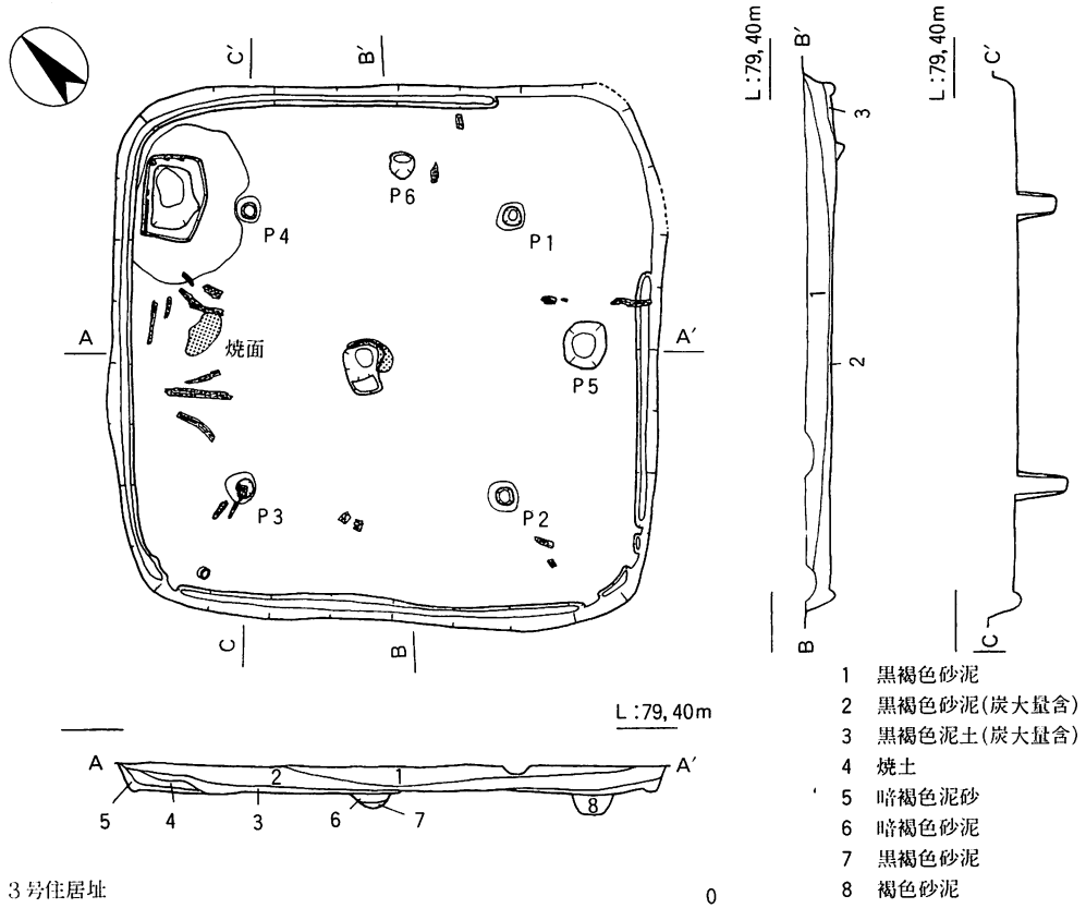
竪穴住居址実測図
