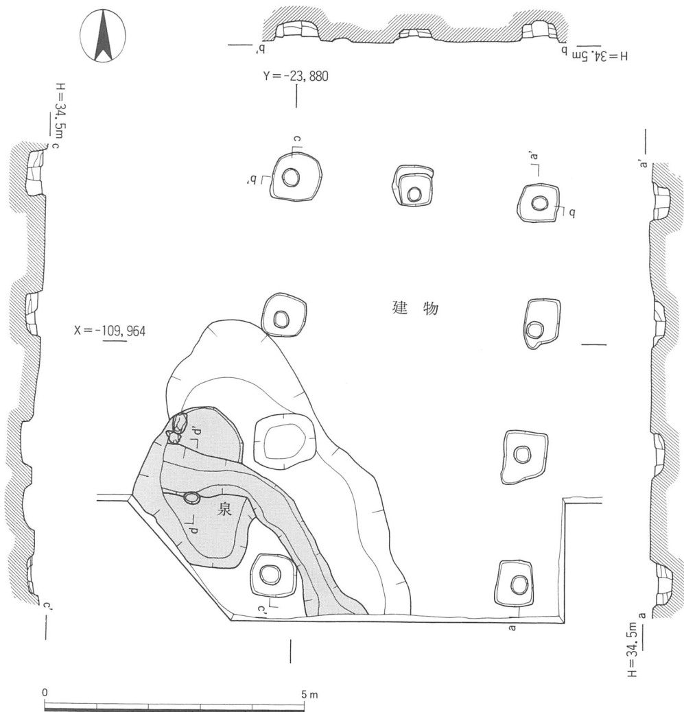
図5 建物・泉実測図(1:100)
