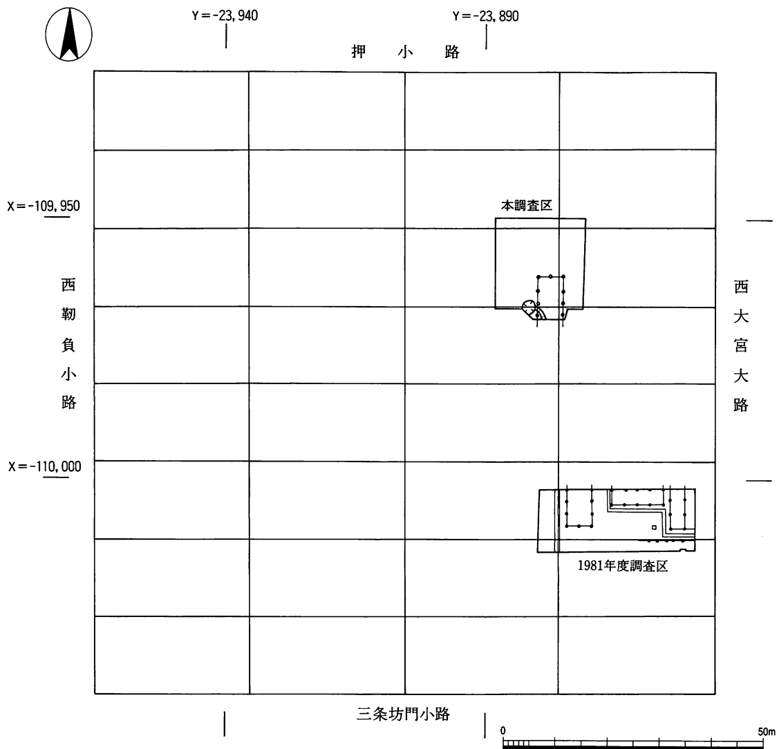
図8 右京三条二坊二町遺構配置図 (1 : 1,000)
