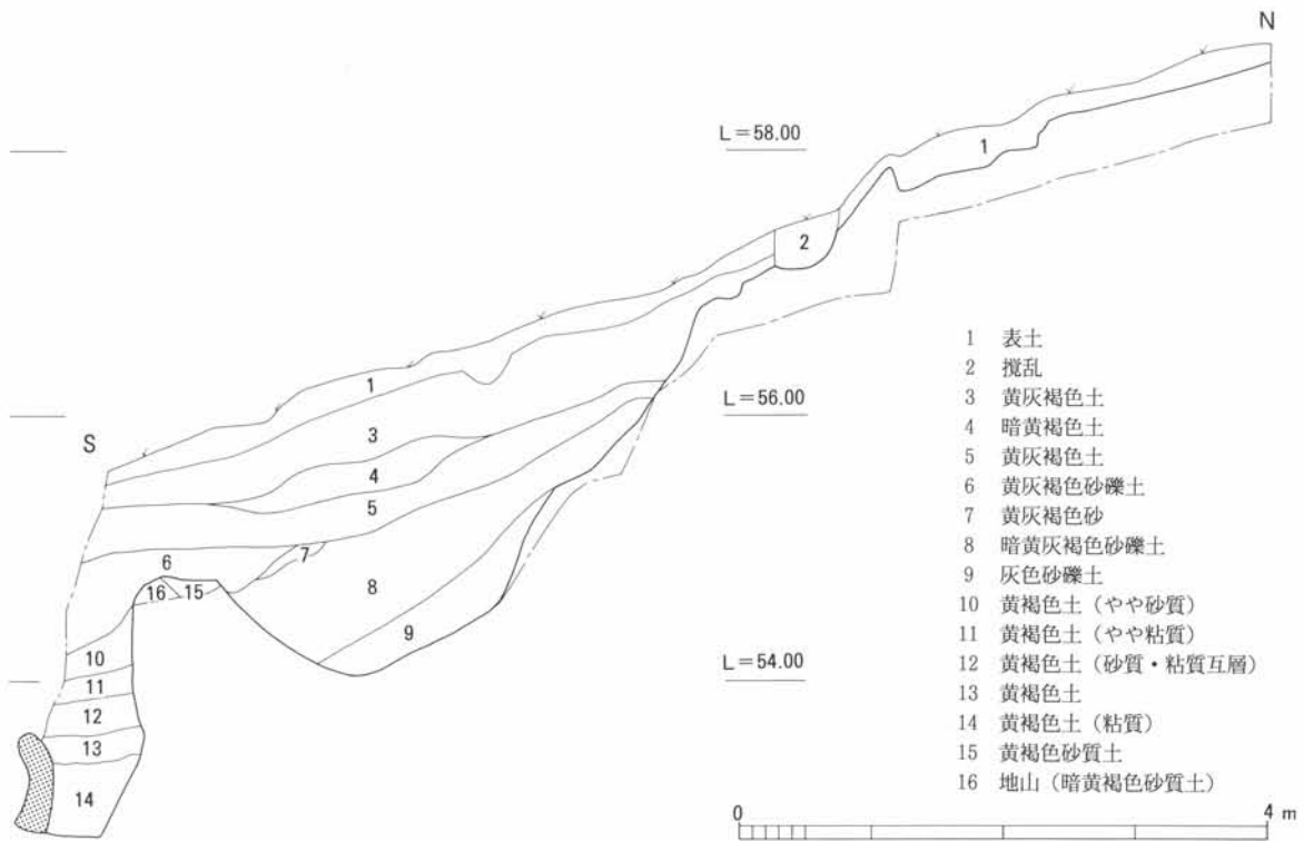
南北方向土層図
