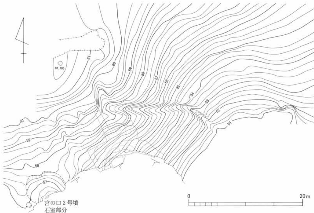
トレンチ配置図
