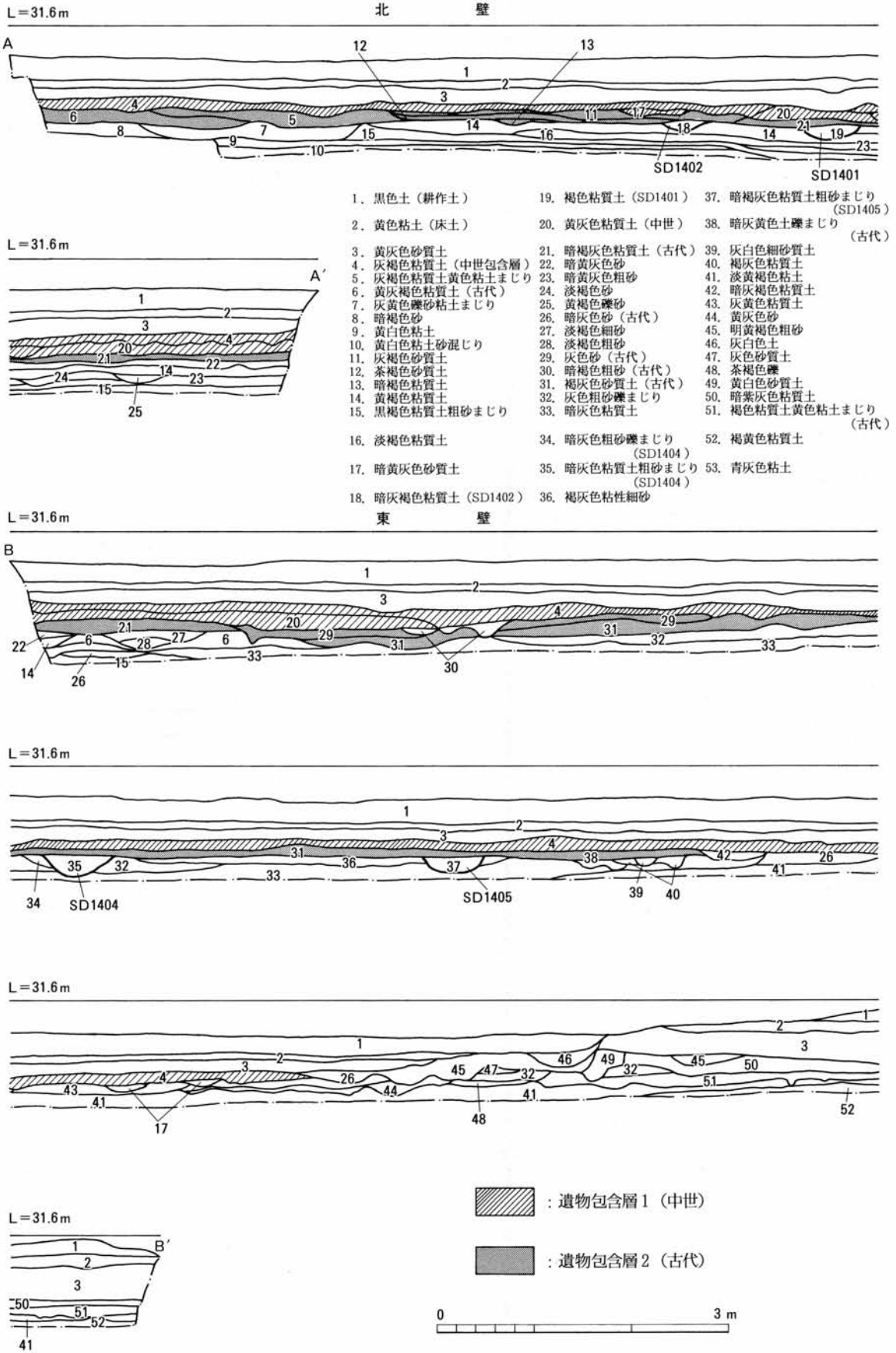
第36図 第14次調査トレンチ 土層断面図
