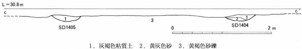
第43図 SD1404・SD1405 断面図
