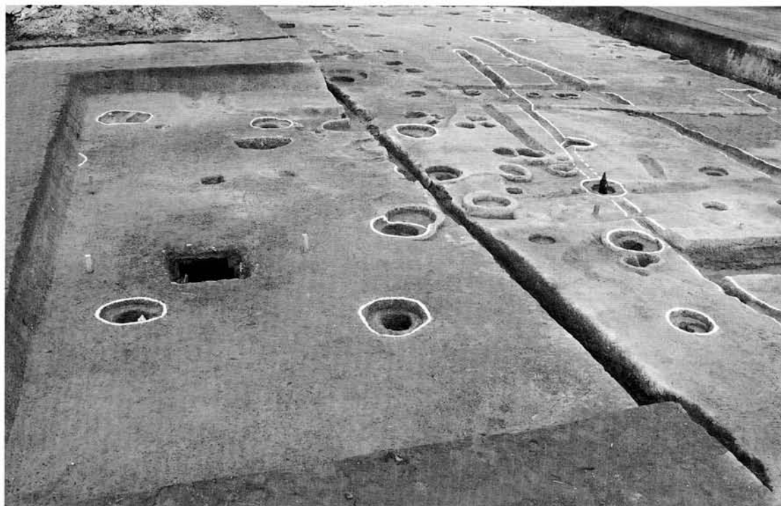
第20図 SB13114 (南から)
