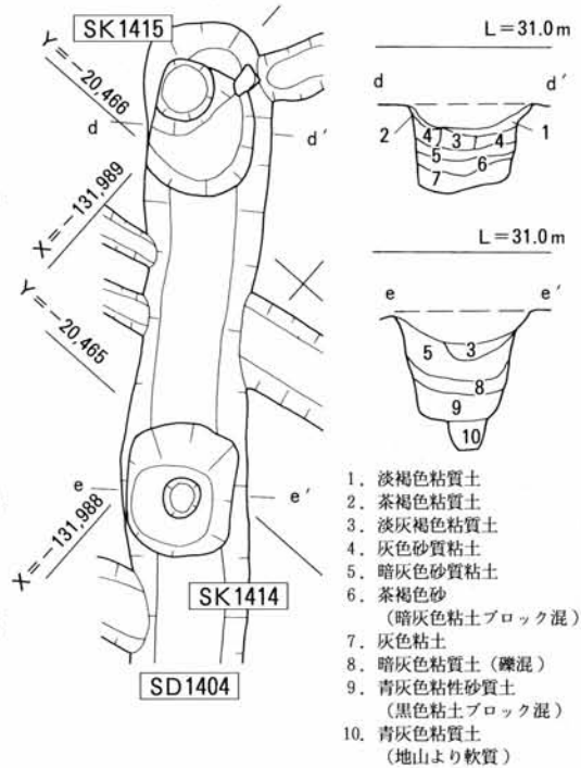
第46図 SK1414・SK1415 実測図 (S=1:40)
