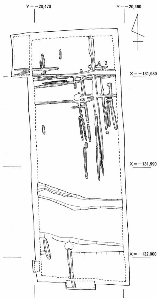
第35図 第14次調査 中世面遺構図 (S=1:200)
