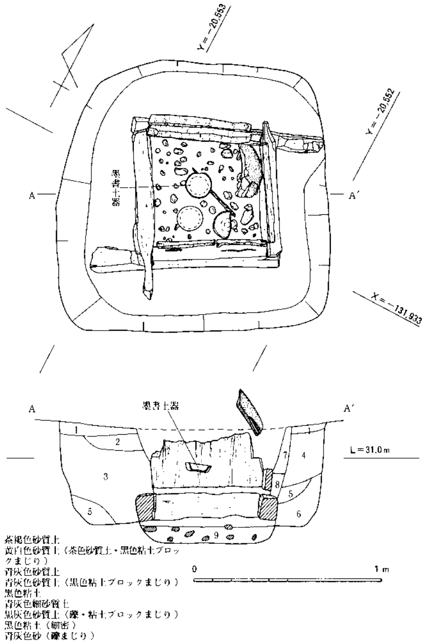
第15図 SE13113 実測図
