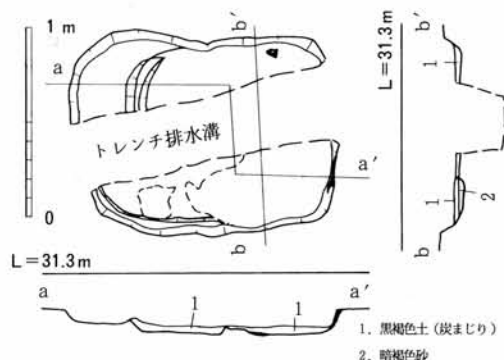
第21図 SX1384 実測図
