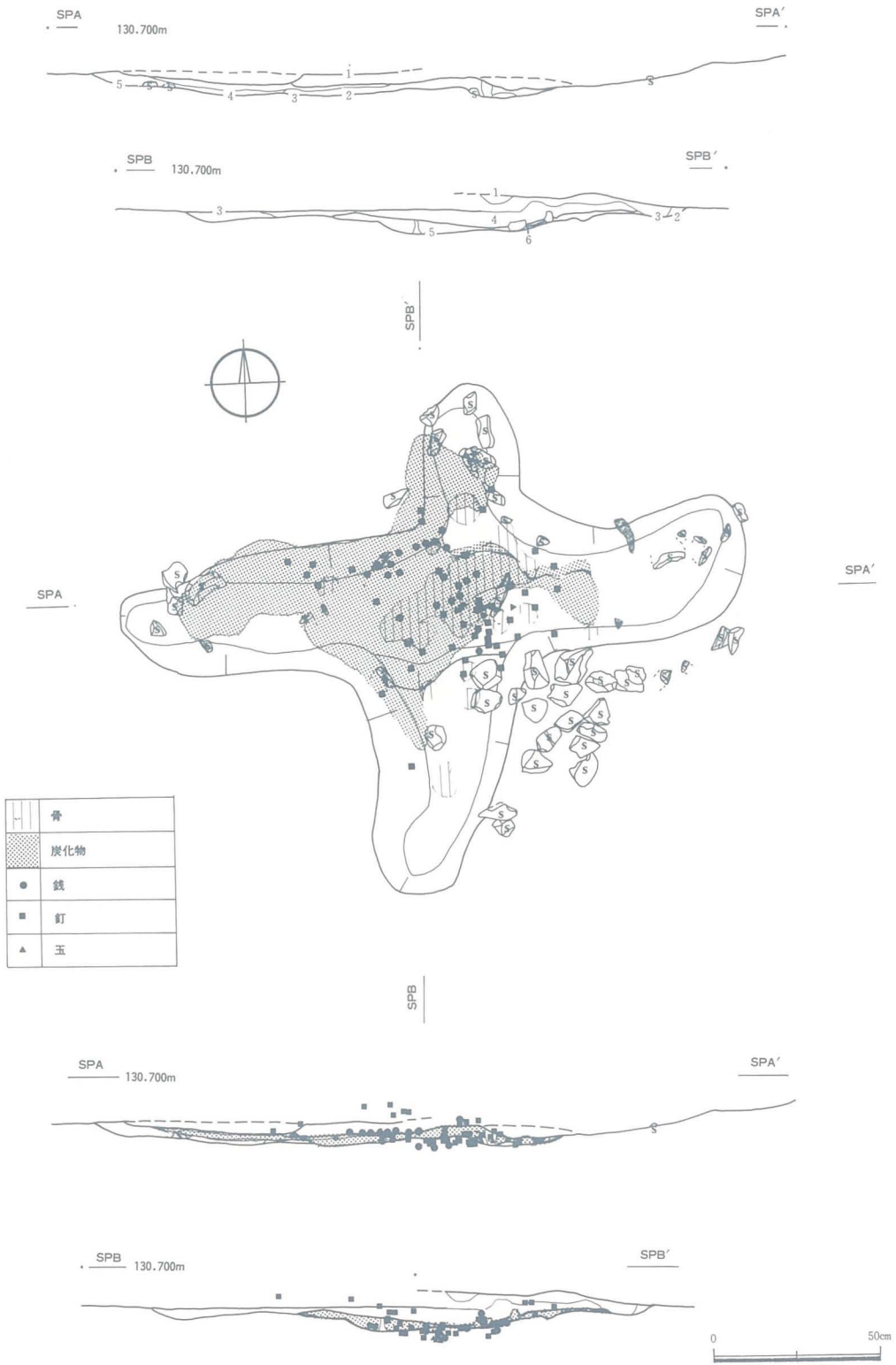
第15図 5号土壌・土層堆積図 5号土壌遺物分布図(釘・錢・玉・炭化物・骨)
