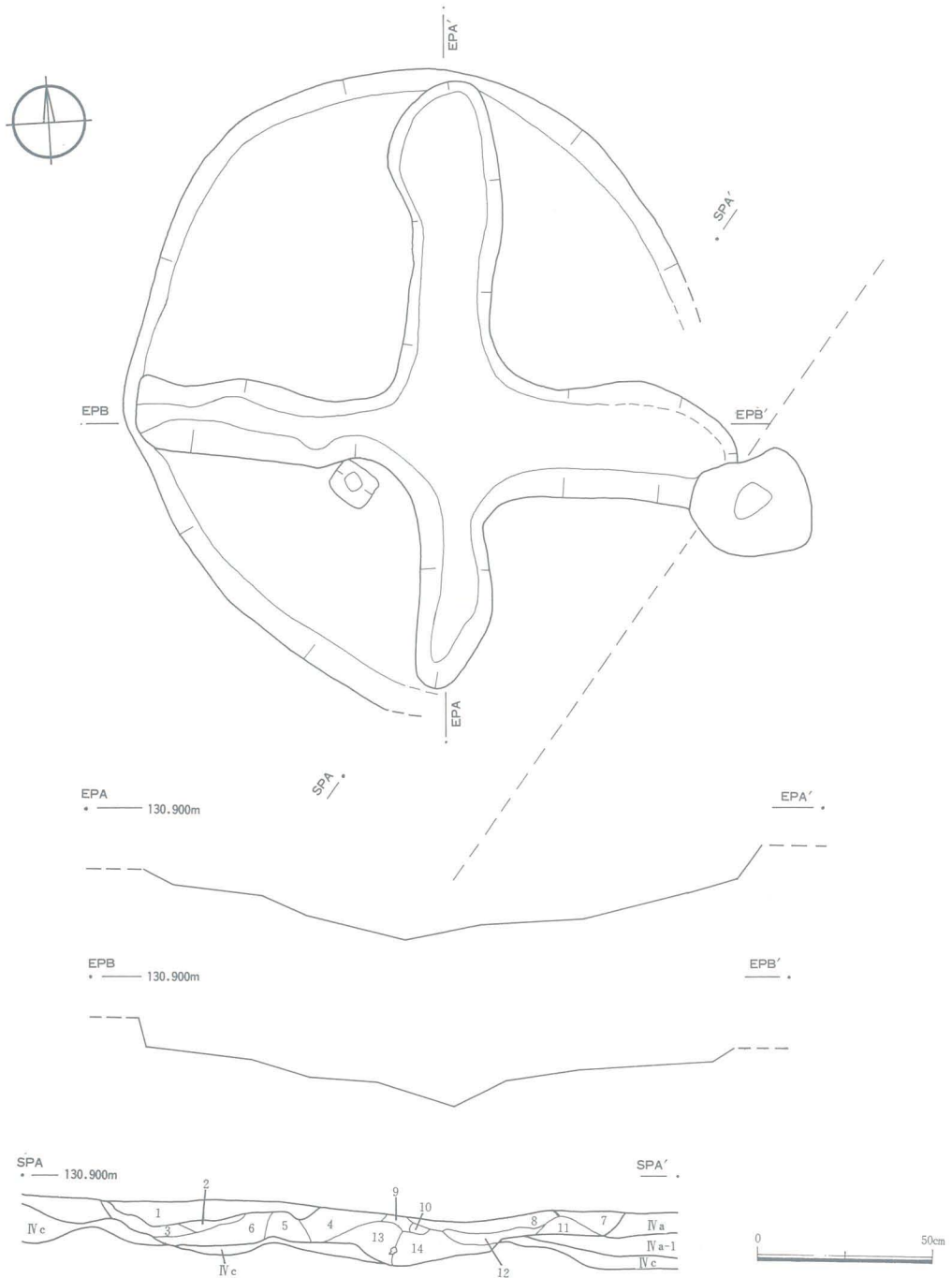
第5図 2号土壌平面図・土層堆積図
