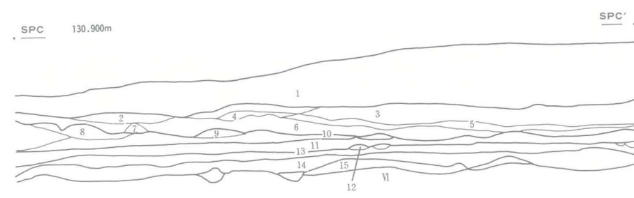
土層堆積 ③
