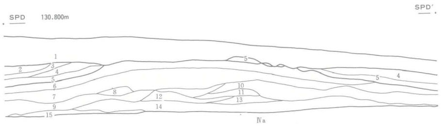
土層堆積 ④
