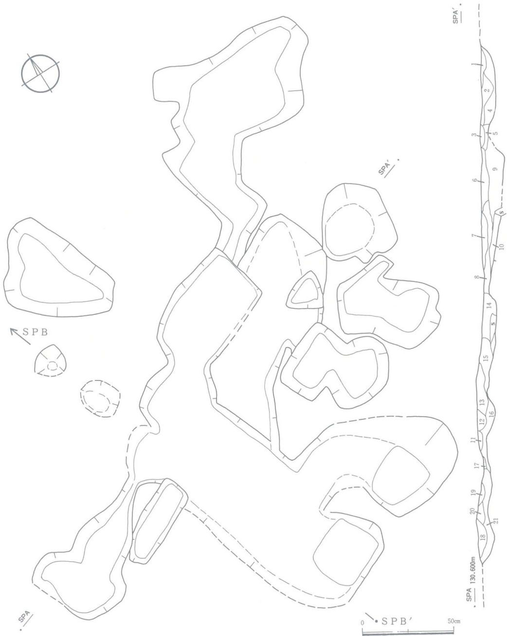
第21図 焼土平面図・土層堆積図
