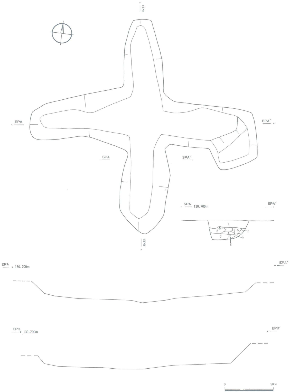
第 2 图 1 号土壤平面图
