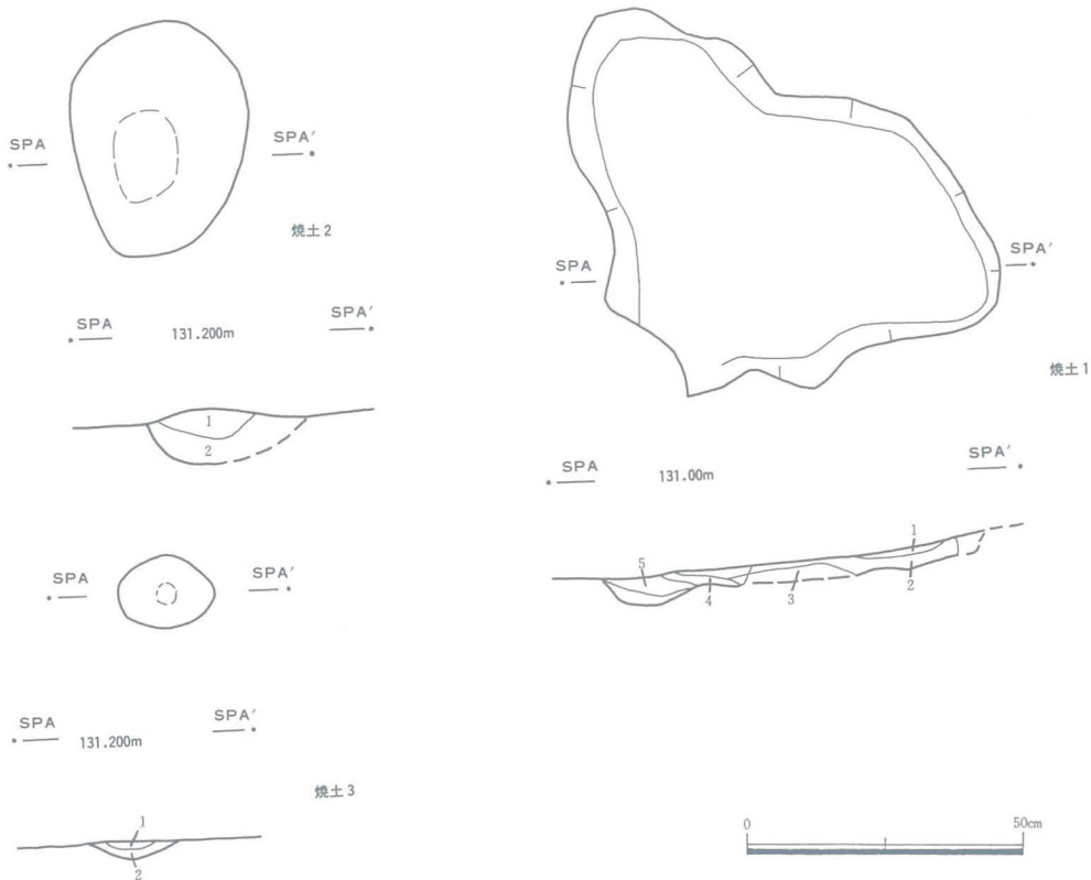
第23図 焼土平面図・土層堆積図
