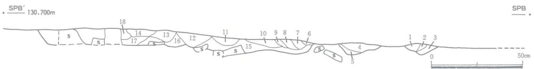
第21図 焼土平面図・土層堆積図
