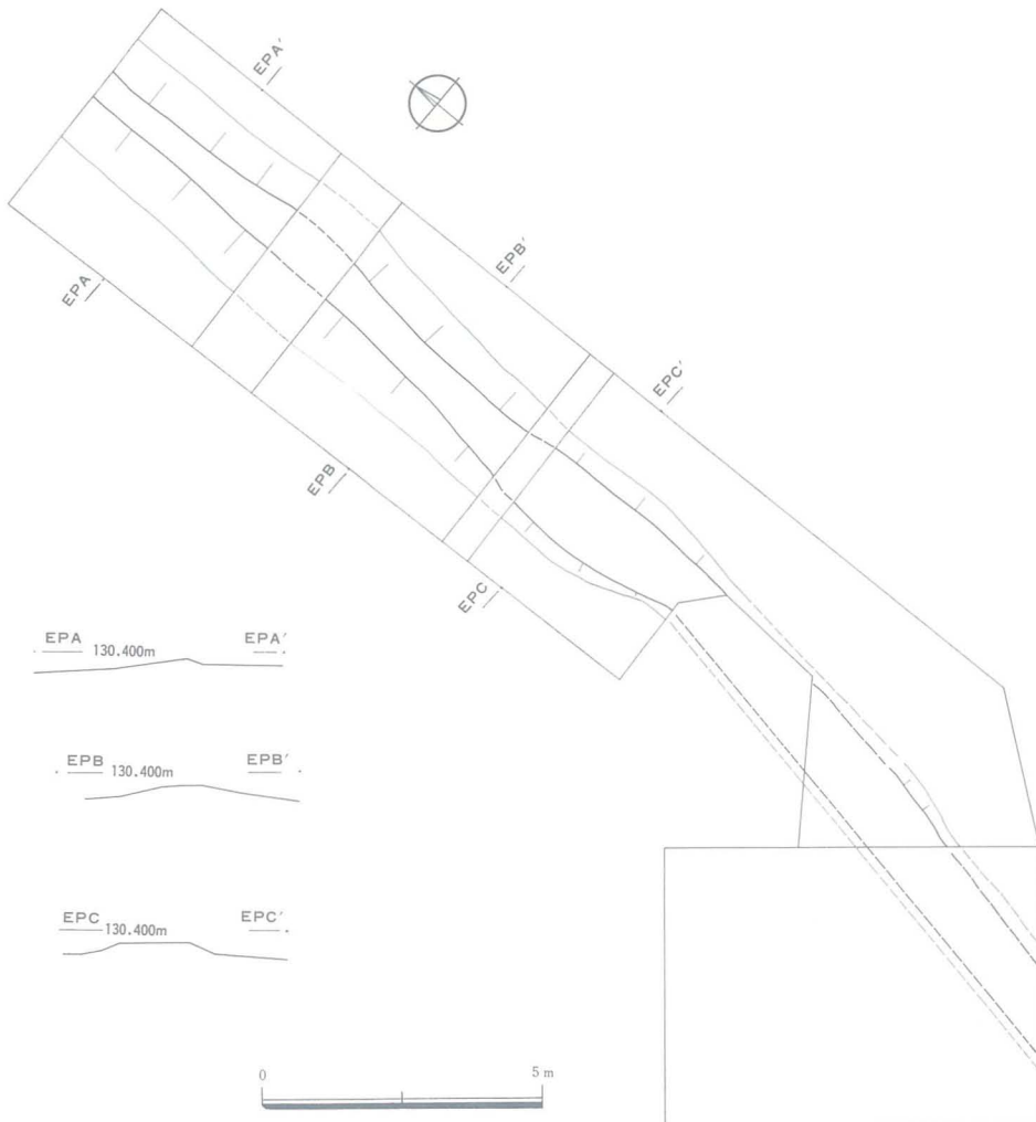
第24図 旧道跡平面図
