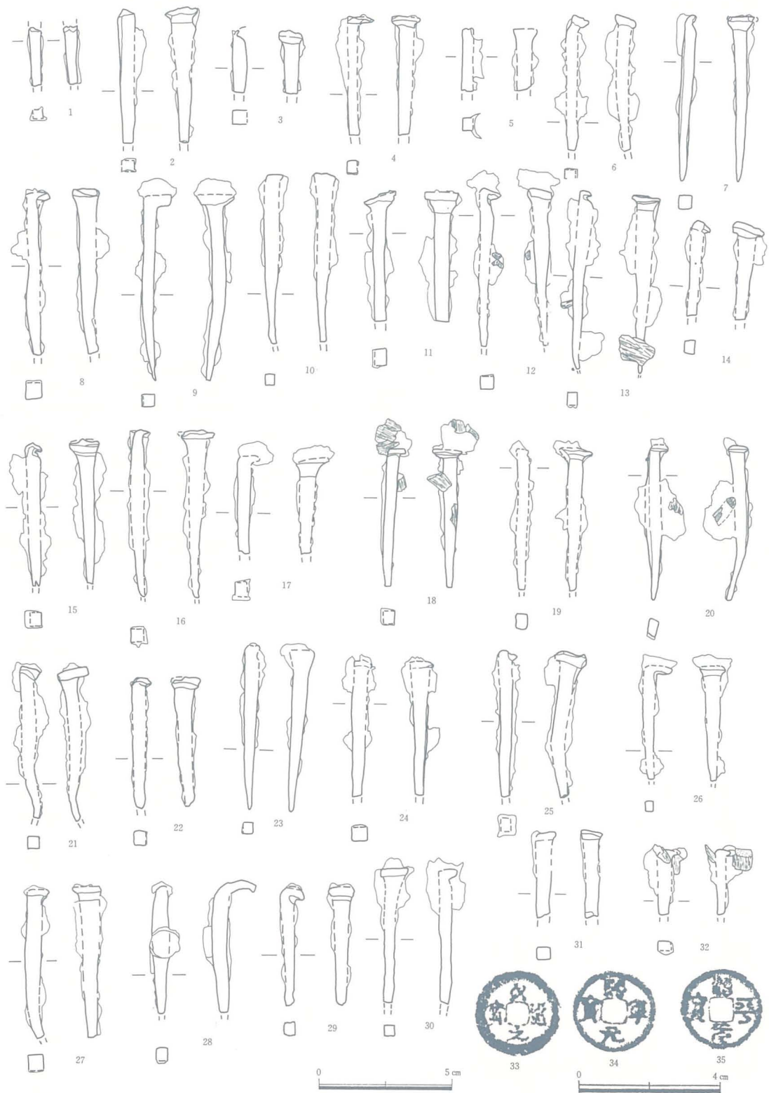
第7图 2号土坑出土遗物
