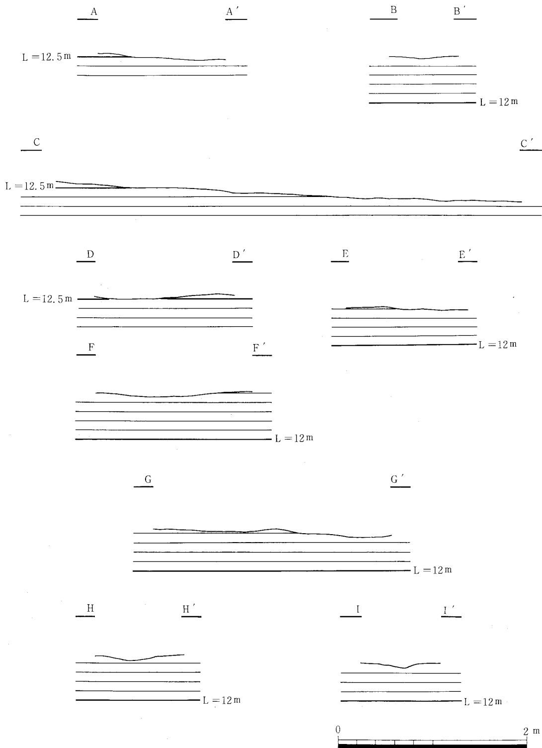
第15図 溝状遺構 1 ~ 3 断面図 (S = 1 / 40)
