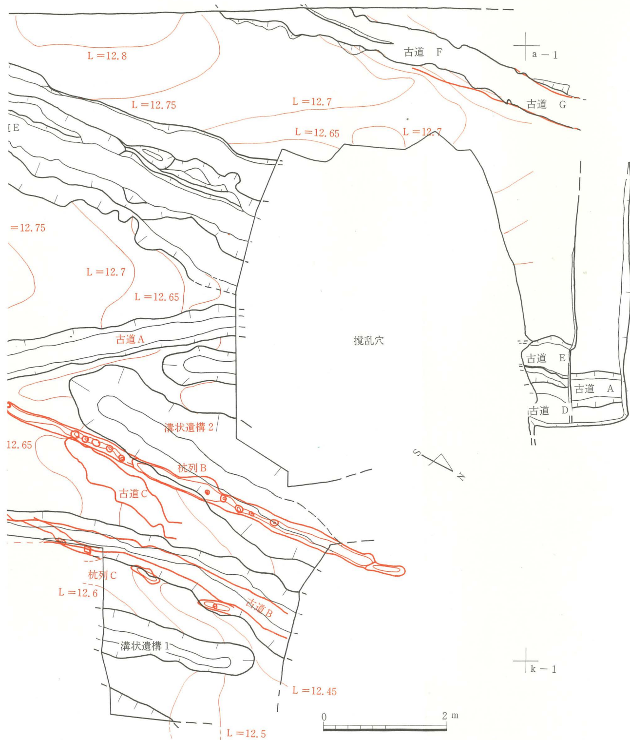
第6図 第6層検出遺構配置図 (S=1/60)
