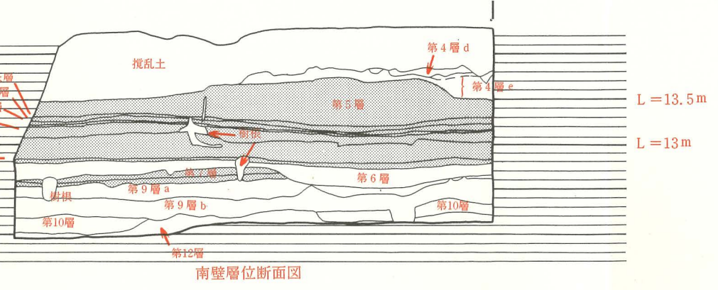
第5図 調査区層位断面図 (S=1/60)
