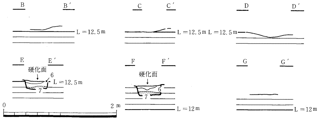
第9図 古道B断面図 (S = 1/40)
