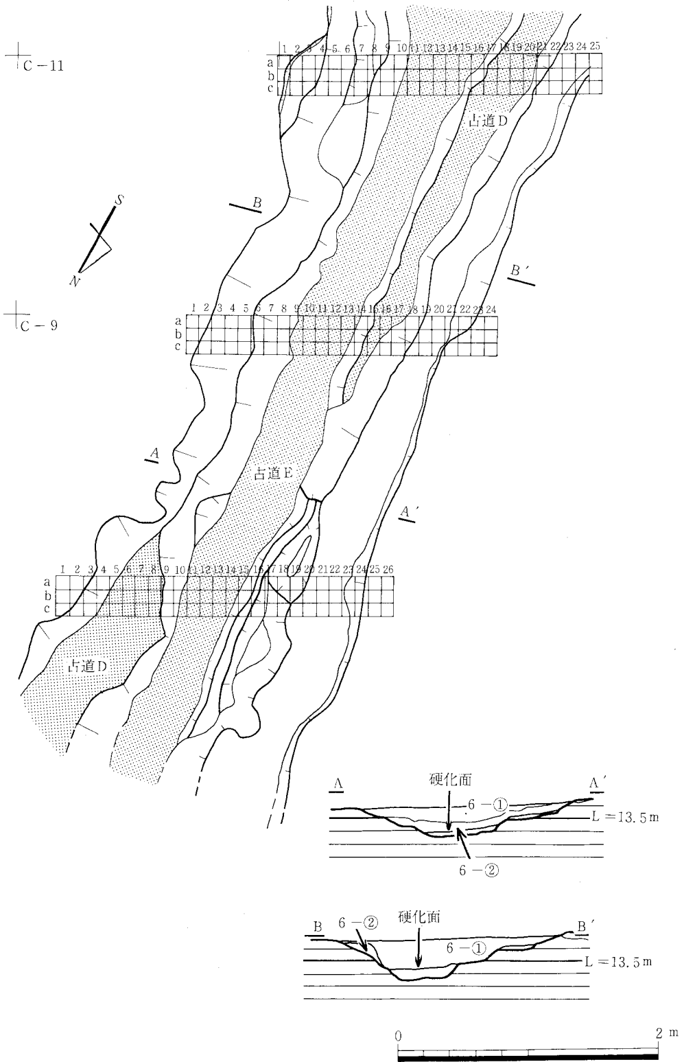
第11図 古道D, E平面図及び断面図 (S = 1 / 20)
