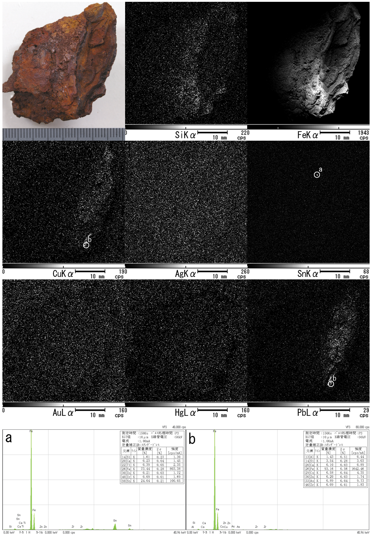
第11図 鉄剣基部近くの破断面の元素マッピング分析結果
