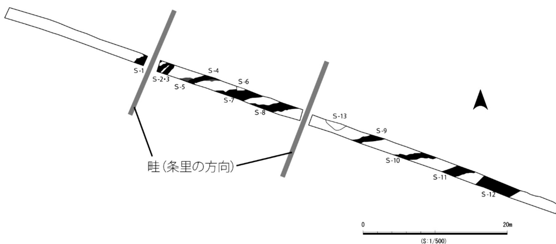
第4図 沖代地区条里跡50次調査遺構分布状況 (S=1/500)
