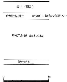
図10 1トレンチ南端東壁土層図
