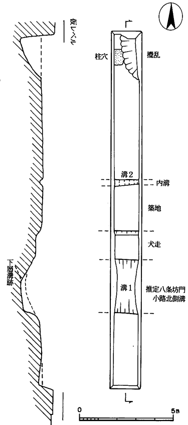
図20 調査平・断面略測図
