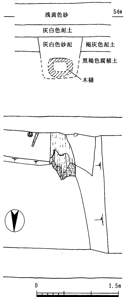
図30 2トレンチ木樋平面図・南壁土層図 (1/40)
