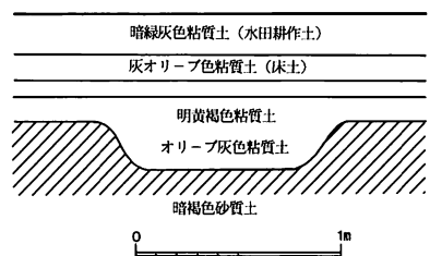
図39 トレンチ中央北壁土層図
