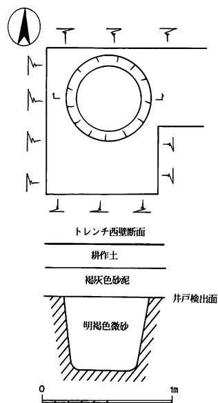
図40 井戸跡平・断面略測図
