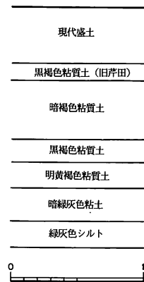
図21 溝1の東壁土層図
