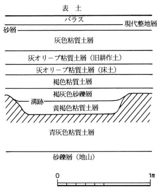
図15 溝跡部分南壁土層図
