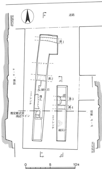
図9 調査平・断面実測図
