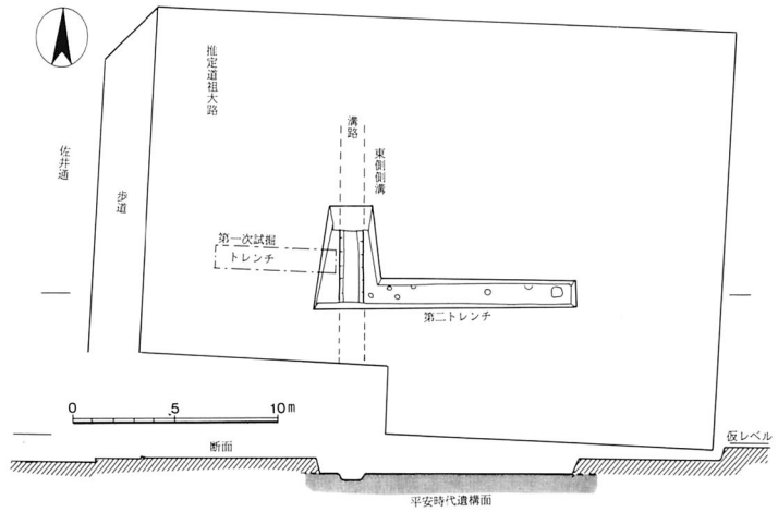
図14 調査平・断面実測図
