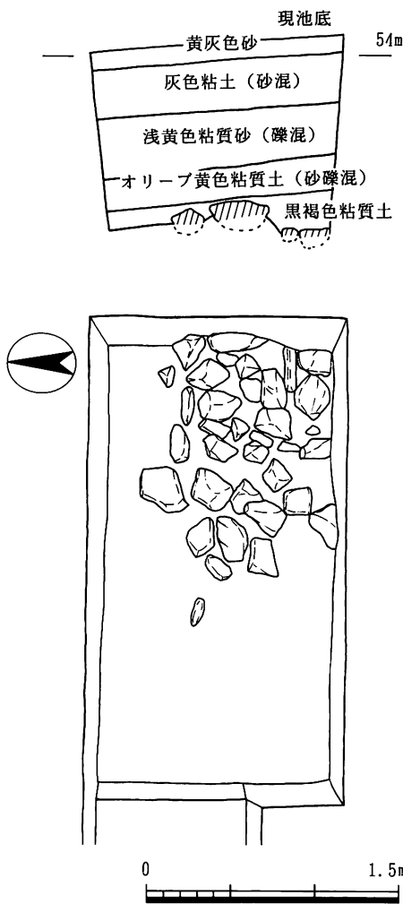
図29 1トレンチ東端部平面図・東壁土層図 (1/40)
