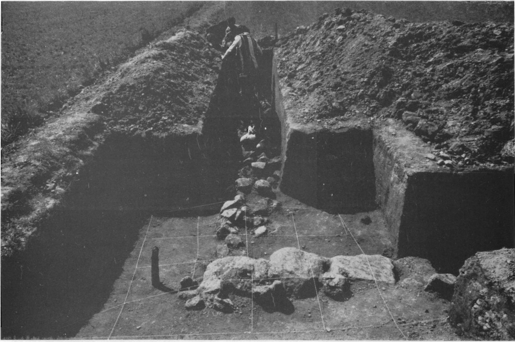
護岸工事に伴う石組遺構
