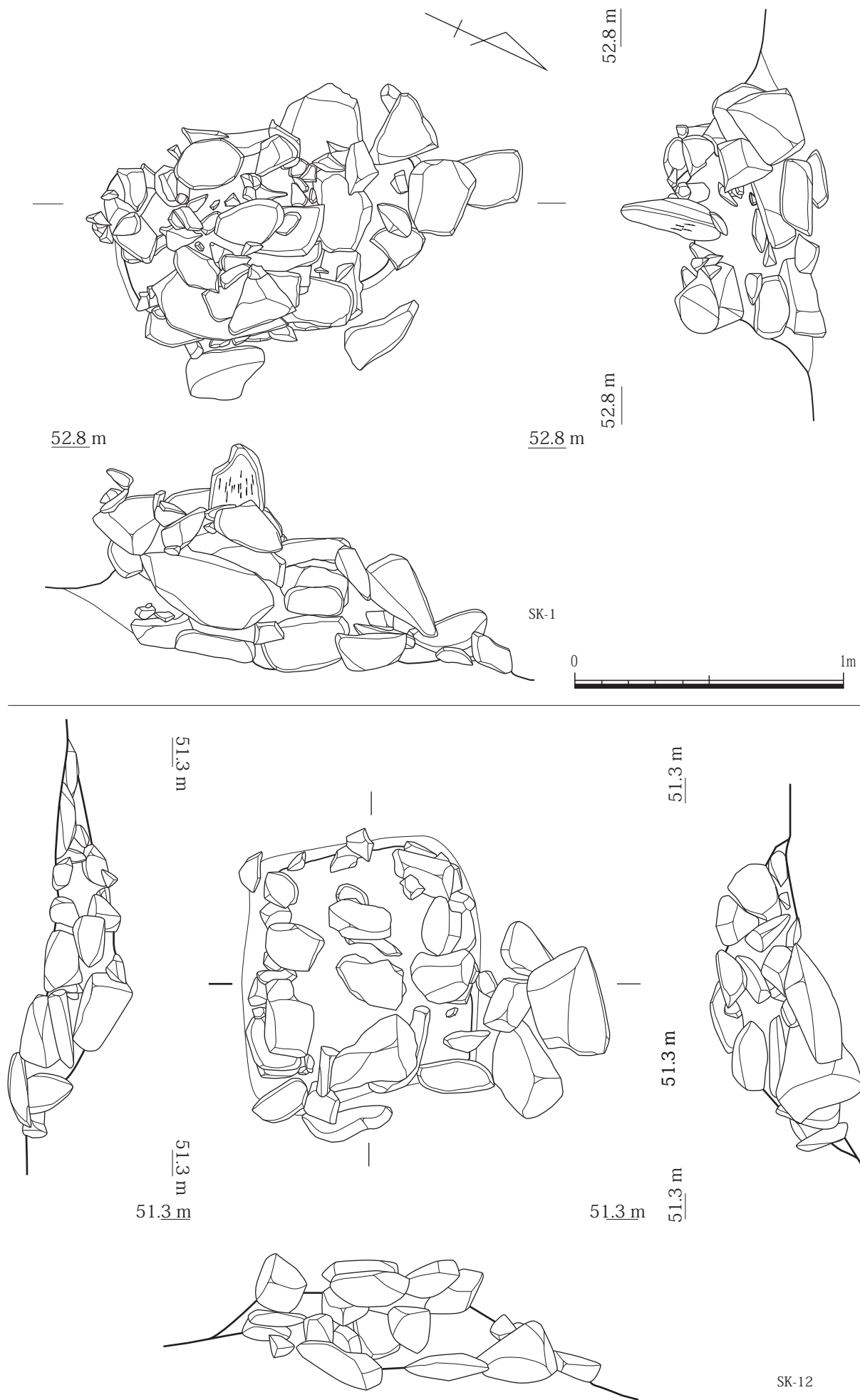
第7図 SK-1、12実測図(1/80)
