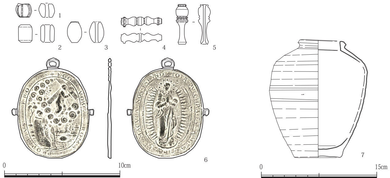
第 14 図 崎津小高浜出土遺物実測図 (1/2、1/3)
