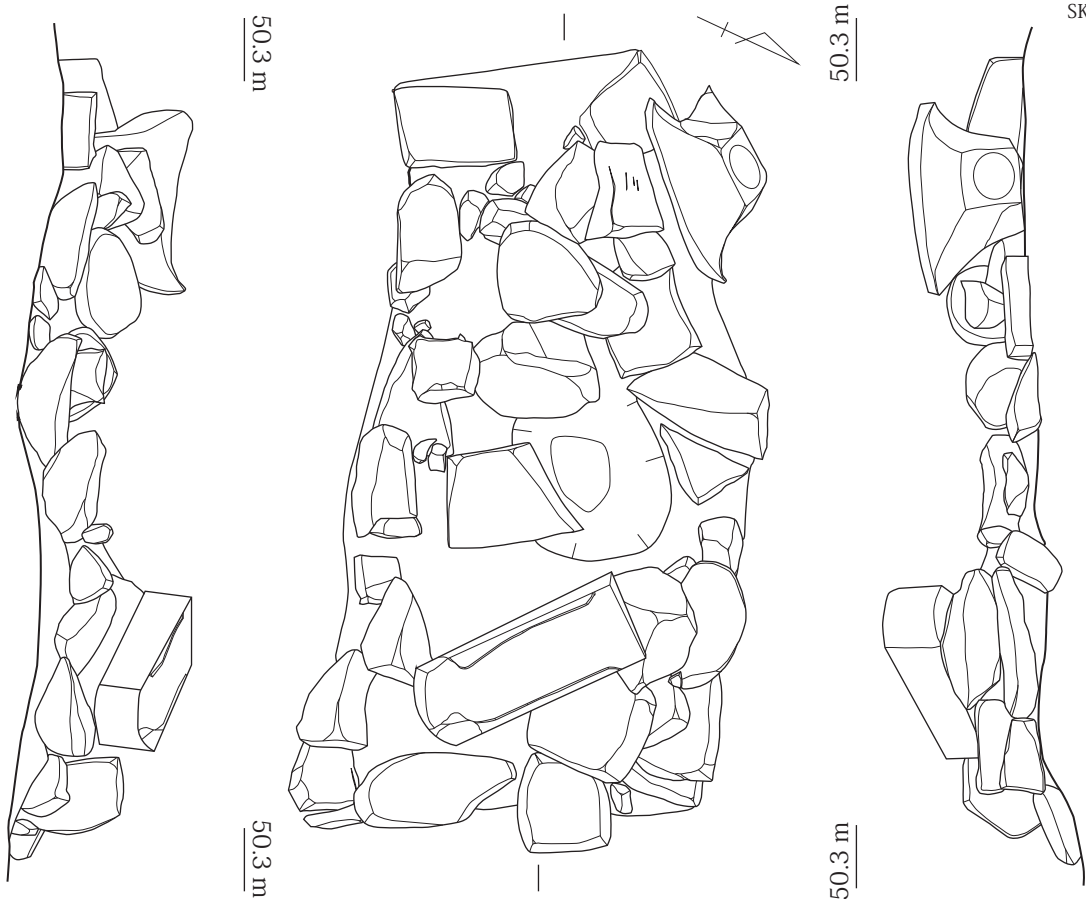
第10图 SK-17、18 实测图 (1/80)
