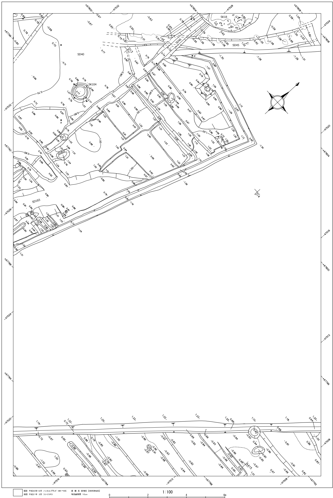
第181図 直江北遺跡 遺構平面図 No.63 [S=1/100]
