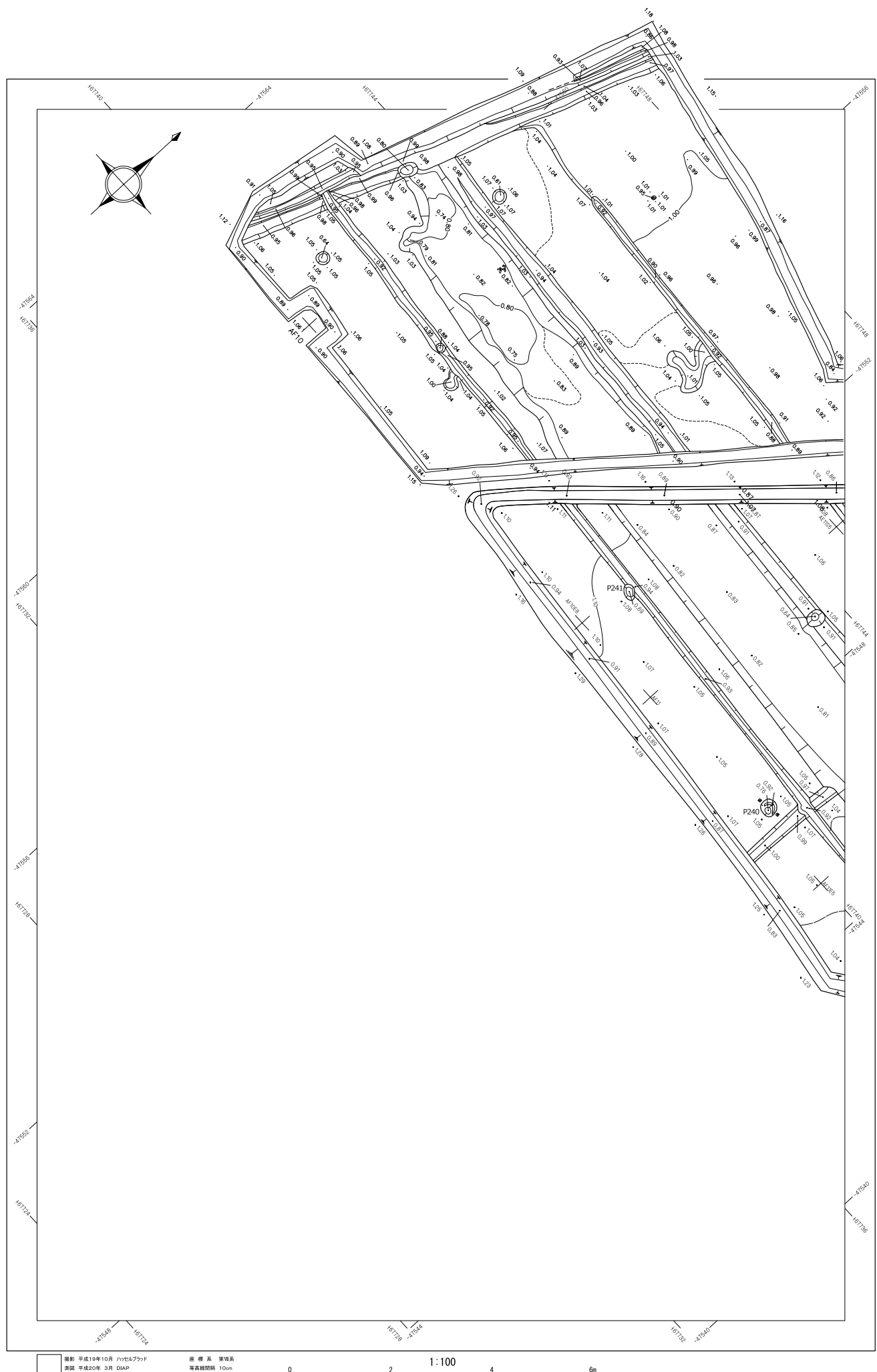
第 182 図 直江北遺跡 遺構平面図 No.64 (S=1/100)
