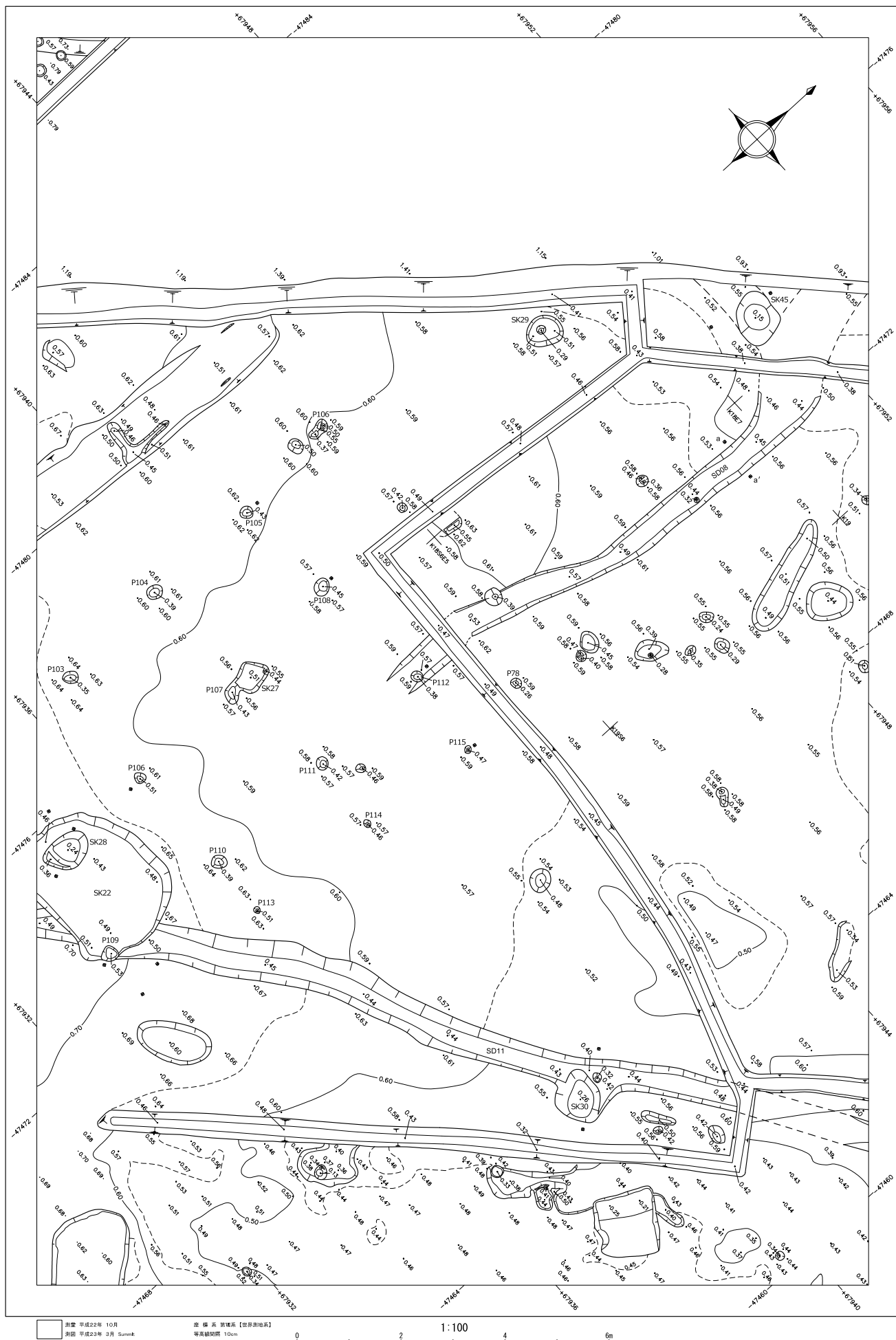
第144図 直江北遺跡 遺構平面図 No.26 (S=1/100)
