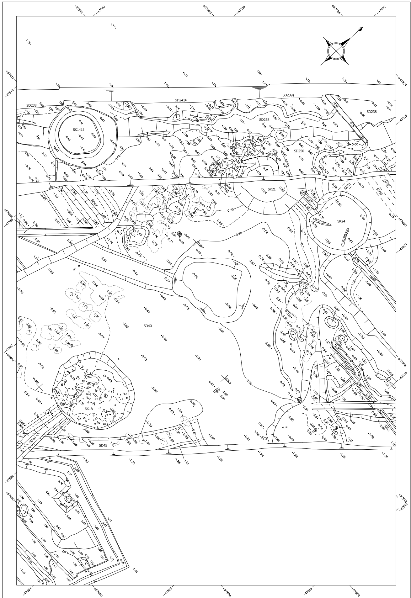
第163図 直江北遺跡 遺構平面図 No.45 [S=1/100]
