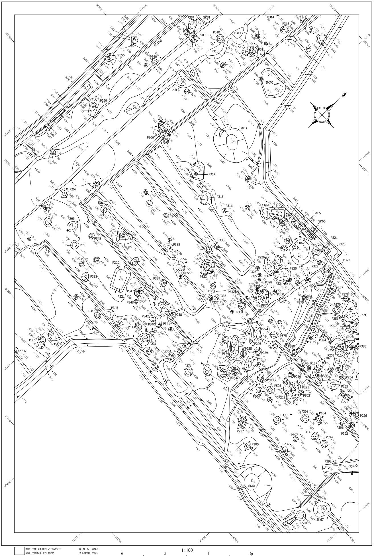
第 202 図 直江北遺跡 遺構平面図 No.84 (S=1/100)
