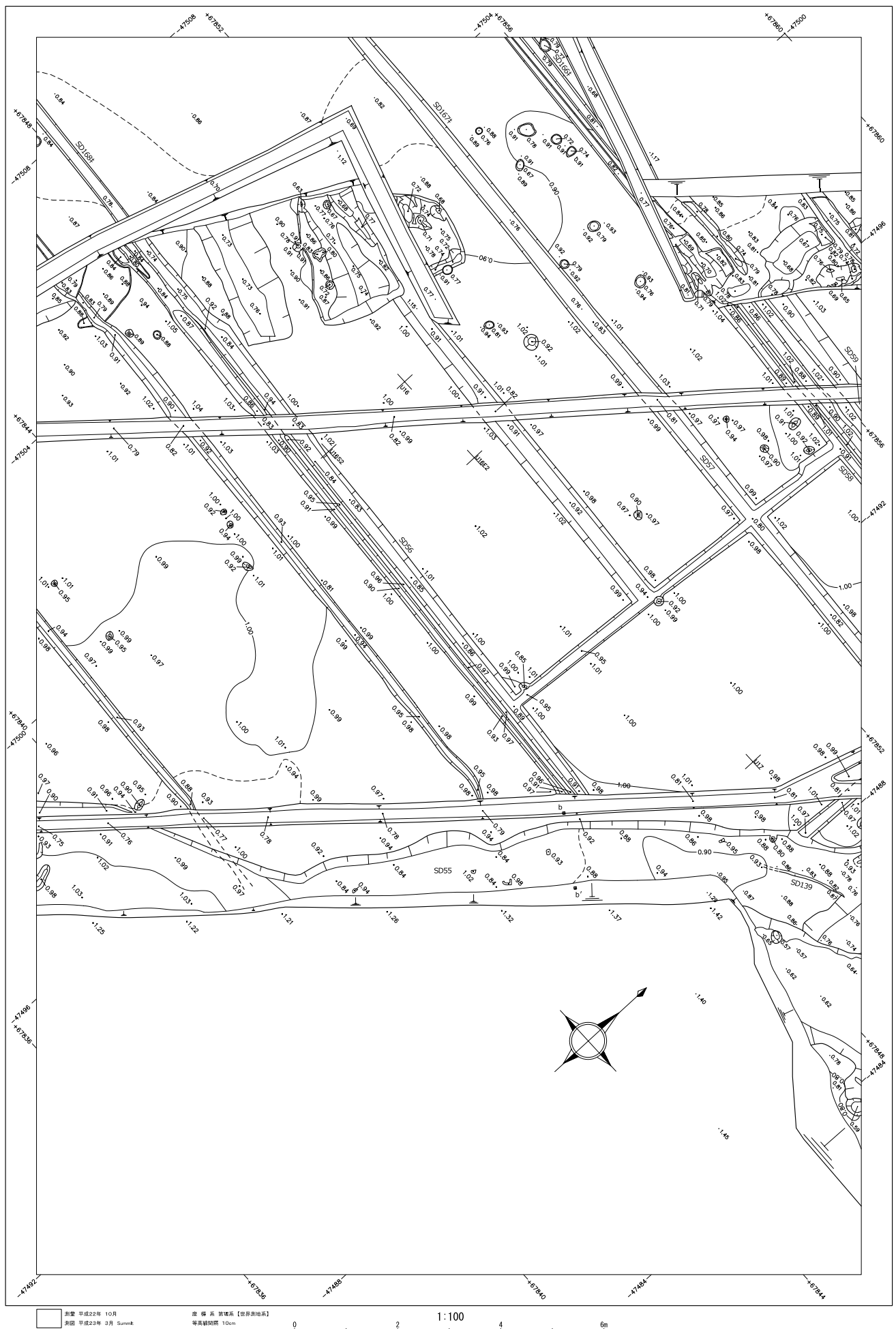
第 166 図 直江北遺跡 遺構平面図 No.48 [S=1/100]
