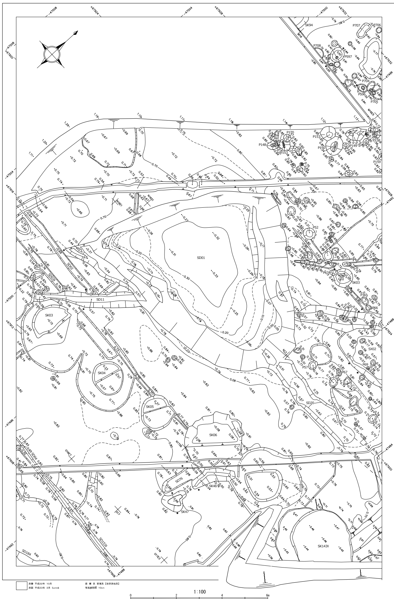
第 142 図 直江北遺跡 遺構平面図 No.24 [S=1/100]
