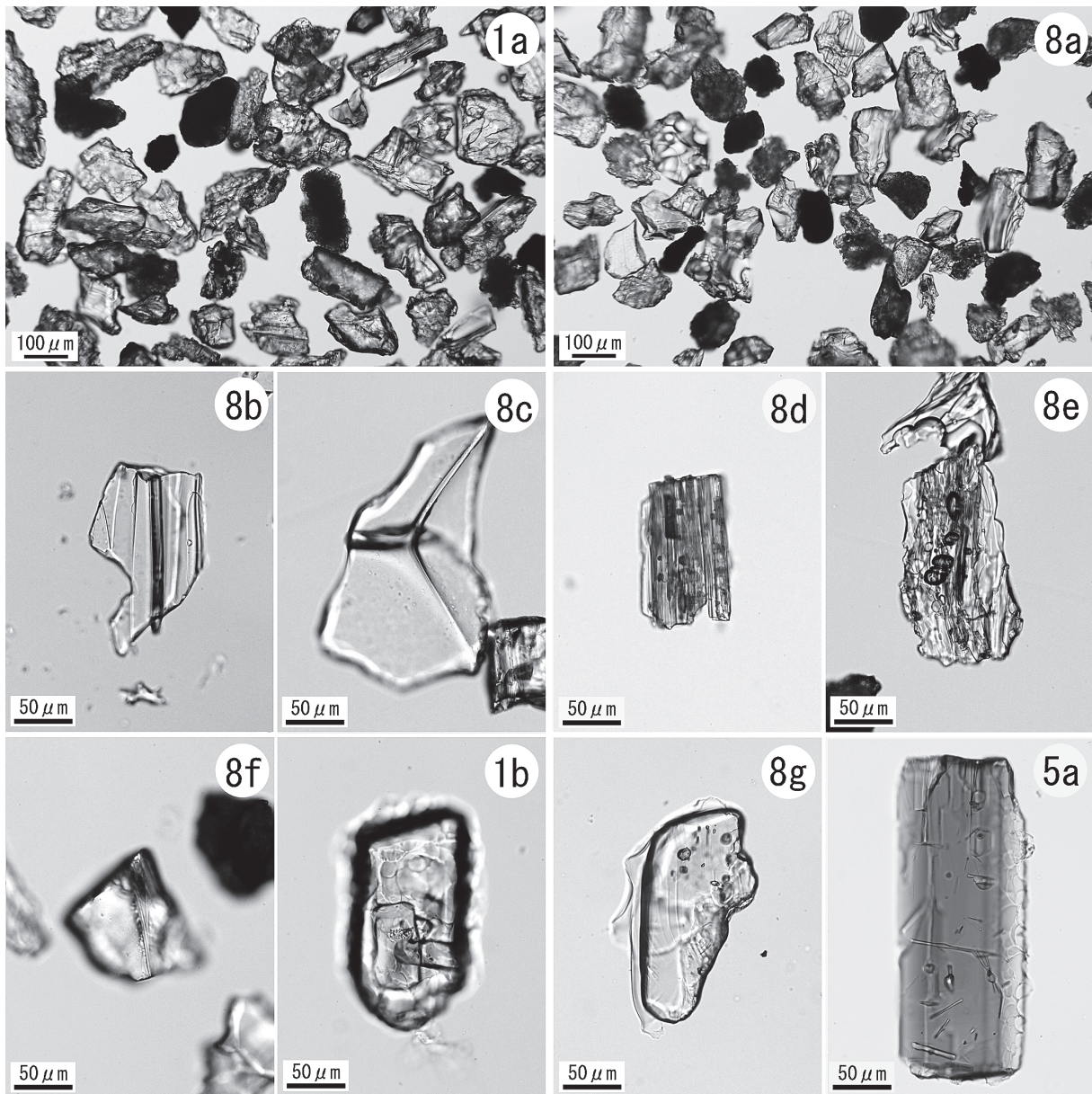
1a. 分析 No.1 (試料 No.7) 8a. 分析 No.8 (試料 No.15) 8b. バブル型平板状ガラス (分析 No.8) 8c. バブル型Y字状ガラス (分析 No.8) 8d. 軽石型繊維状ガラス (分析 No.8) 8e. 軽石型スポンジ状ガラス (分析 No.8) 8f. 急冷破碎型フレーク状ガラス (分析 No.8) 1b. 斜方輝石 (分析 No.1) 8g. 単斜輝石 (分析 No.8) 5a. 角閃石 (分析 No.5)
