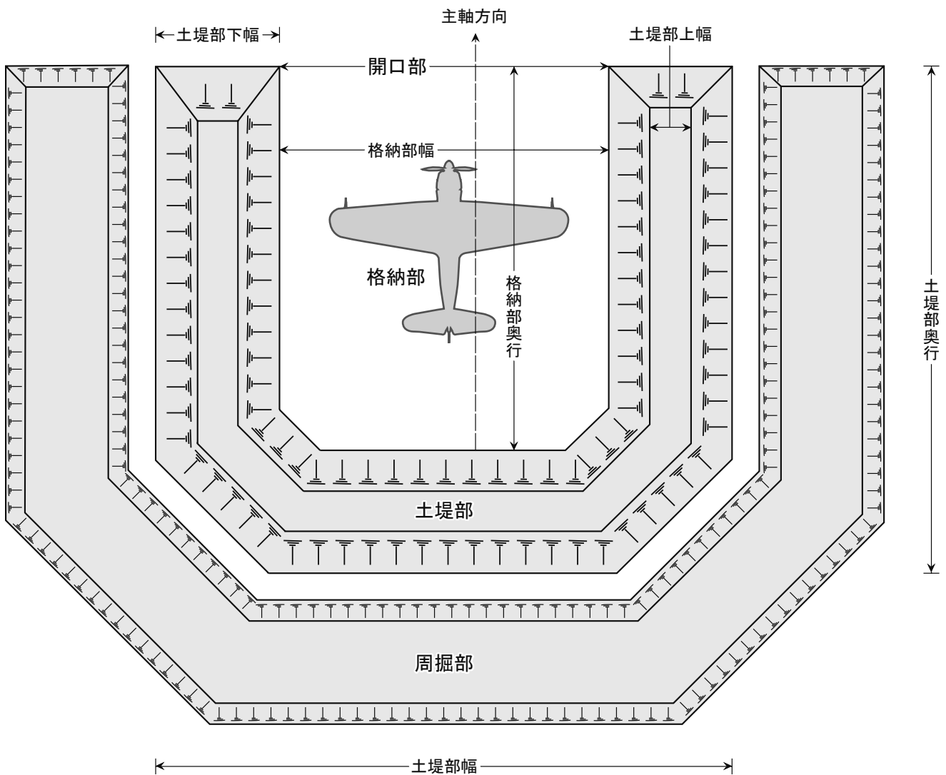
第4図 C字型無蓋掩体壕の模式図
