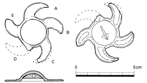
図3 宮平遺跡出土 巴形銅器 (S=1/2)
