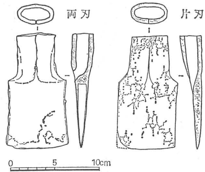
Fig. 57 両刃と片刃の鉄斧 (『メスリ山古墳』報告書より)
