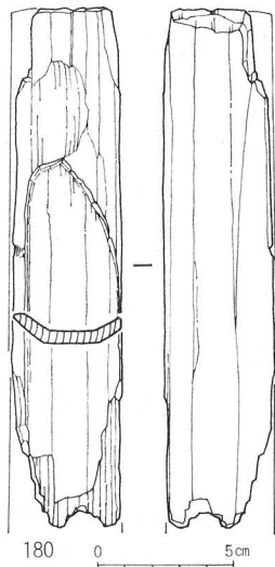
Fig. 34 刀鞘実測図
