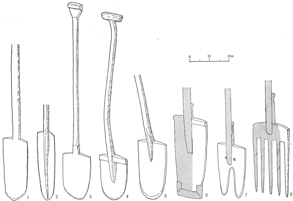
Fig. 60 鋤・フォーク状木器模式図
