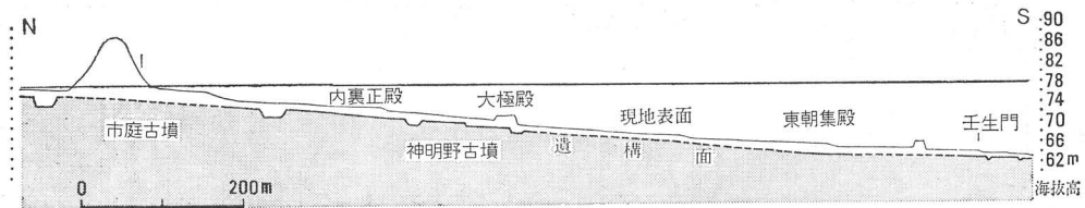
Fig. 38 第二次朝堂院・内裏地区の南北高低差模式図
