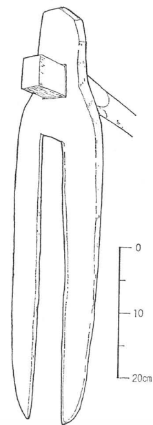
Fig. 59 北部九州の股鍬模式図 (板付第2区遺跡)
