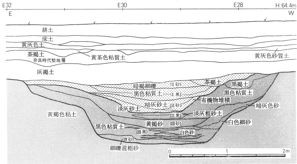
3 S D 6030南区土層図
