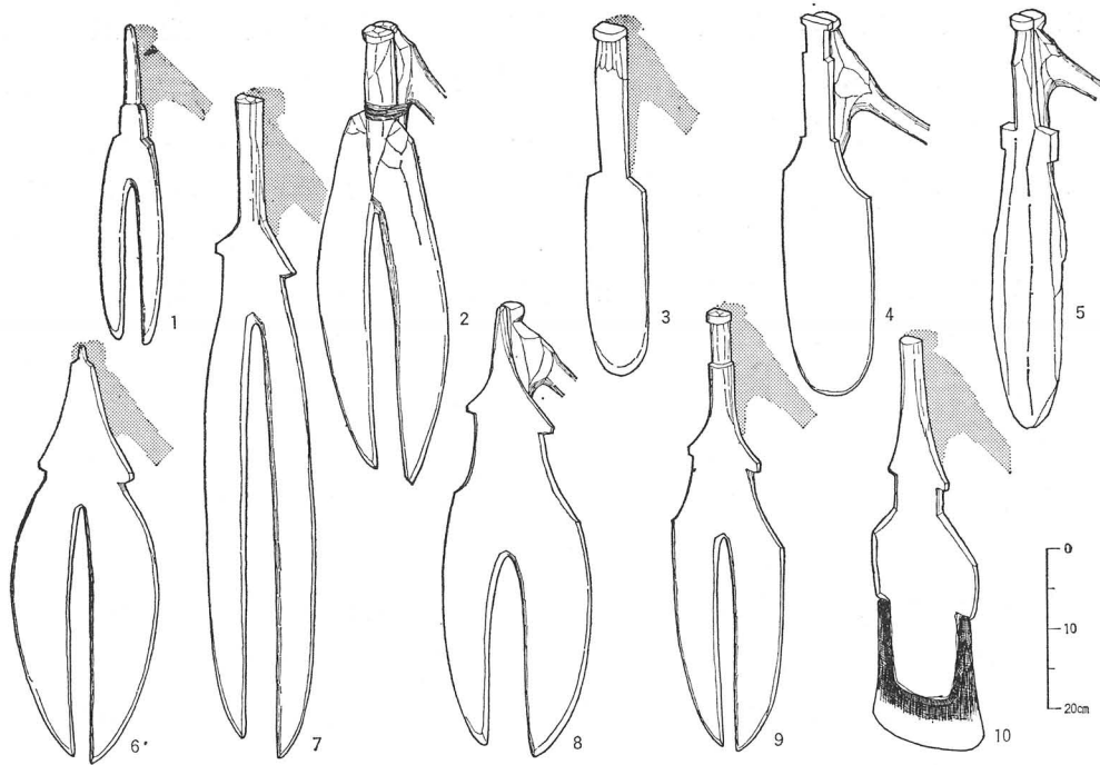
Fig. 58 膝柄鋏と膝柄股鋏模式図
