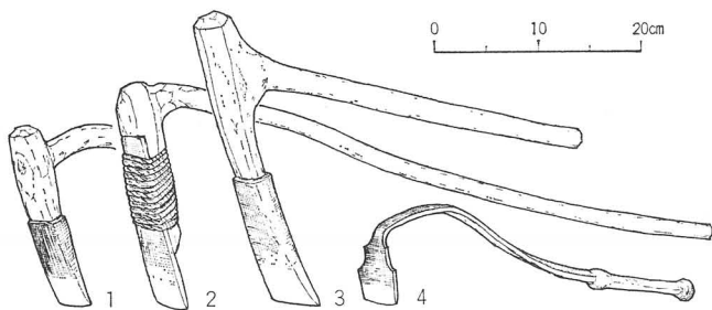
Fig. 56 横斧模式図
