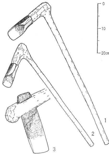
Fig. 55 縦斧模式図
