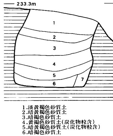
第8圖 袋状竖穴遺構実測圖
