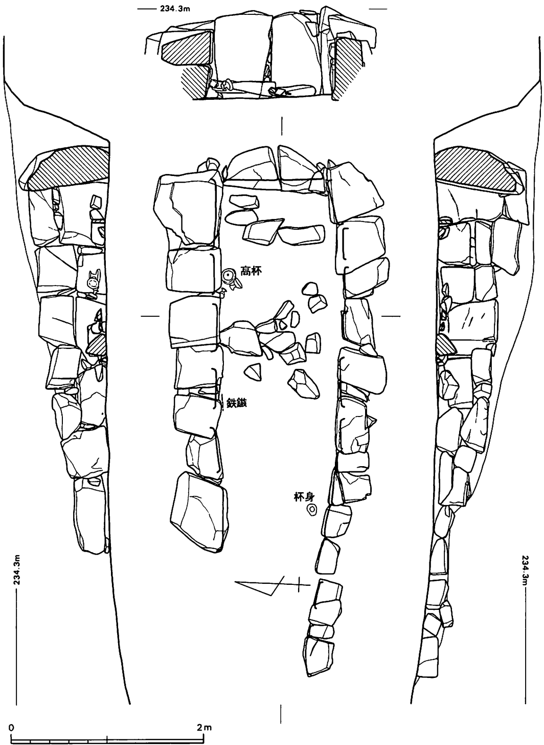
第25圖 ST03石室實測圖
