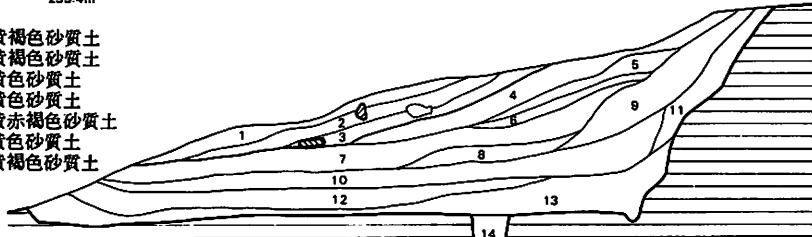
第6図 SB10実測図
