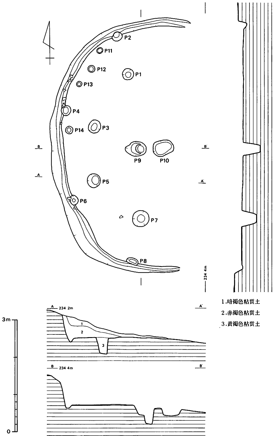
第15图 SB01实测图
