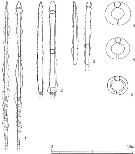
第26図 ST03出土遺物実測図
