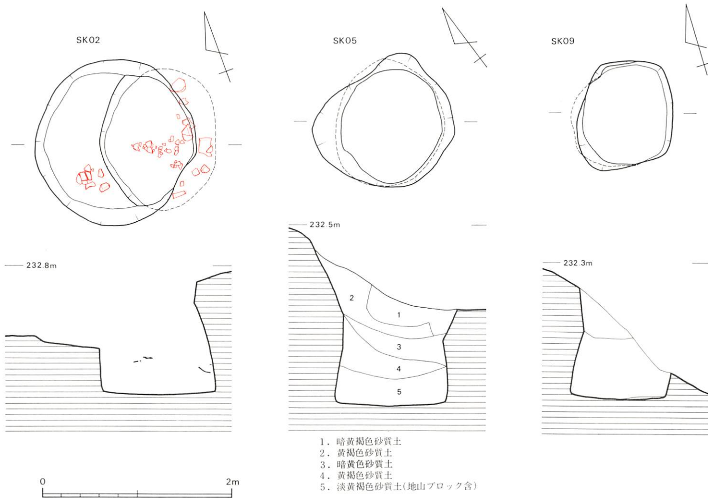
第7図 袋状竖穴遺構実測図
