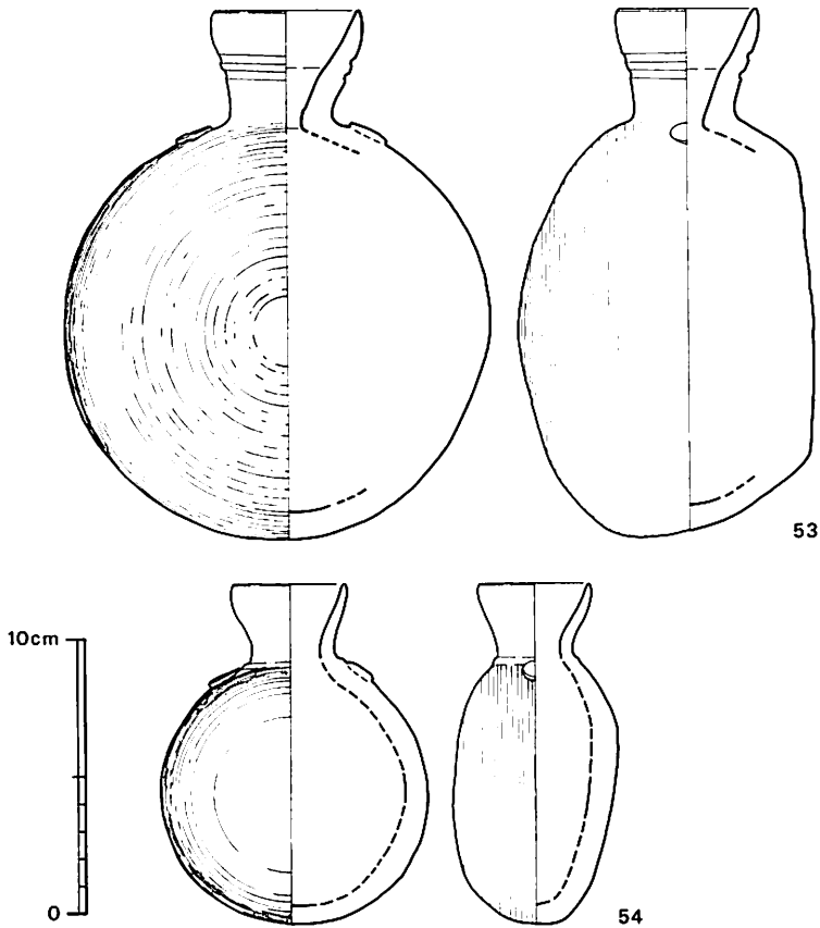
第28図 ST03出土遺物実測図
