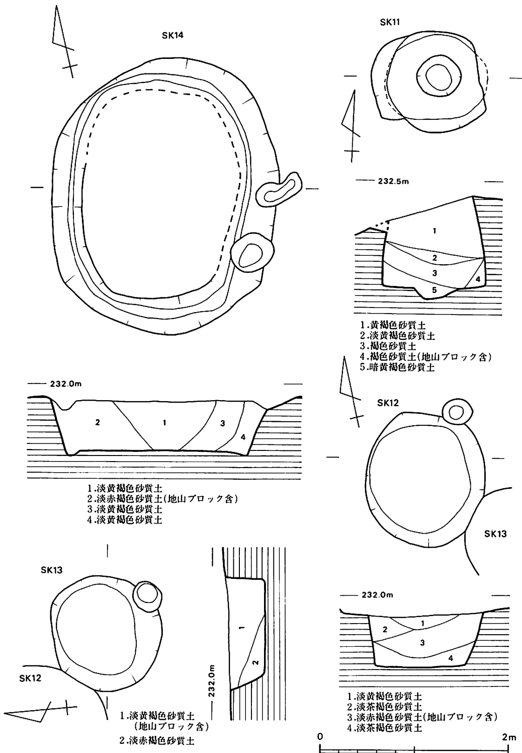
第9図 袋状堅穴遺構実測図
