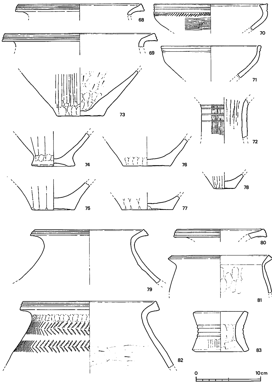
第20图 SB02、03出土土器夷测图
