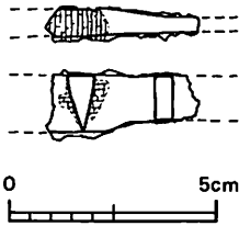
第18図 SB03出土鉄器 実測図
