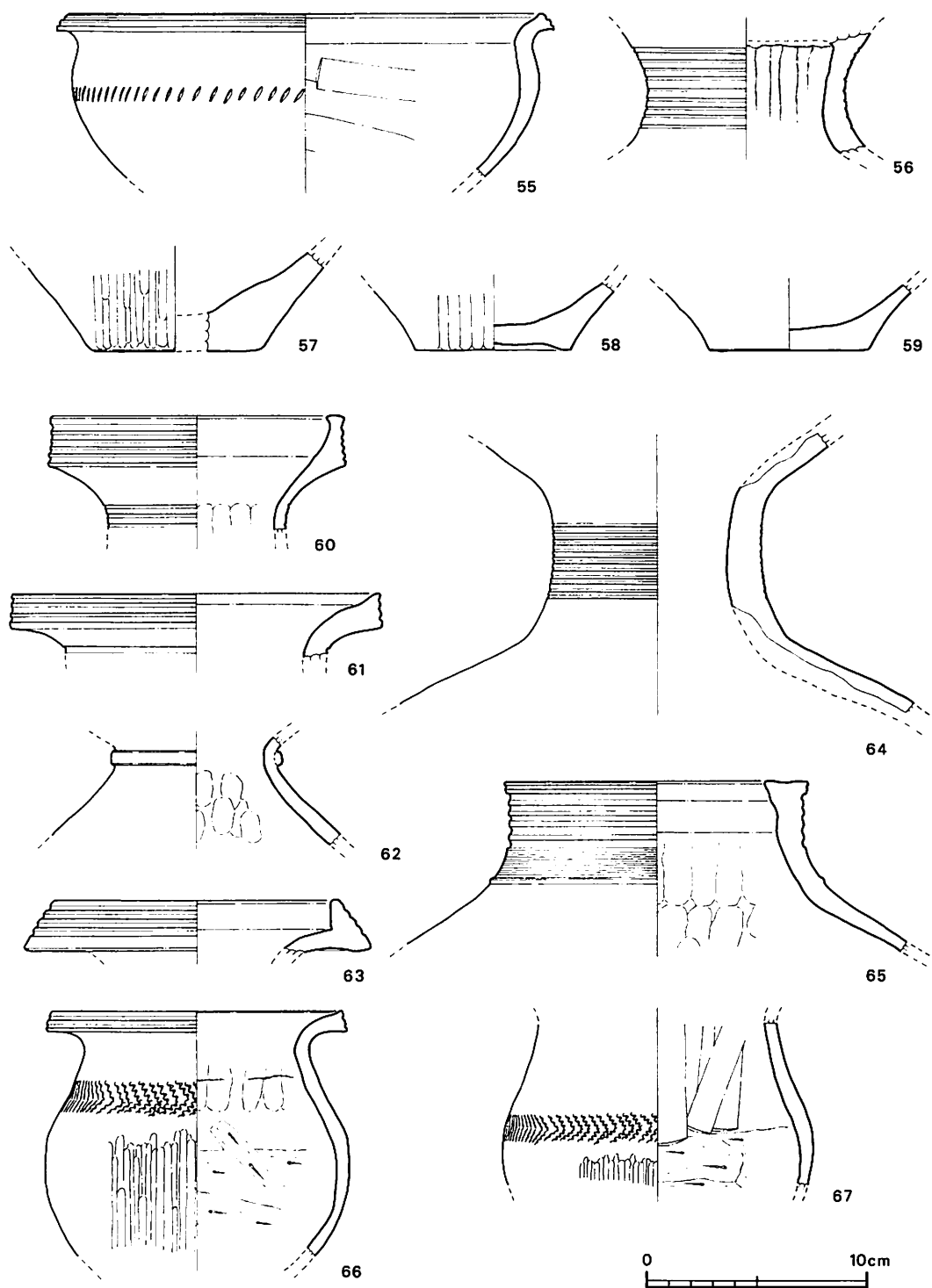
第19图 SB01、02出土土器实测图
