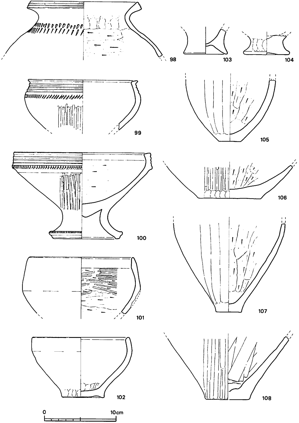
第23图 土器集中部出土土器实测图
