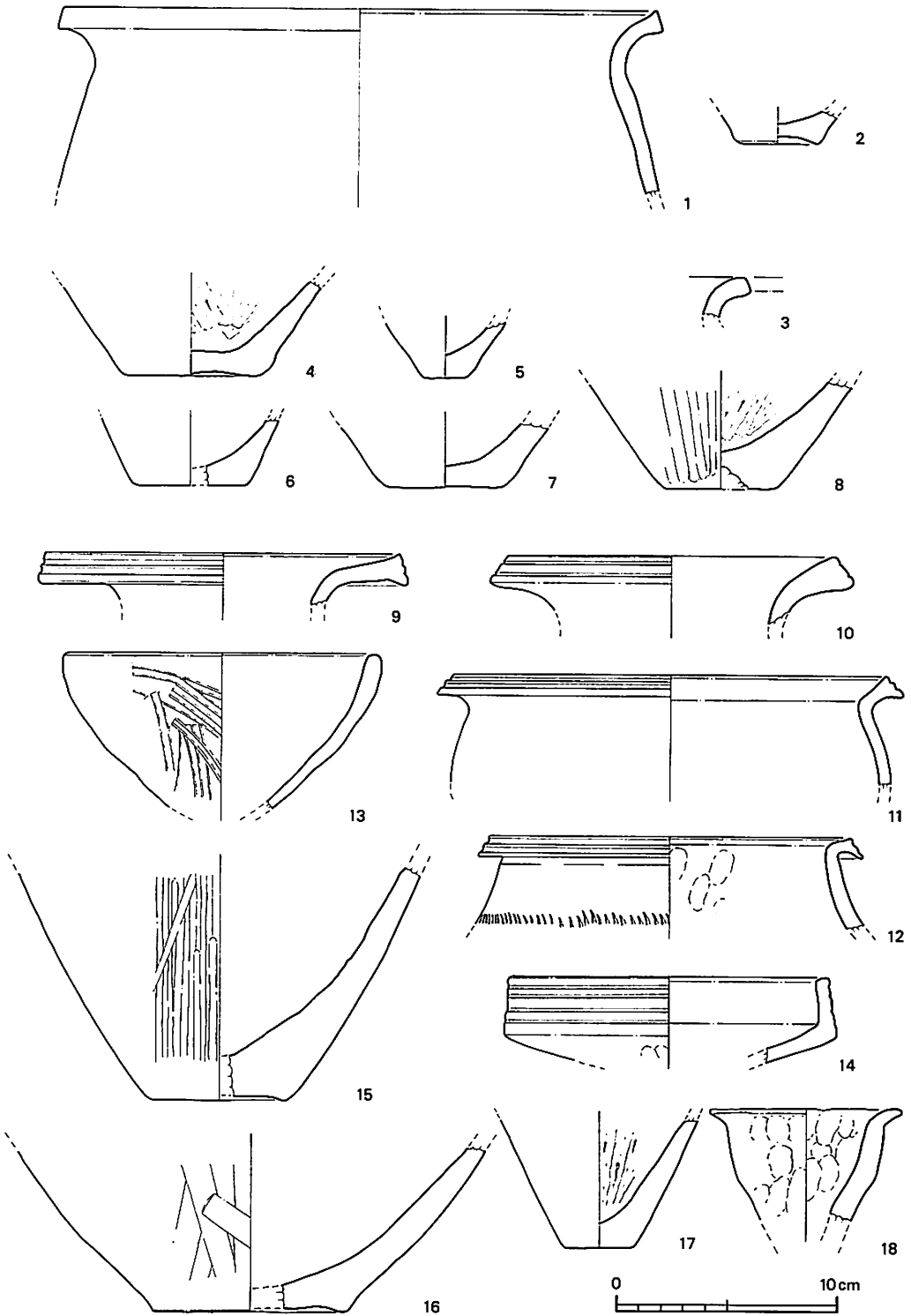
第10图 SB01、04、10出土土器实测图
