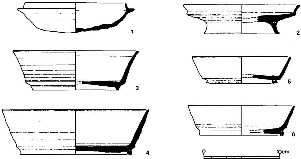
第2図 上下町内出土遺物実測図(1:3)
