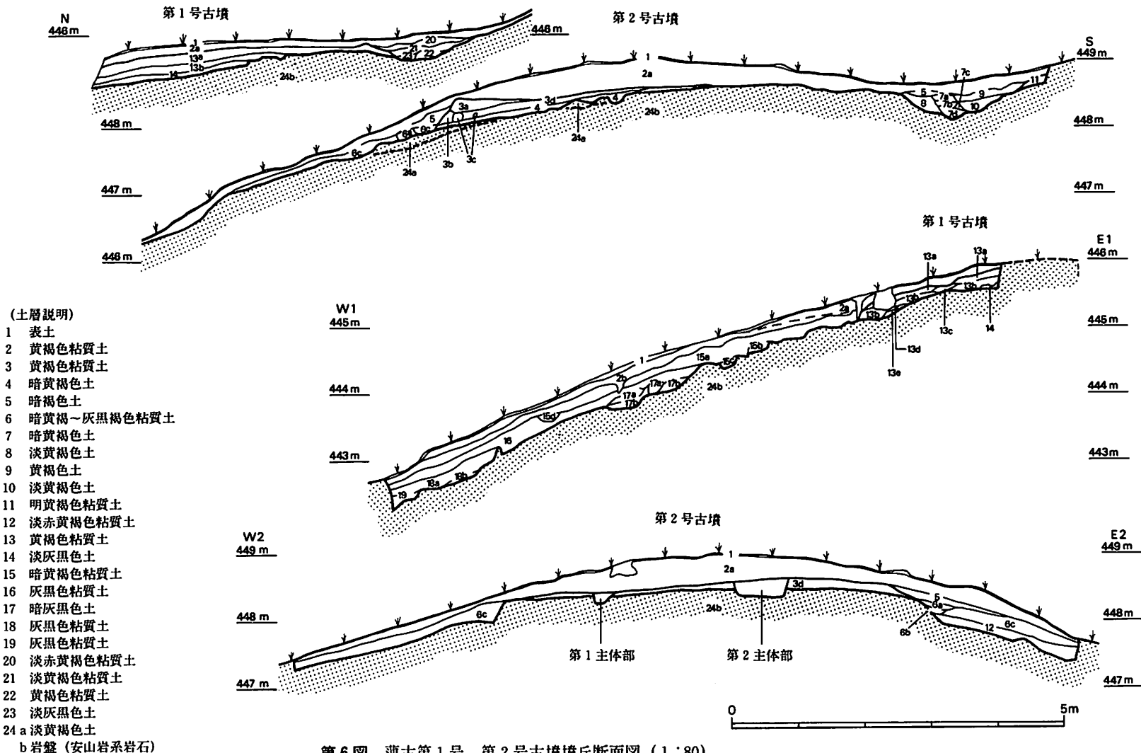
第 6 图 薄古第 1 号, 第 2 号古墳墳丘断面图 (1 : 80)
