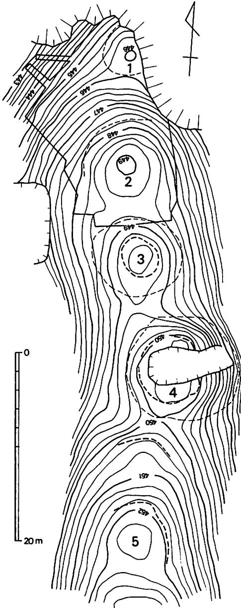
第4図 薄古墳群地形測量図 (1:400)
