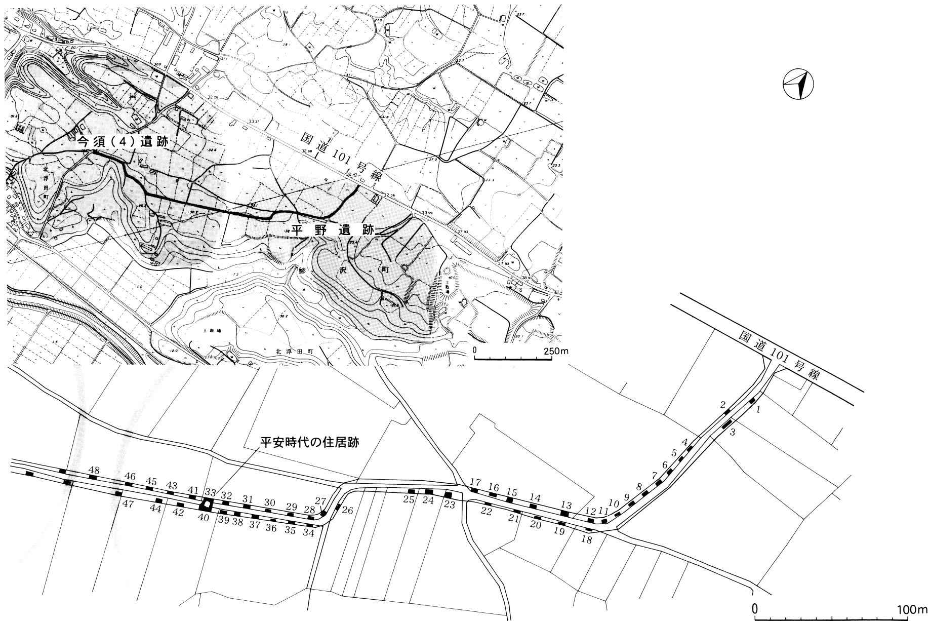
図3 平野遺跡トレンチ配置図
