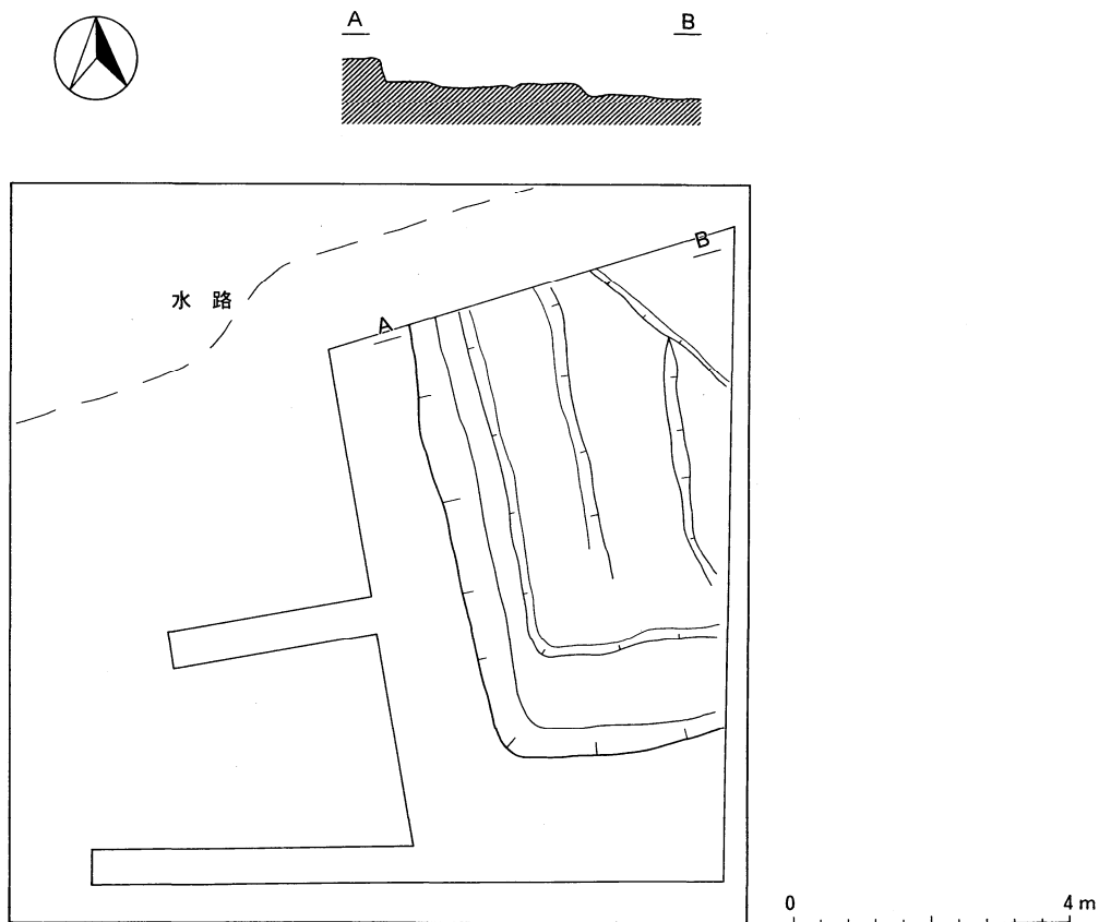
図8 沖館A線No.2 鉄塔調査区域図
