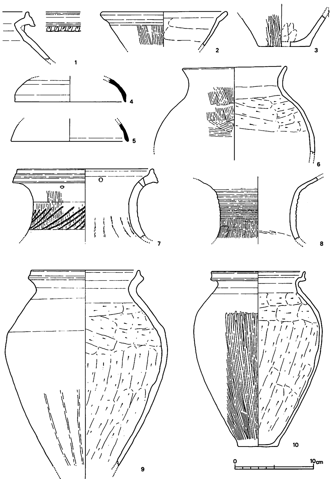
第16图 出土土器实测图(I) (1:3) (1~3:SB01、4~6:SB02、7~10:SB03)
