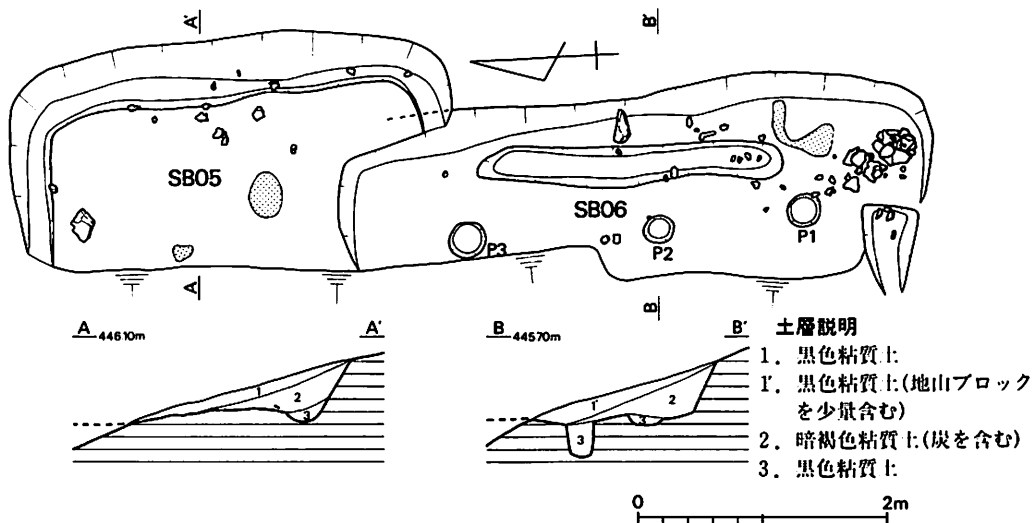
第 9 図 SB05・06 実測図(1:60)(アミ目:焼土)
