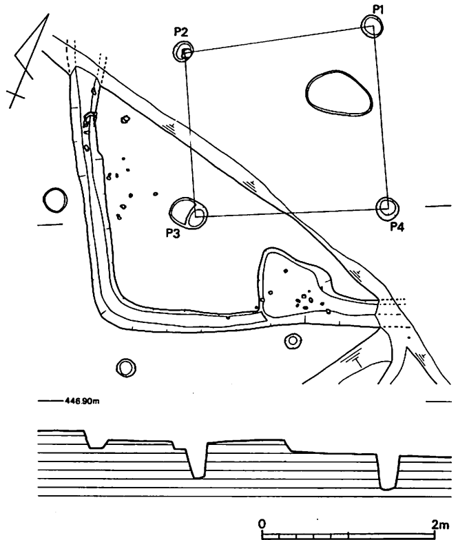
第6図 SB02 実測図(1:60)
