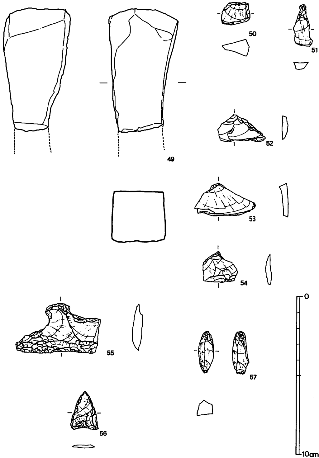
第20图 出土石器实测图(2:3) (49:SB02、50:SB03、51:SK10、52:SK11、53:SD01、54:SD02、55~57包含层)
