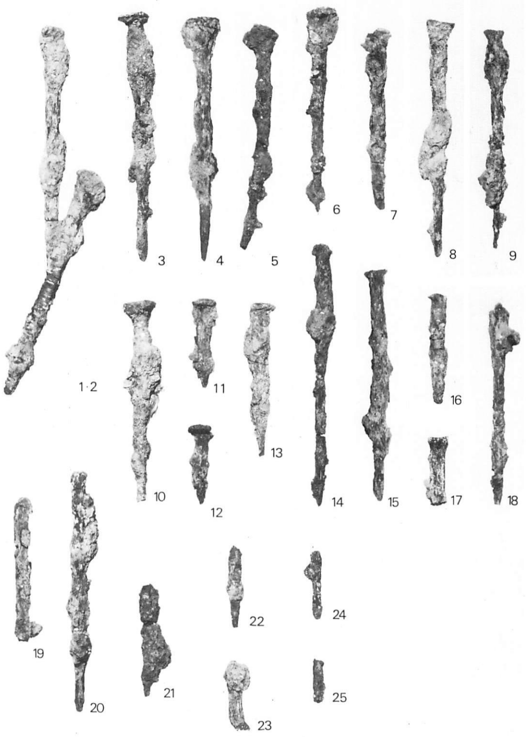
第18図 第2号古墳出土遺物 鉄釘
