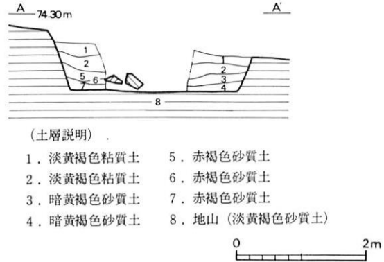
第10図 第2号古墳石室掘り方土層断面図 (1:80)
