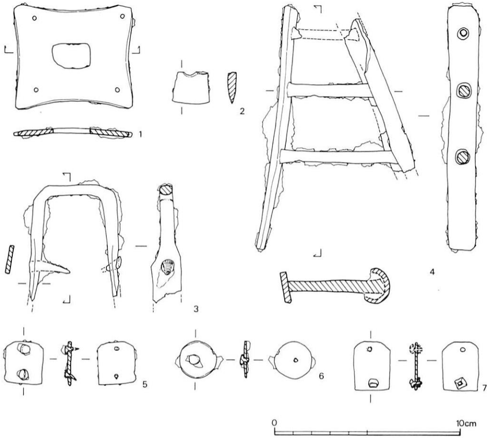
第44図 第5号古墳出土遺物実測図(4) (1:2) (周溝内) 鉄製品
