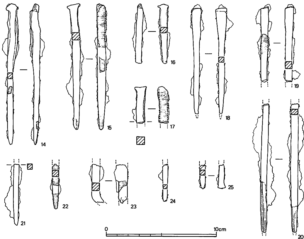
第17図 第2号古墳出土遺物実測図(3) (1:2) 鉄釘
