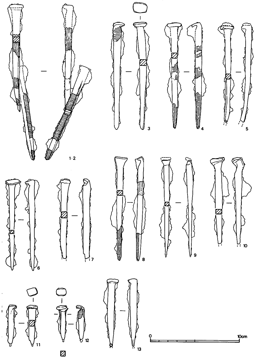
第16圖 第2号古墳出土遺物実測圖(2) (1:2) 鐵釘
