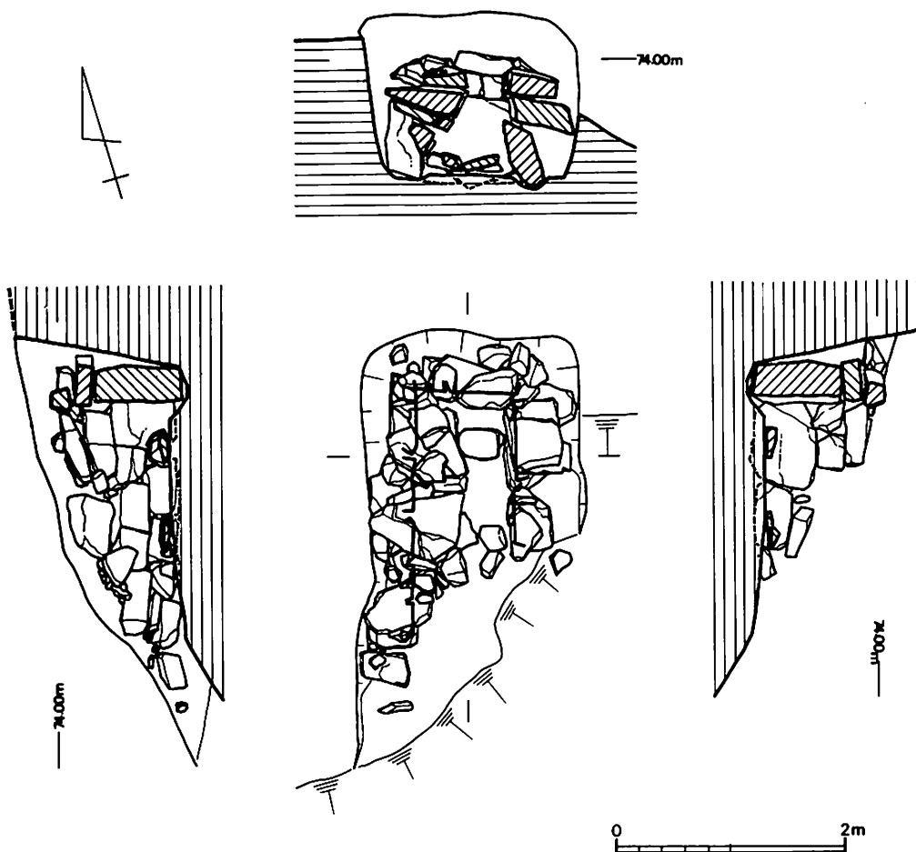
第22図 第4号古墳石室実測図（1：60）
