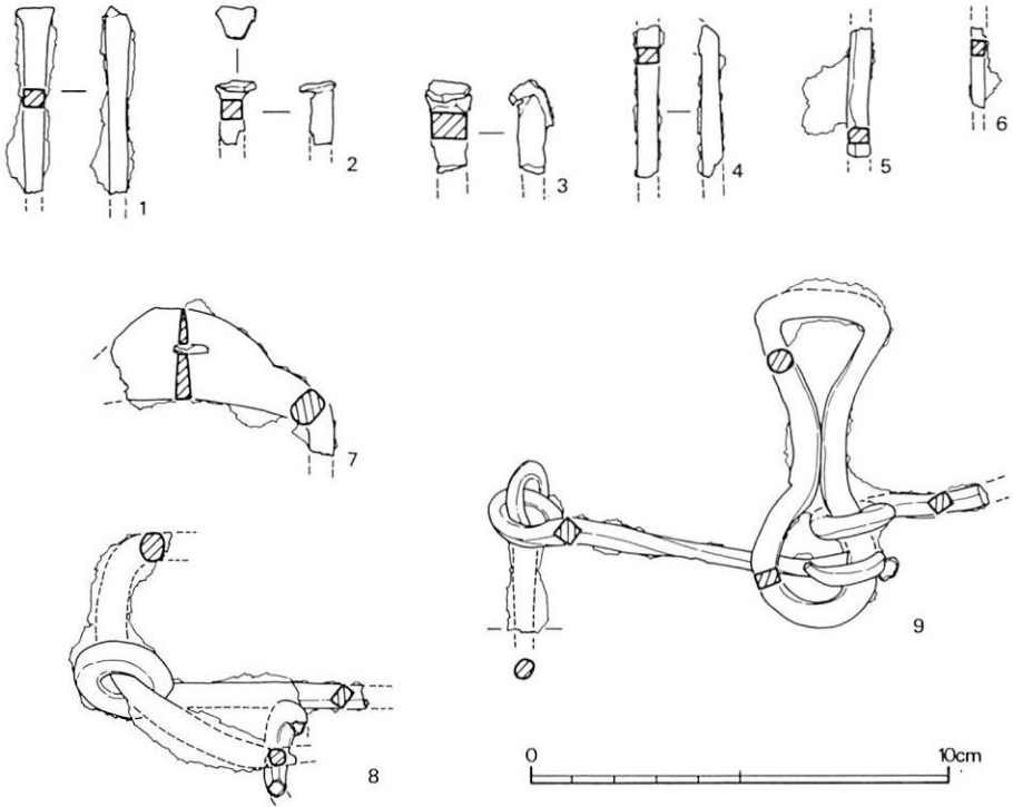
第26图 第4号古墳出土遺物実測図(1:2)鉄製品
