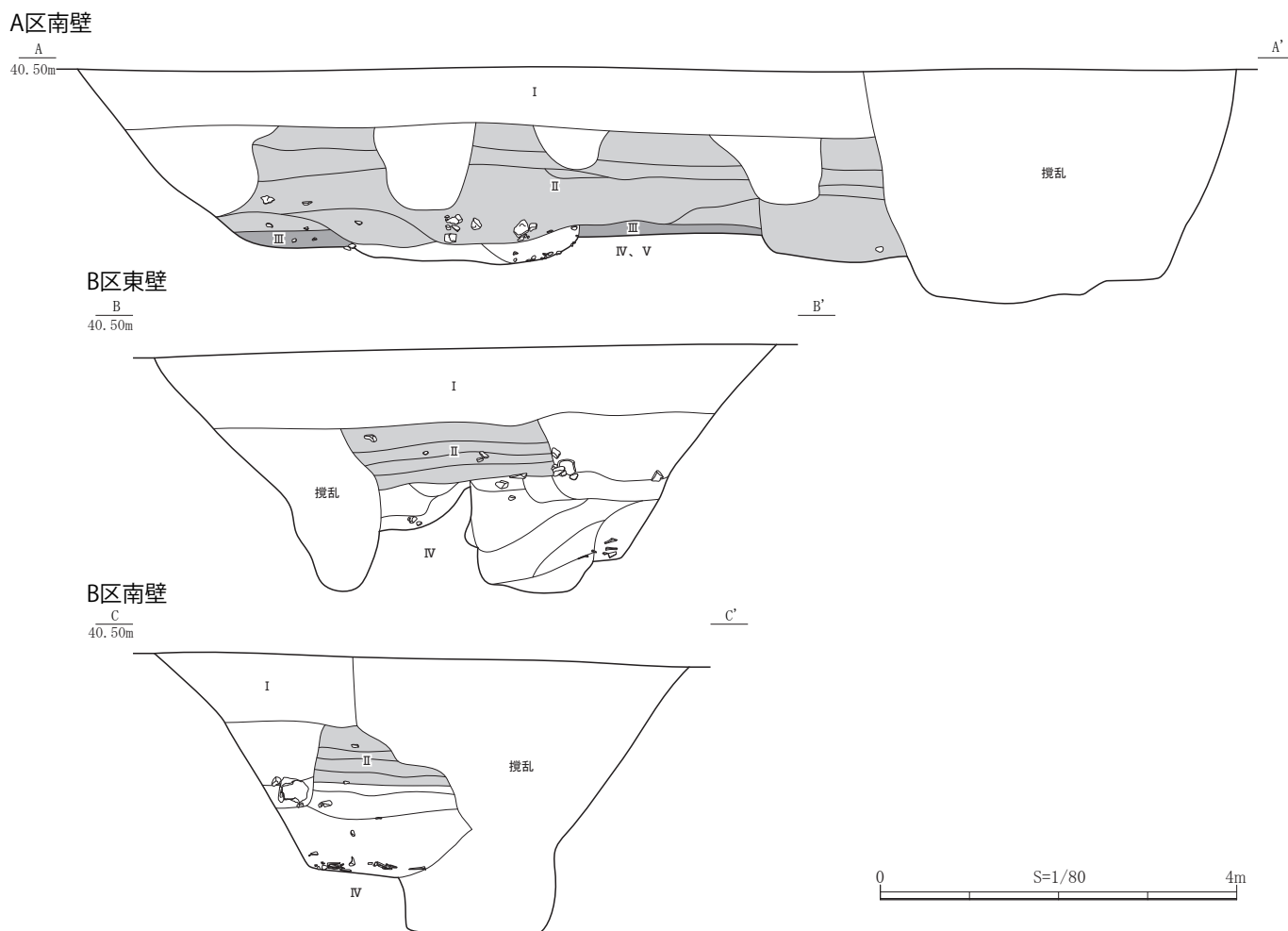
第5図 基本土層図 (縮尺 1/80)
