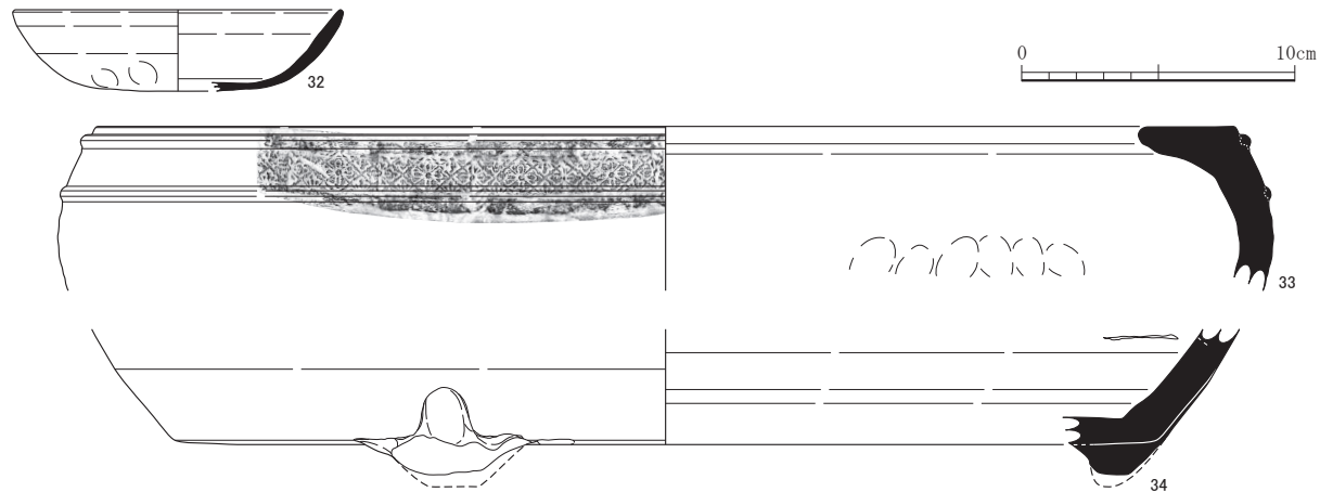
第 15 図 第 2 面出土遺物実測図 1（縮尺 1/3）
