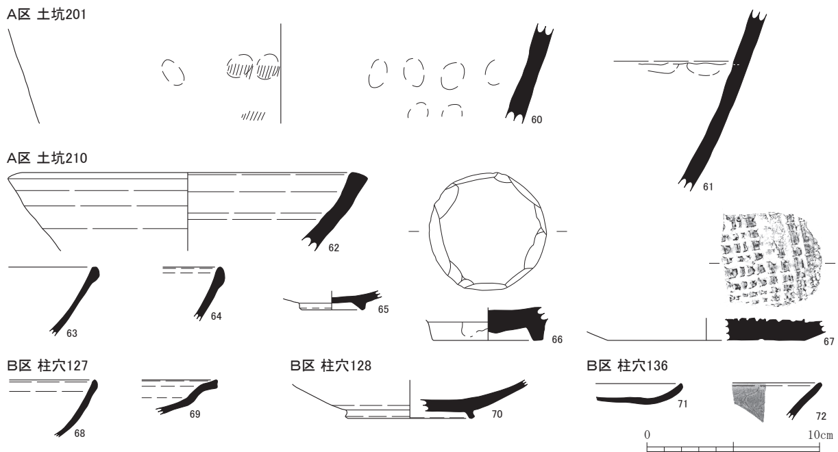
第 17 図 第 2 面出土遺物実測図 3 (縮尺 1/3)
