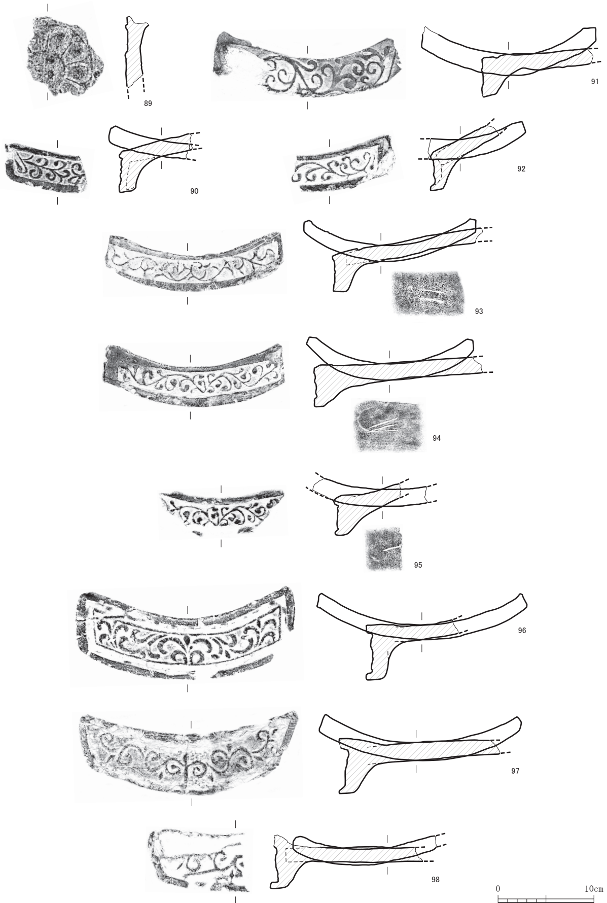
第20图 出土瓦实测图2 (缩尺1/4)
