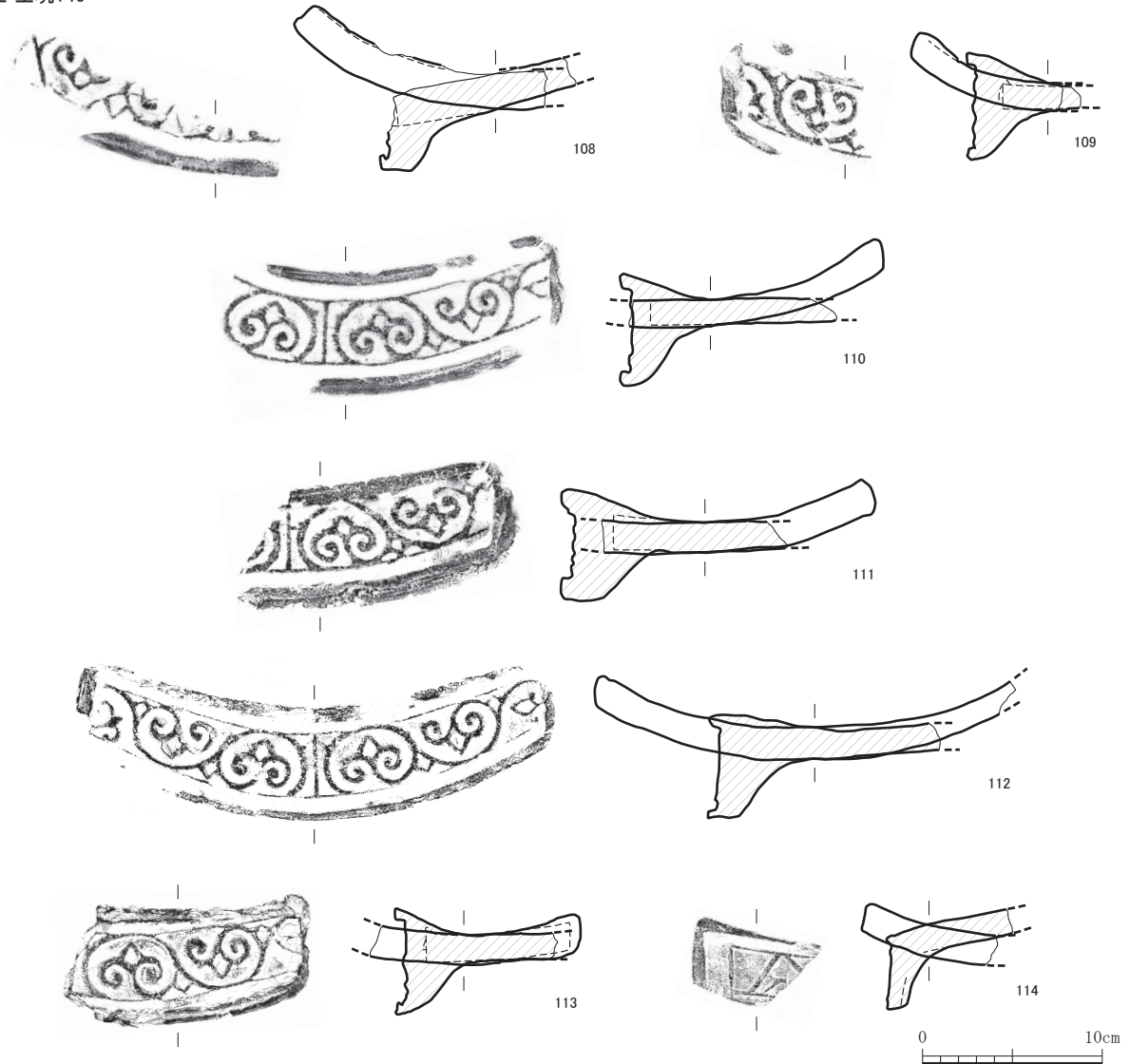
第22図 出土瓦実測図4 (縮尺1/4)
