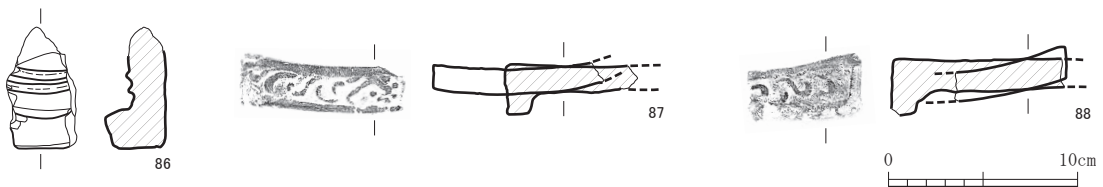
第 19 図 出土瓦実測図 1 (縮尺 1/4)
