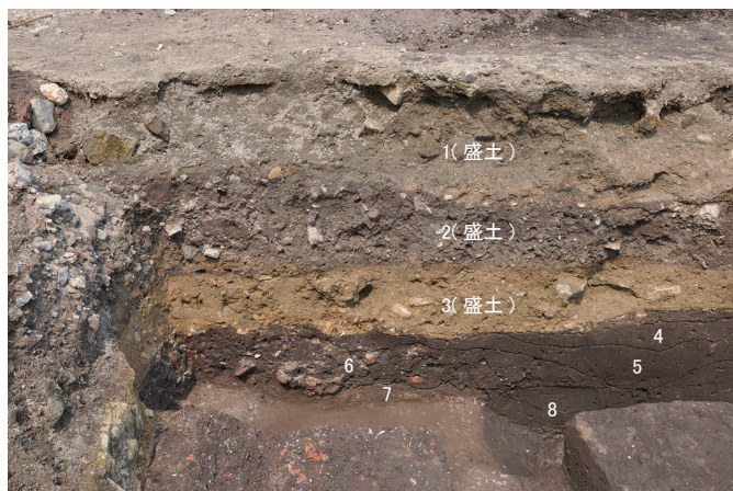
⑥ 25トレンチ北壁断面状況（南から）
