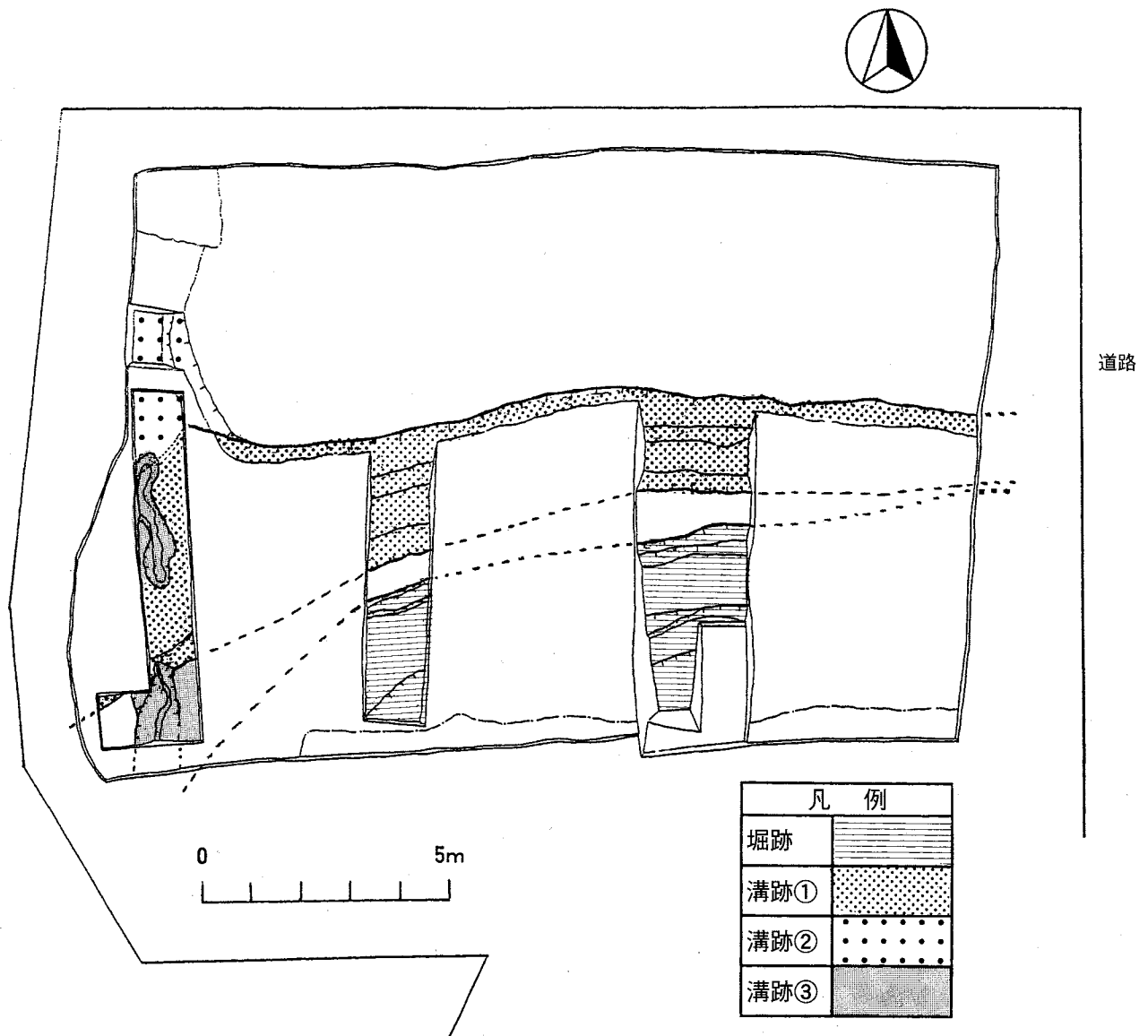
第13図 里館遺跡第52次調査区全体図
