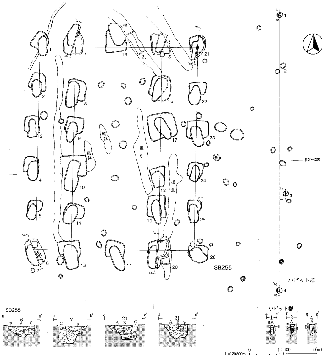
第3図 志波城跡第100次調査区SB255掘立柱建物跡・小ピット群
