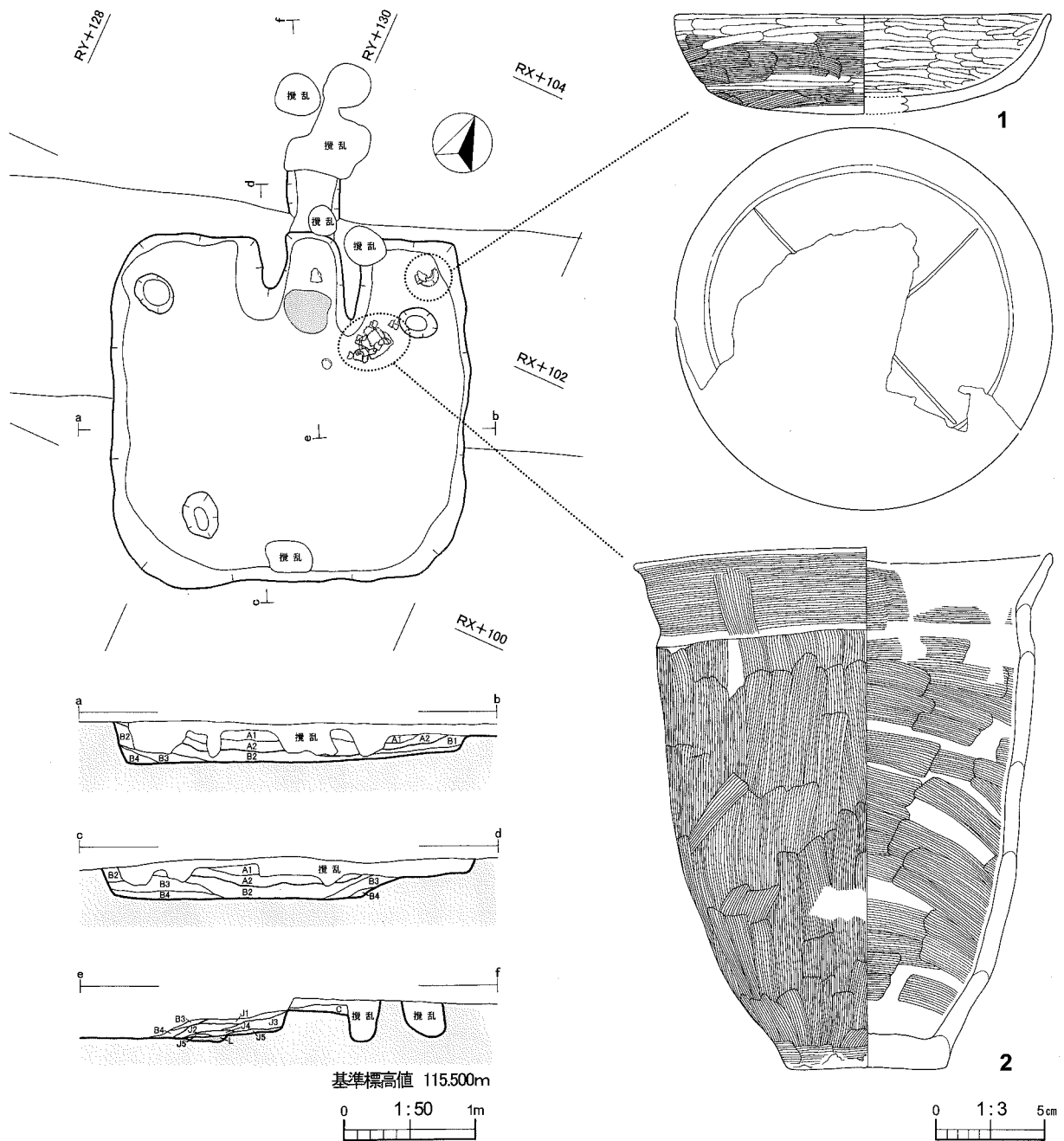
第4図 RA042 住居跡
