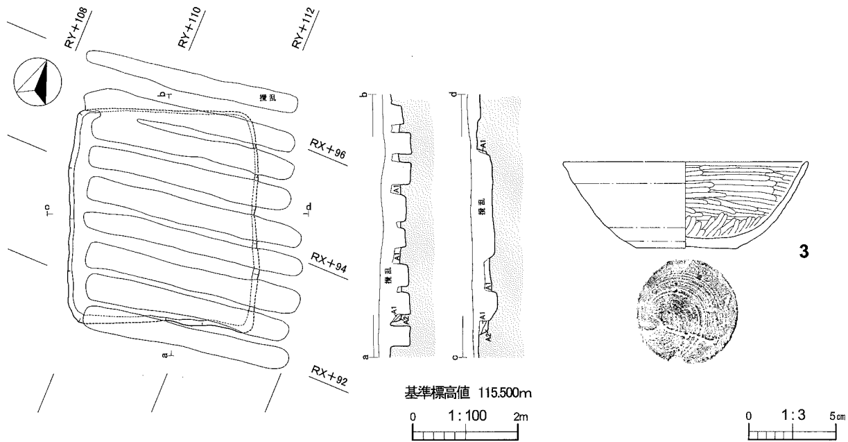
第5図 RE004 竖穴状遺構
