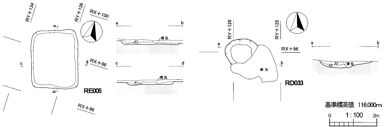
第6図 RE005 竪穴状遺構・RD033 土坑
