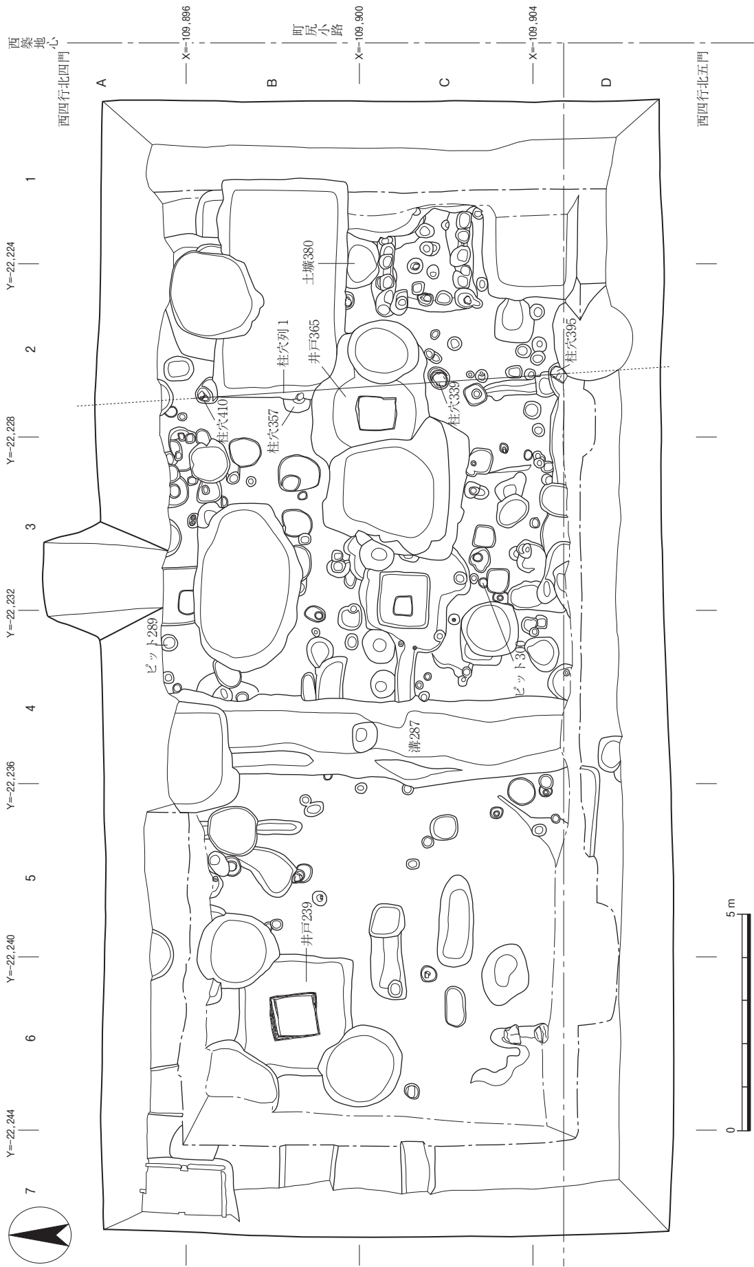
図19 第4面実測図 (1/120)
