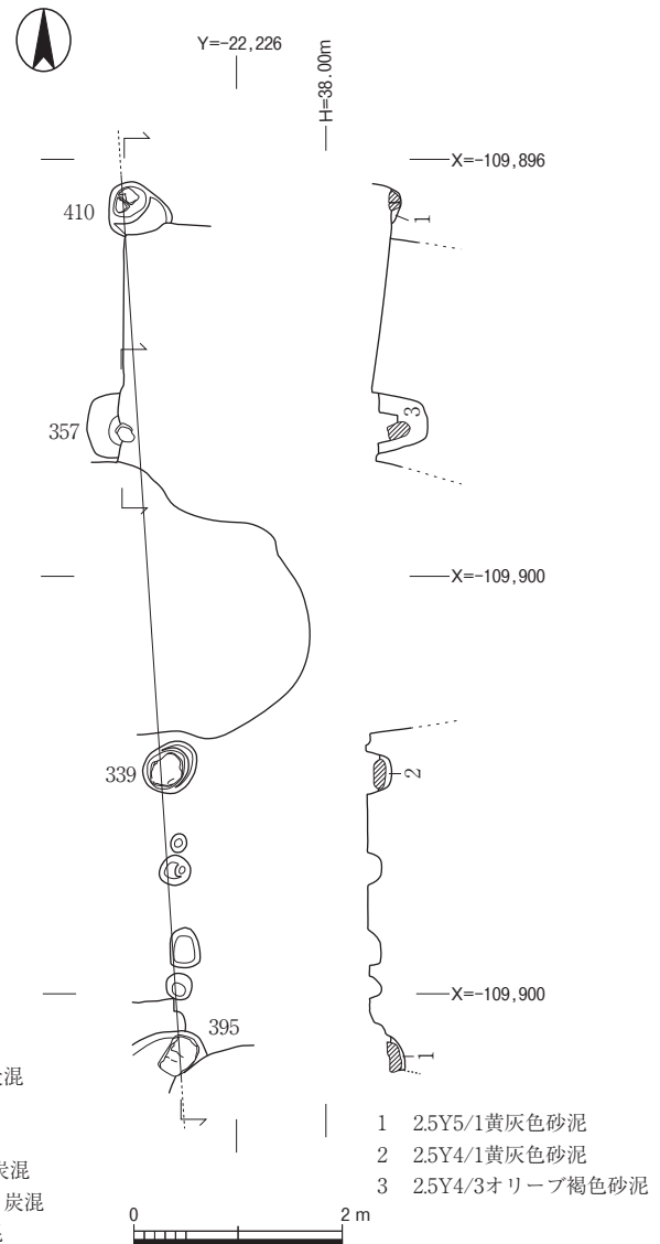
図22 柱穴列1実測図 (1/80)
