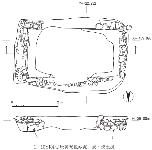
図8 石室9実測図 (1/80)
