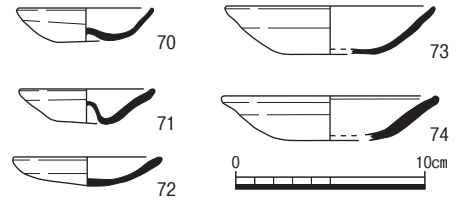
図30 石室135出土土器実測図 (1/4)
