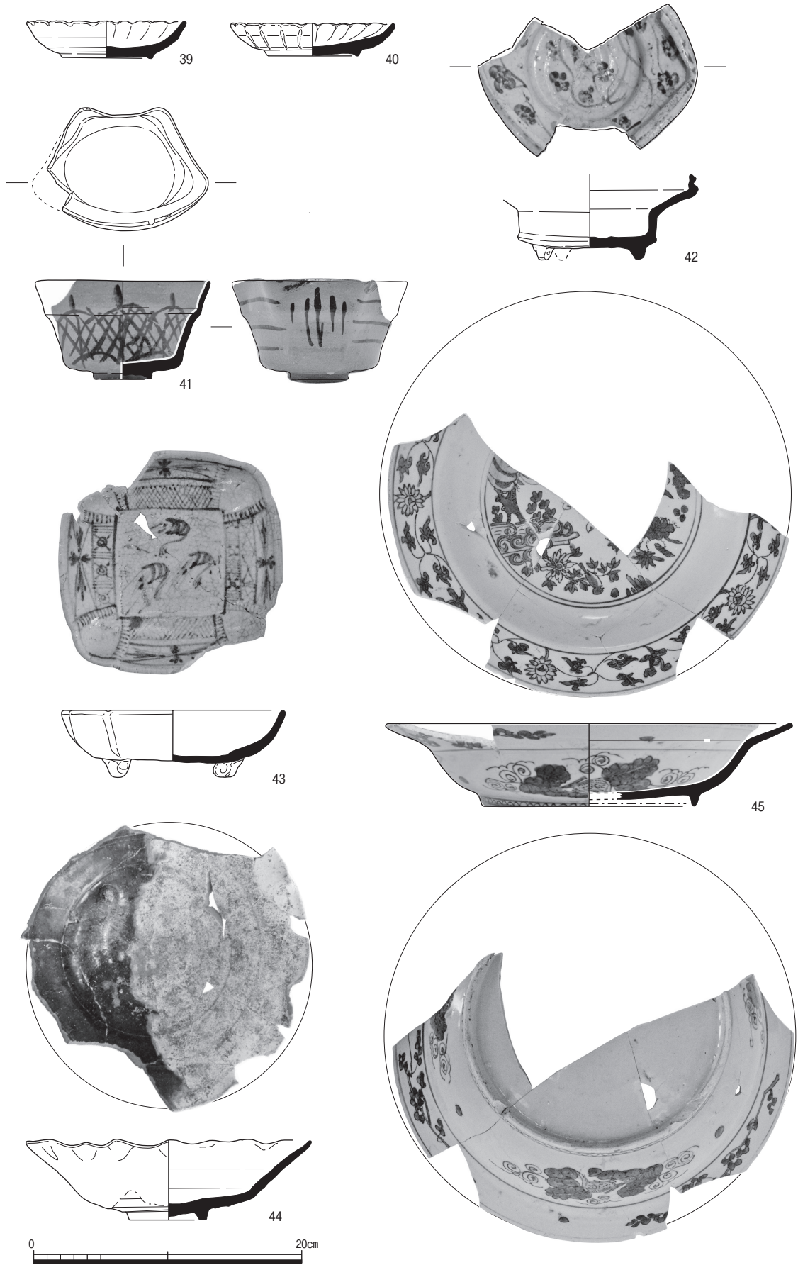
图27 土壙93·98出土土器实测图 (1/4)
