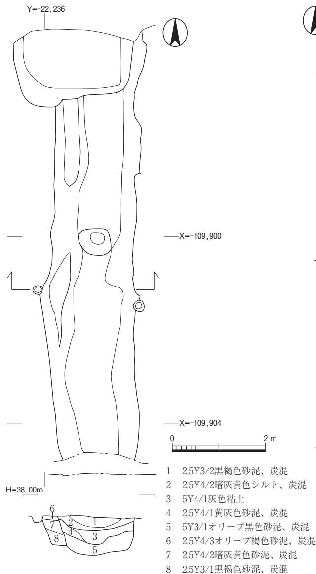
図21 溝287実測図 (1/80)
