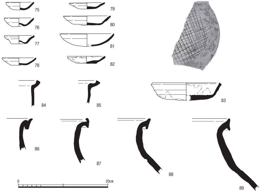
図31 地下室127出土土器実測図 (1/4)
