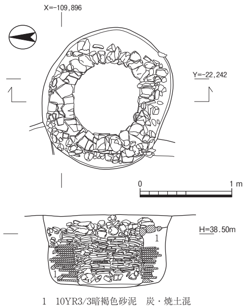
図9 瓦組99実測図 (1/40)
