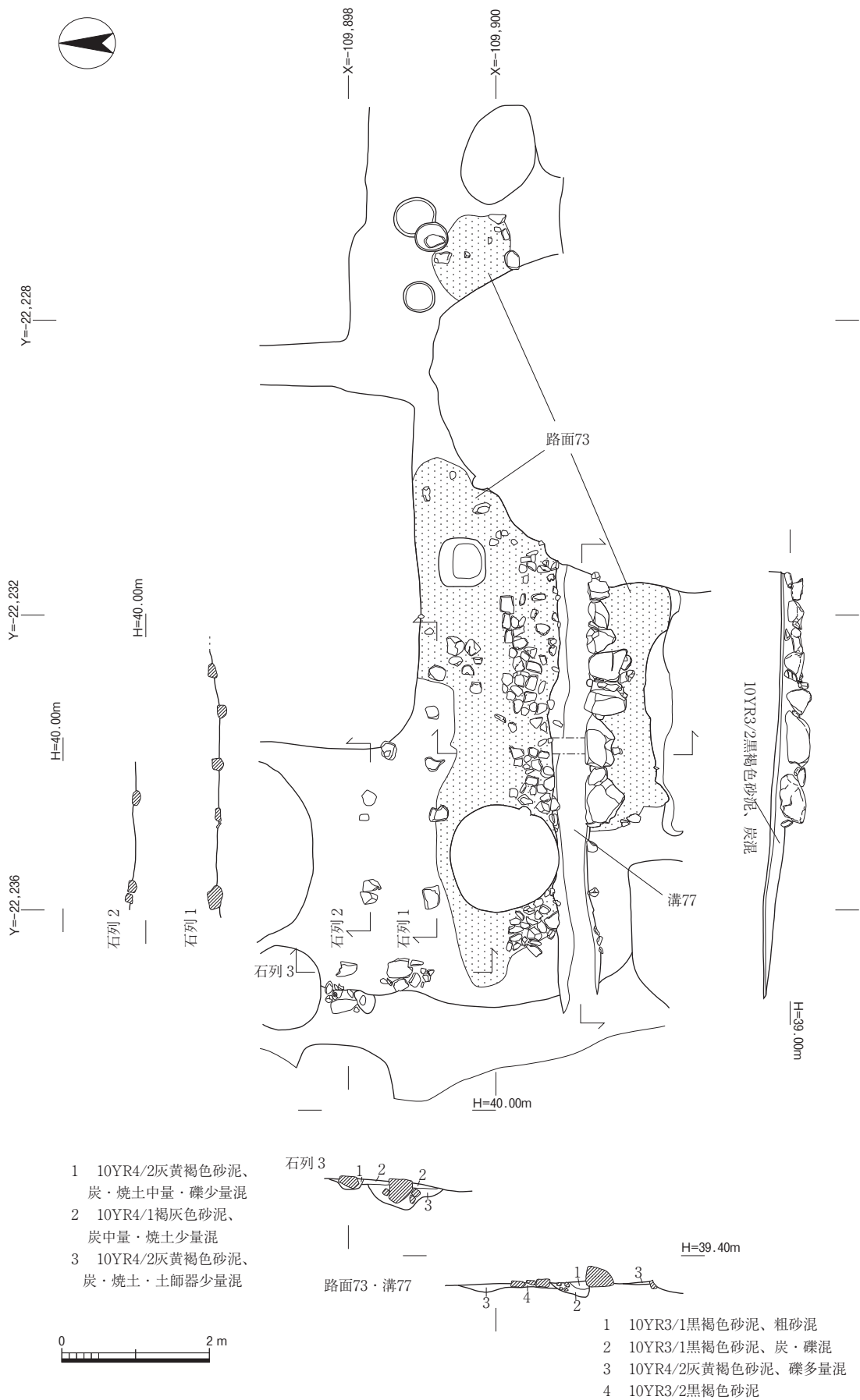
图10 石列1~3·路面73·溝77实测图 (1/80)
