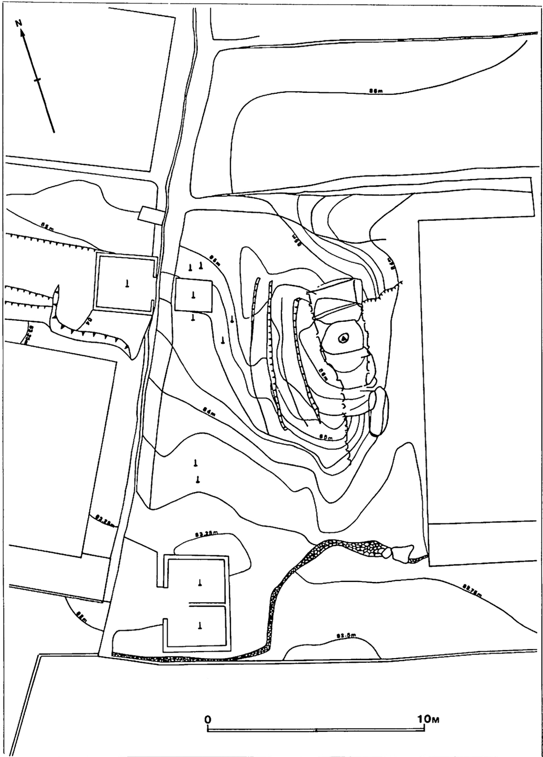
第2図 海原古墳墳丘実測図 (単位m, 海拔高を示す, conta25cm, ▲86.52m)
