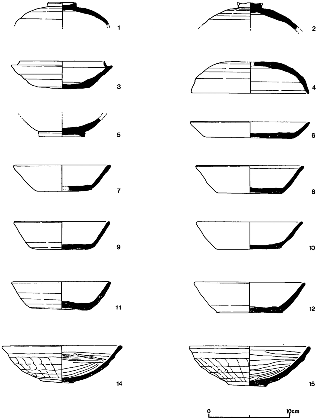
第6图 遗物实测图(2)
