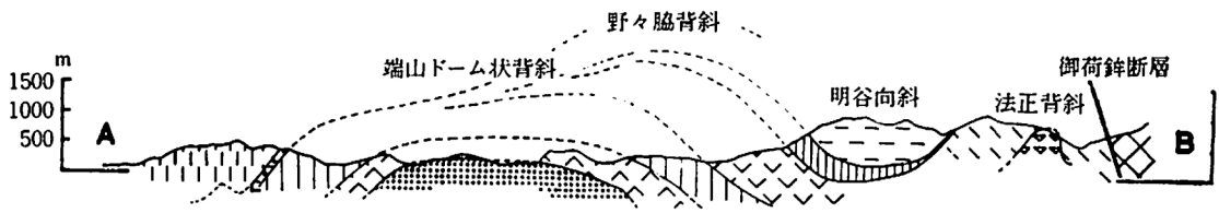
第8図 貞光川地域地質図(9)
