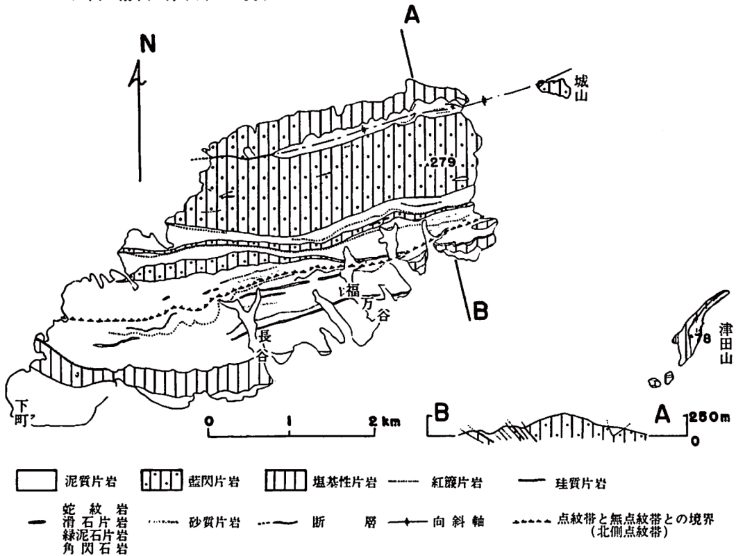
第3図 眉山・城山・津田山地質図(6)
