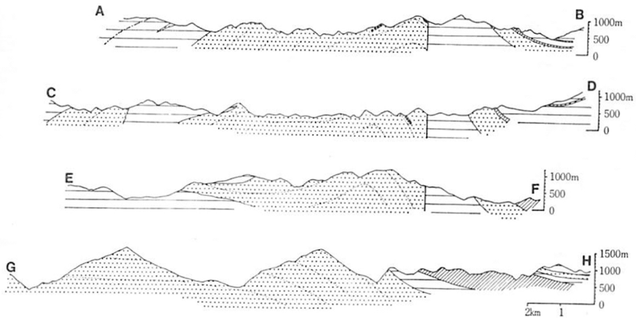
第6図 大歩危地域地質断面図(11)
