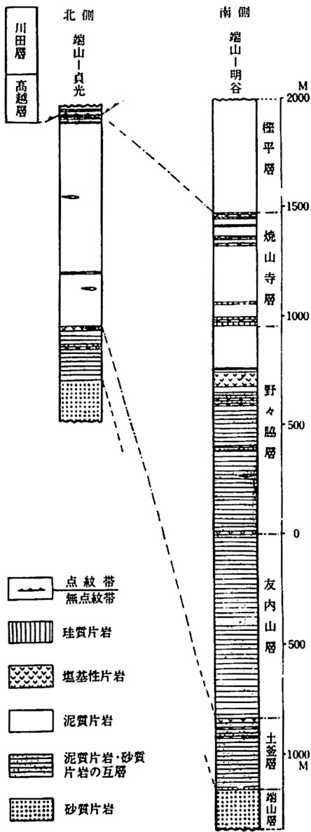
第9図 端山ドーム状背斜両側の結晶片岩柱状図
