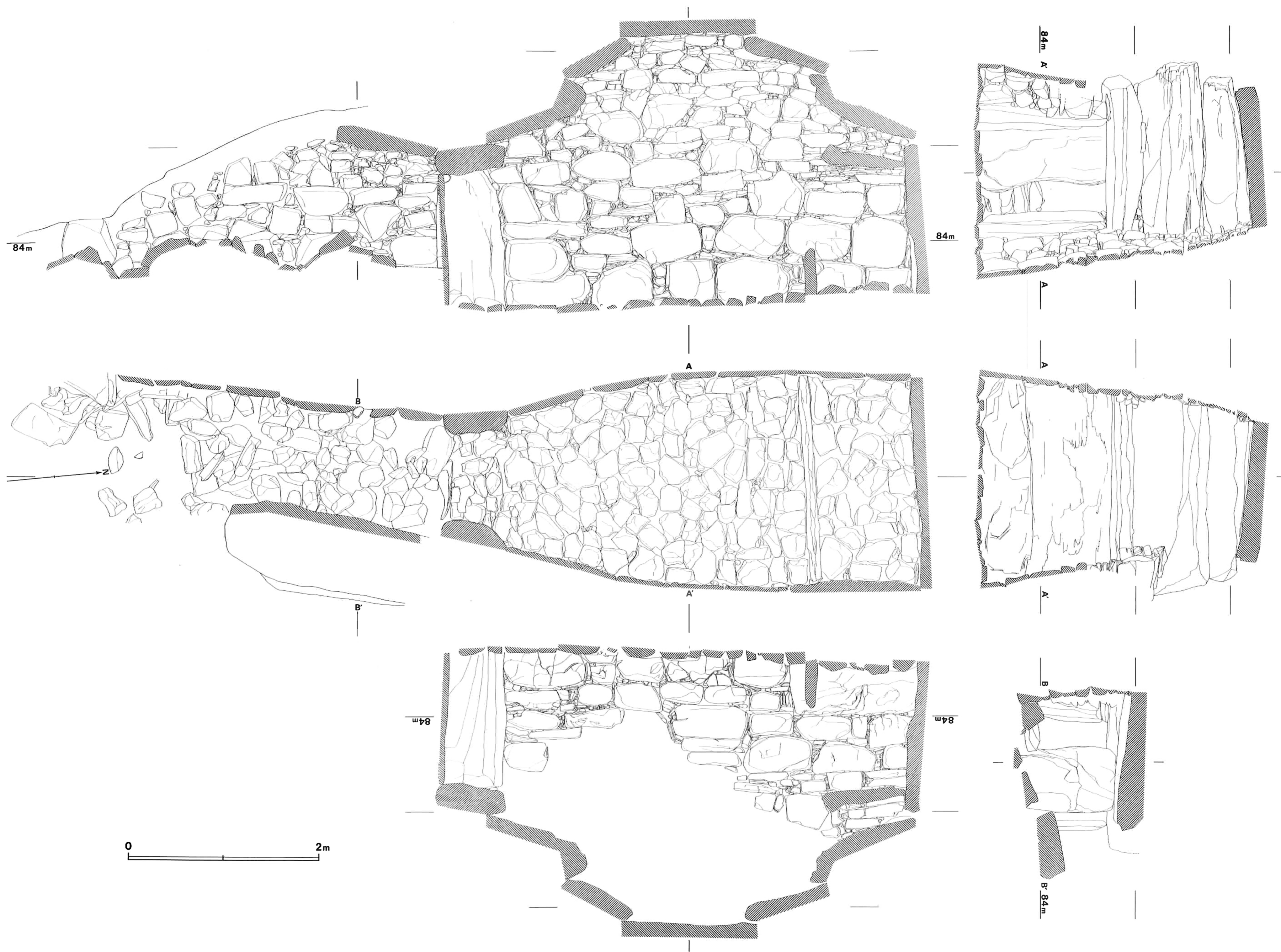
第3図 海原古墳横穴式石室実測図 (海拔高を示す)
