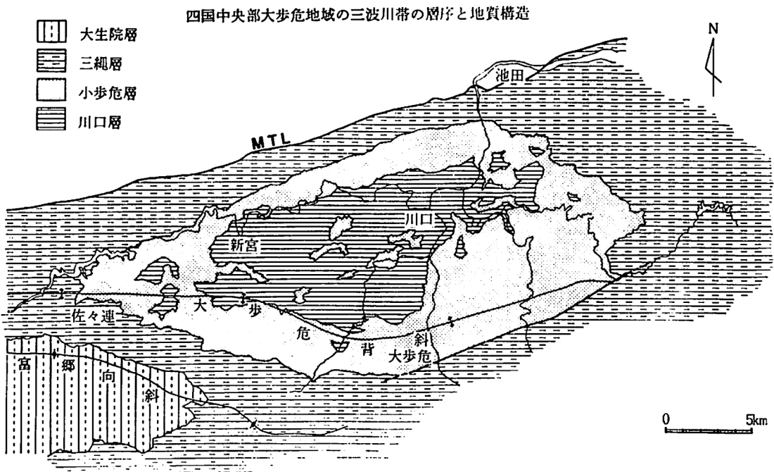
第7図 四国中央部三波川帯の地質図
