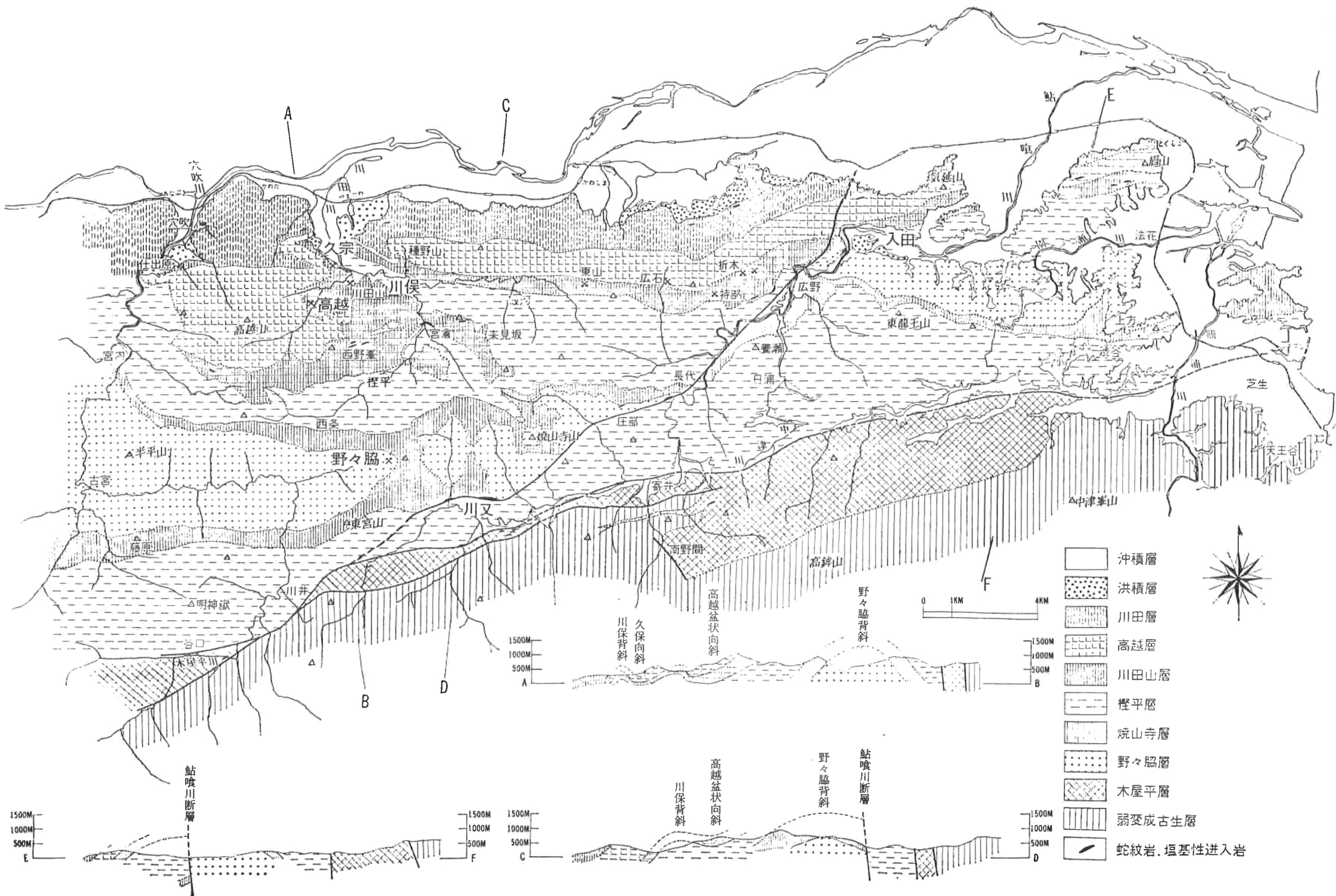
第4図 三波川帯東部地域地質図(3)
