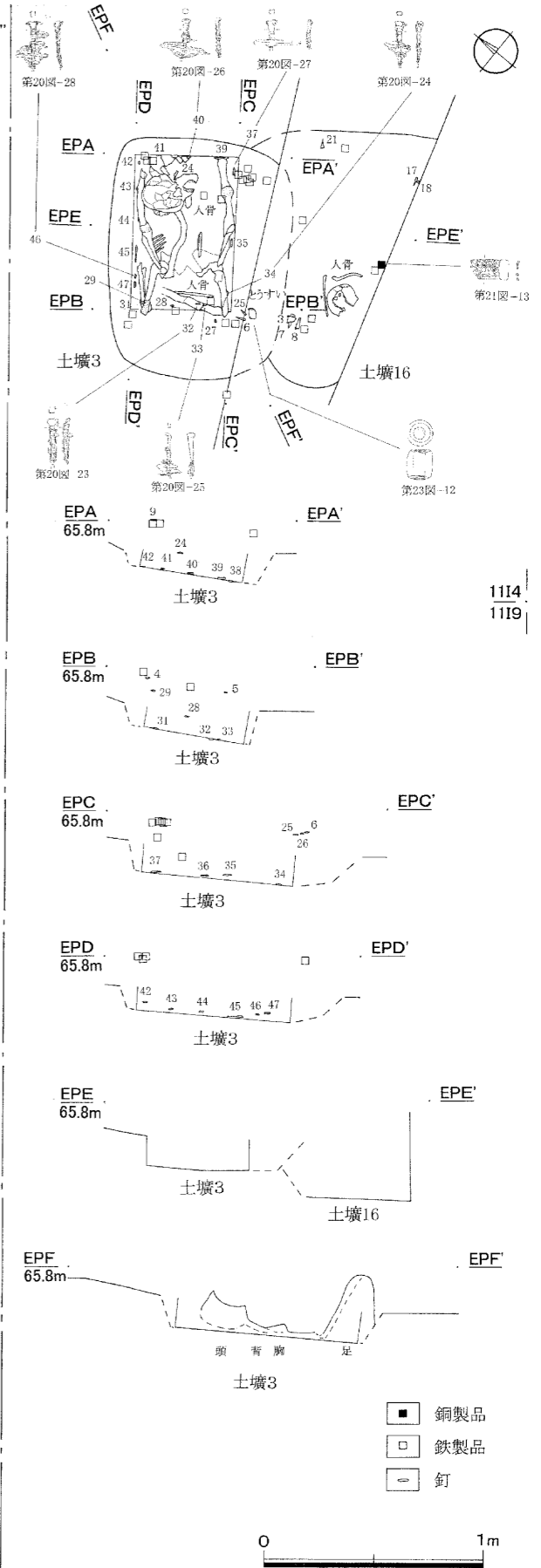
第8図 トレンチ3 土層3 遺構平面図他
