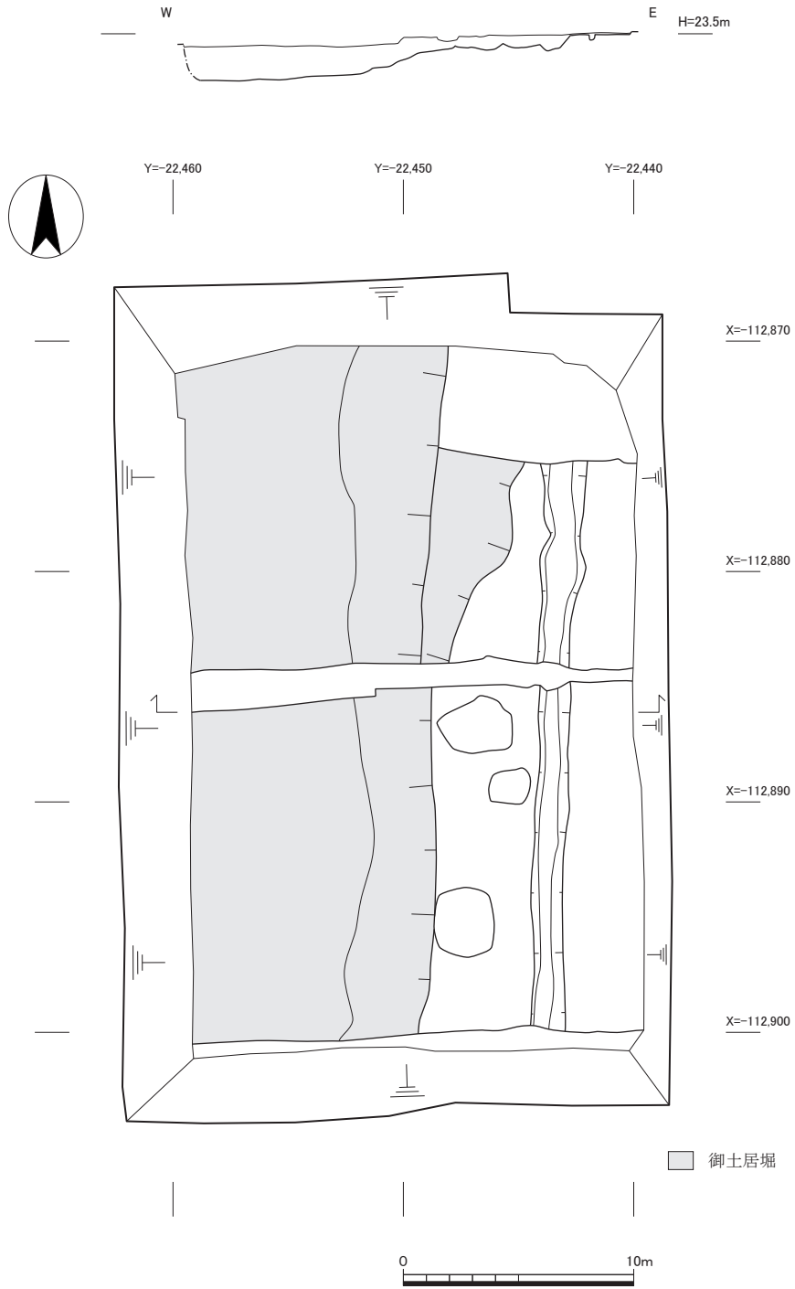
図5 調査3遺構実測図 (1:300)
