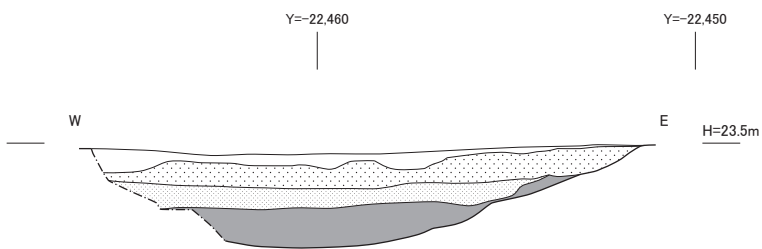
調査4 堀断面図
