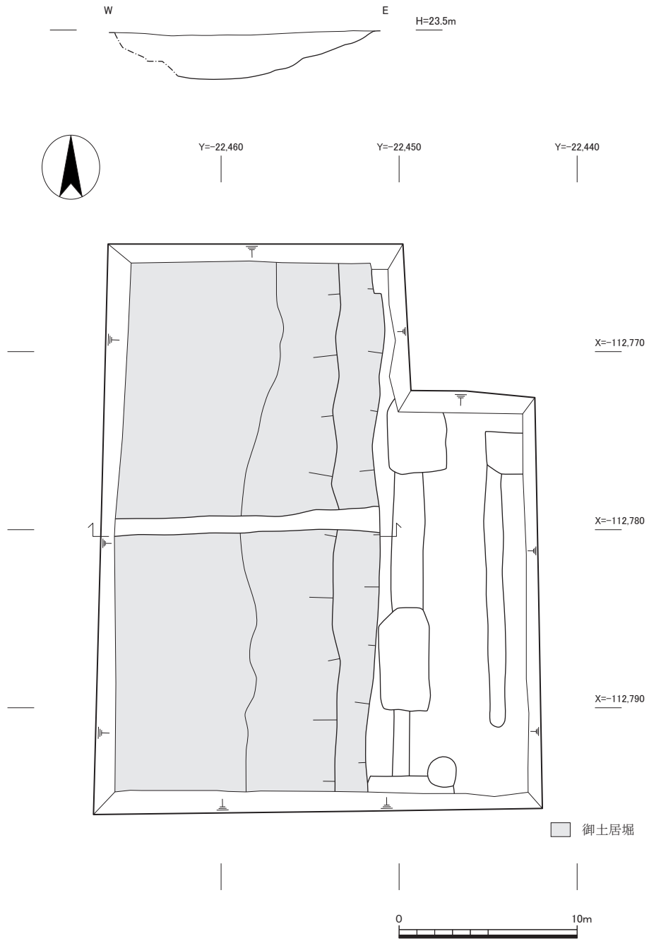
図6 調査4遺構実測図 (1:300)
