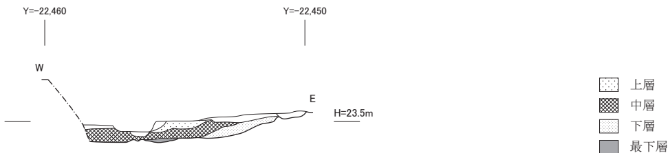
調査5 堀断面図
