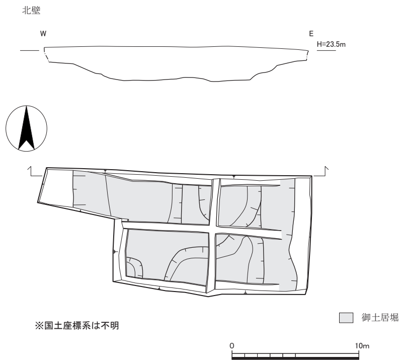
図3 調査1 遺構実測図 (1:300)
