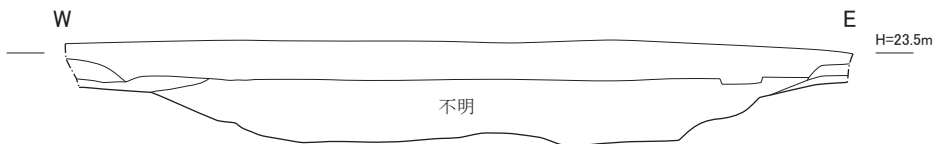
調査1 北壁堀断面図
