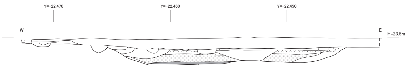
調査2 北壁堀断面図
