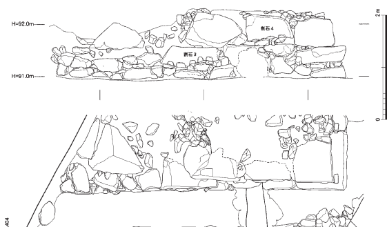
図 13 銀閣寺旧境内（京都市）石垣
