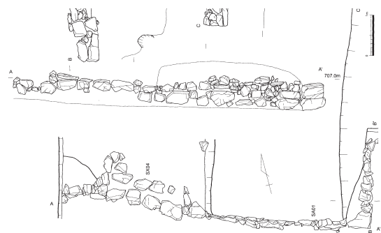
図 14 弥高寺跡（米原市）石垣
