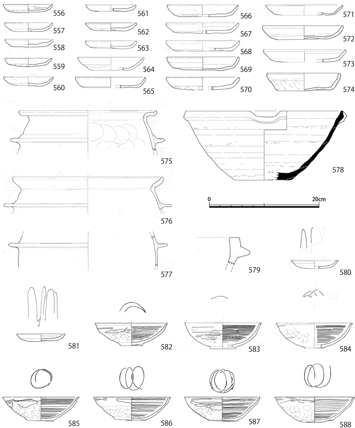
図 45 中層遺構 SD146 上層出土 土器 (S = 1/4)
