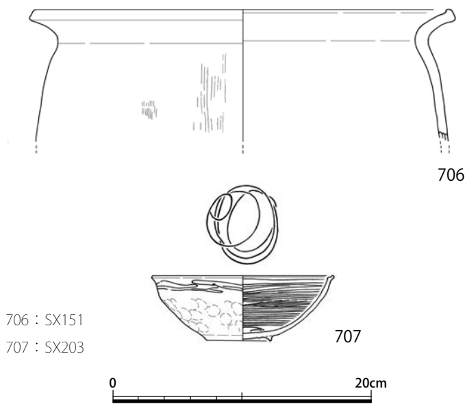
図 58 中層遺構 SX151・SX203 出土 土器 (S = 1/4)
