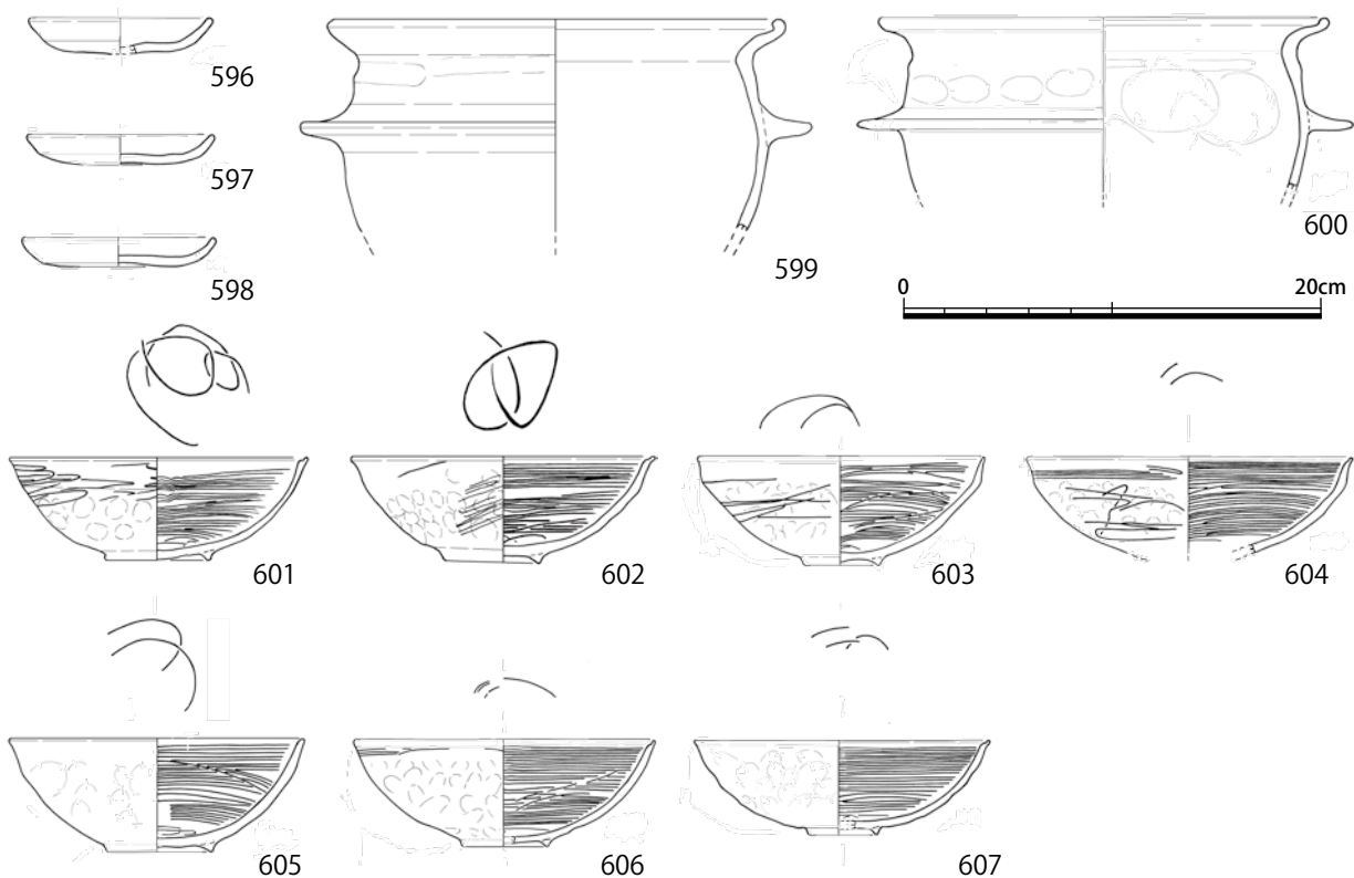
図 47 中層遺構 SD147 出土 土器 (S = 1/4)
