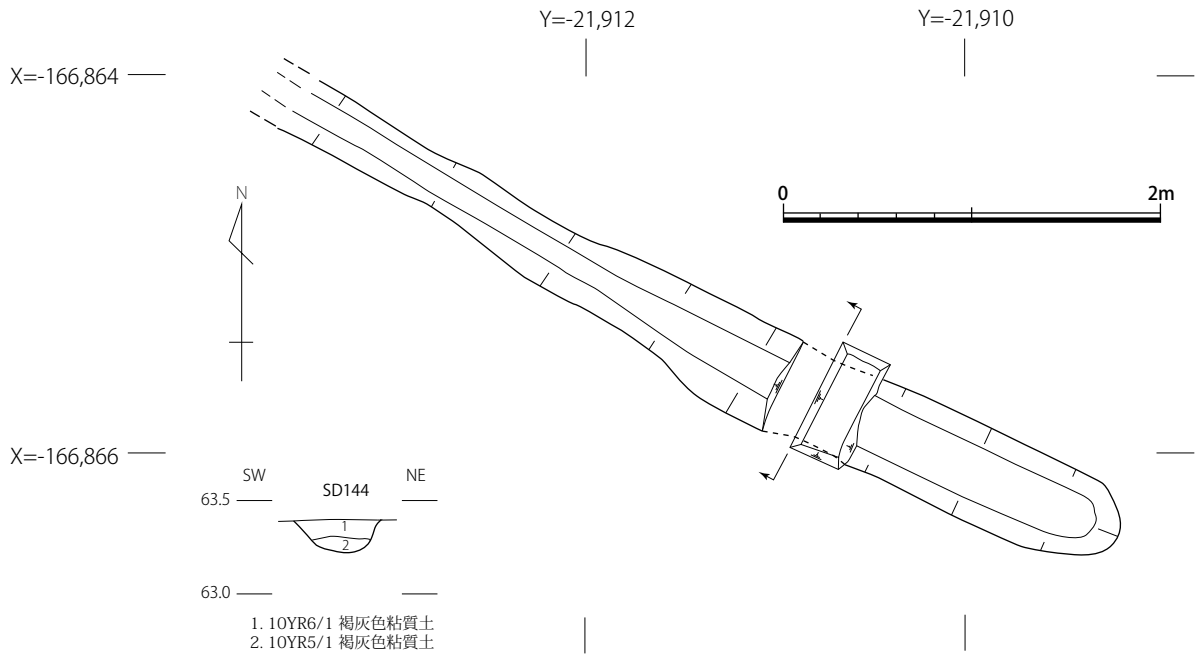
図 15 SD144 東半部平面・断面図 (S = 1/40)
