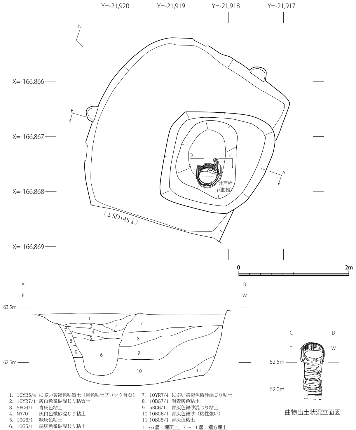
図 17 SE149 平面・断面図 (S = 1/40)
