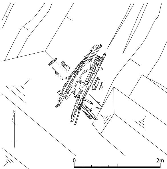
图 11 河道内 木組み遺構出土状況図 (S = 1/50)
