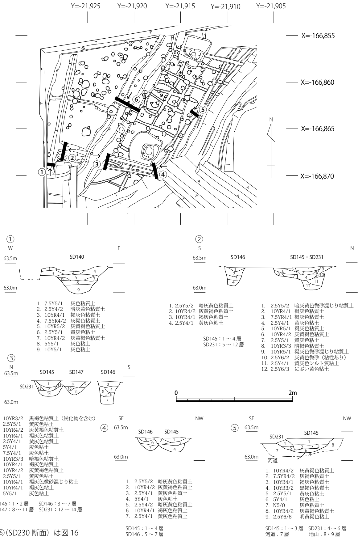
図14 区画溝土層断面図 (S = 1/40)
