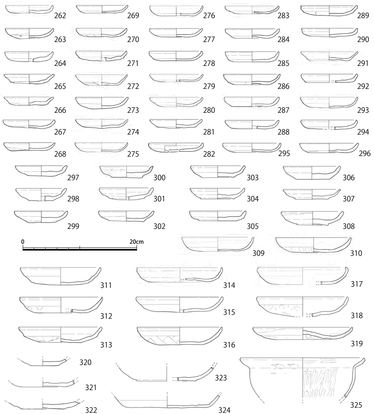
図34 中層遺構 河道3層出土 土器① (S = 1/4)
