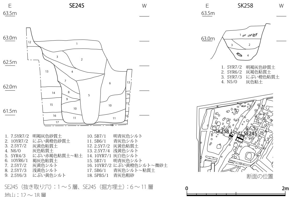
図 24 下層遺構土層断面図 (S = 1/40)
