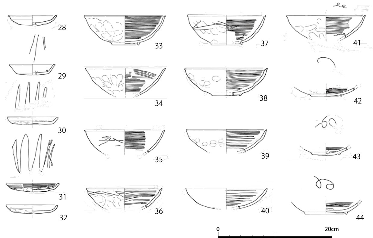
图 25 上層遺構 耕作溝群出土 土器 (S = 1/4)
