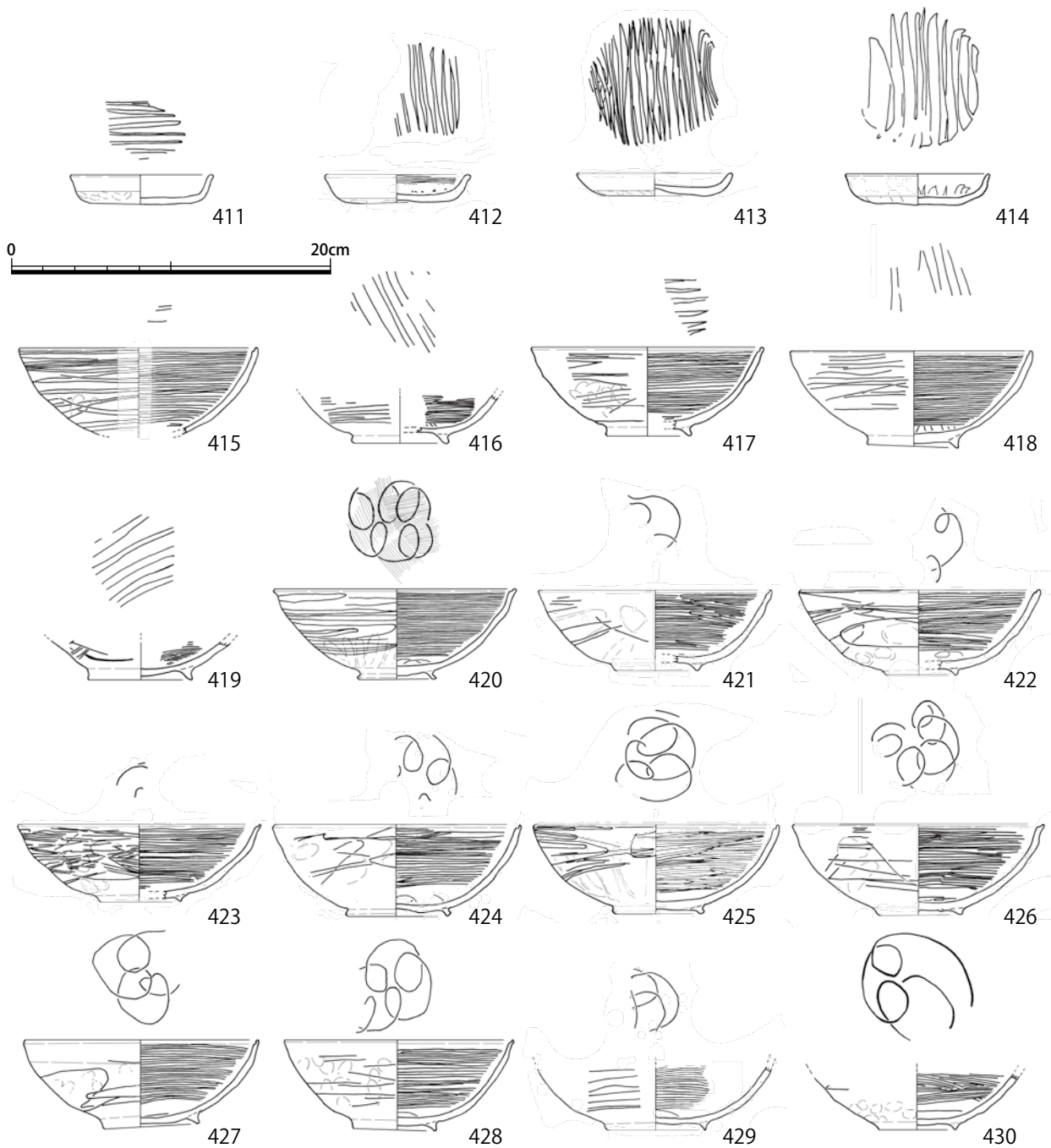
図38 中層遺構 河道4層出土 土器② (S = 1/4)
