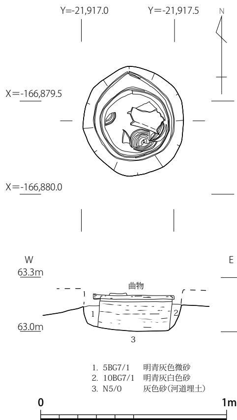
図7 SE131 平面・立面図 (S = 1/20)
