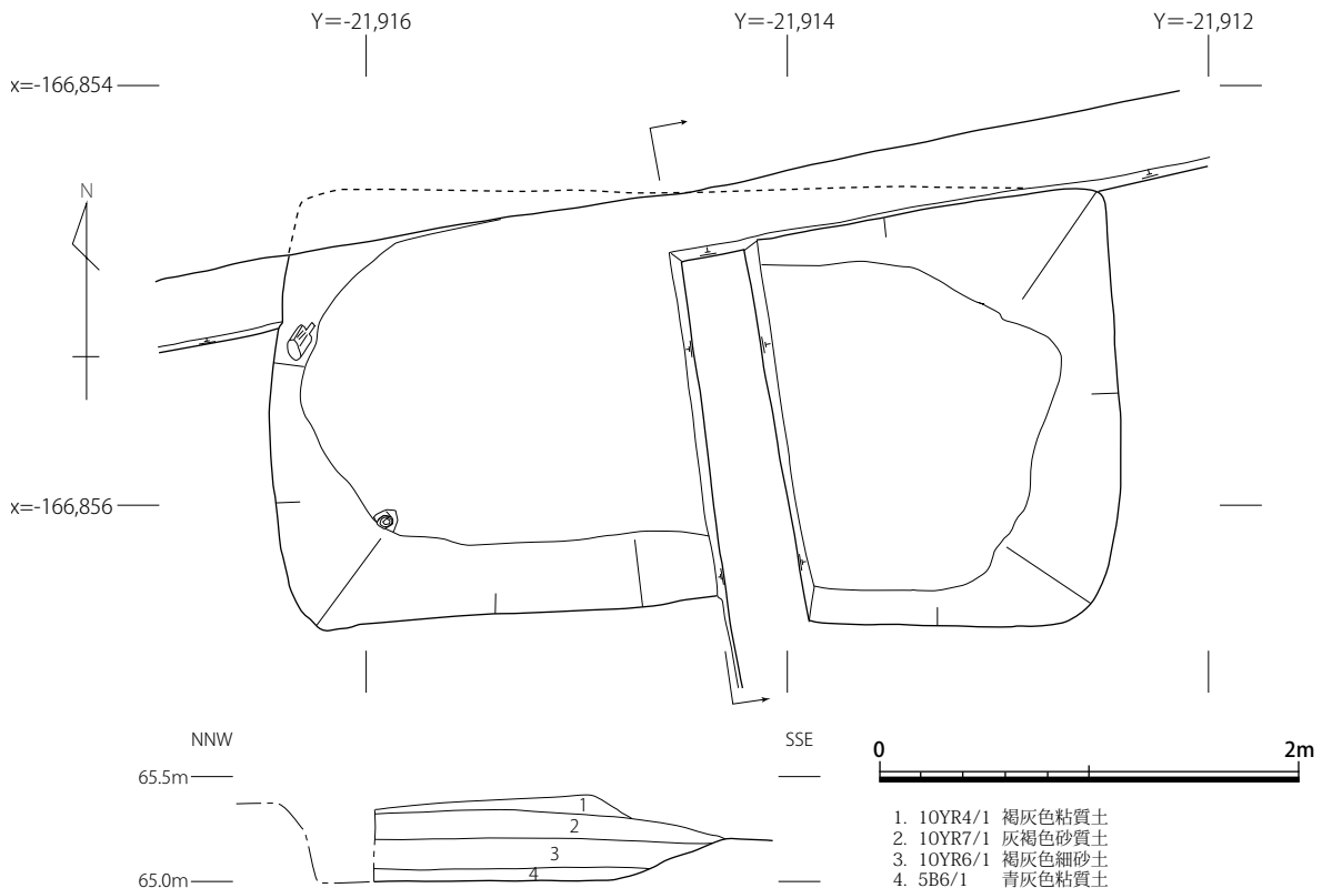
図 20 SX148 平面・断面図 (S = 1/40)
