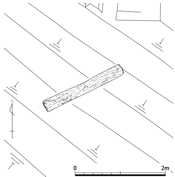
图 12 河道内 木桶出土状況図 (S = 1/50)
