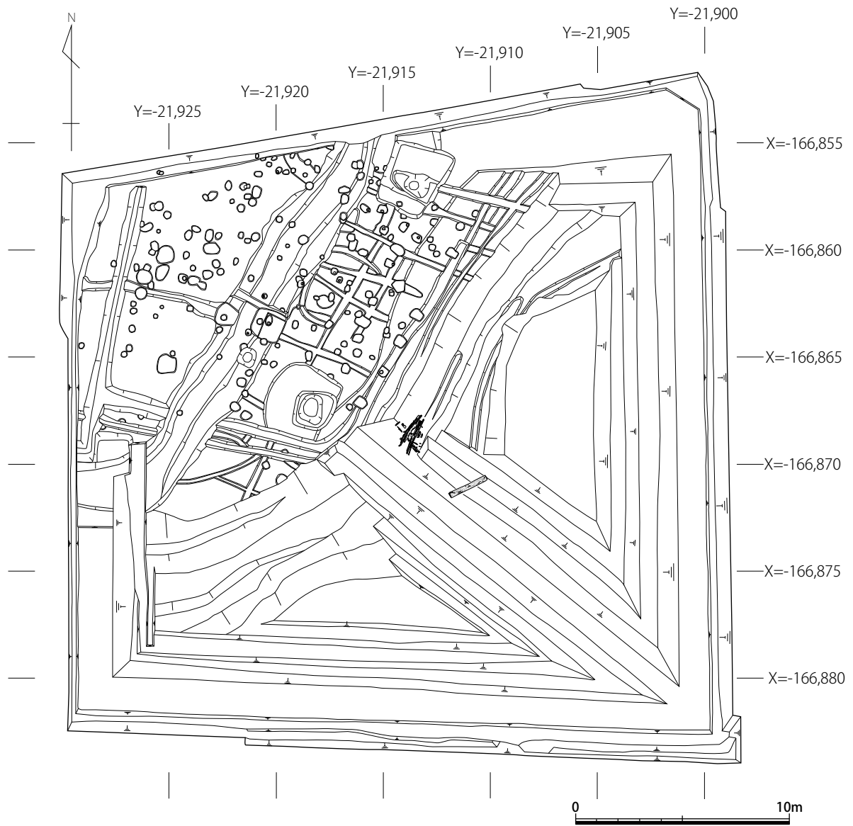
图 10 中層・下層完掘状況図 (S = 1/250)
