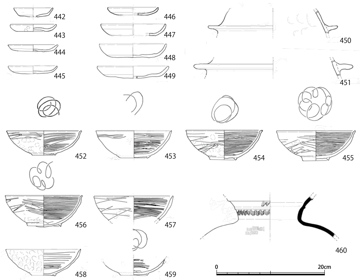
図 40 中層遺構 SD140 上層出土 土器 (S = 1/4)
