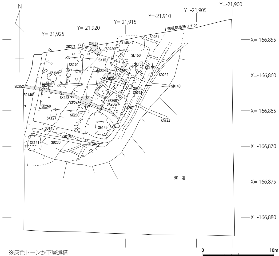
図8 中層・下層遺構配置図 (S = 1/250)
