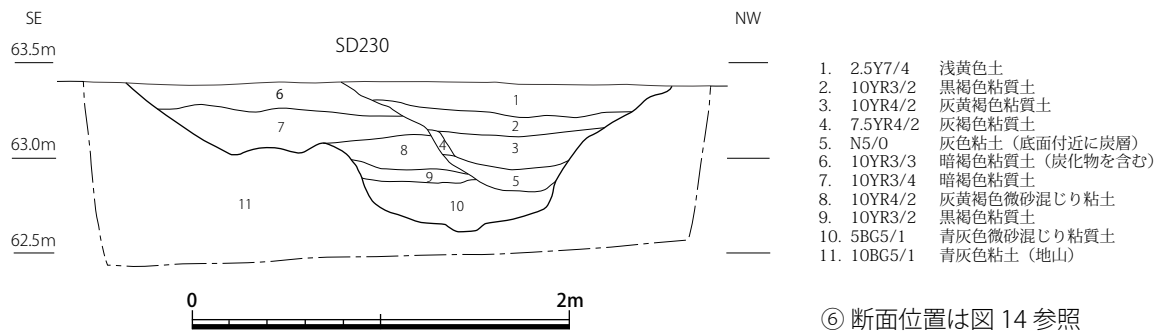
図 16 SD230 断面図 (S = 1/40)
