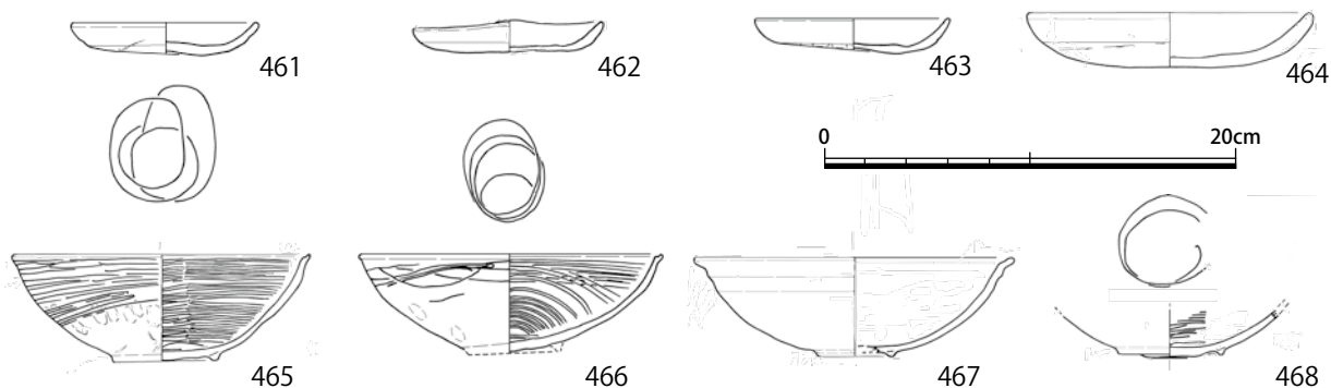
図 41 中層遺構 SD140 下層出土 土器 (S = 1/4)
