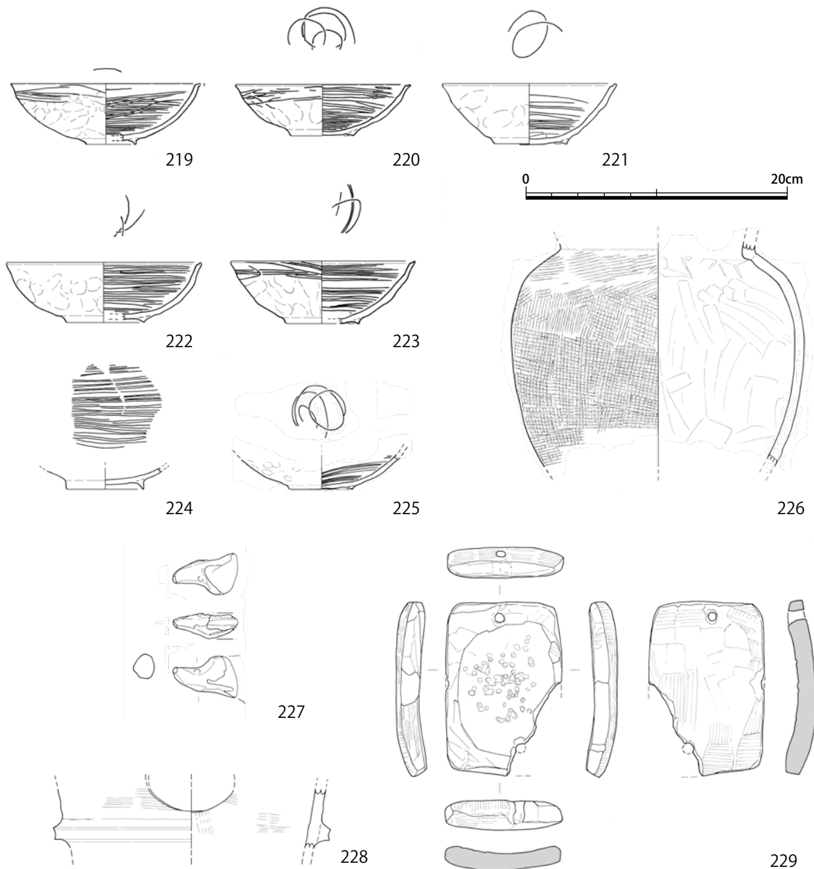
図 31 中層遺構 河道 1 層出土 土器⑤・土製品・石製品 (S = 1/4)
