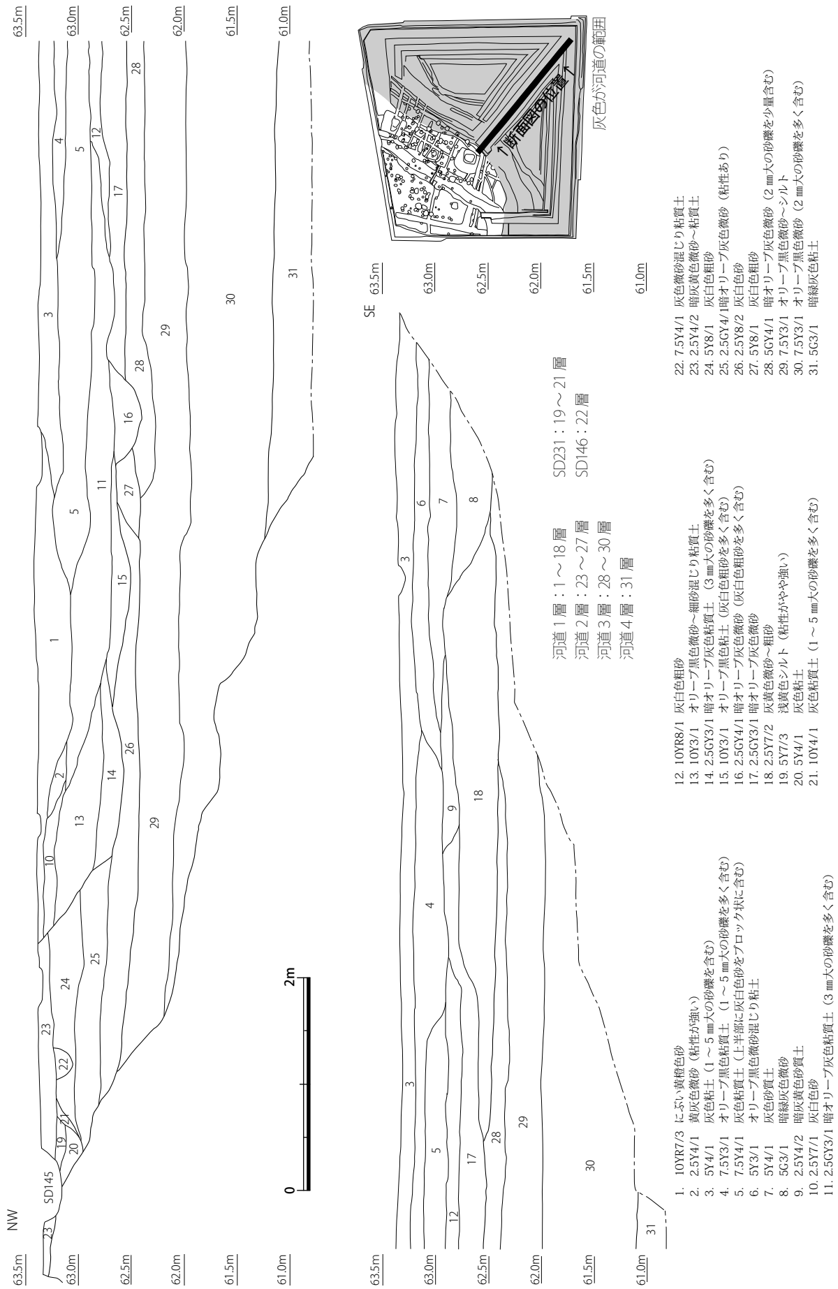
図 13 河道土層断面図 (S = 1/150)
