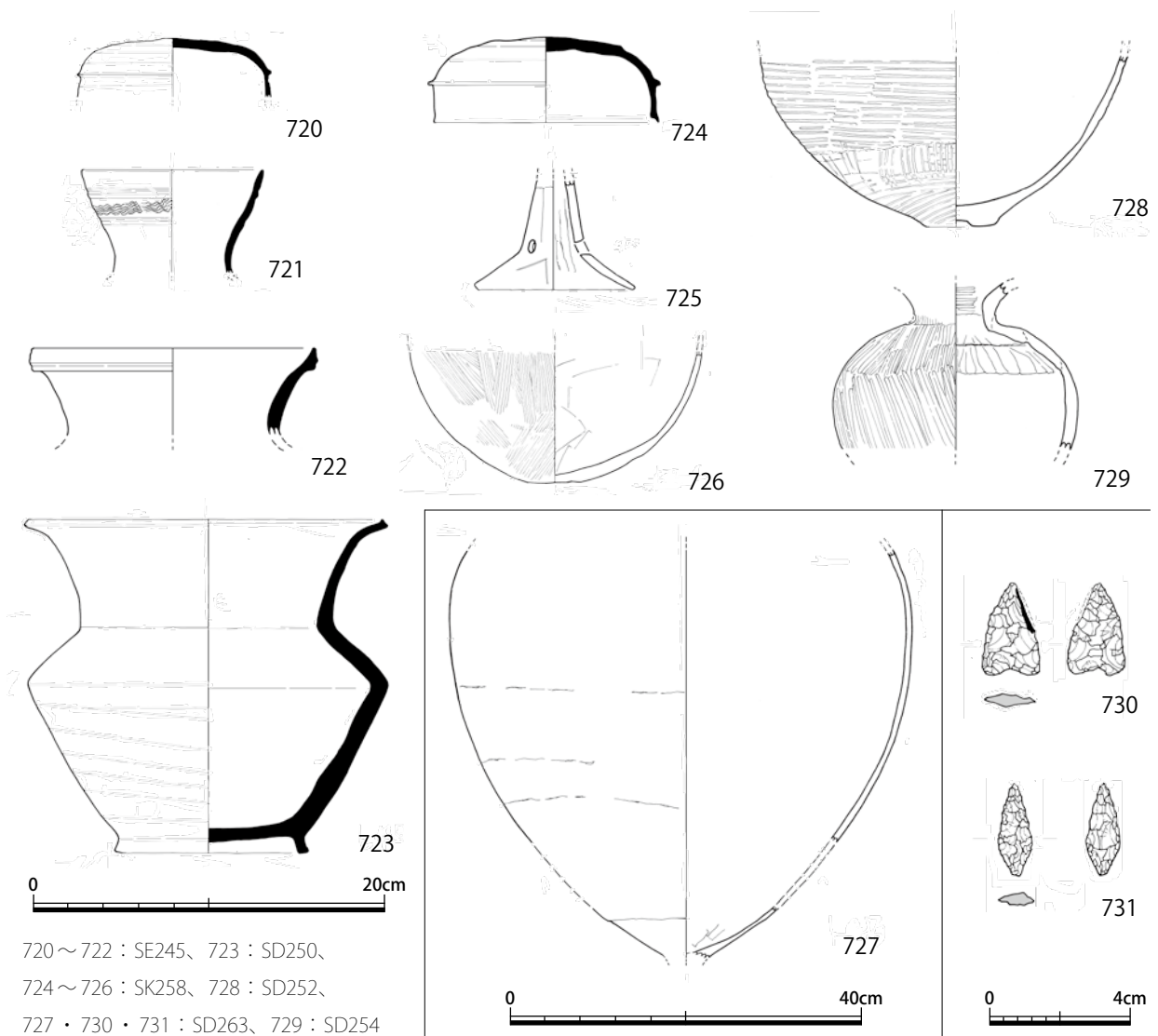
図60 下層遺構出土 土器・石器 (S = 1/4・1/8・1/2)
