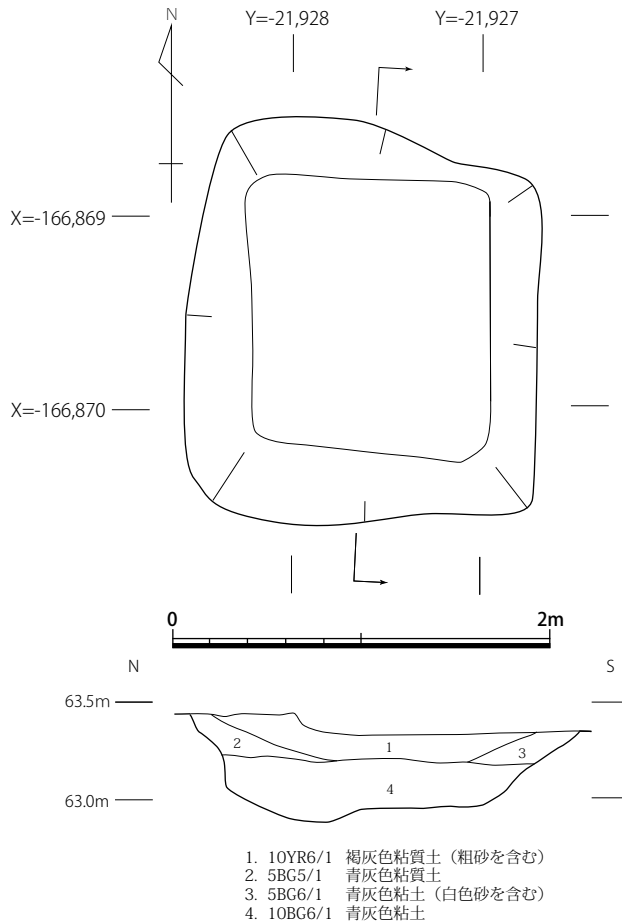
図 19 SX141 平面・断面図 (S = 1/40)
