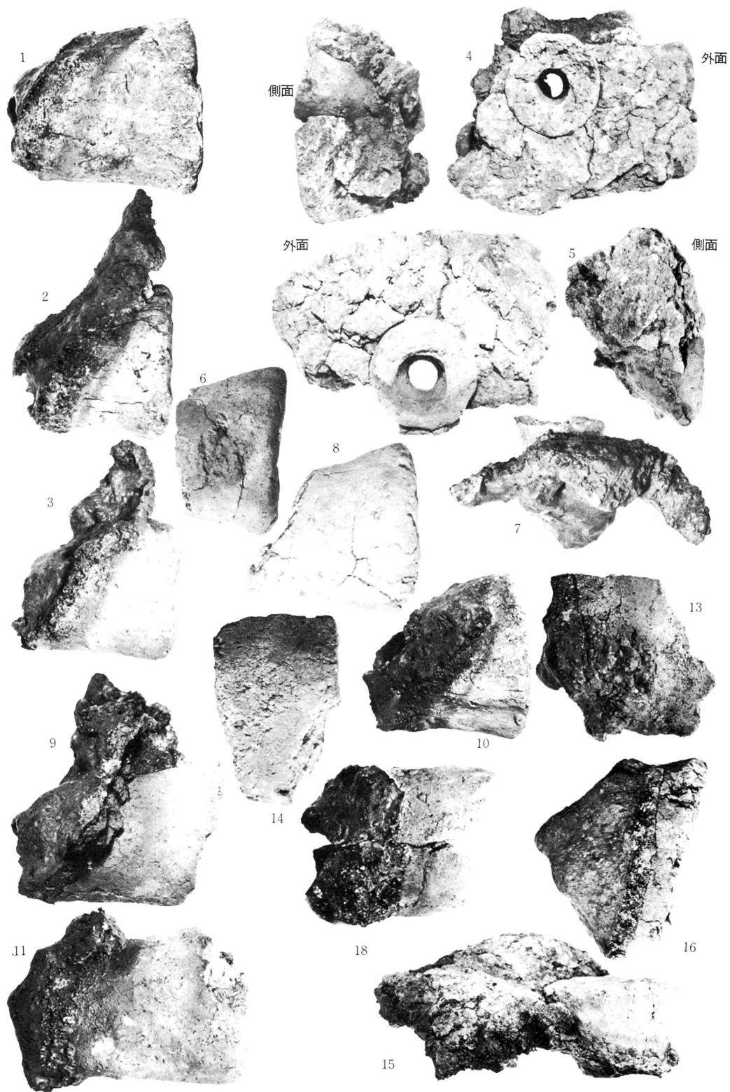
M区西側出土鞆羽口 (番号は計測表・第15図と同じ) 図版 9
