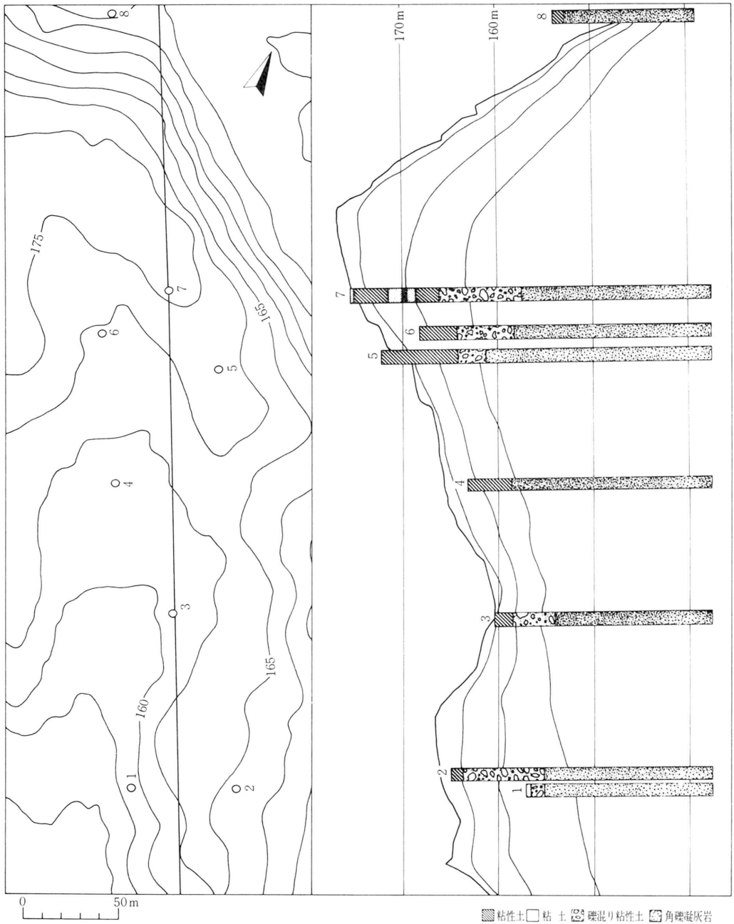
第2図 地形及び地質推定断面図
