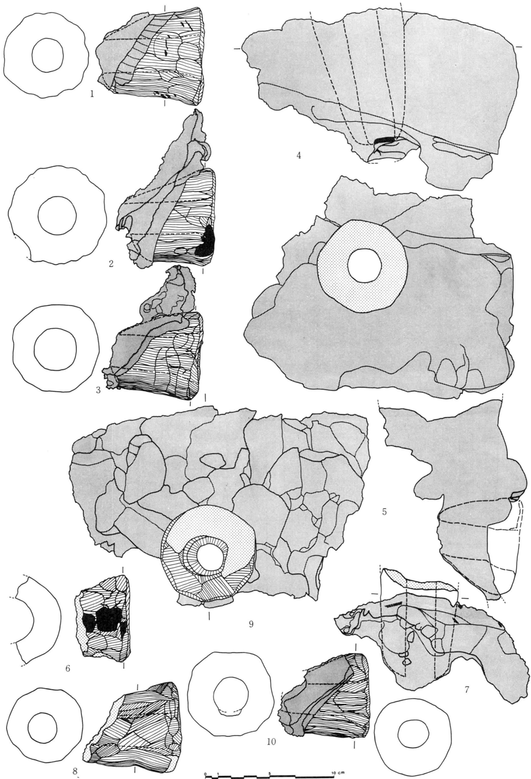
第15图 M地区西侧窯壁・鞆羽口集積地出土品 I
