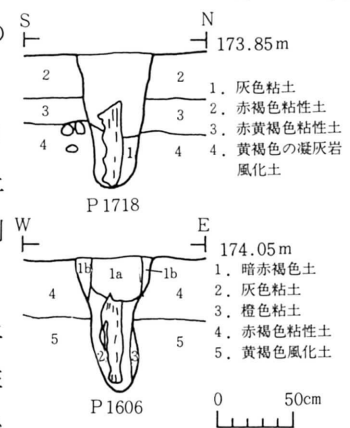
第13図 一の郭柱穴断面図
