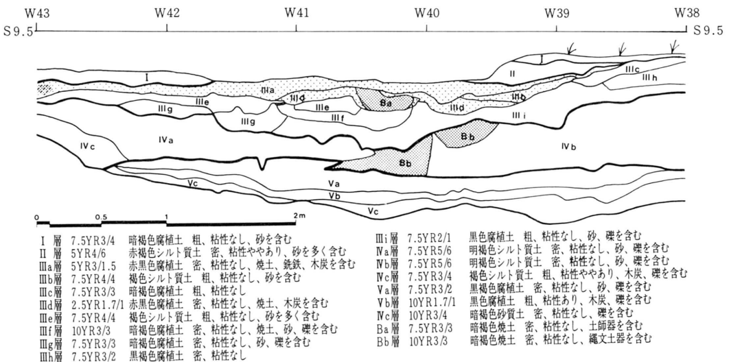
第2図 Md42地区基本層序
