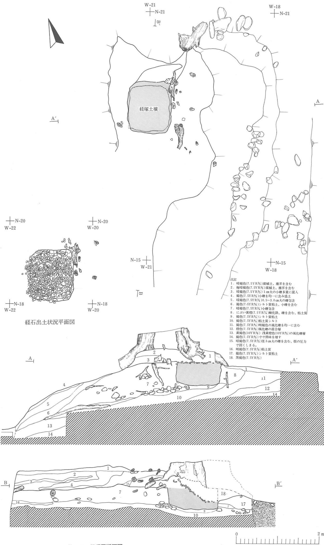
第69図 経塚断面図
