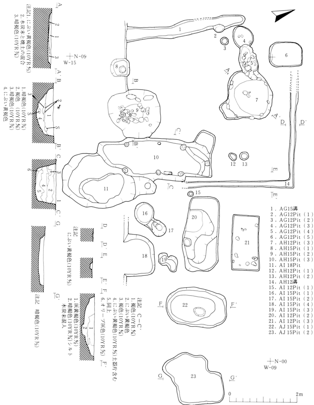
第82図 A区ピット群平面図
