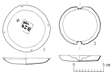
第65図 御飯屋堀跡出土天秤皿
