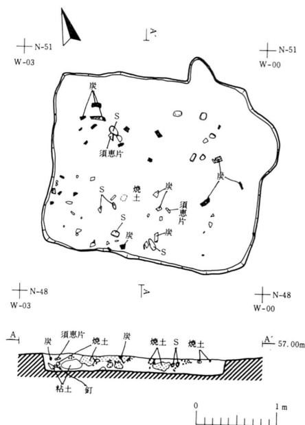
第78図 X C 09掘込み土壌平面断面図
