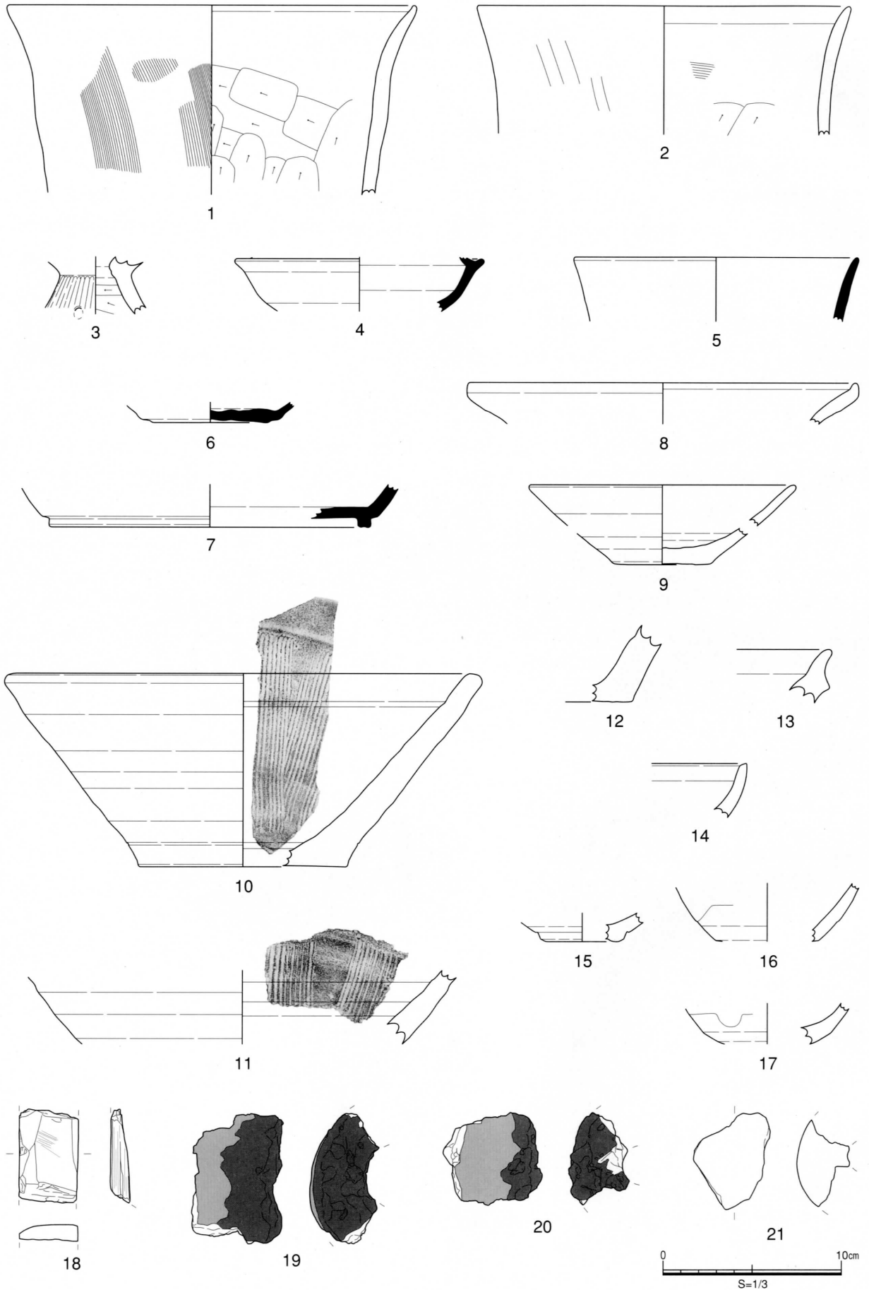
第6图 遺物実測図1
