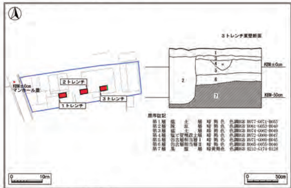
第3図 トレンチ配置と 3トレンチ東壁断面図 (1,200・1/60)
