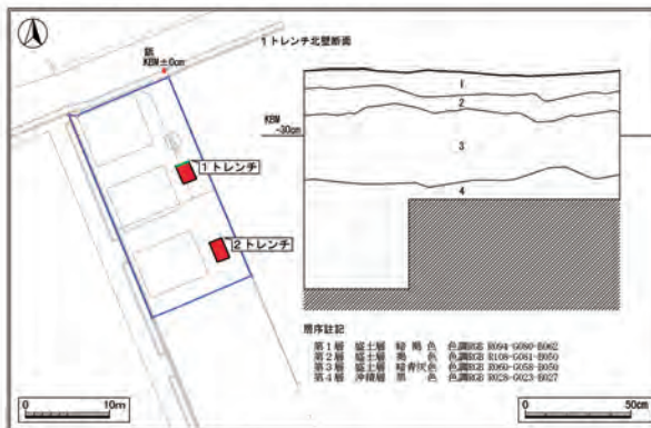
第3図 トレンチ配置と 1トレンチ北壁断面図(1/1,000・1/40)
