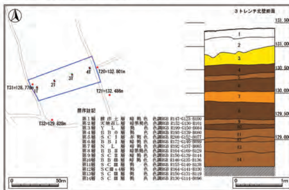
第3図 トレンチ配置と3トレンチ北壁断面図 (1/4,000・1/80)
