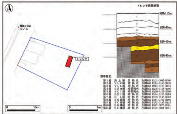
第3図 トレンチ配置とトレンチ西壁断面図(1/800・1/80)
