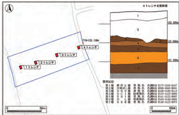
第3図 トレンチ配置と4トレンチ北壁断面図(1/2,000・1/60)
