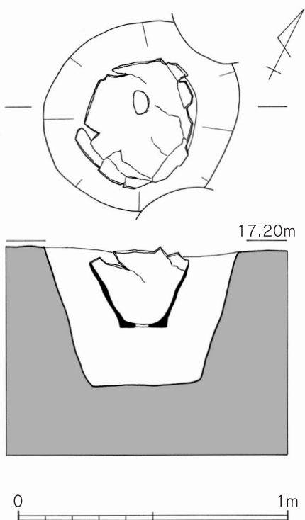
第5図 埋甕遺構実測図(縮尺1/20)
