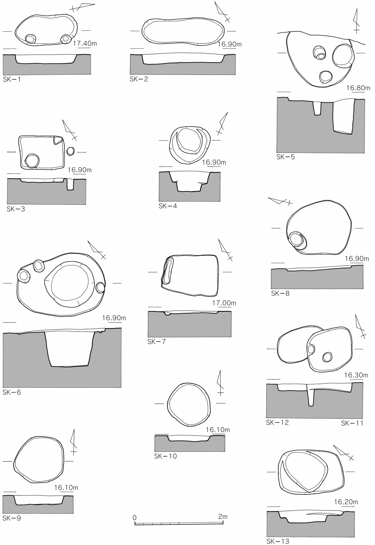
第21図 その他の遺構実測図・1(縮尺1/50)
