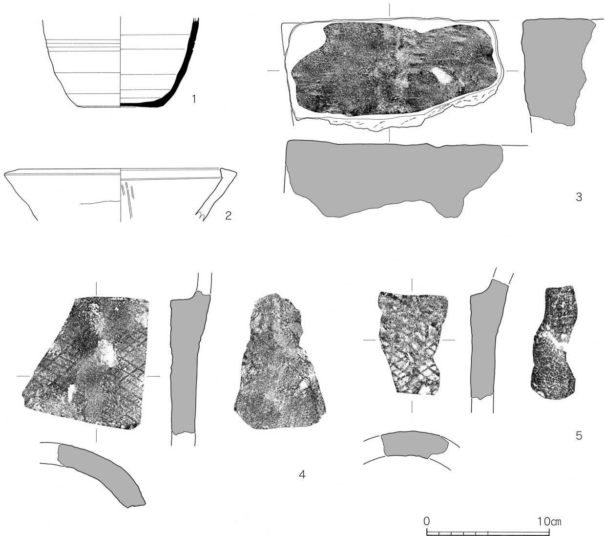
第20図 石組遺構出土遺物実測図(縮尺1/3)
