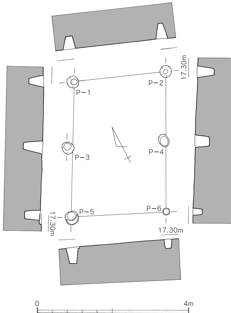
第15図 4号掘立柱建物跡実測図(縮尺1/60)
