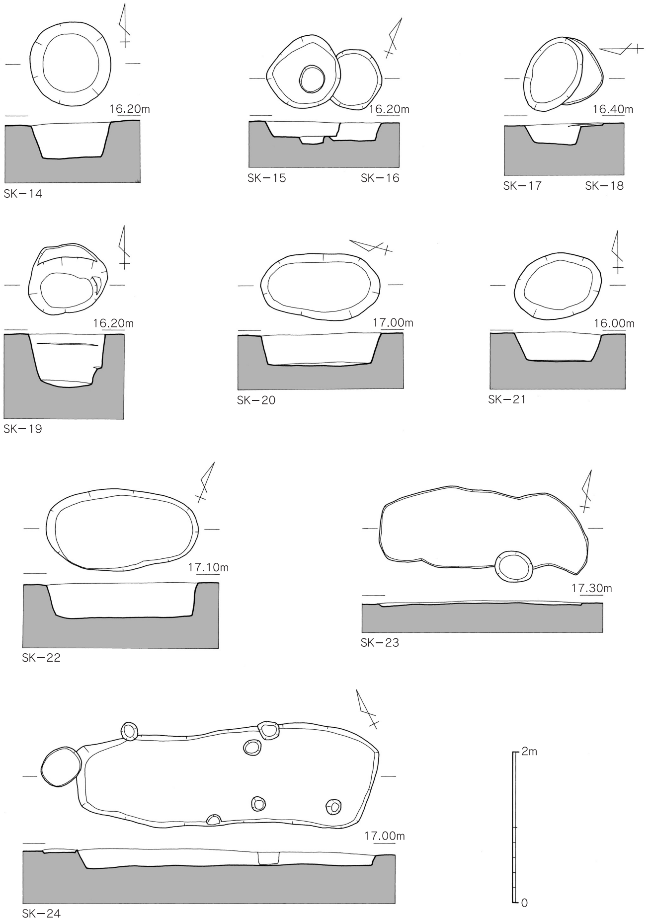
第22図 その他の遺構実測図・2(縮尺1/50)
