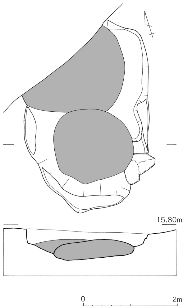
第19図 円形石組遺構実測図(縮尺1/50)
