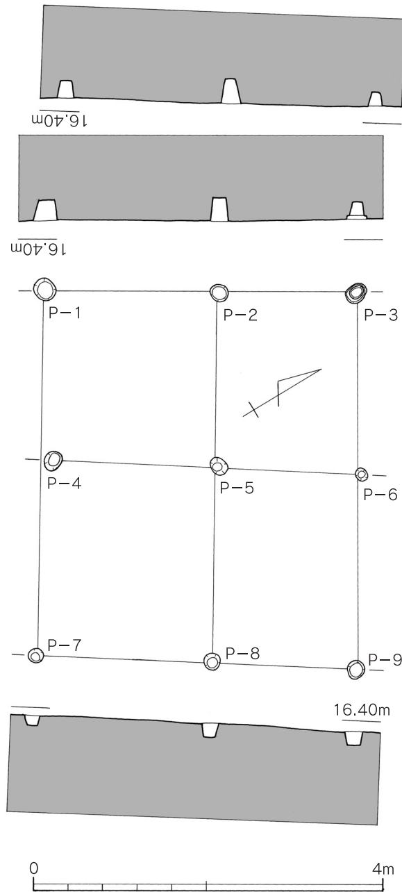
第16図 5号掘立柱建物跡実測図(縮尺1/60)
