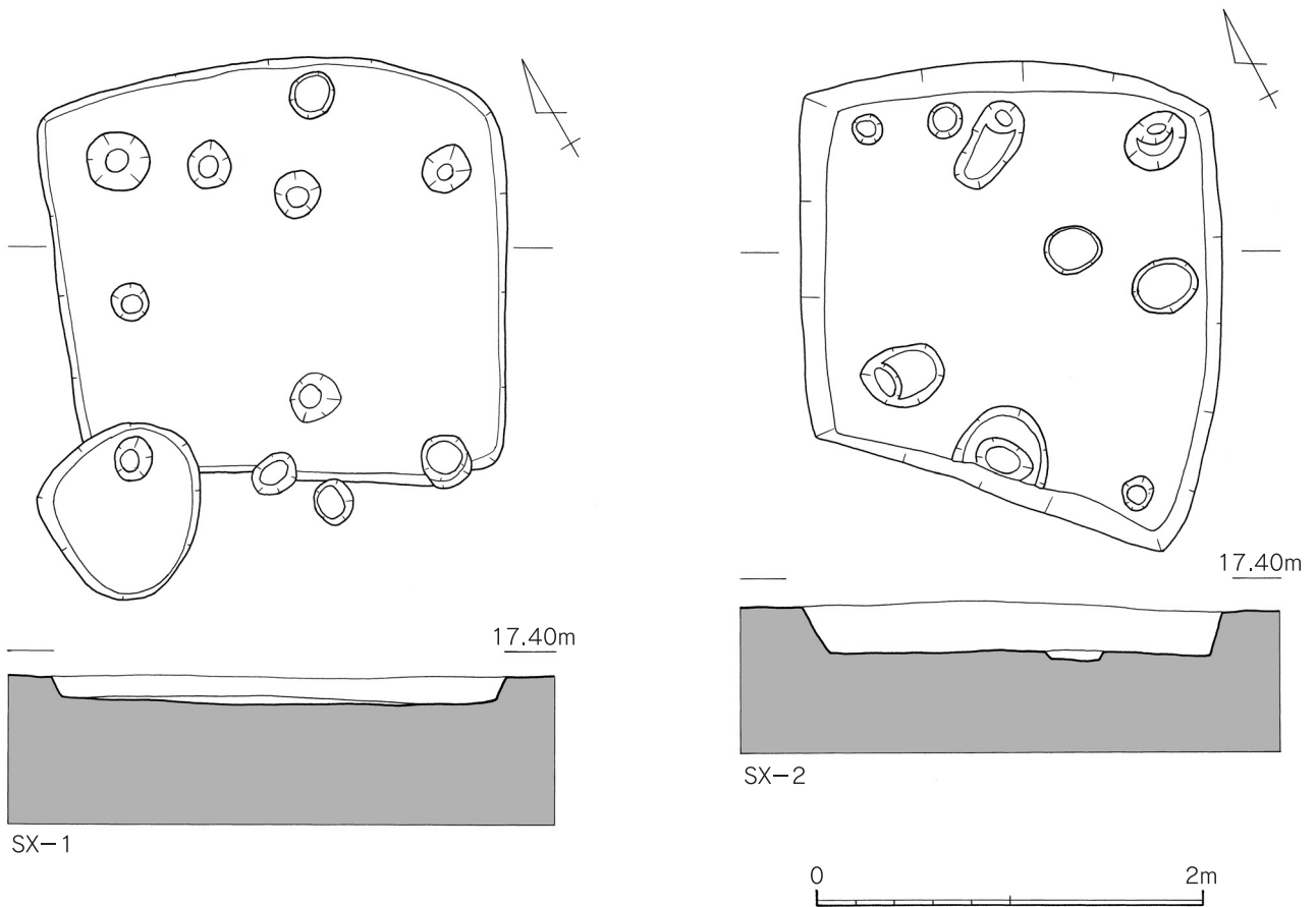
第9図 竪穴遺構実測図(縮尺1/40)
