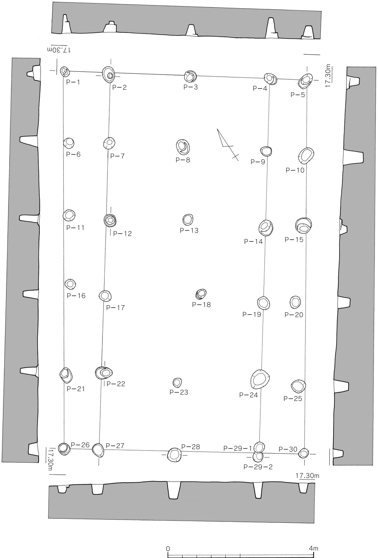
第12図 1号掘立柱建物跡実測図(縮尺1/60)
