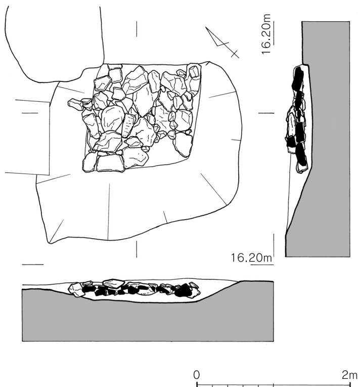
第18図 方形石組遺構実測図(縮尺1/50)
