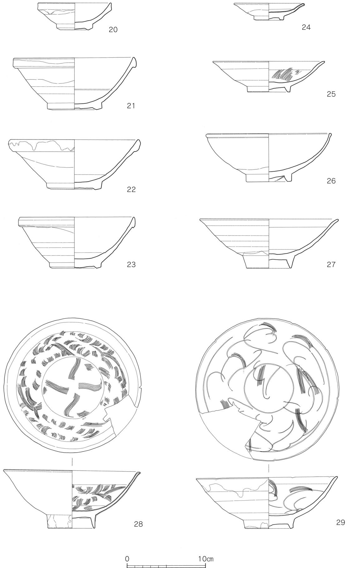
第24図 その他の遺構出土遺物実測図・2(縮尺1/3)
