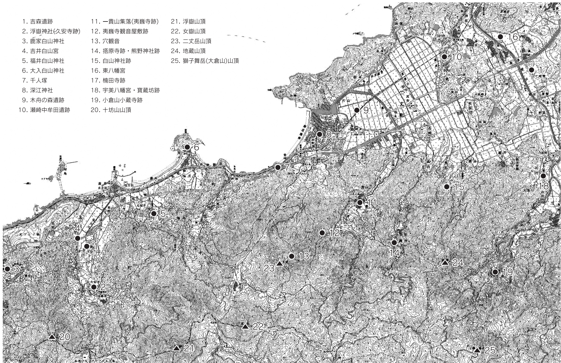
第1図 糸島市西部域図(縮尺 1/50,000)
