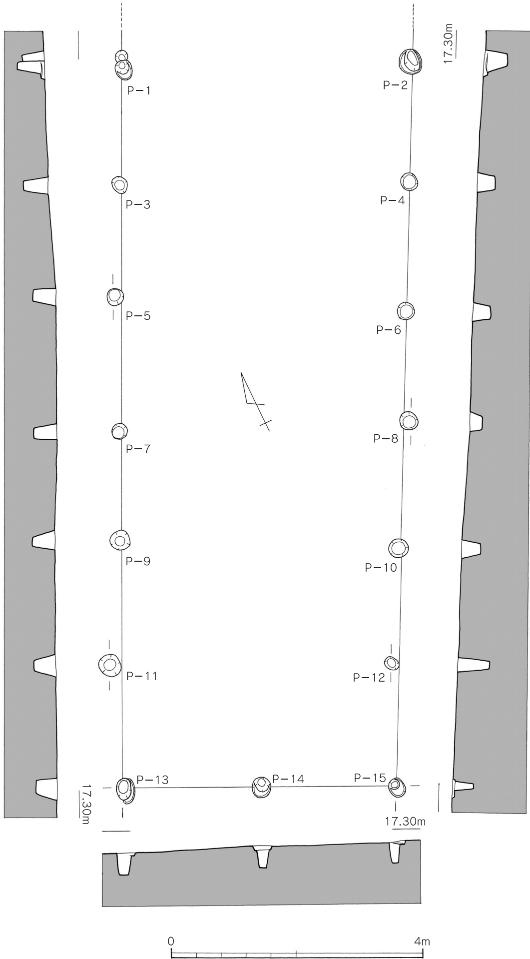
第13图 2号掘立柱建物跡実測図(縮尺1/60)
