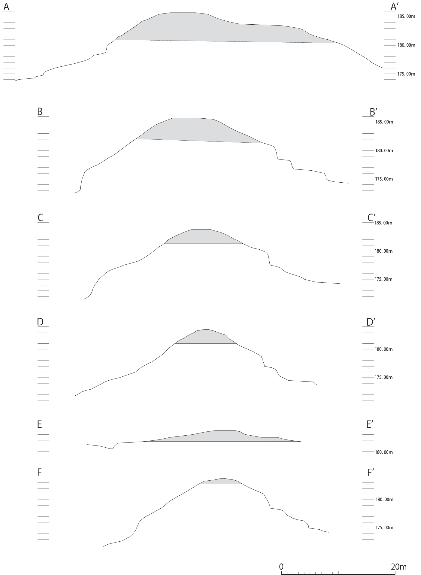
第 6 図 大久保 1・3 号墳縦横断面図 (1/400)
