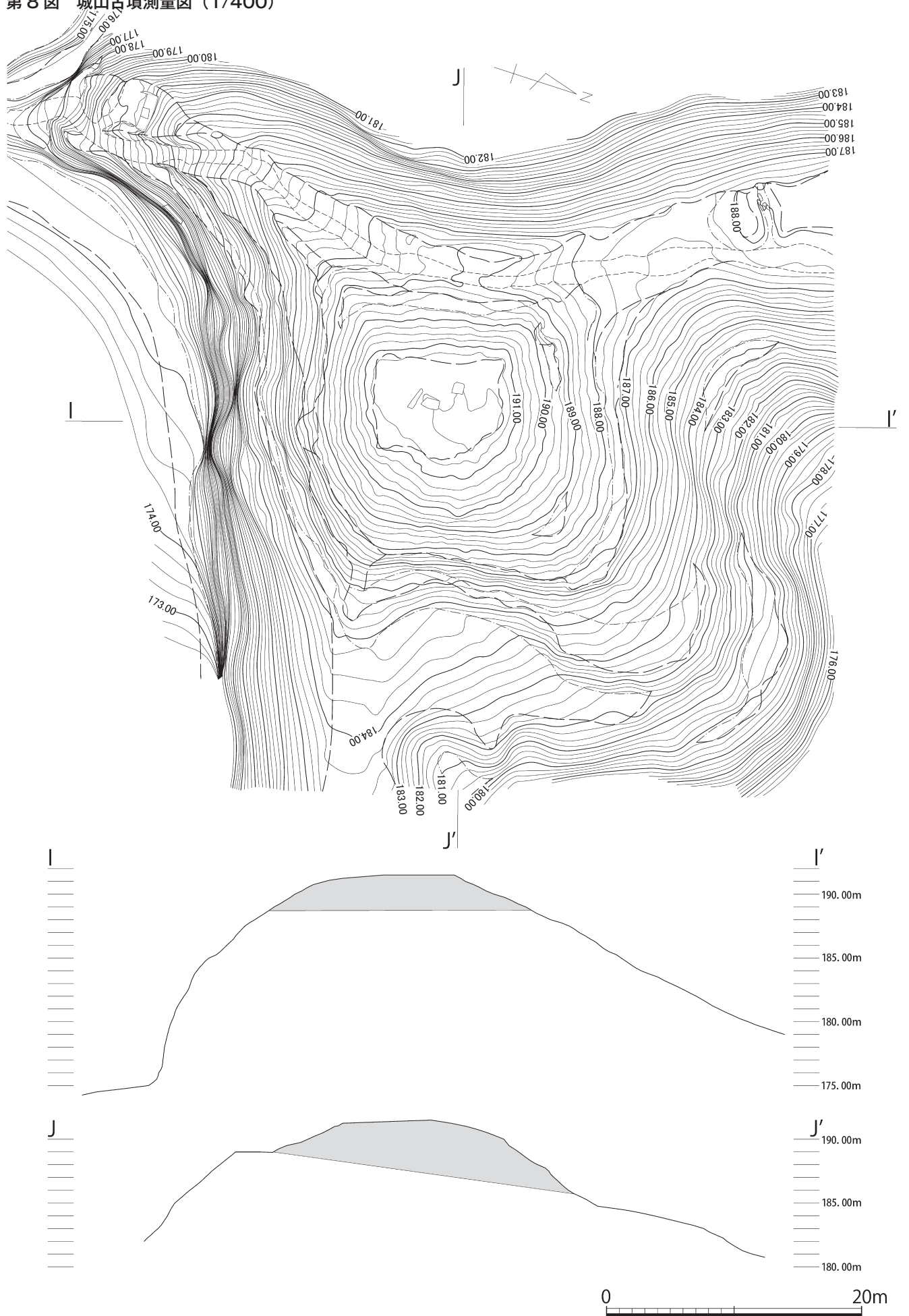
第 8 図 城山古墳測量図 (1/400)
