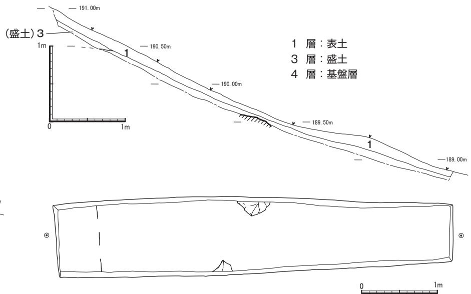
第17図 城山古墳 第1トレンチ (50分の1)
