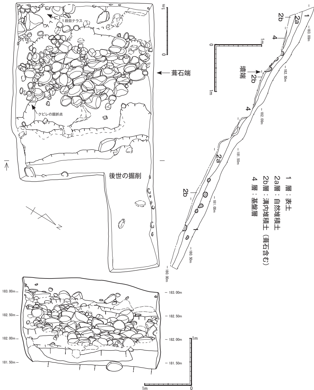
第11図 大久保1号墳 第2トレンチ (50分の1)
