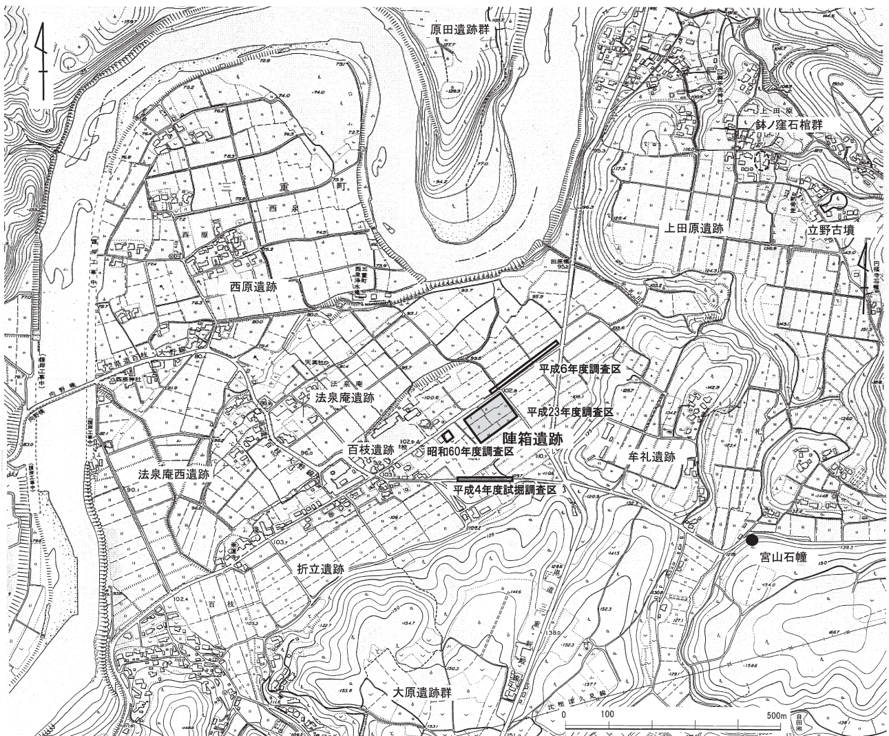
第19図 陣箱遺跡周辺地形図
