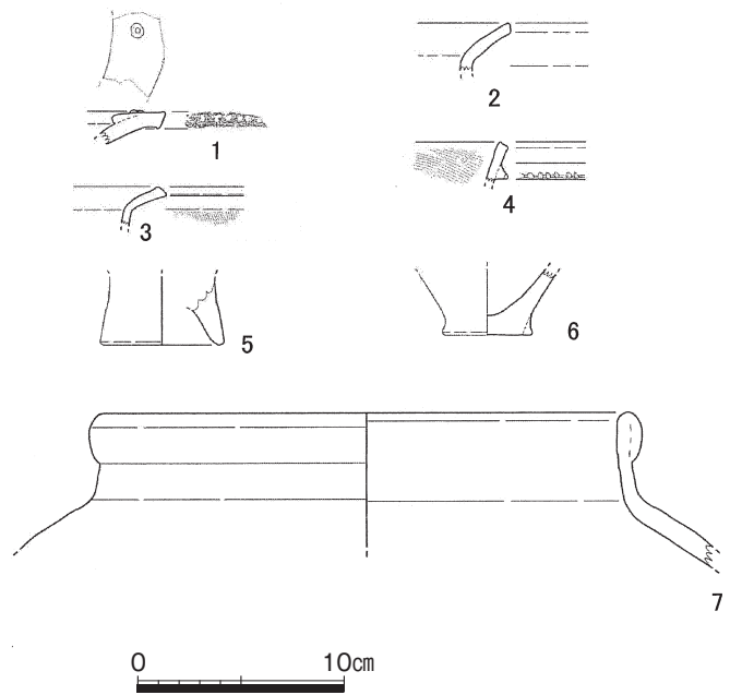
第 35 図 杉園中原遺跡採集遺物実測図
