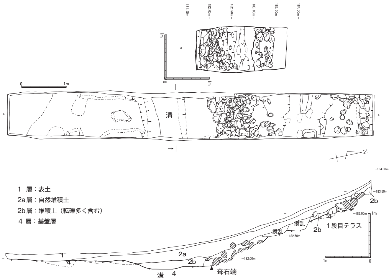
第10図 大久保1号墳 第1トレンチ (50分の1)
