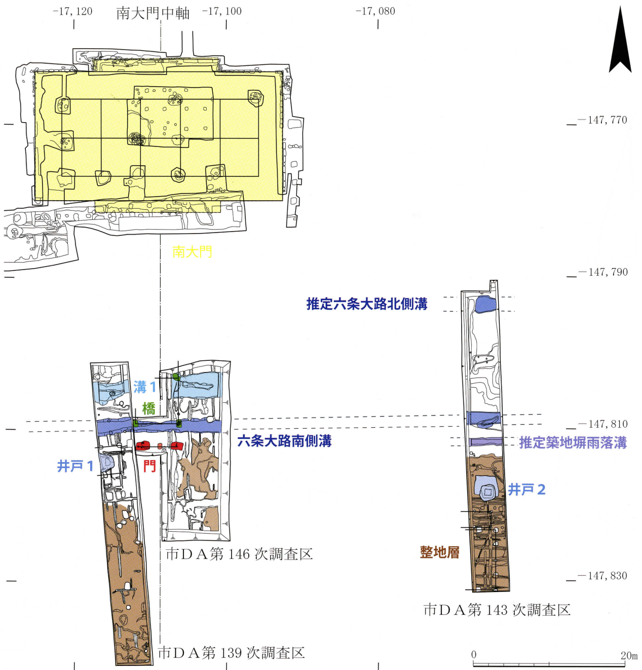
遺構平面図 (1/500)
