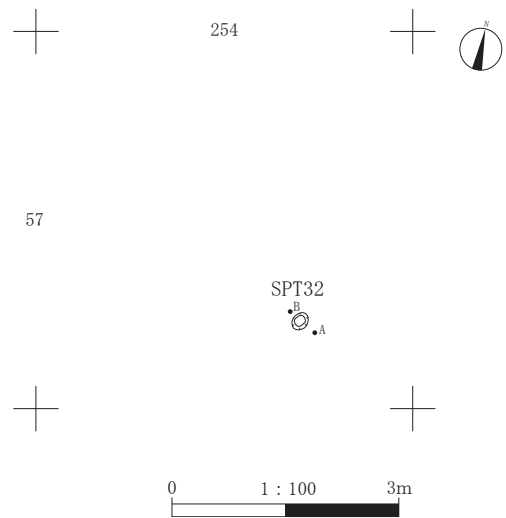
図 61 管理棟地点検出の小ピット平面図(10)
