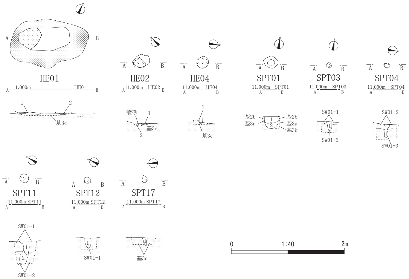
図 21 獣医学研究科大動物実験研究施設地点 HE 01, HE 02, HE 04, SPT 01, SPT 03, SPT 04, SPT 11, SPT 12, SPT 17 の平面図及びセクション図
