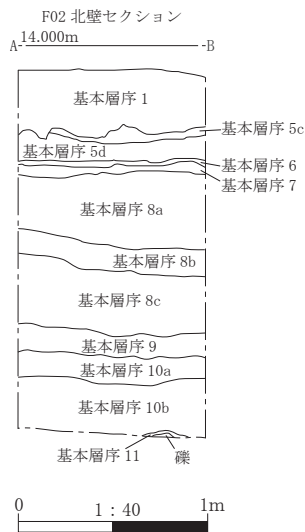
図 45 管理棟地点 F02 セクション図
