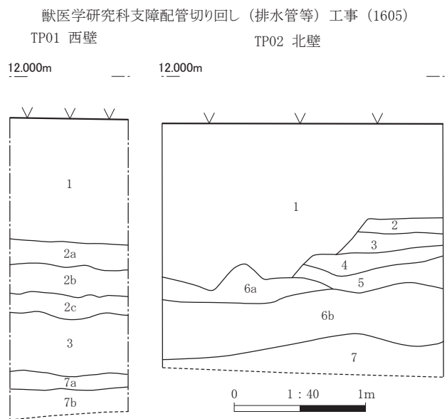
図80 構内確認・立会調査セクション図
