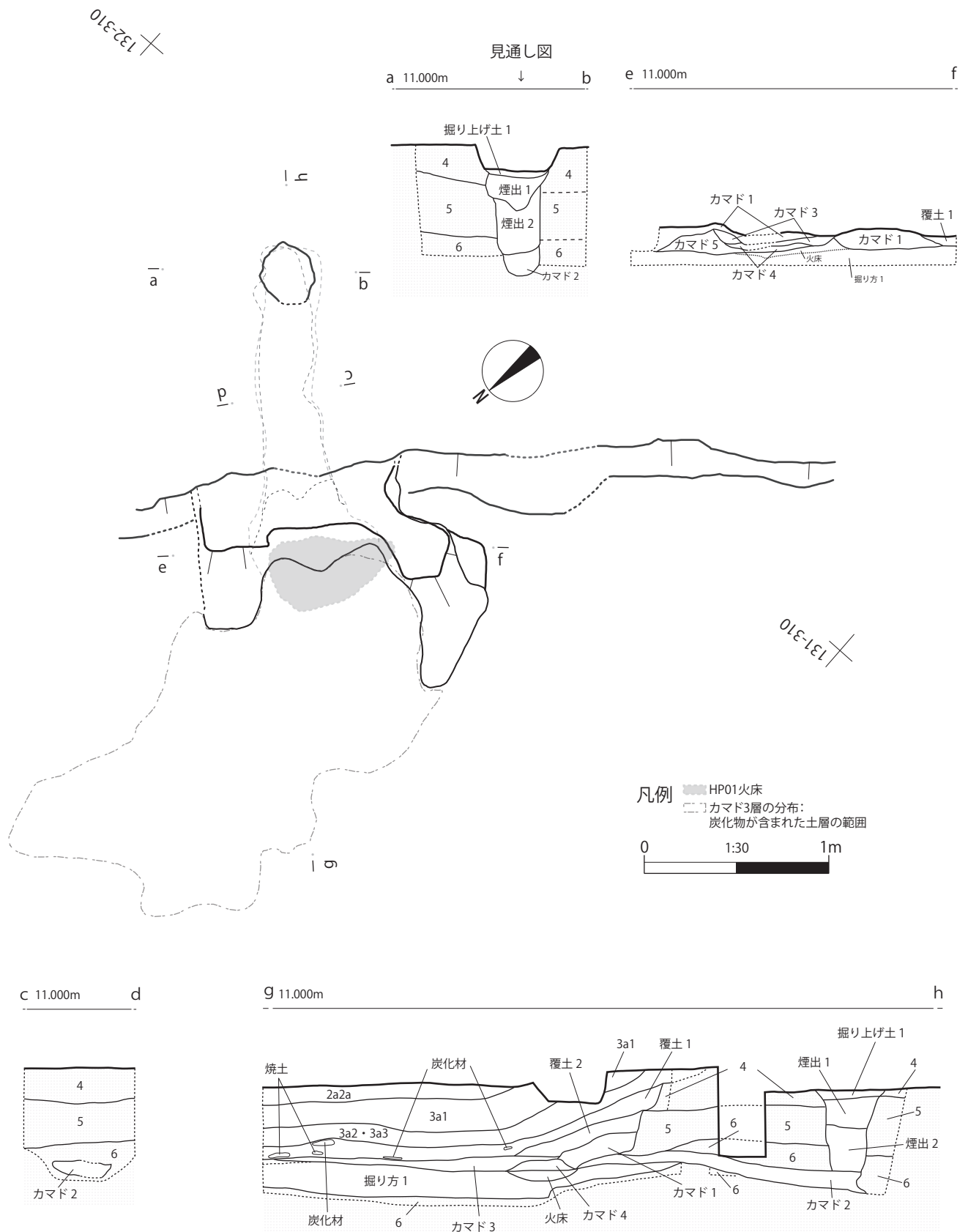
図 31 獣医学研究科大動物実験研究施設地点 HP 01 カマド平面図及びセクション図
