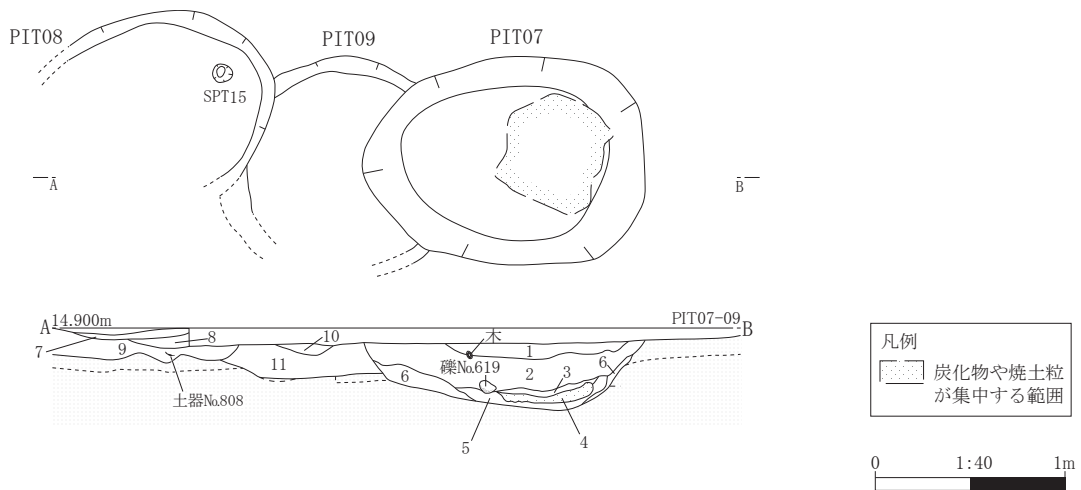
図 51 管理棟地点検出の土坑 PIT 07, 08, 09 南北断面図
