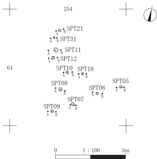
図 54 管理棟地点検出の小ピット平面図(3)
