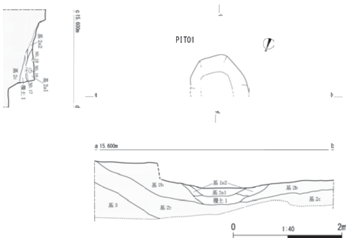
図 34 旧留学生センター改修地点 PIT 01 の平面図及びセクション図
