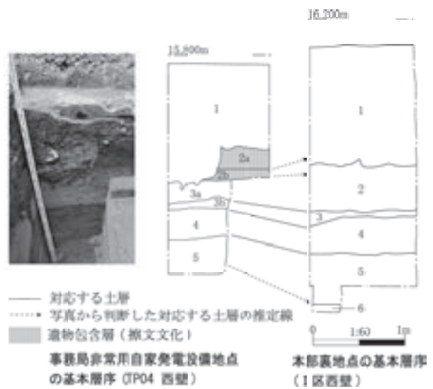
図 12 事務局非常用自家発電設備地点の基本層序と土層対比
