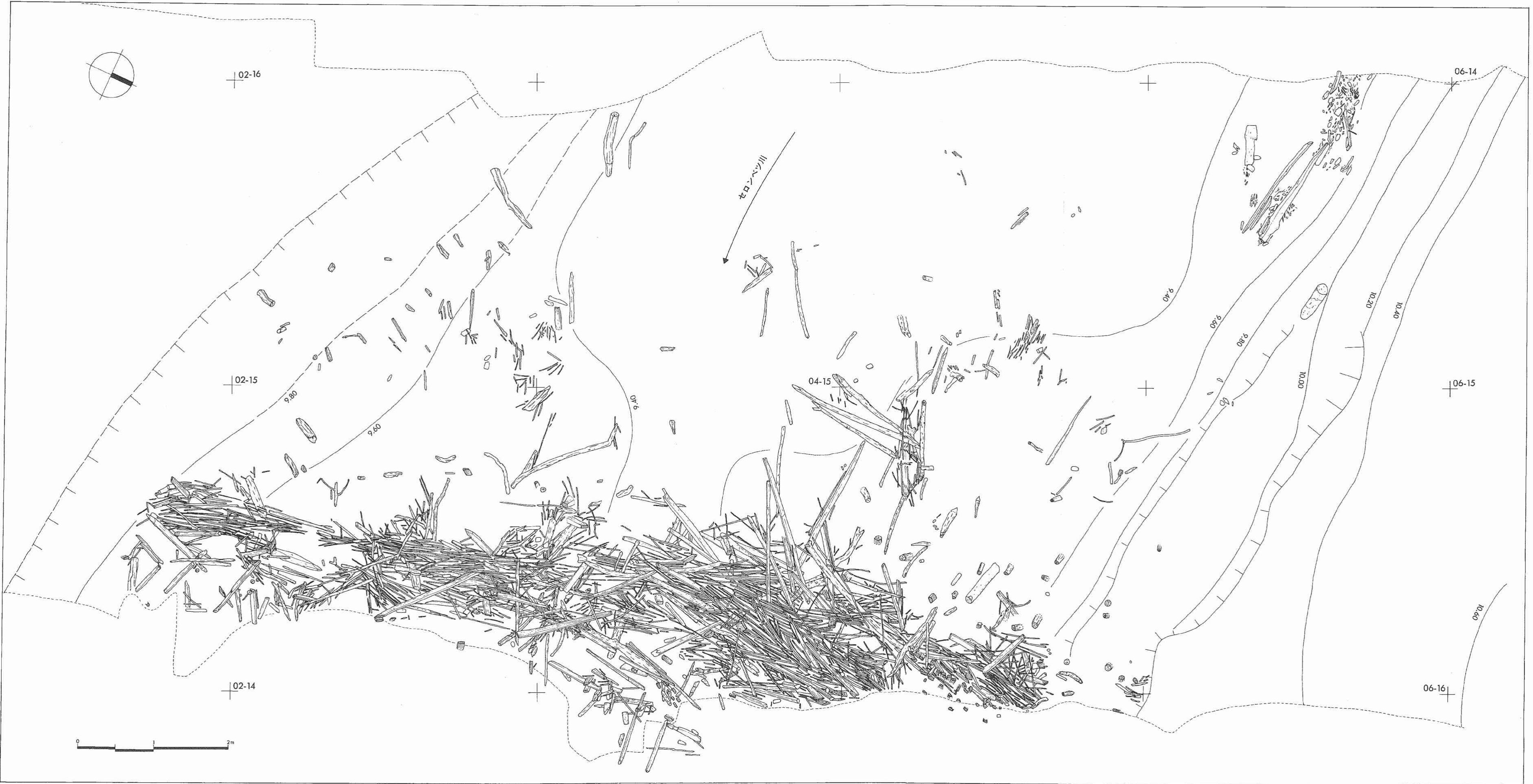
第7図 堰状遺構(テシ)実測図
