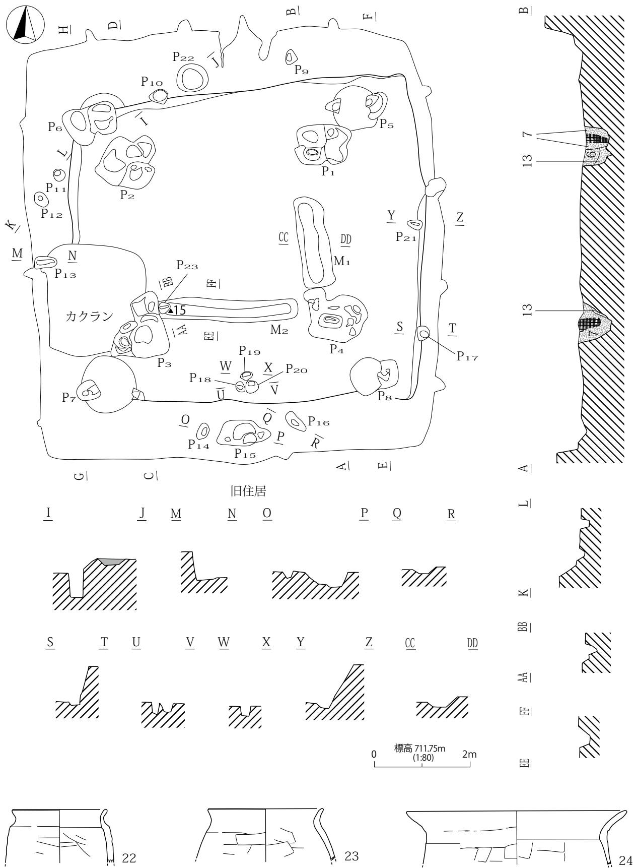
第 619 図 H458 号住居址 (3)
