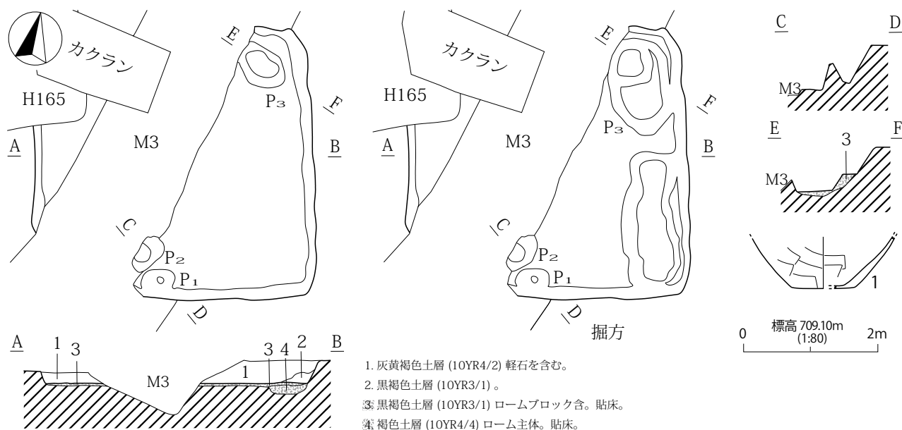
第 322 図 H51 号住居址
