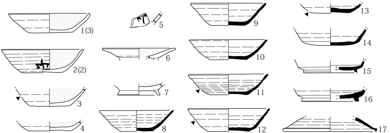
第353図 H158号住居址(1)
