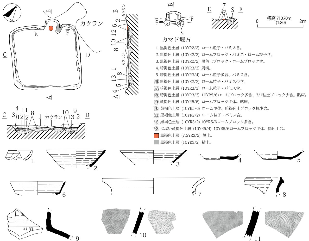
第 575 図 H404 号住居址
