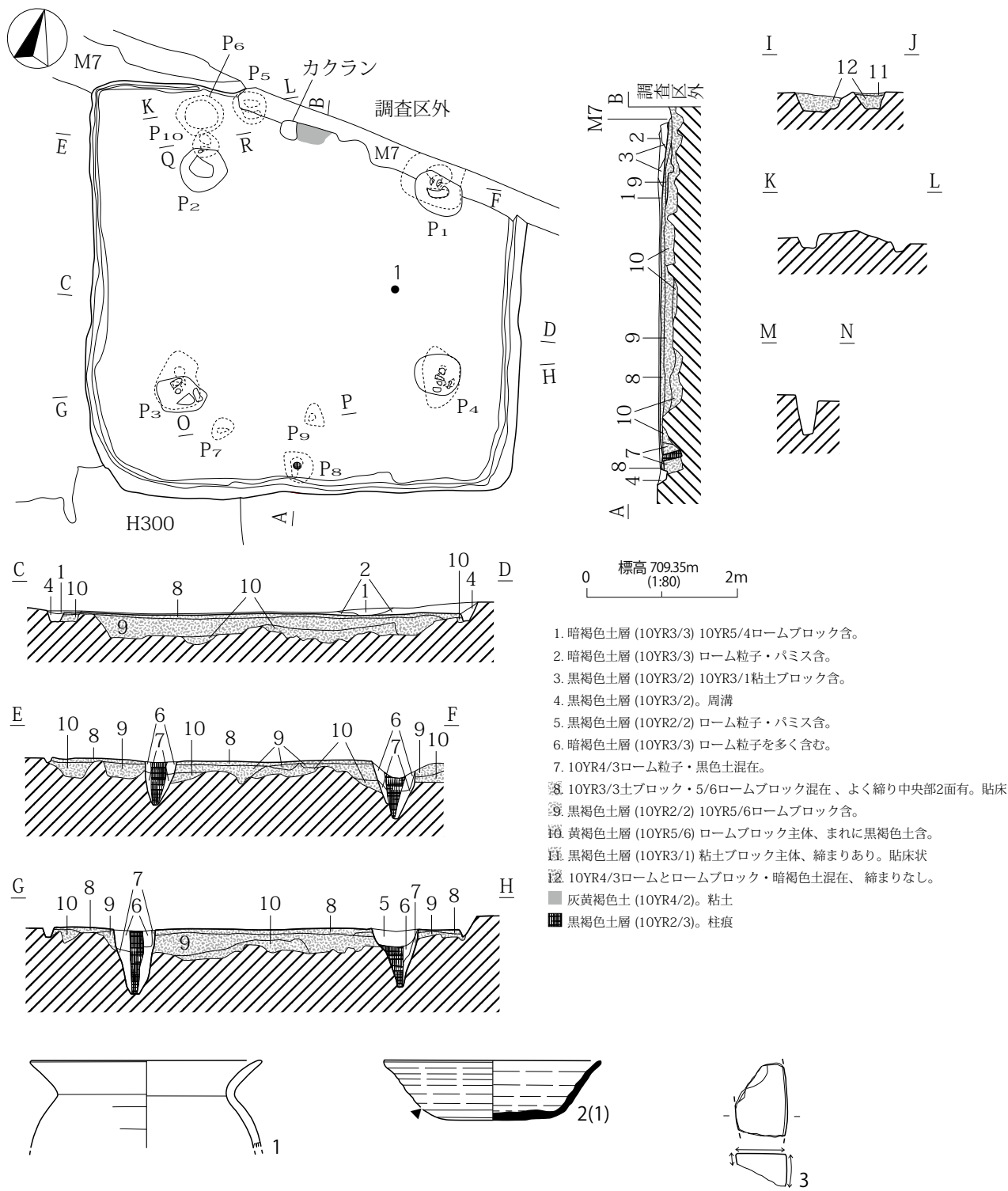
第381図 H211号住居址
