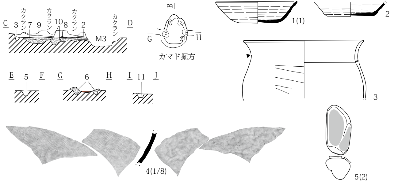
第492図 H314号住居址
