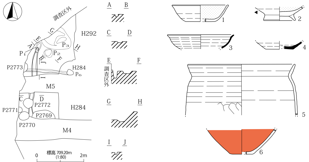
第502図 H323号住居址
