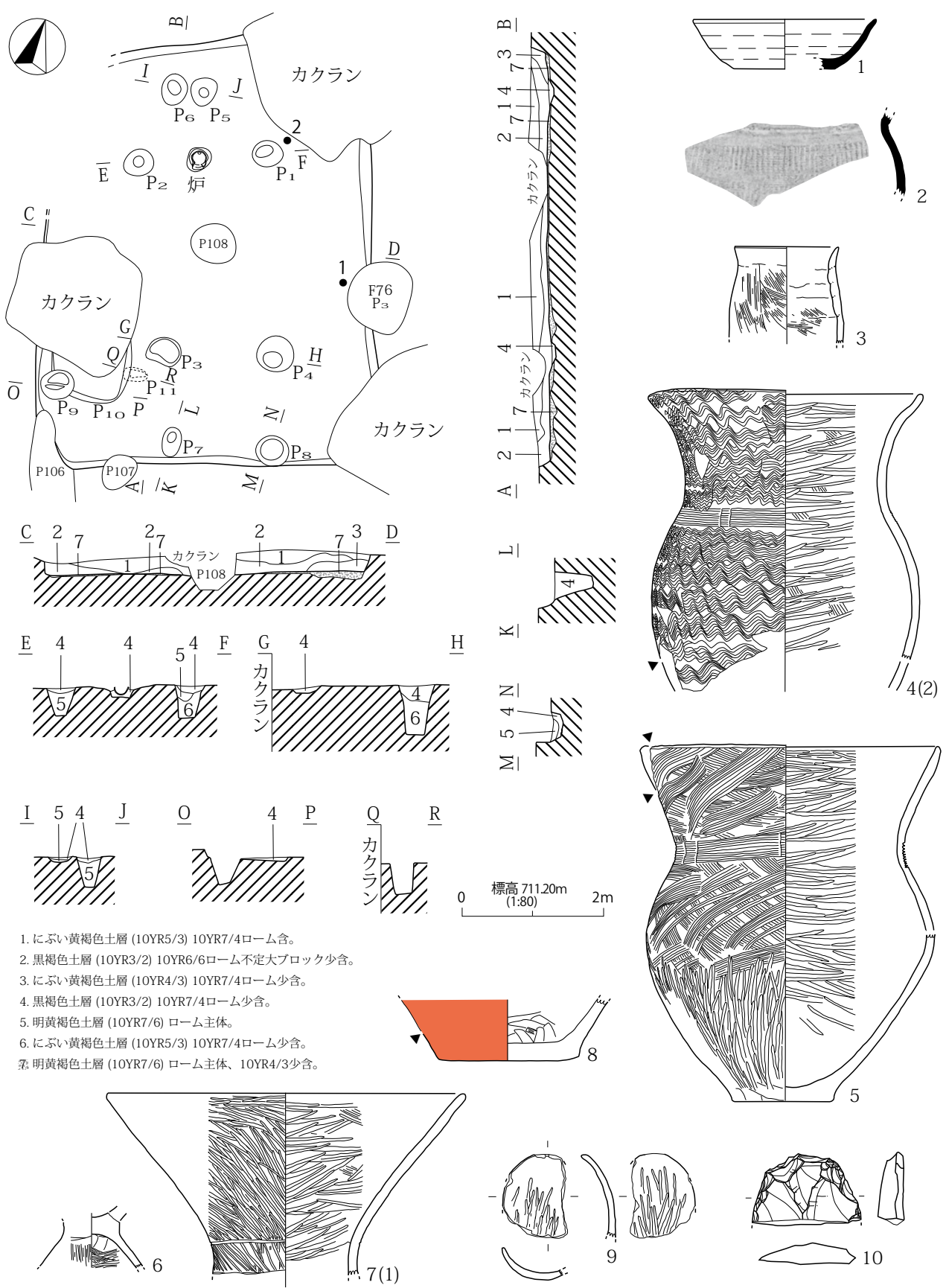
第 305 図 H2 号住居址
