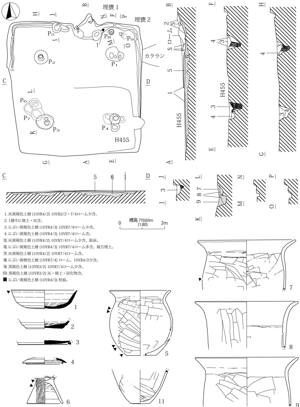
第609図 H455号住居址(1)
