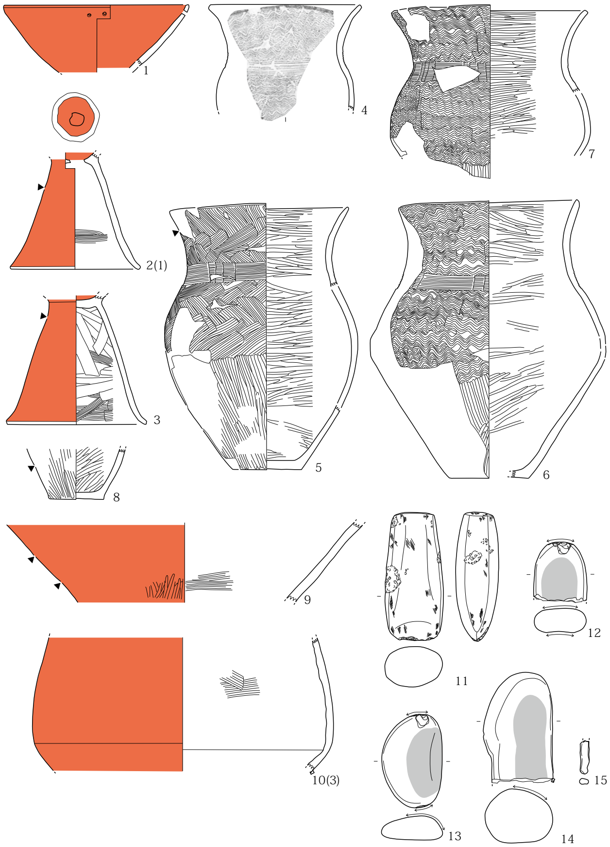
第 613 图 H454 号住居址 (2)
