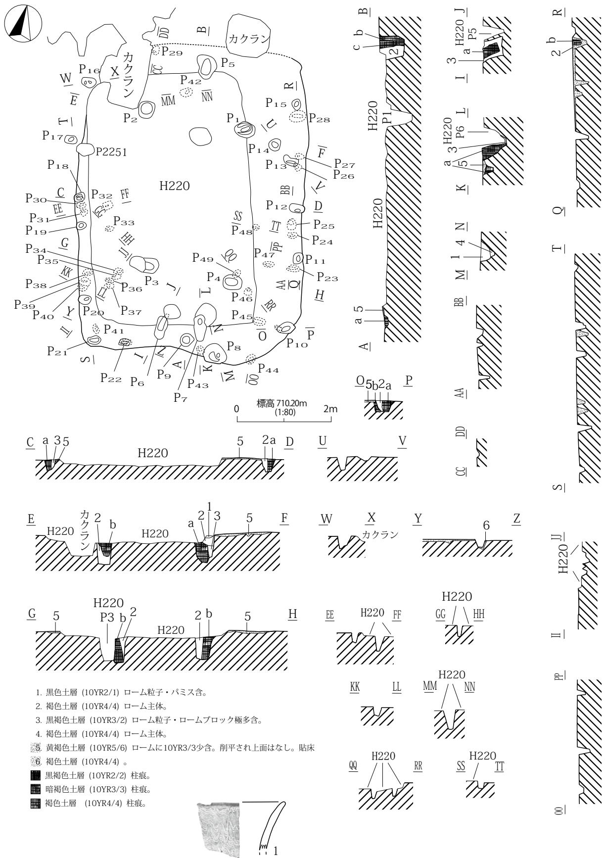
第429図 H237号住居址
