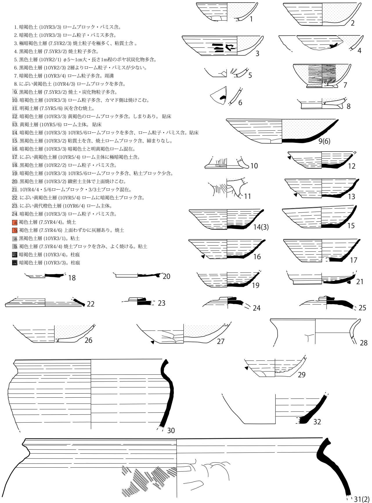
第330図 H71号住居址(2)
