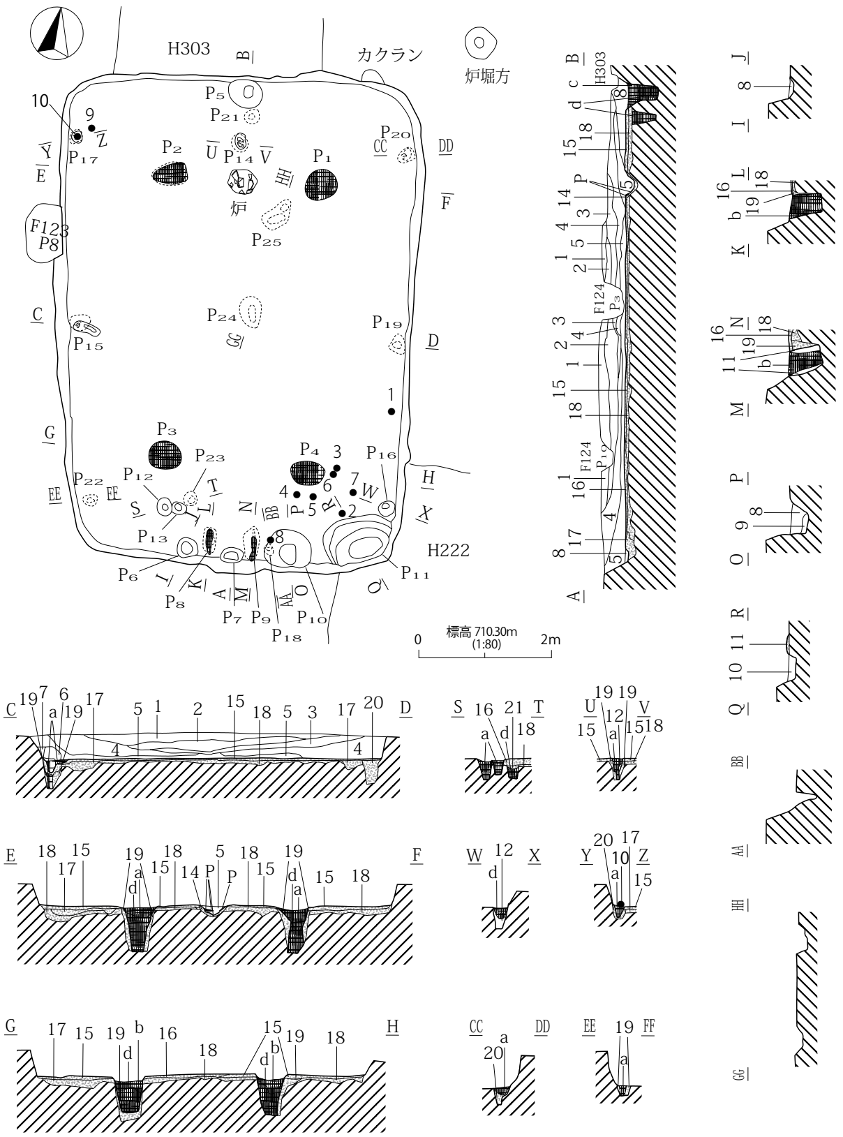
第473図 H304号住居址(1)
