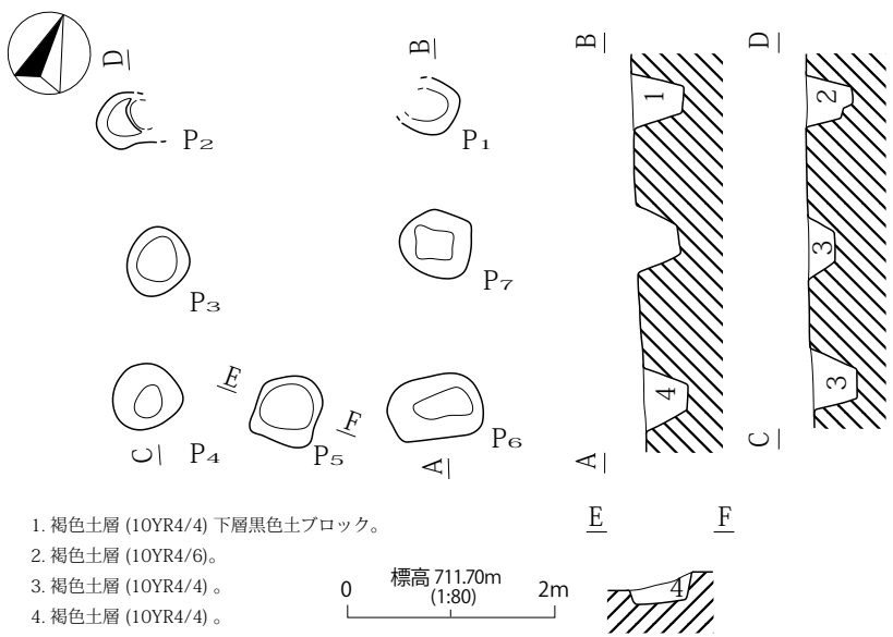
第 636 図 F1 号掘立柱建物址
