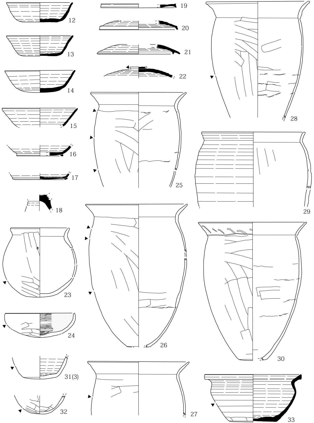
第 542 图 H356 号住居址 (2)
