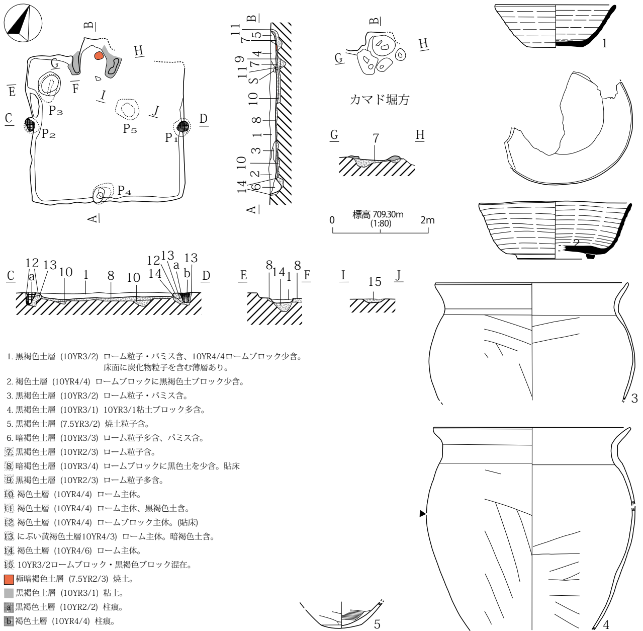
第469図 H300号住居址
