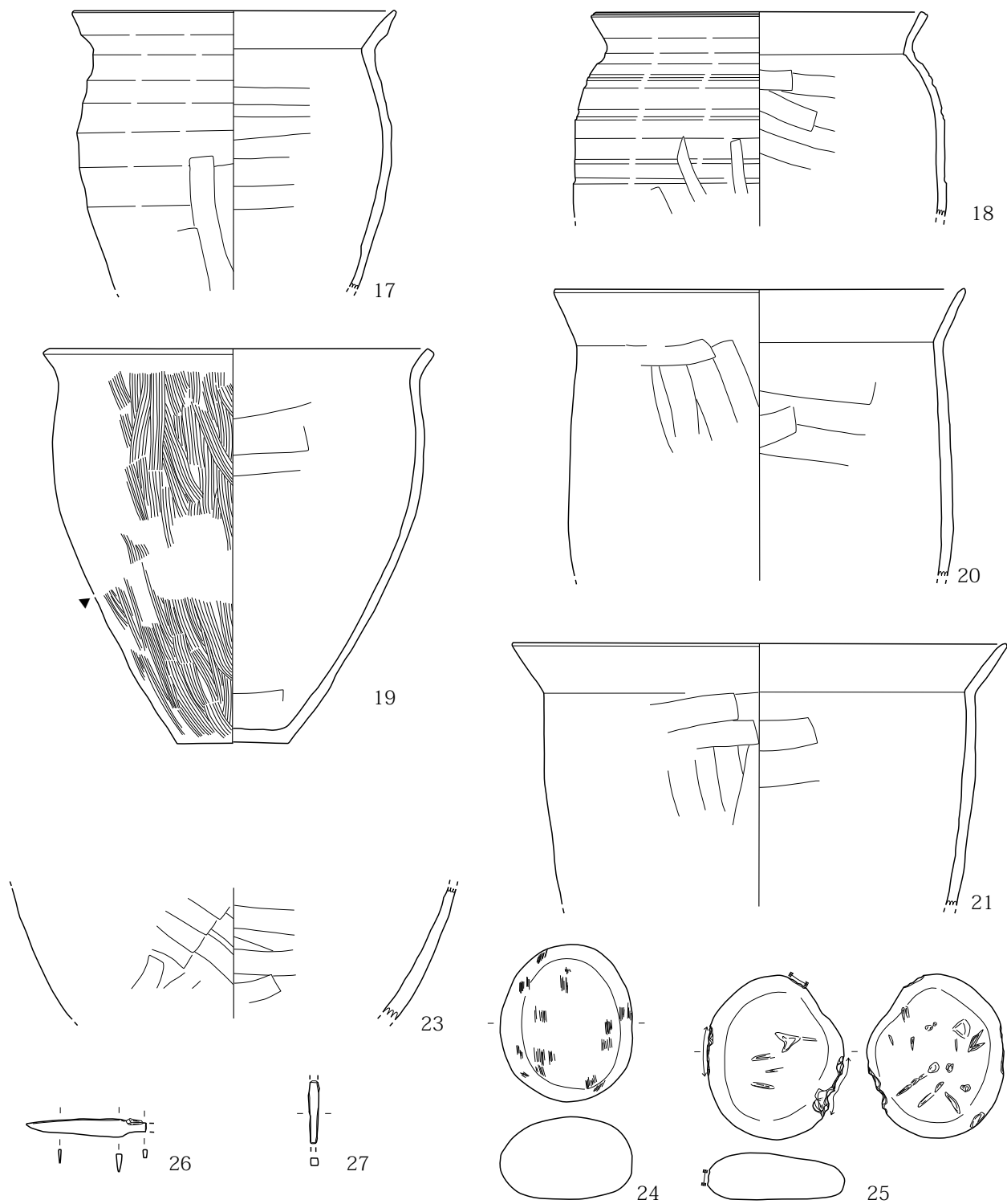
第534图 H348号住居址(2)
