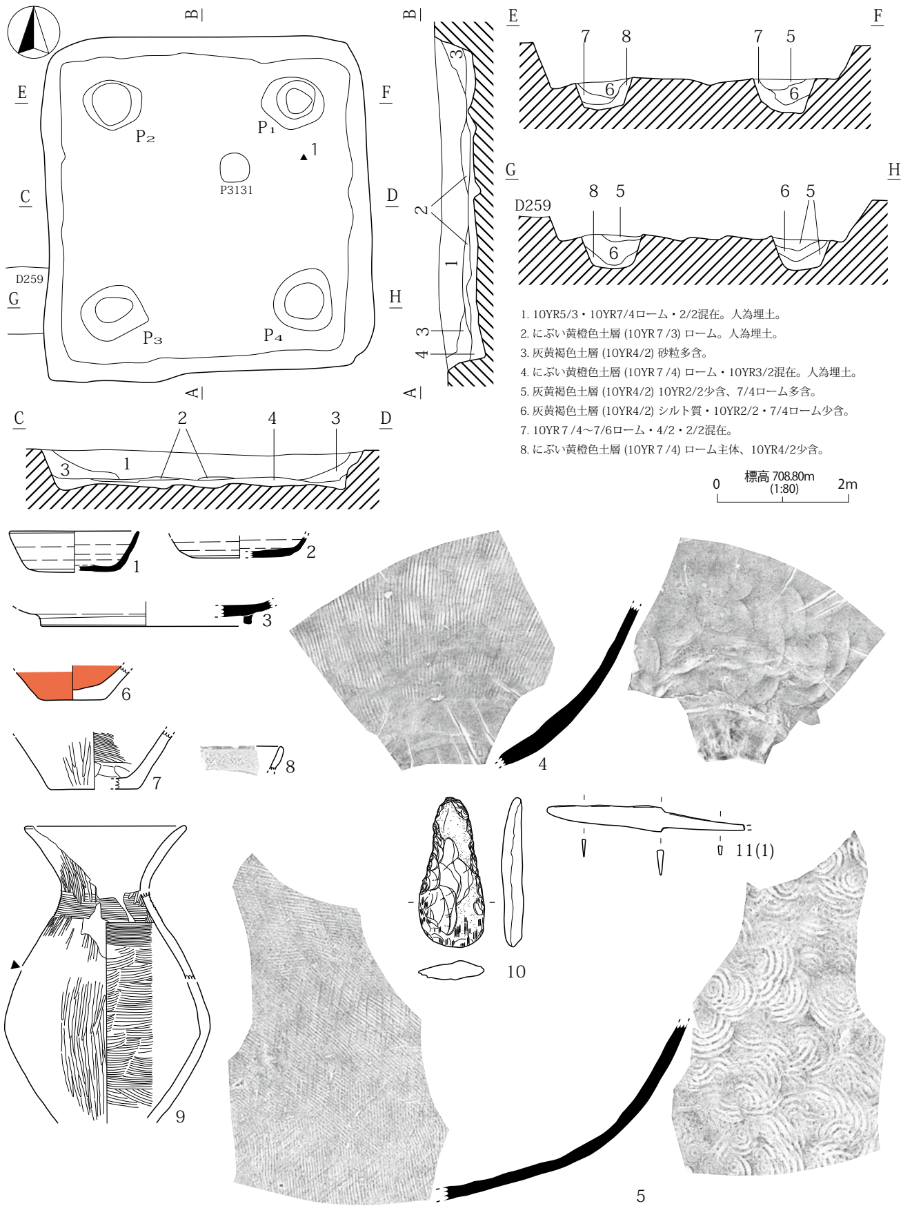
第 551 図 H361 号住居址
