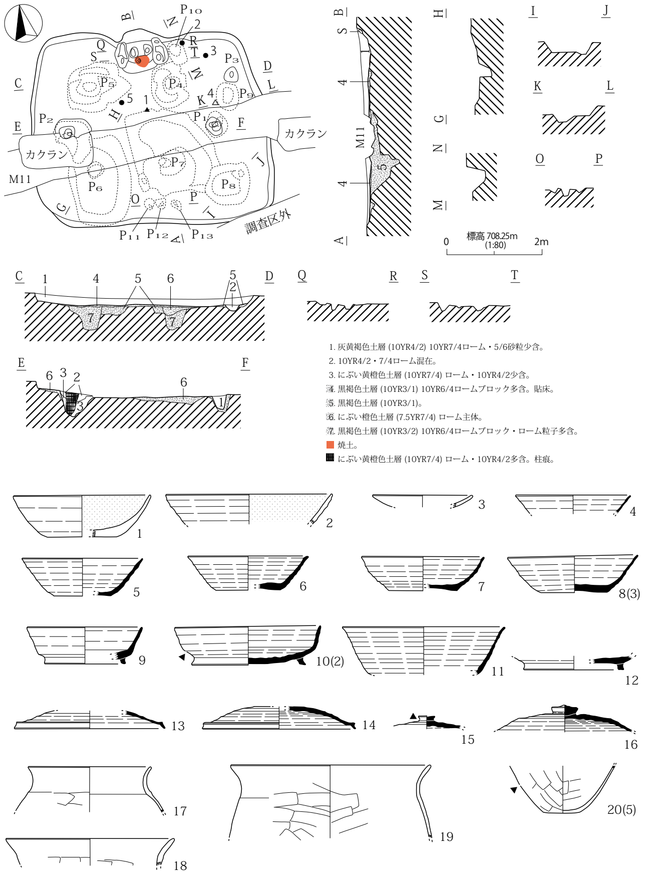
第 548 図 H359 号住居址 (1)
