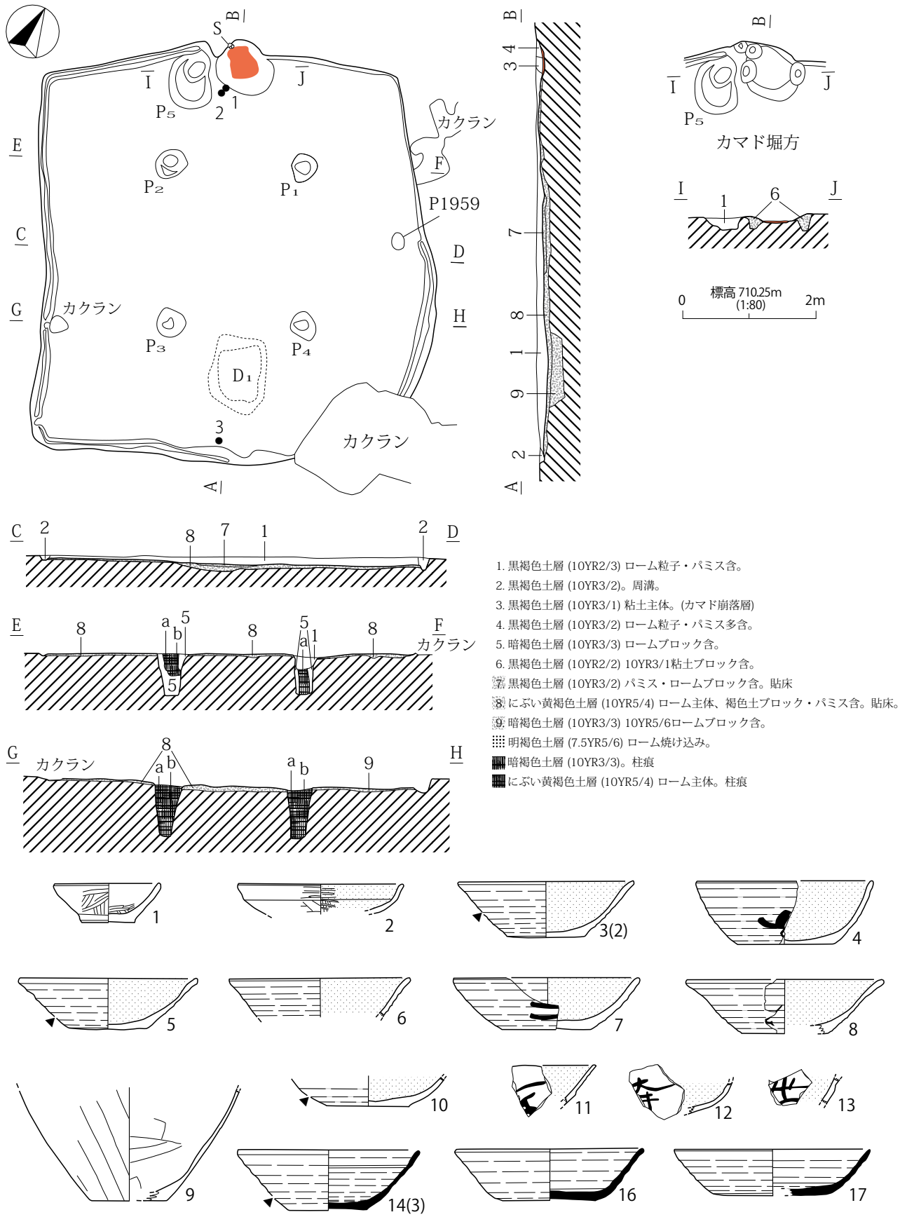
第386図 H214号住居址(1)
