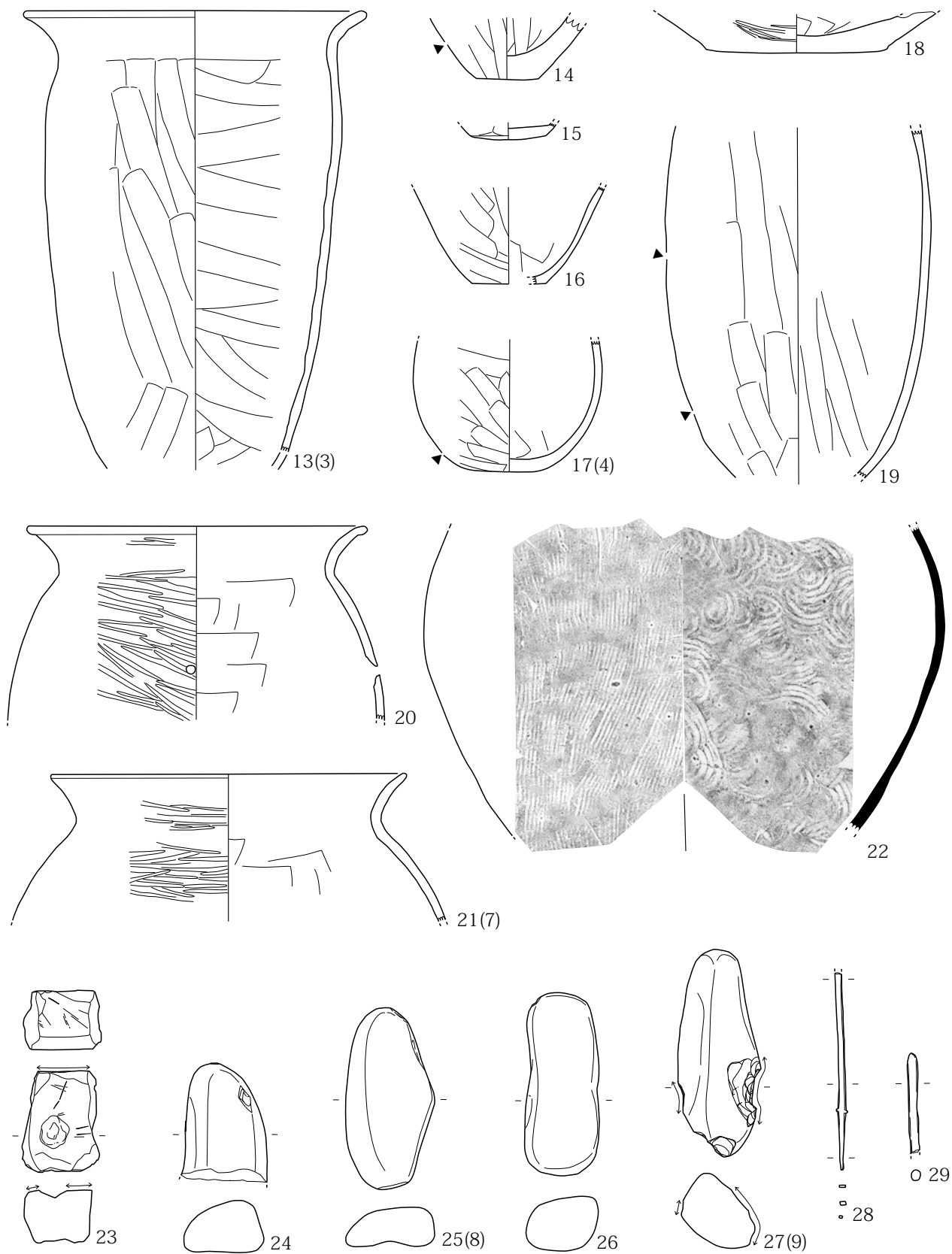
第 436 图 H249 号住居址 (2)
