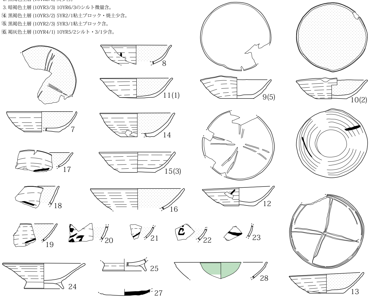
第 447 図 H285 号住居址 (1)
