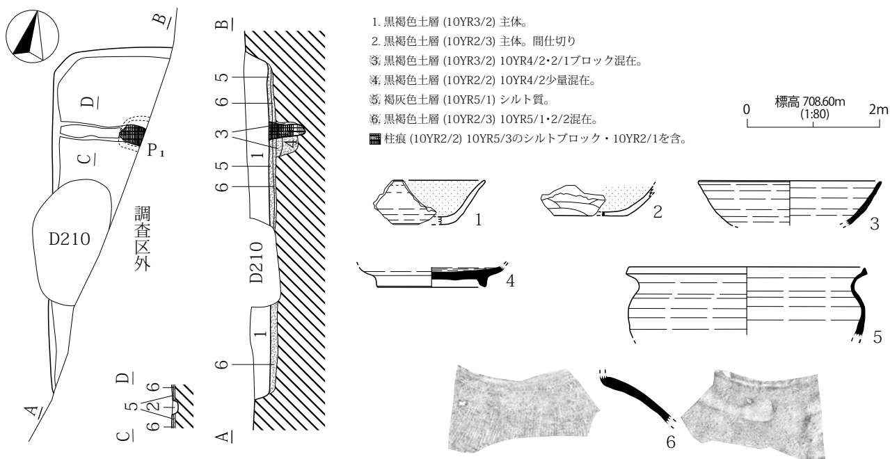
第 508 図 H330 号住居址
