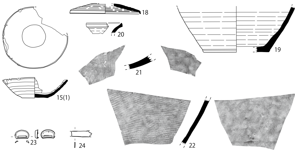
第387图 H214号住居址(2)
