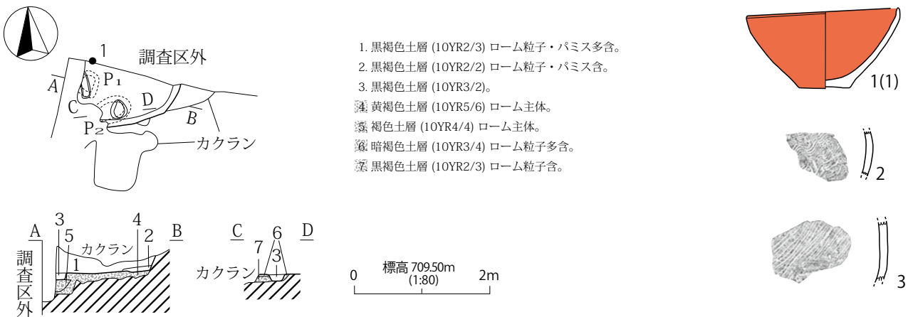
第368図 H175号住居址
