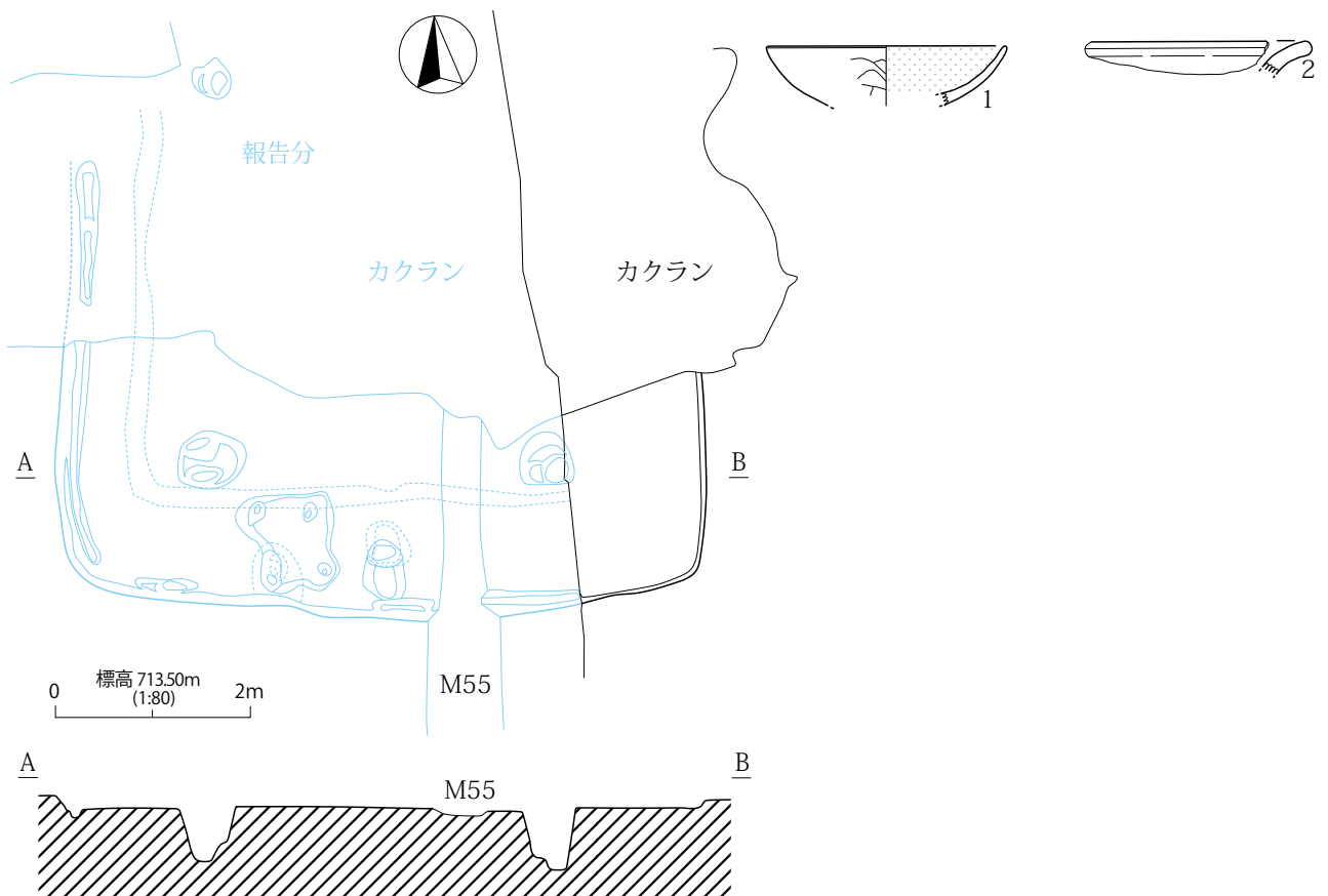
第 370 図 H199 号住居址
