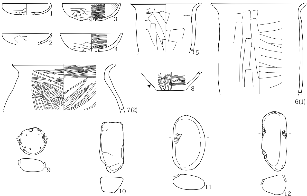
第 489 図 H312 号住居址 (2)
