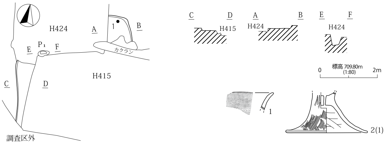
第 591 図 H427 号住居址
