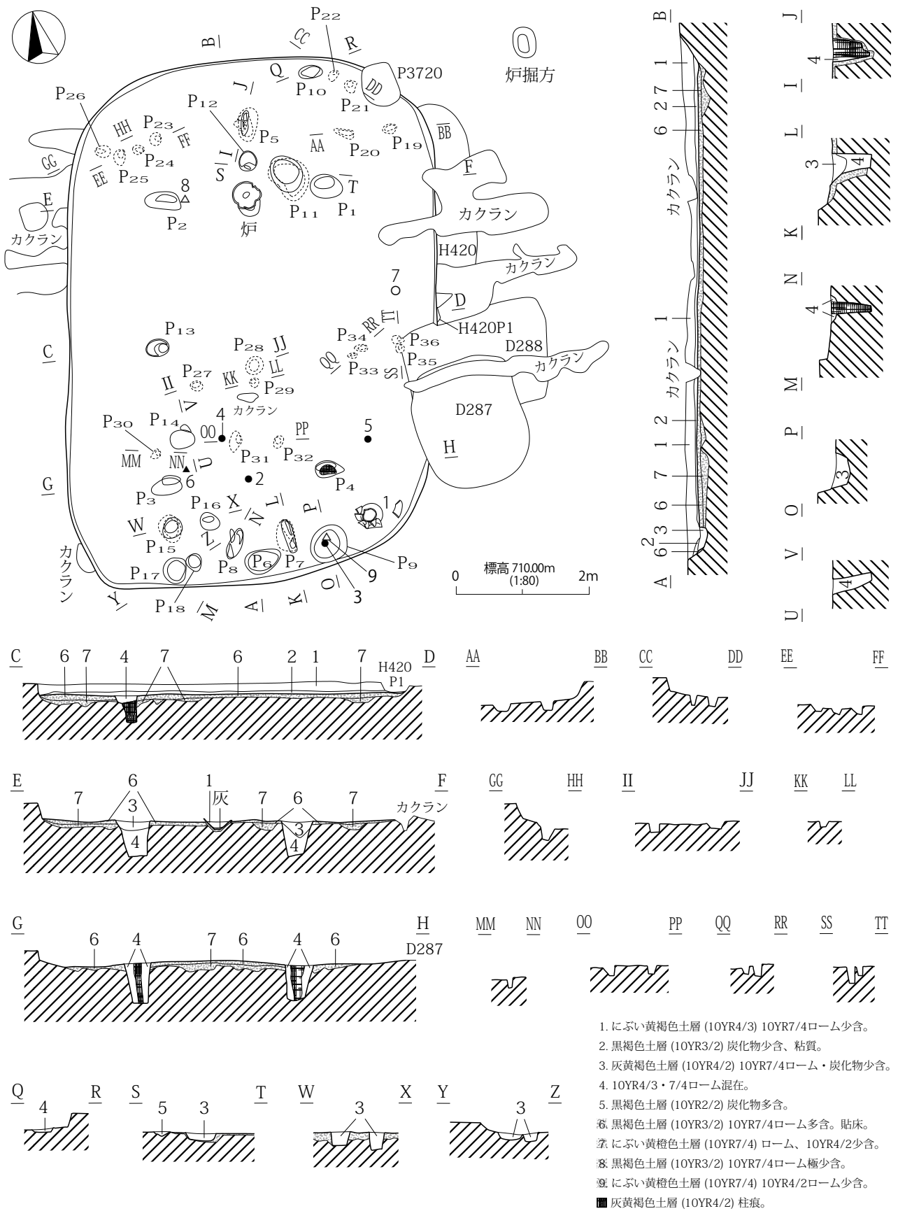
第584図 H421号住居址(1)
