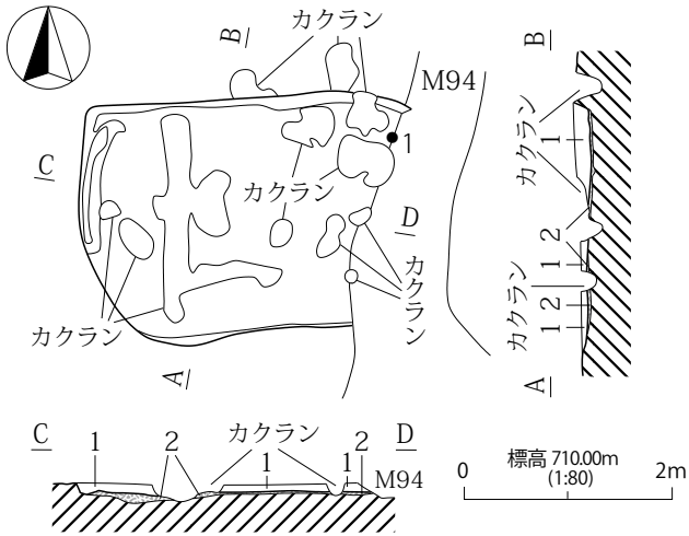
第 601 図 H445 号住居址
