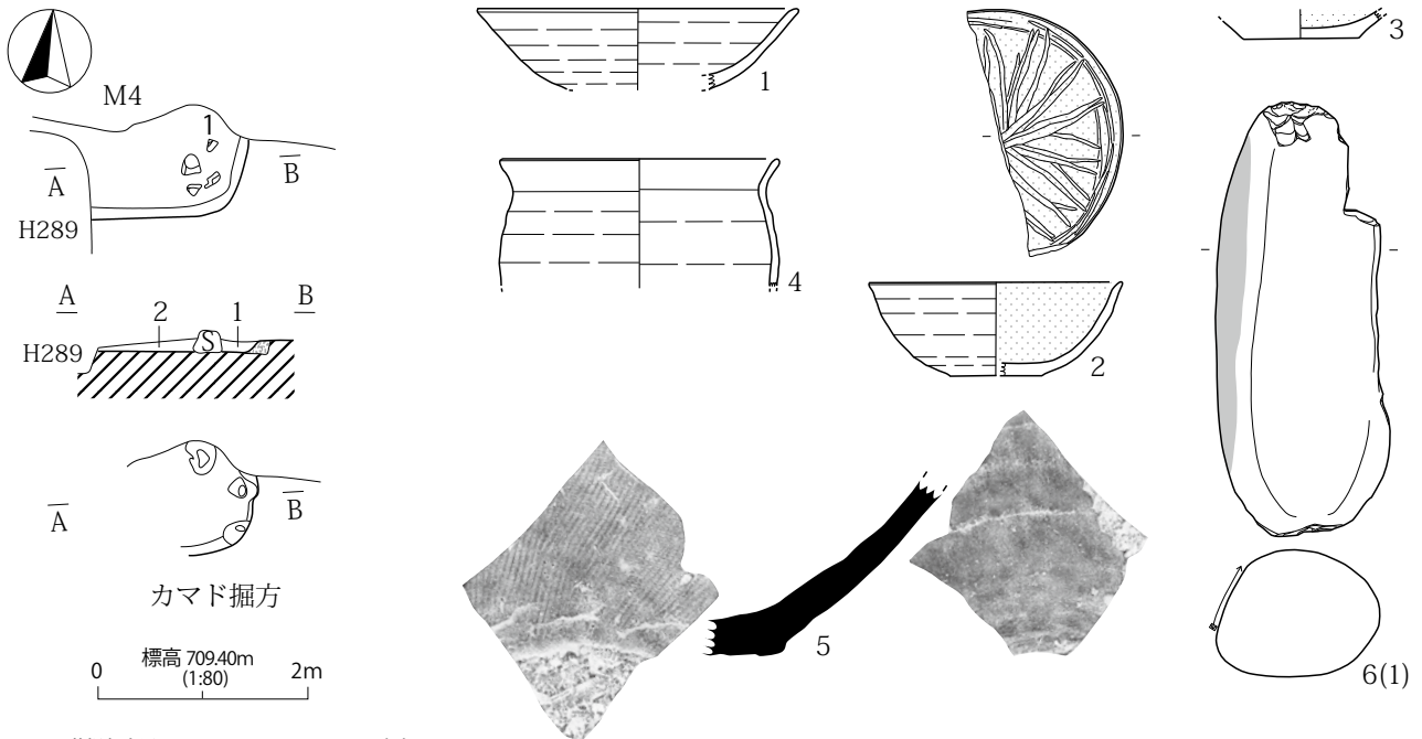
第465図 H297号住居址(2)
