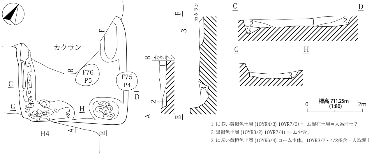
第 347 図 H119 号住居址
