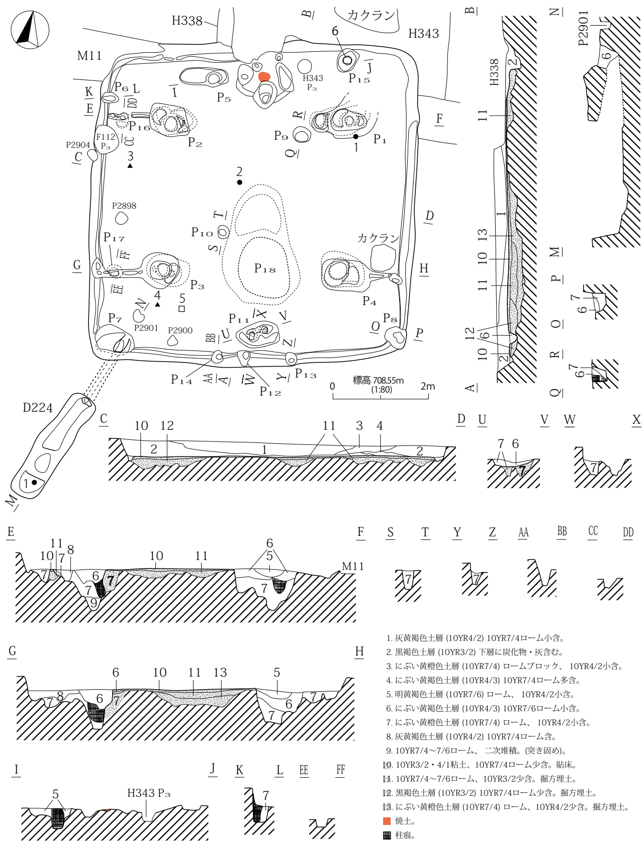
第 518 図 H337 号住居址・D224 号土坑 (1)
