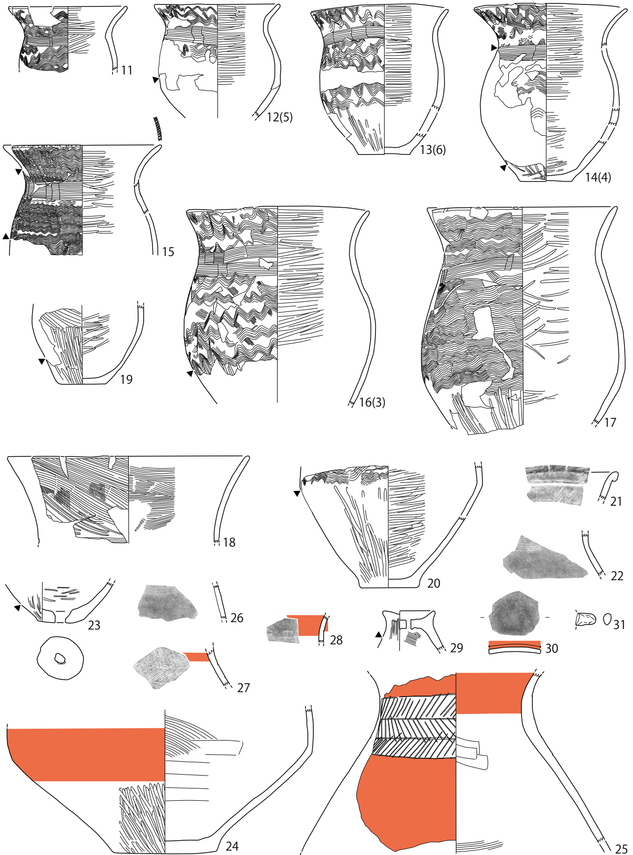
第 403 图 H223 号住居址 (2)
