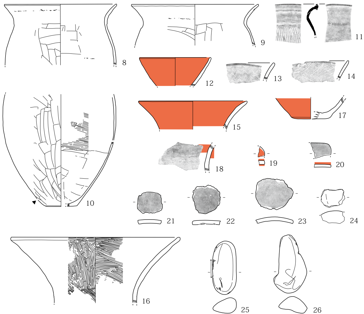
第 580 图 H415 号住居址 (2)
