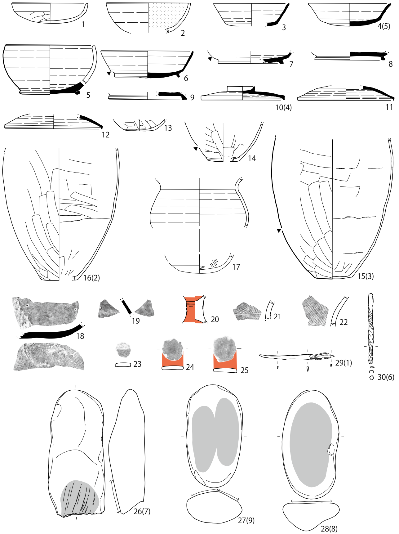
第 378 图 H208 号住居址 (2)
