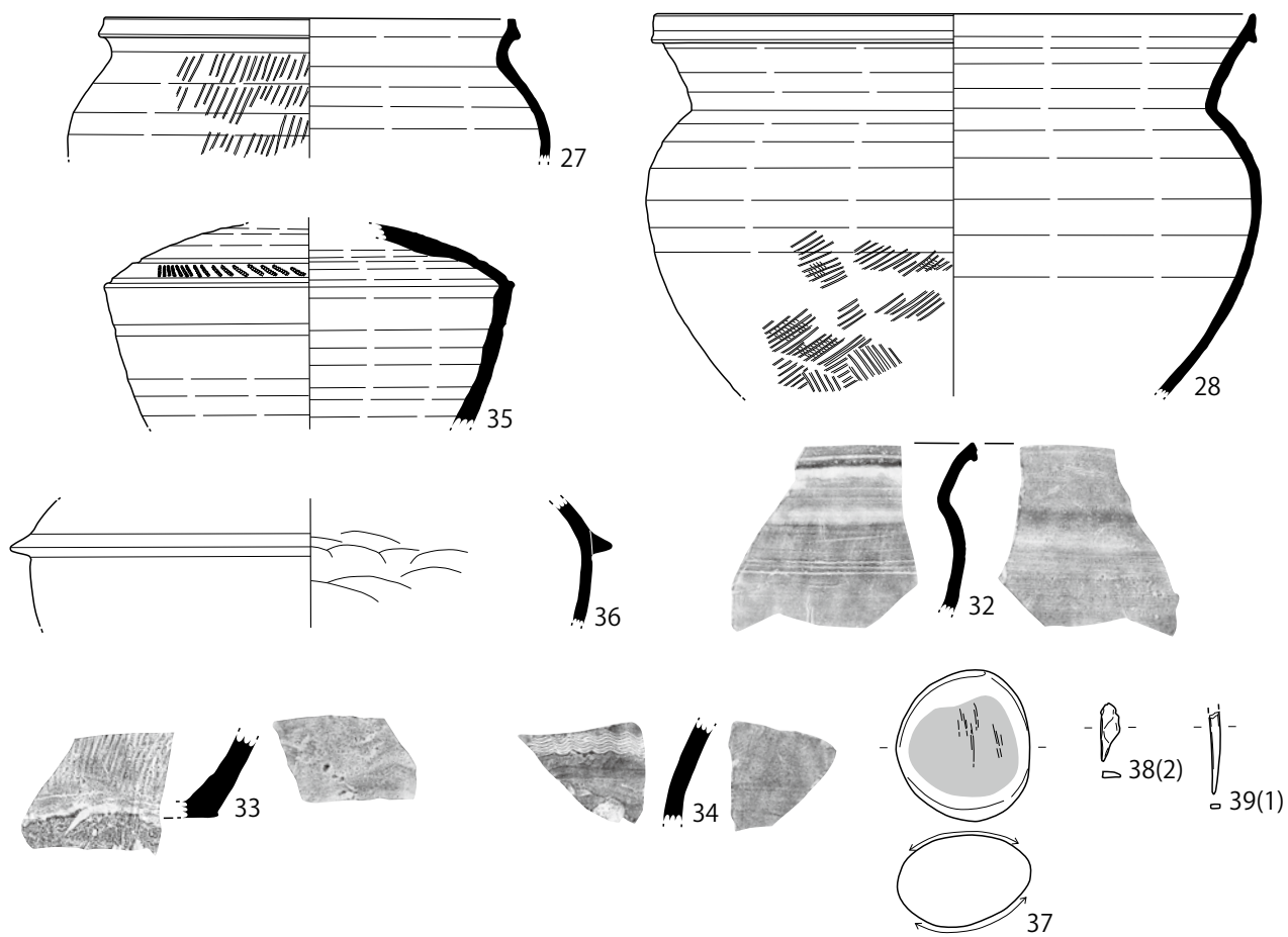
第384图 H212号住居址(3)
