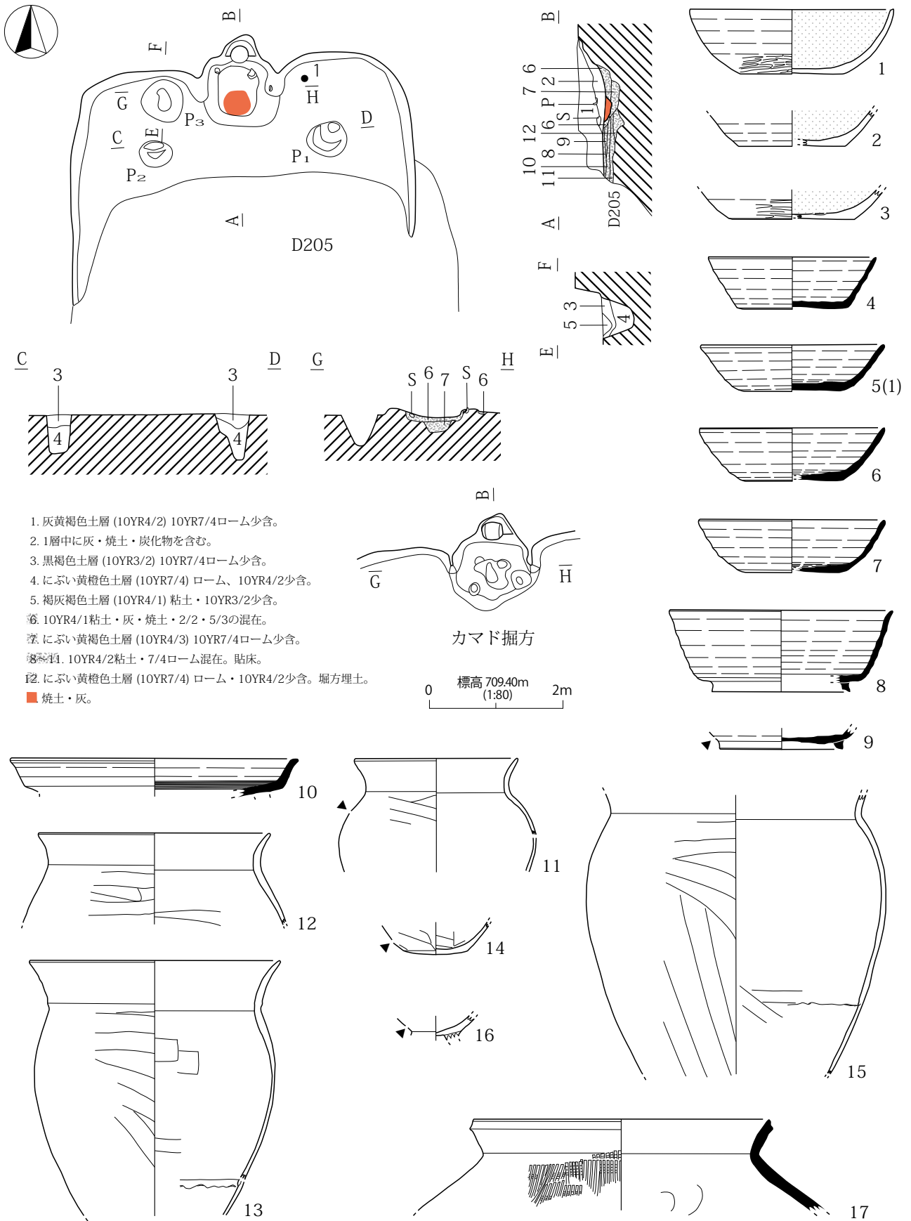
第464図 H297号住居址(1)
