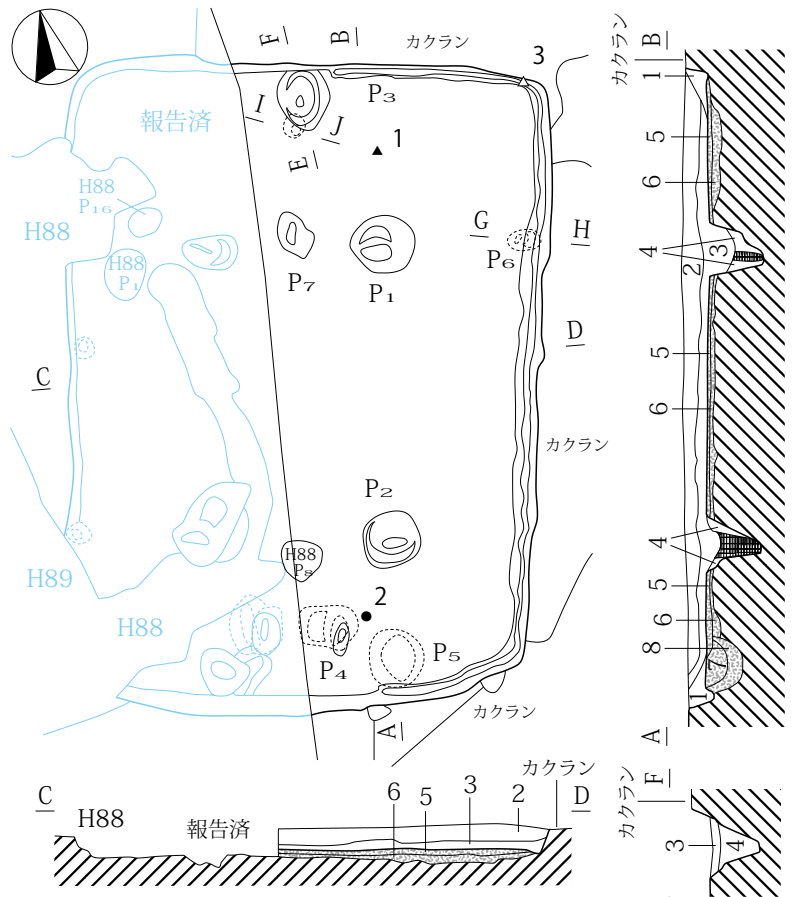
第350図 H129号住居址(2) 14(3)
