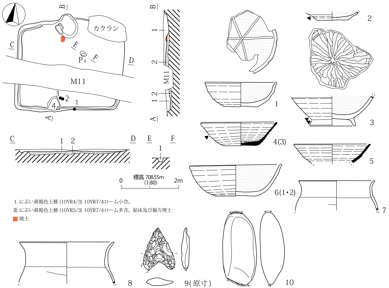
第521図 H338号住居址
