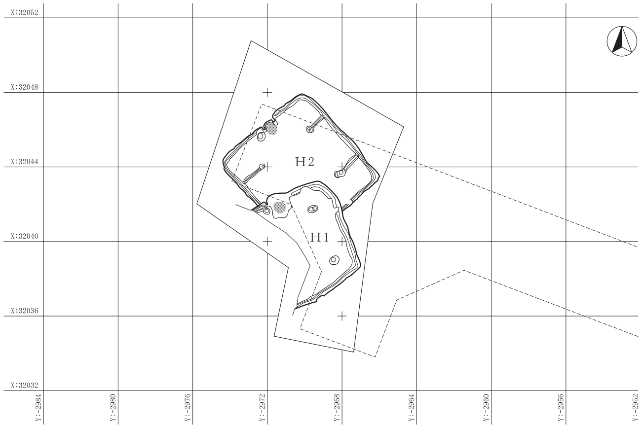
遺構配置図(1:200)
