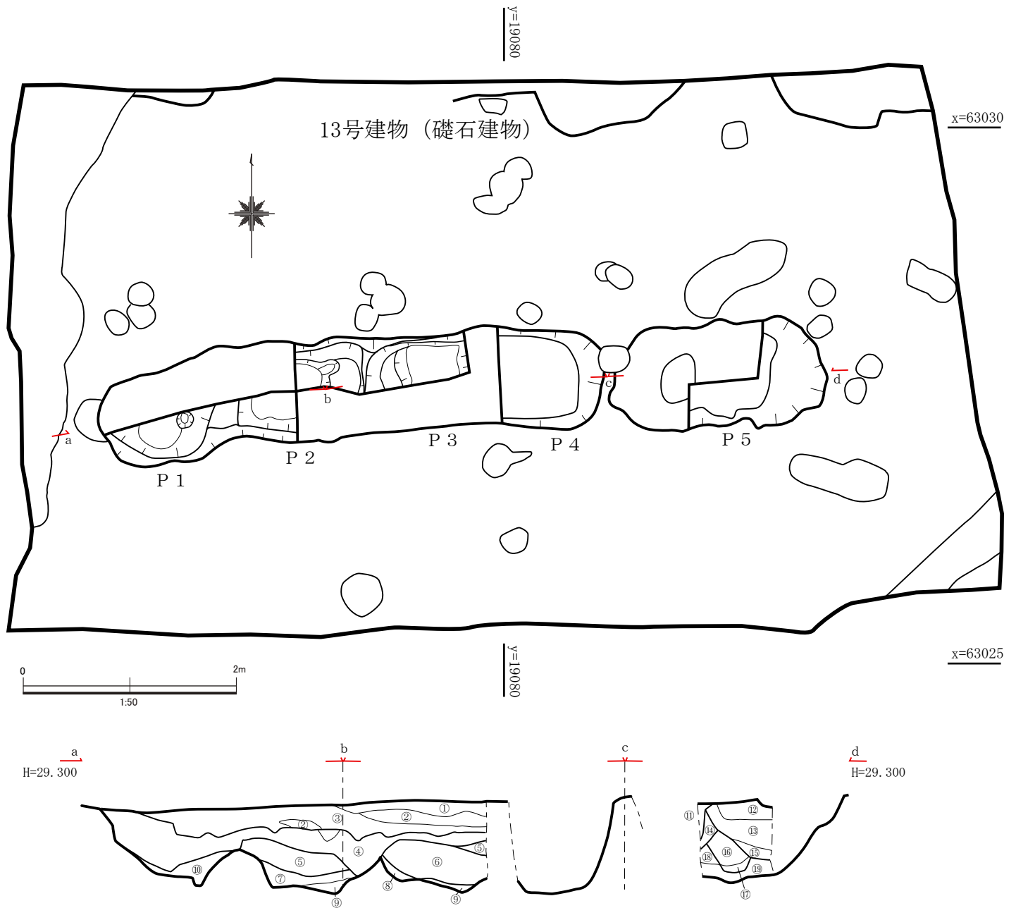
第22図 長者屋敷官衙遺跡13号建物南溝平面図・堆積状況図 (S=1/50)
