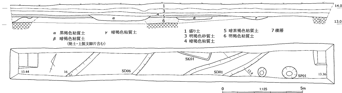
Fig.5 北トレンチ実測図
