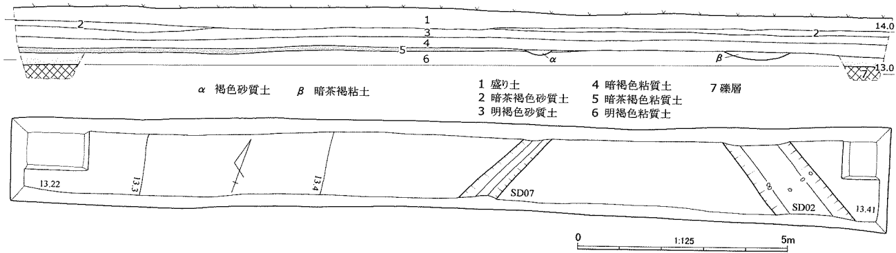
Fig.7 南トレンチ実測図
