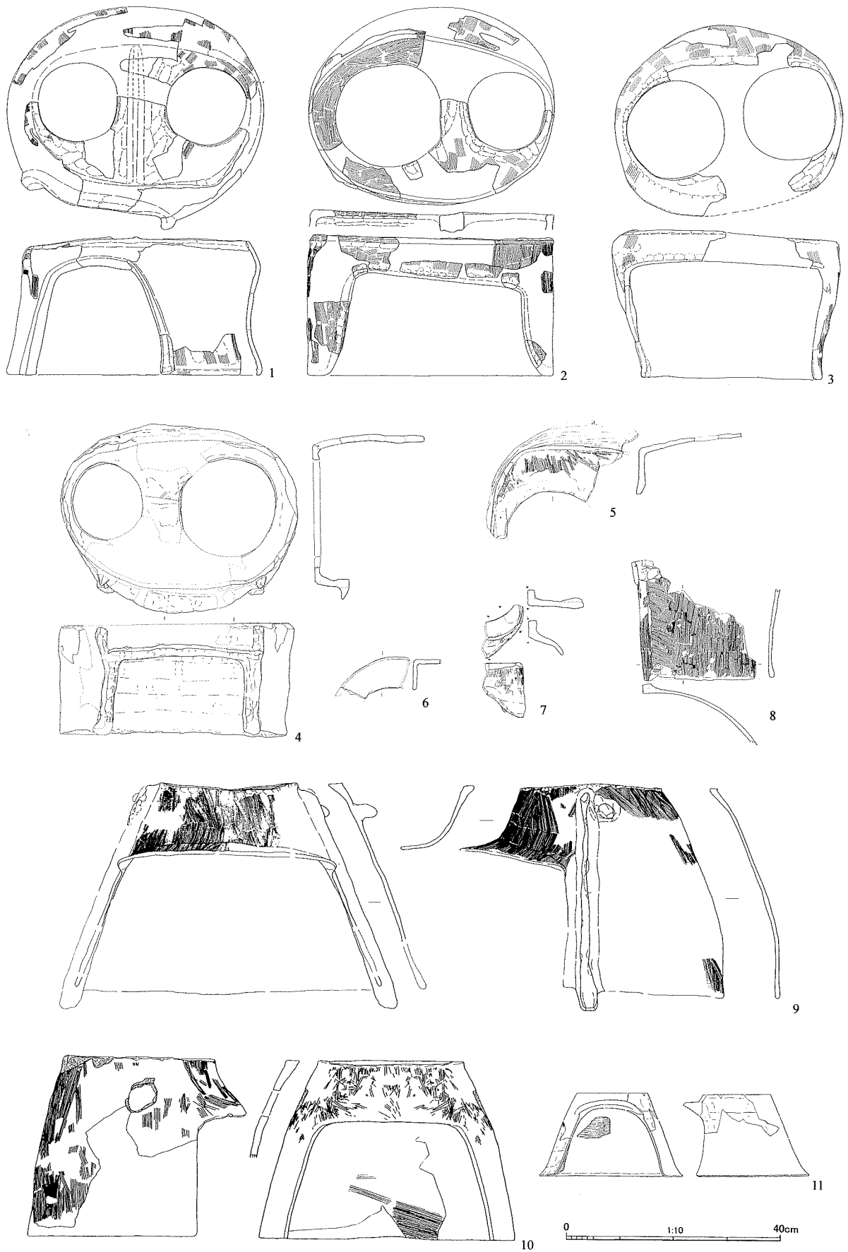
Fig.16 移動式窠集成 (1~3: 西畑屋 4~8: 下滝 9: 江古山 10: 梅坪 11: 笠井若林)
