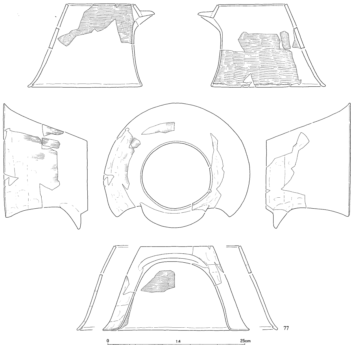
Fig.14 SD03出土移動式竈
