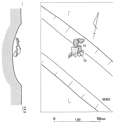
Fig.9 SD03移動式竈出土状態
