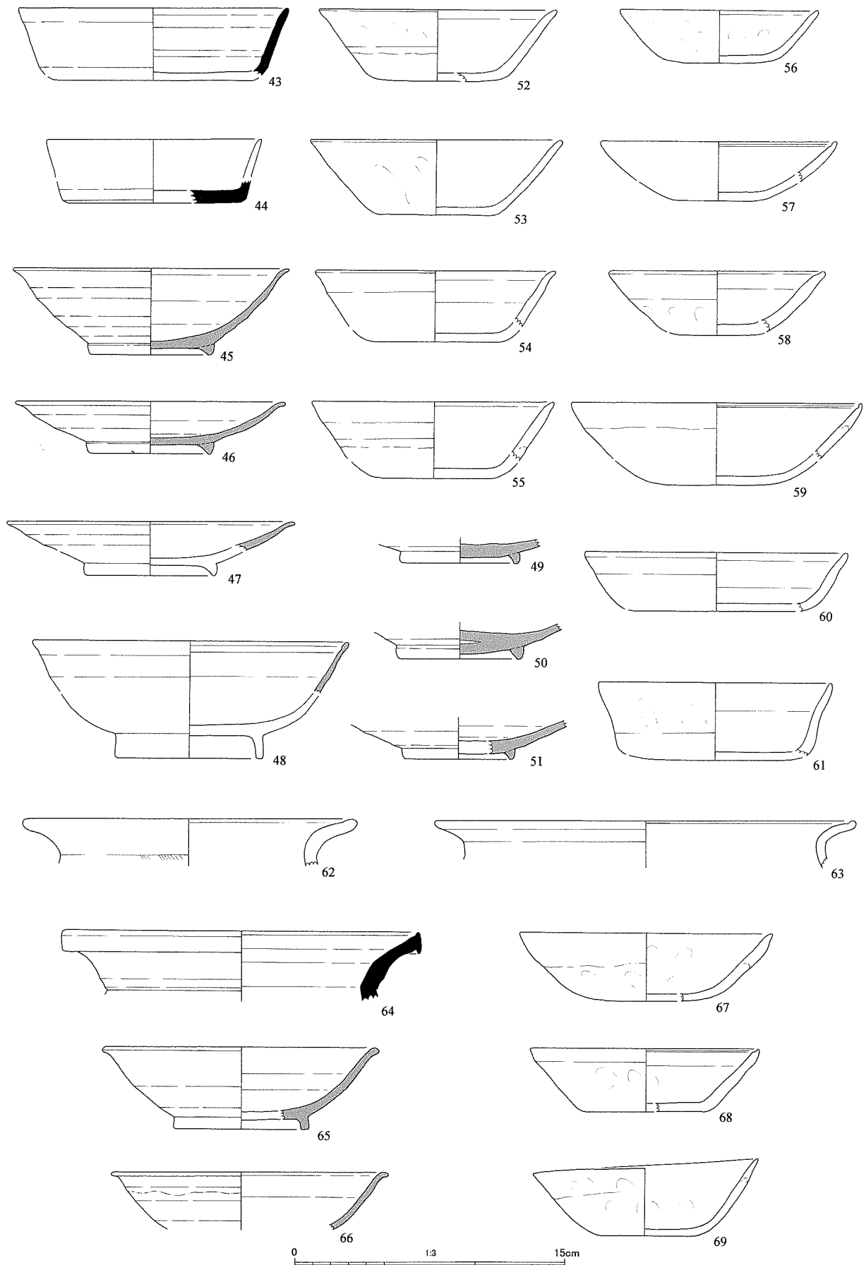
Fig.12 南トレンチ出土遺物 (43~63 : SD02 64~69 : 包含層)
