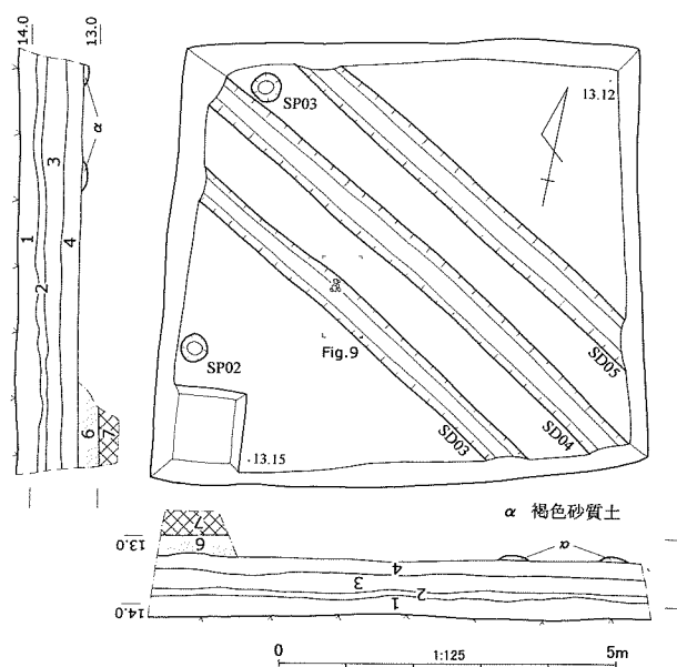
Fig.8 南西別区実測図
